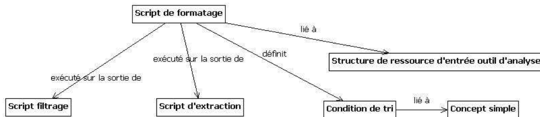
Figure 58 Script relatif à l'opération de formatage
