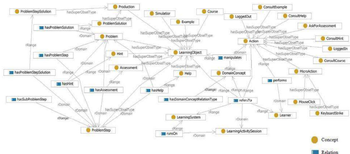
Figure 5 Modèle RDF de la trace d'activité d'apprentissage individuel (LATM) (Settouti et al., 2010)
