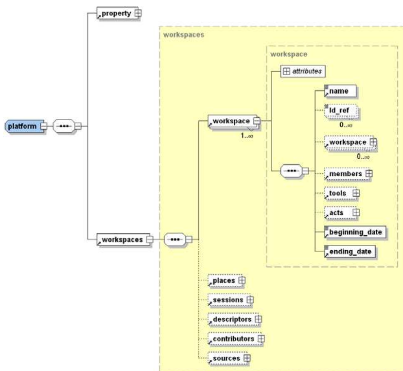
Figure 21 Extrait du schéma XML du format des traces d'interaction proposé (Reffay et al., 2008)
