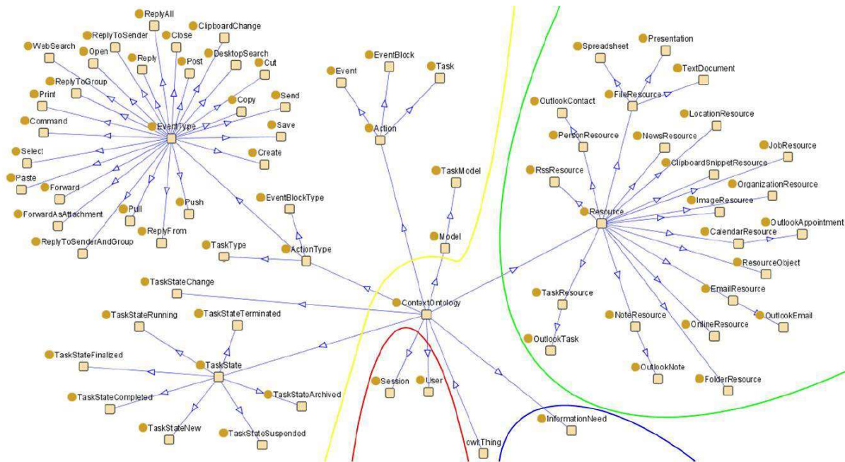
Figure 13 Les concepts des quatre dimensions de l'ontologie UICO
