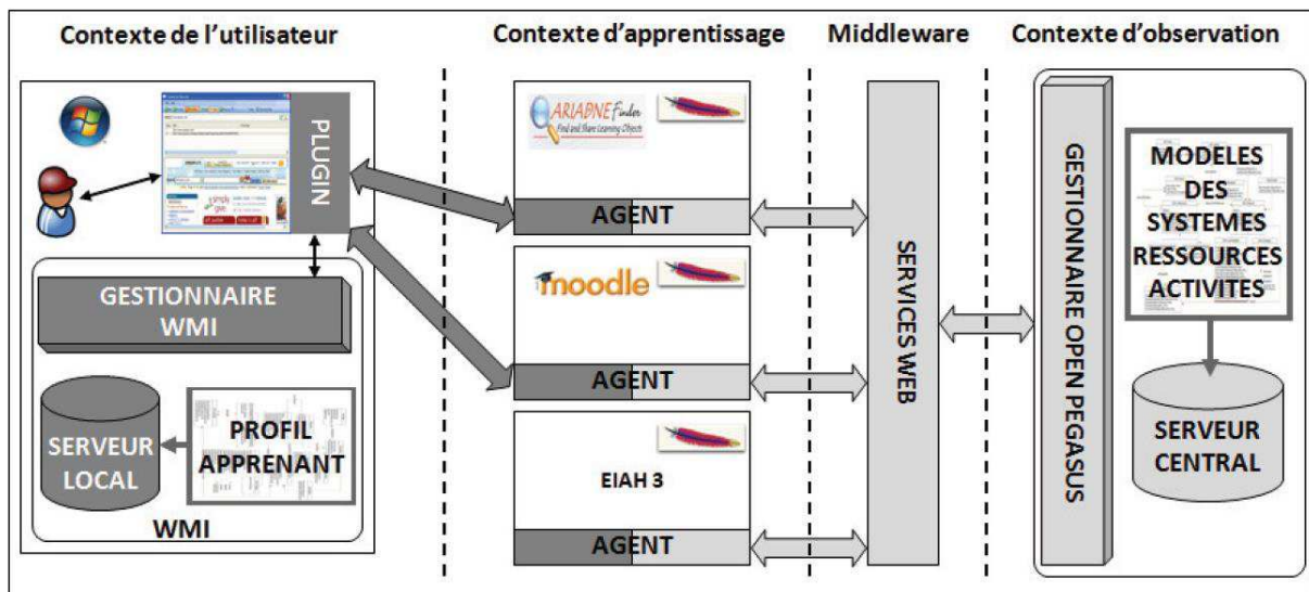
Figure 11 Architecture basée sur le standard CIM pour la collecte et le partage des CAM (Butoianu et al., 2011)
