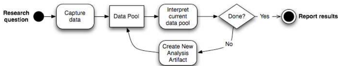
Figure 6 Modèle du processus d'analyse de TATIANA (Dyke, 2009)
