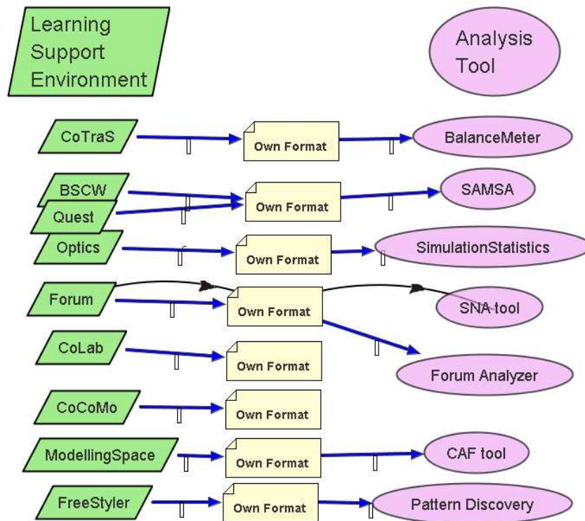
Figure 14 Situation initiale - outils d'analyse fortement couplés aux environnements d'apprentissage (Martínez et al., 2005)
