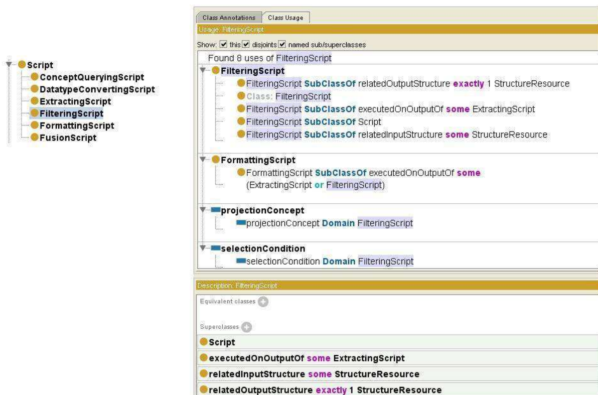
Figure 68 Extrait du modèle opérationnel formalisé par l'ontologie – formalisation du concept « script de filtrage » (visualisé à l'aide de l'éditeur d'ontologie Protégé)
