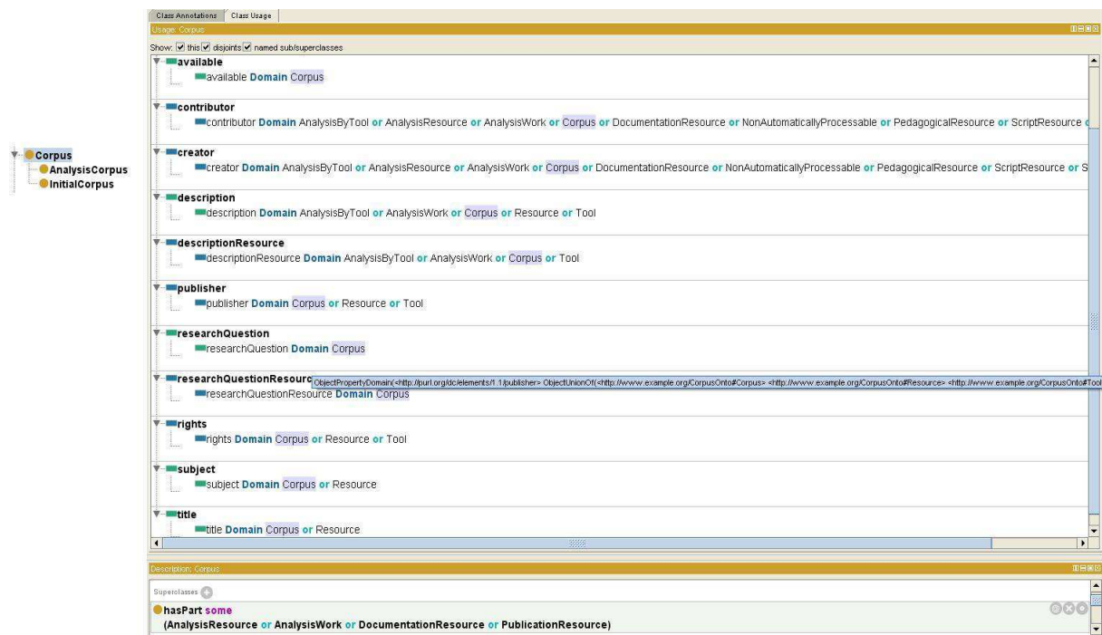
Figure 65 Extrait du modèle de corpus formalisé par l'ontologie (visualisé à l'aide de l'éditeur d'ontologie Protégé)
