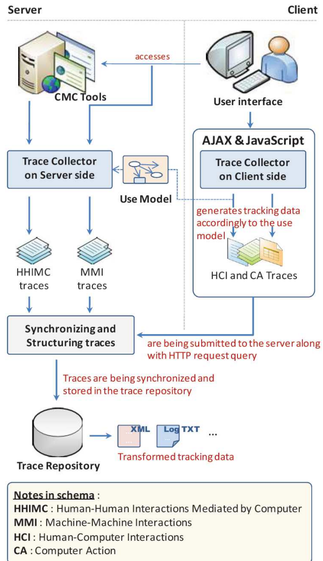
Figure 8 Architecture web du système de traçage côté client et serveur (May et al., 2008)
