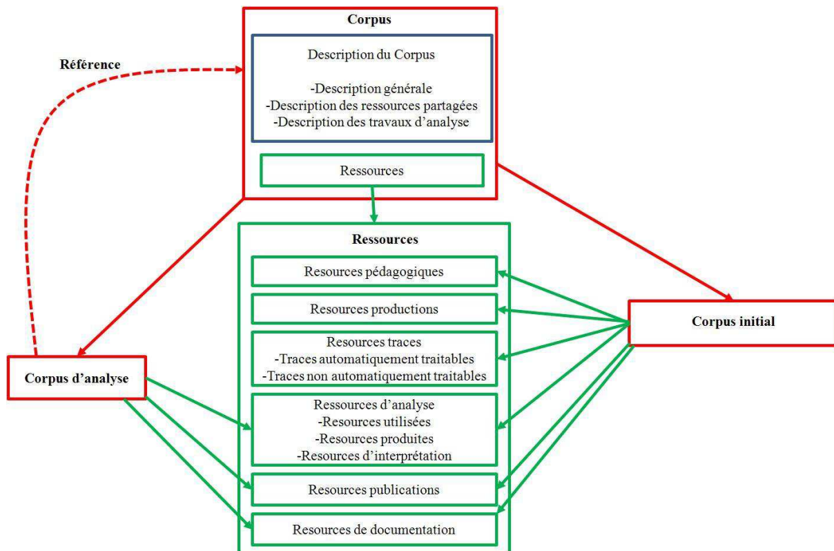
Figure 30 Structure des corpus partagés : corpus initial et corpus d'analyse
