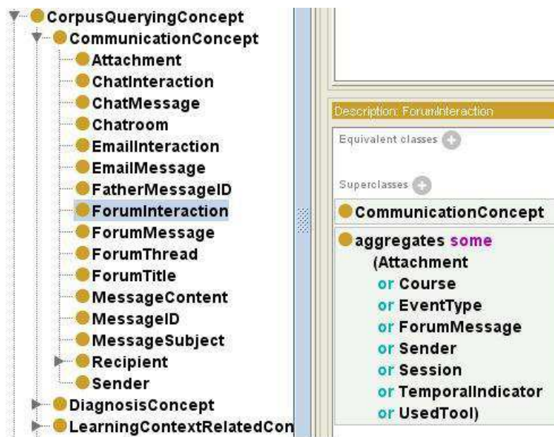
Figure 89 Extrait du modèle sémantique : définition du concept complexe « interaction de forum » comme l'agrégation de concepts complexes et de concepts simples
