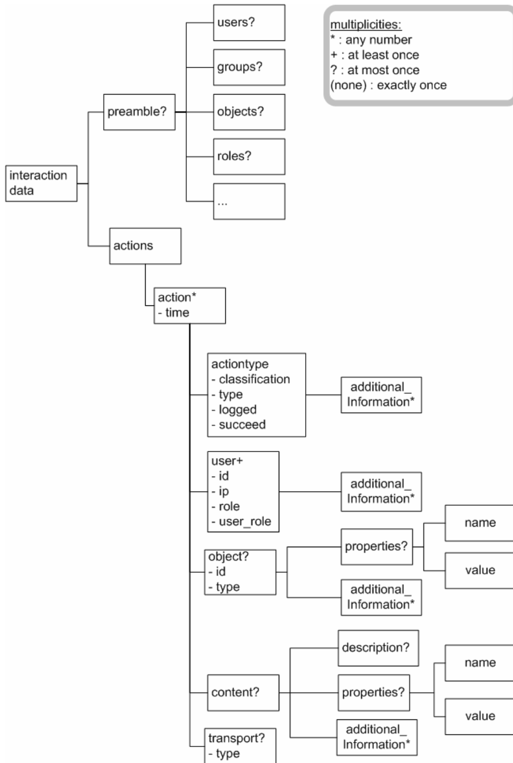
Figure 15 Partie de la DTD du format commun (Martínez et al., 2005)
