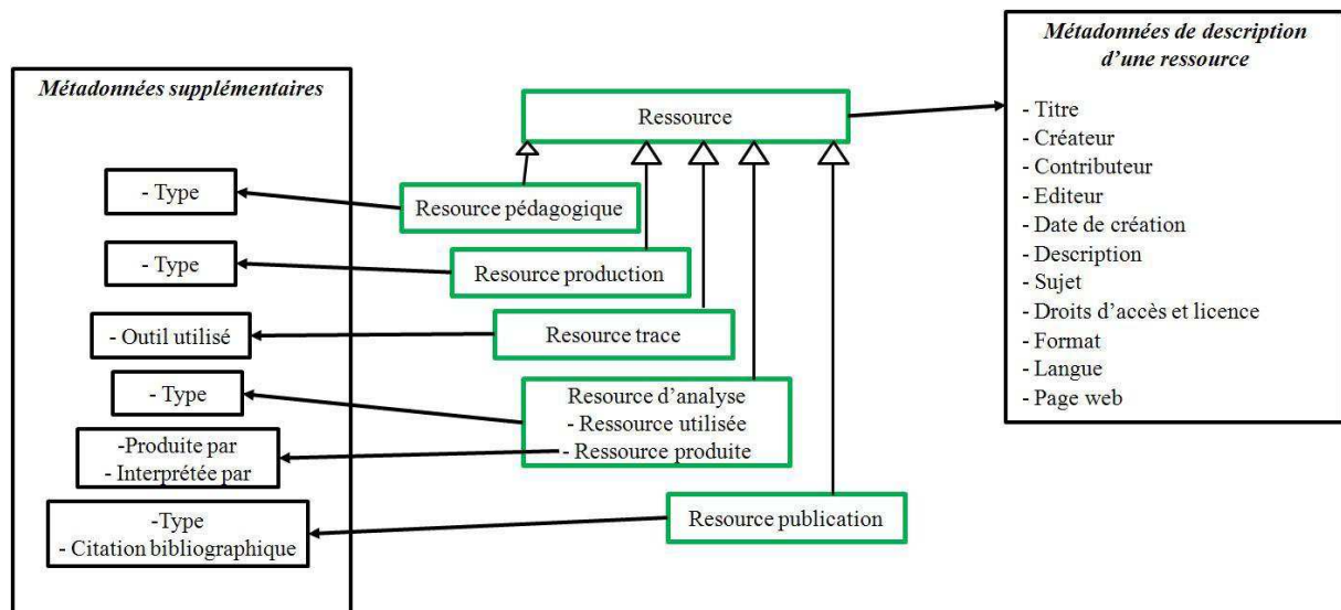
Figure 37 Métadonnées de description des ressources
