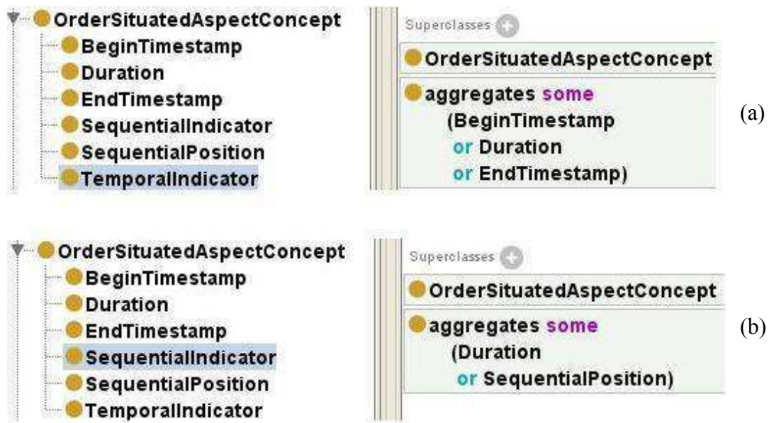
Figure 41 Concepts relatifs à l'aspect situé des interactions tracées
