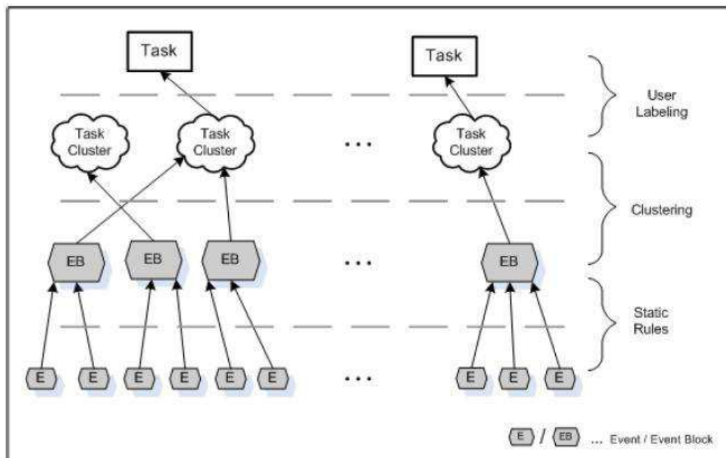
Figure 12 Pyramide sémantique: représentation conceptuelle des relations entre événements, blocs d'événements, et tâches pour la détection du contexte
