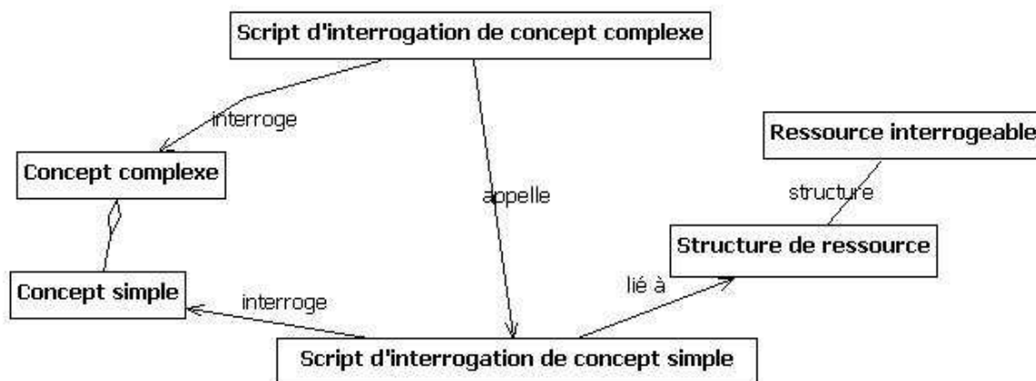
Figure 49 Script relatif à l'opération d'interrogation de concept
