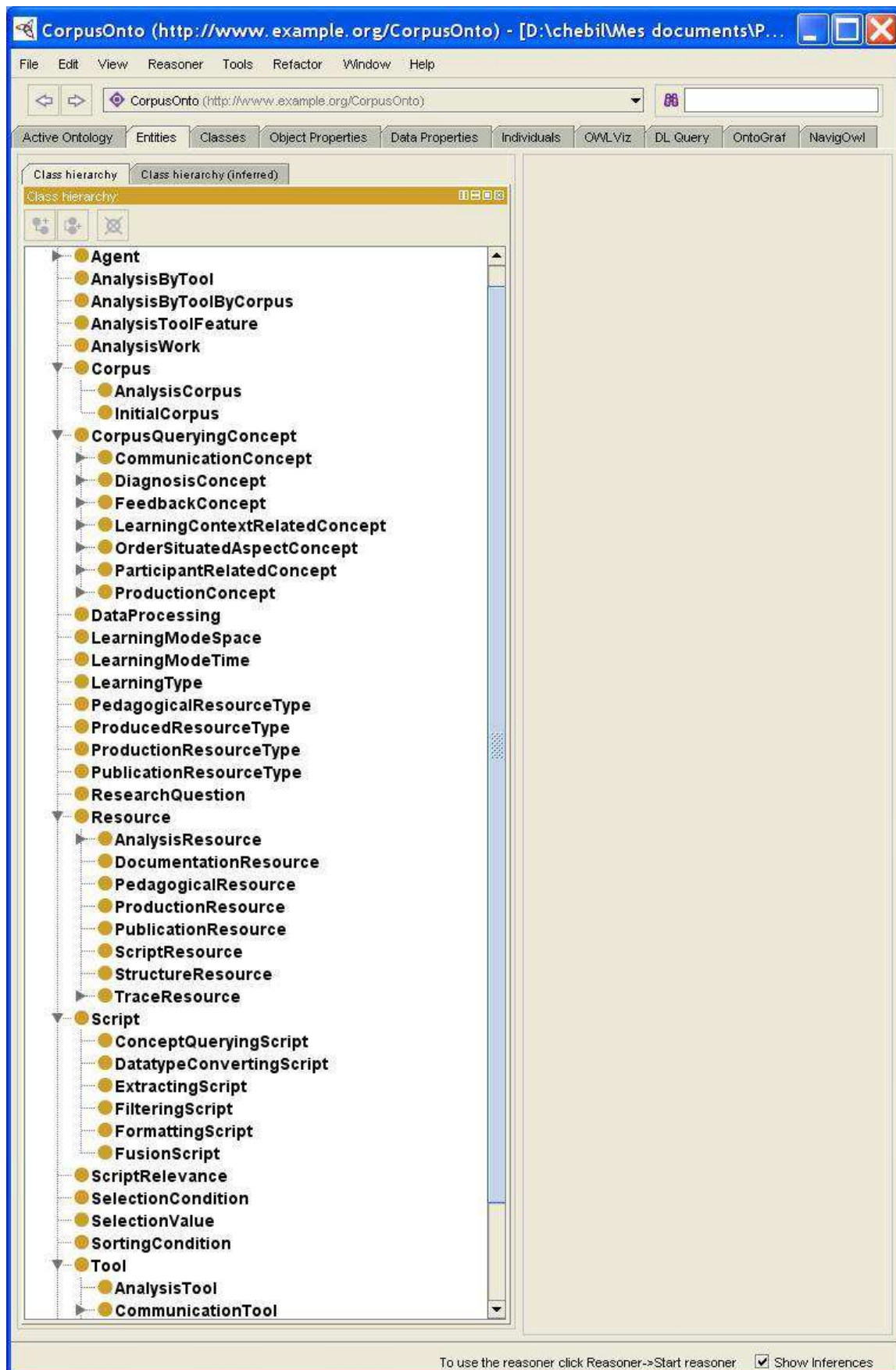
Figure 101 Aperçu de l'ontologie dans l'éditeur Protégé
