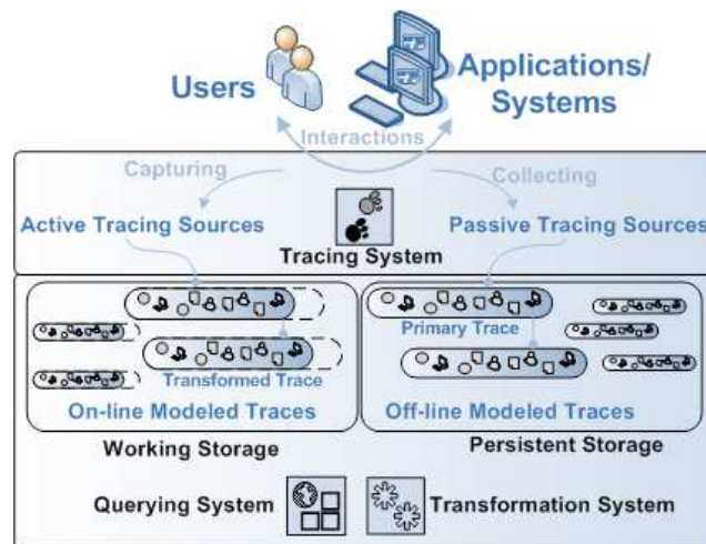
Figure 2 Architecture d'un Système à Base de Trace (Settouti et al., 2009)
