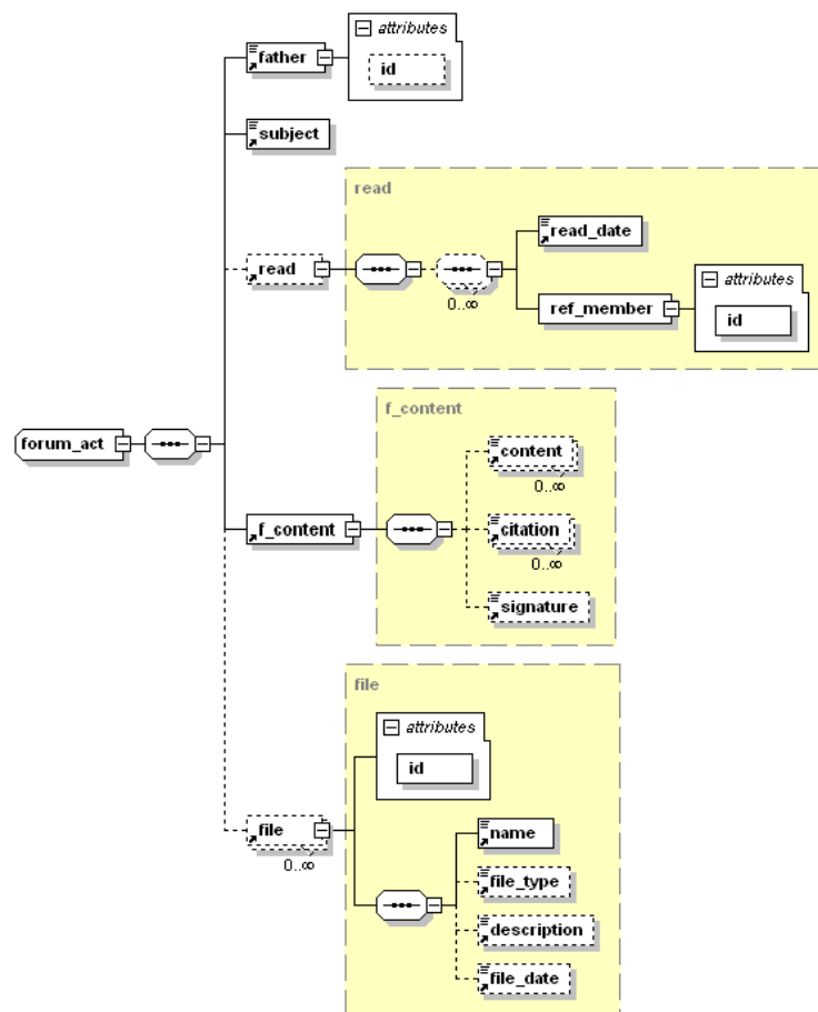
Figure 23 Extrait du schéma XML, Concept d'acte de forum (Reffay et al., 2008)
