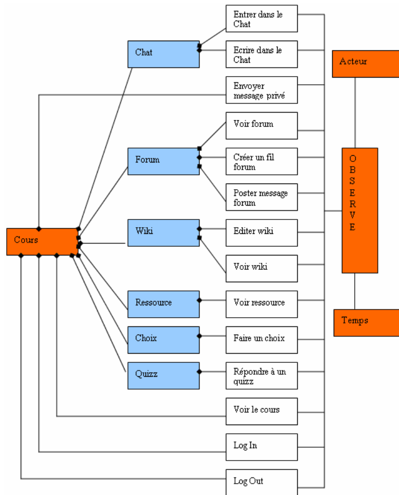
Figure 3 Ontologie pour le modèle d'utilisation de la trace
