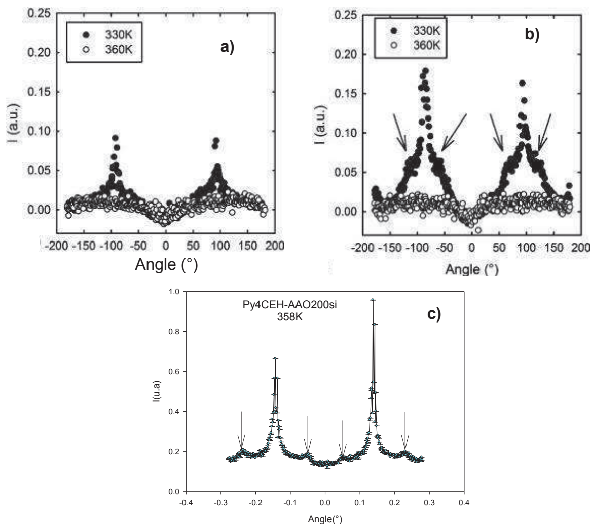
Figure IV.21: Représentation azimuthale de l'intensité intégrée de diffusion du Py 4 CEH confiné dans les a) AAO 50, b) AAO 50-CH 3 (greffée) et c) AAO200-CH 3 (greffée). Les flèches verticales indiquent les pics supplémentaires de la symétrie hexagonale (épaulement).
