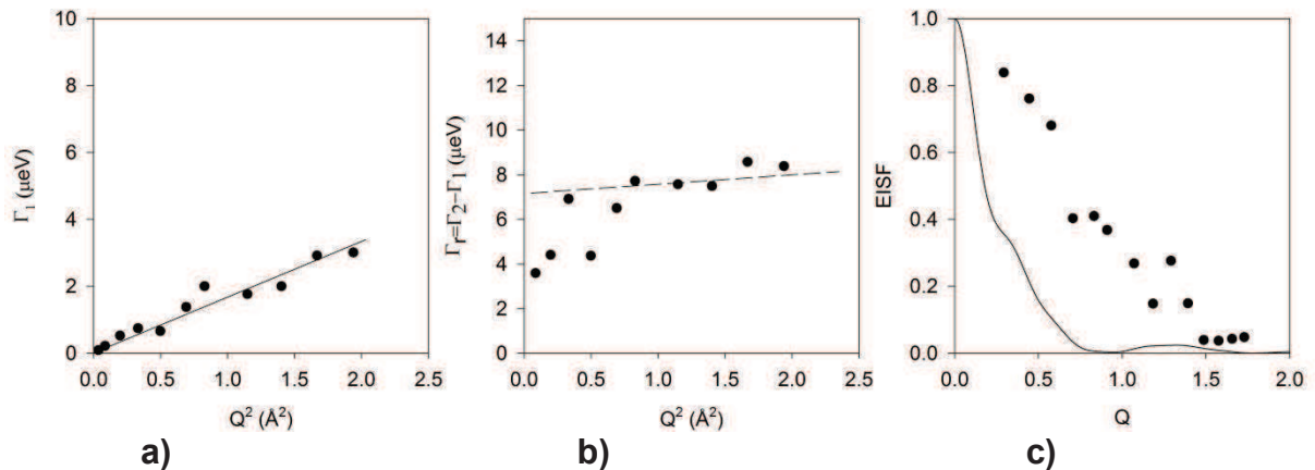
Figure V.4: Demi-largeur à mi-hauteur des deux fonctions lorentziennes fittant les données de BS sur le Py 4 CEH bulk dans la phase isotrope. a) FWHM de la ligne attribuée au processus de diffusion translationnelle; b) FWHM et c) l'EISF de la ligne attribuée à un deuxième processus localisé. La ligne pleine en (c) représente une moyenne de l'EISF théorique attendu pour une rotation isotrope de la molécule.
