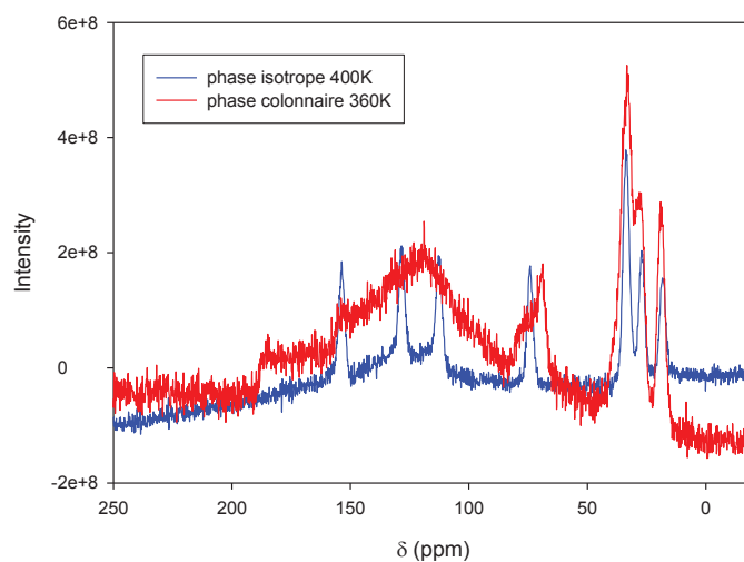
Figure IV.12 : Spectres ^{13}\text{C} du HPT confiné dans AAO statique découplé à T= 360\text{K} en phase colonnaire (courbe rouge) et statique et découplé à T= 400\text{K} dans la phase isotrope (courbe bleue).
