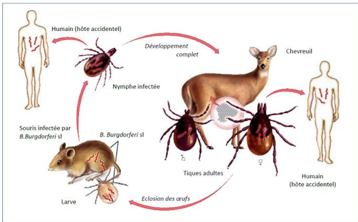
Figure 3 : Cycle de développement de la tique et acquisition de l'infection (d'après Talaro, 2005)
