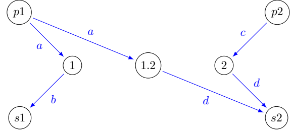
FIGURE 1.12 – Clôture mixte
