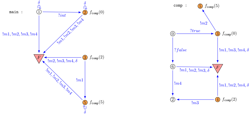
FIGURE 7.2 – Exemple d'un testeur canonique.
