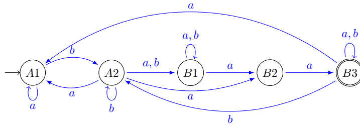
FIGURE 1.6 – Itération de l'automate représenté en figure 1.5
