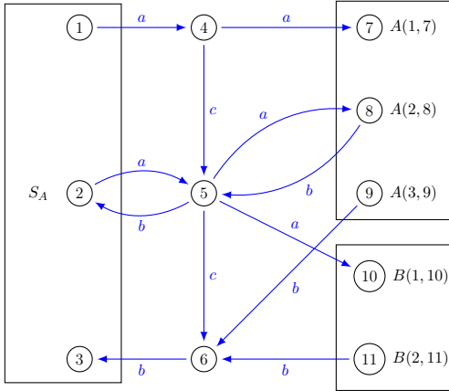
FIGURE 5.1 – Axiome du RTS de l'exemple 17.
