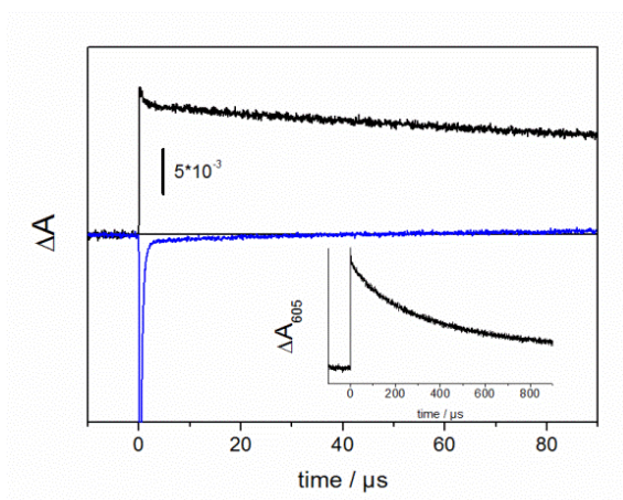
Figure 10: Absorption transitoire à 605 (noir) et 450 nm (bleu) du Ru-Trp dans une solution de MeCN/H 2 O (50:50) saturée à l'argon et en présence de 10 mM MV 2+ comme accepteur externe d'électron, suite à une excitation par une lumière flash nanoseconde à 460 nm. Figure en insert: cinétique à 605 nm enregistrée sur un temps plus long.
