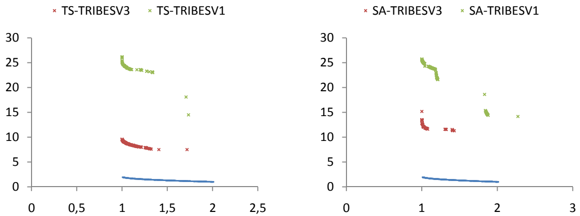
Figure 4.17 : Fronts de Pareto pour la fonction R_ZDT4
