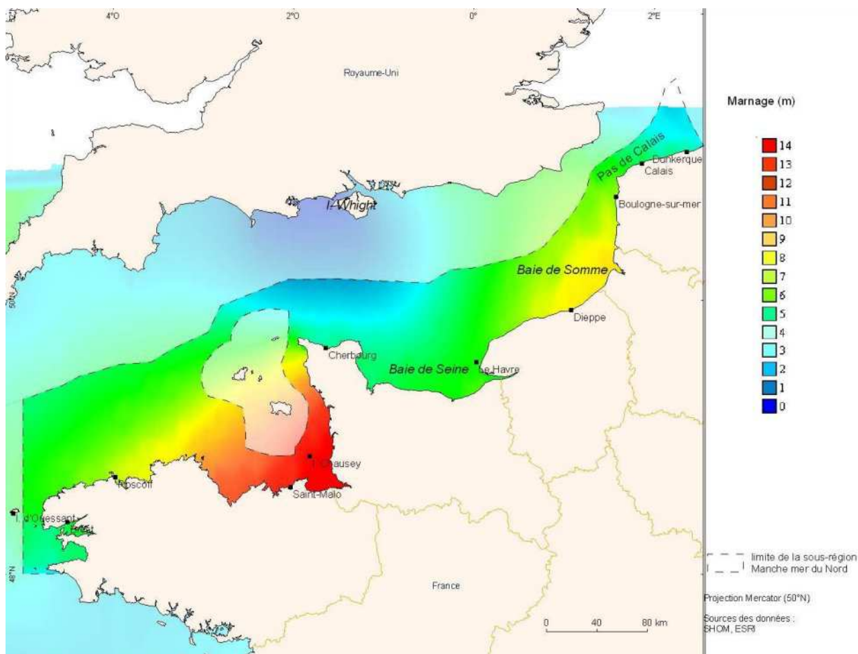
Fig. 1.3. Marnage en Manche (issu du modèle de marée CSTFRANCE).
