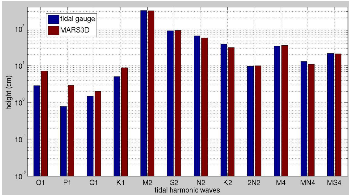
Fig. 2.5 -Comparaison entre le modèle et le marégraphe des amplitudes de 12 harmoniques du signal de marée pour le port de Boulogne sur mer.
