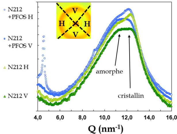
FIGURE 4.17 – Spectres de WAXS mesurés sur ID13 du Nafion 212 dopé (bleu) ou non (vert). Les données sont regroupées en secteurs H et V, comme indiqué sur l'image 2D.
