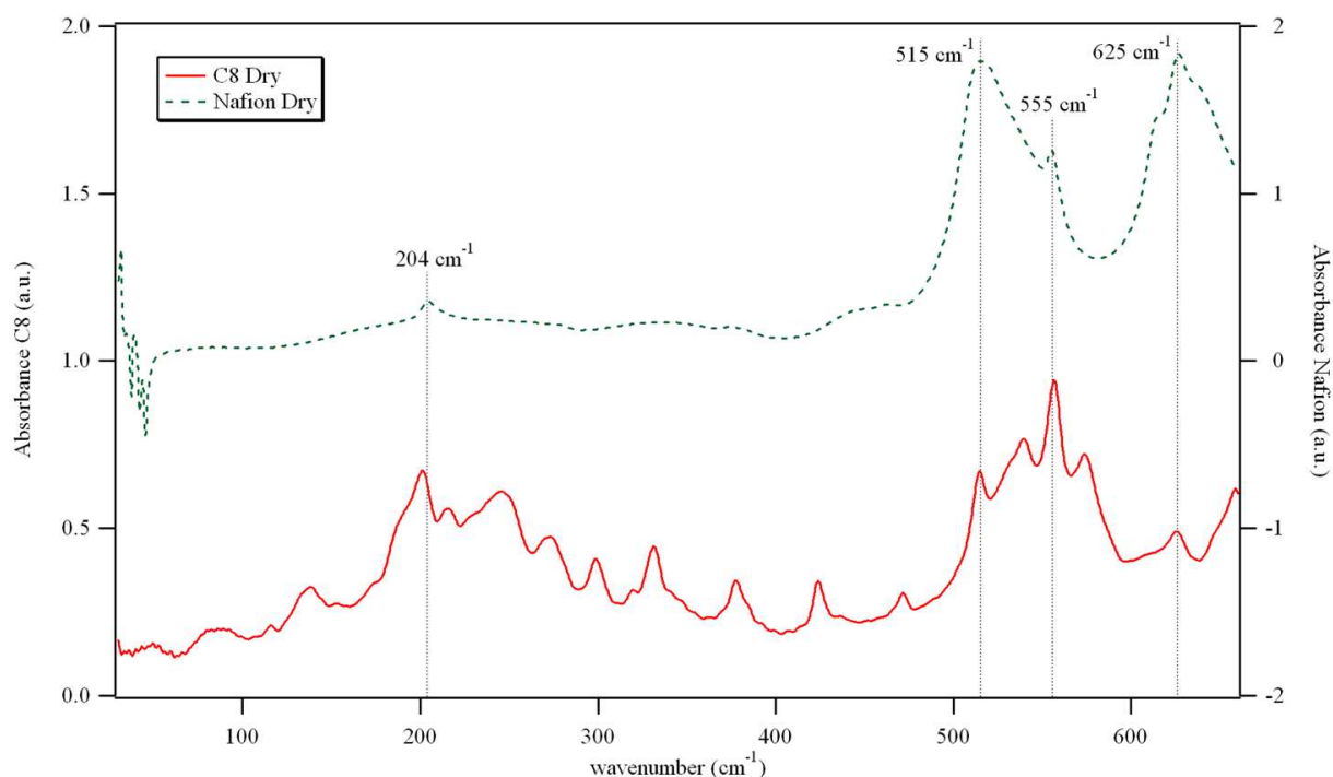
FIGURE 5.8 – Spectres IR du PFOS 95% comparé au Nafion séché à 60^{\circ}C . Bandes communes : 204\text{ cm}^{-1} rocking CF_2 ; 515\text{ cm}^{-1} bending OSO du groupe SO_3^- ; 555\text{ cm}^{-1} bending CF_2 ; 625\text{ cm}^{-1} wagging CF_2
