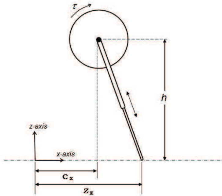
Figure 6.9: Le modèle de pendule inversé linéaire avec un volant d'inertie pour prendre en compte les effets inertiels du haut du corps
