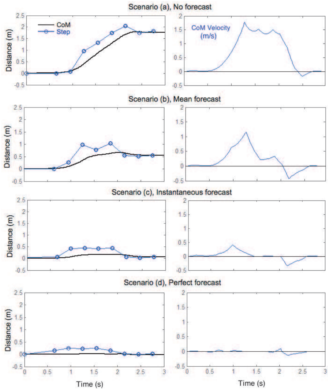
Figure 6.15: Rattrapage d'équilibre pour une perturbation longue selon 4 modalités d'anticipation de la perturbation de qualité croissante : évolution temporelle de la position (gauche - noir) et de la vitesse (droite - bleu) du CdM, ainsi que position des pas (gauche, point bleus).
