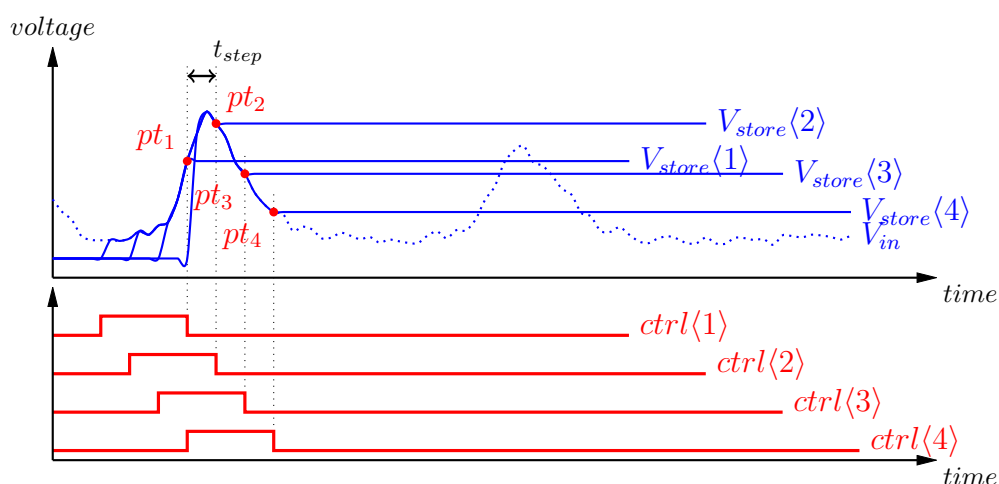
Figure 10.13 – Principe de l'échantillonnage avec un groupe de quatre cellules. Ici 4 cellules sont reliées et contrôlées par quatre signaux de commande identique décalée dans le temps par t_{step} .
