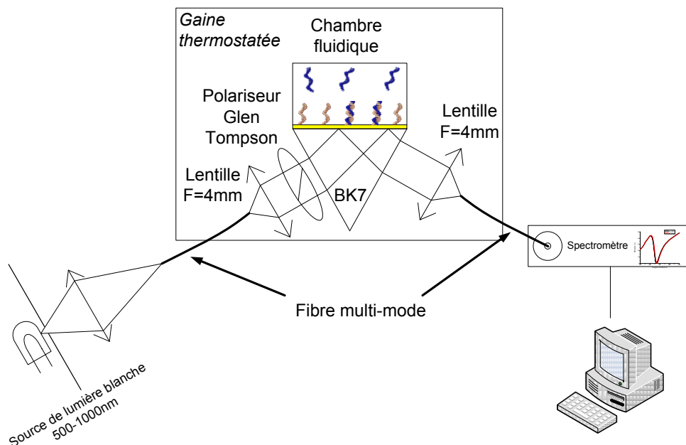
Figure 3.22 Schéma du système SPR spectroscopique proposé pour coupler la microcalorimétrie. Il y a seulement le prisme, deux lentilles pour collimater le faisceau et couplées dans les fibres et le polariseur qui doivent être dans la gaine thermostatée. La source de lumière blanche ainsi que le spectromètre de mesure peuvent être à l'extérieur de la gaine.
