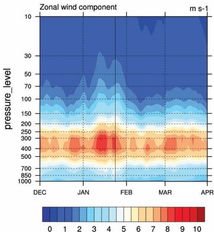
Figure 13: Coupe temps-pressure de la dispersion d'ensemble (écart-type inter-membres) sur le vent zonal polaire, sur la période décembre 2009 à mars 2010. La ligne verticale noire représente la date de début d'affaiblissement du vortex stratosphérique polaire.
