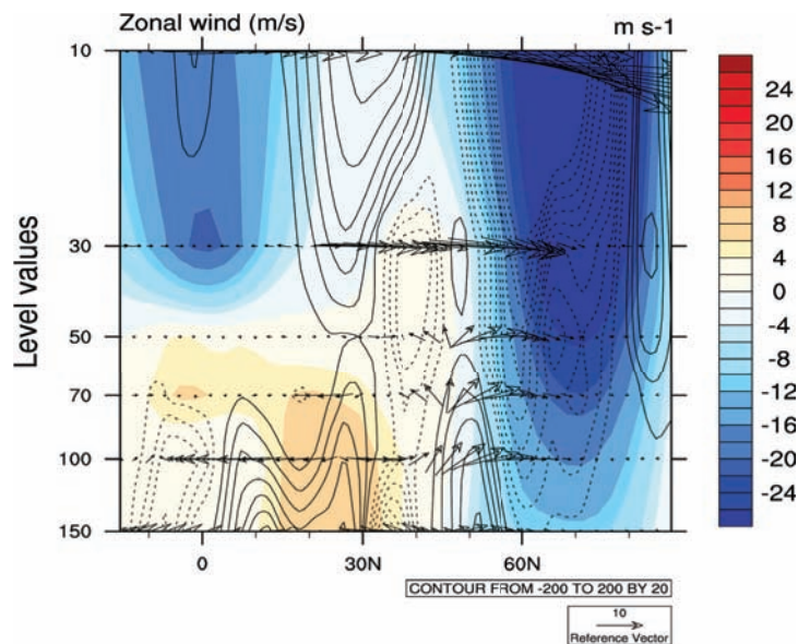
Figure 4: Anomalies de flux d'Eliassen-Palm (flèches noires, en m^2/s^2 ) au cours du réchauffement stratosphérique soudain. Les contours noirs représentent la divergence des flux (la convergence \nabla F négative est en pointillés, et indique un ralentissement du vent). L'anomalie du vent zonal en moyenne zonale est représentée en plage colorée. Données Era-Interim.
