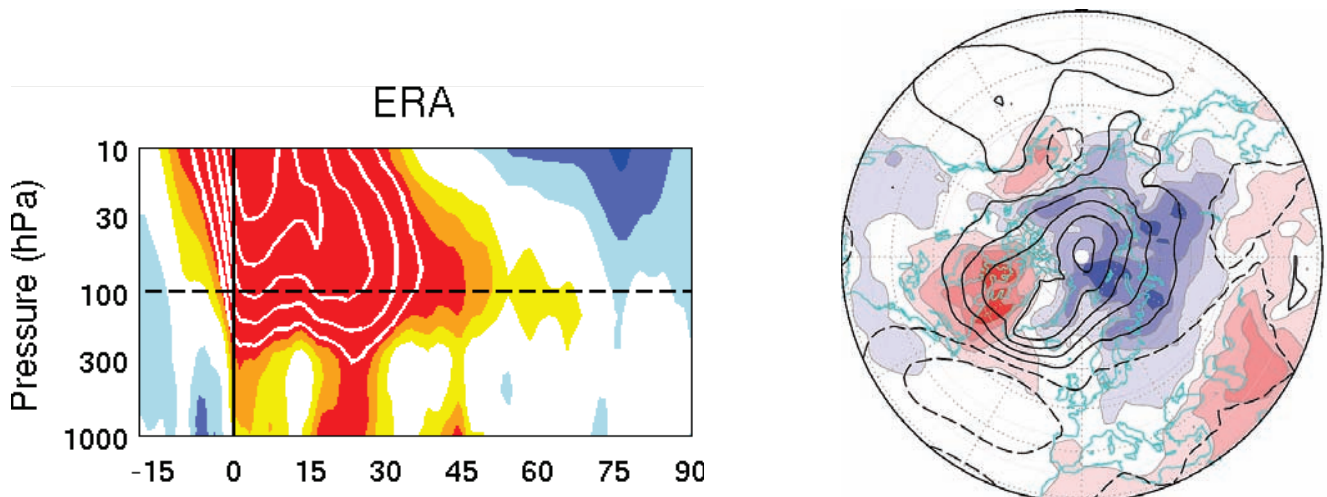
Figure 17: Signature des réchauffements stratosphériques soudains (RSS) sur la troposphère: a) Coupe temps-pression des composites du mode annulaire après les RSS; b) Composites des champs de température de surface (plages colorées) et de pression au niveau de la mer (contours noirs) observés en moyenne dans les deux mois suivant les RSS. D'après M. Sigmond, Workshop SSW du 24 février 2012, article en préparation.
