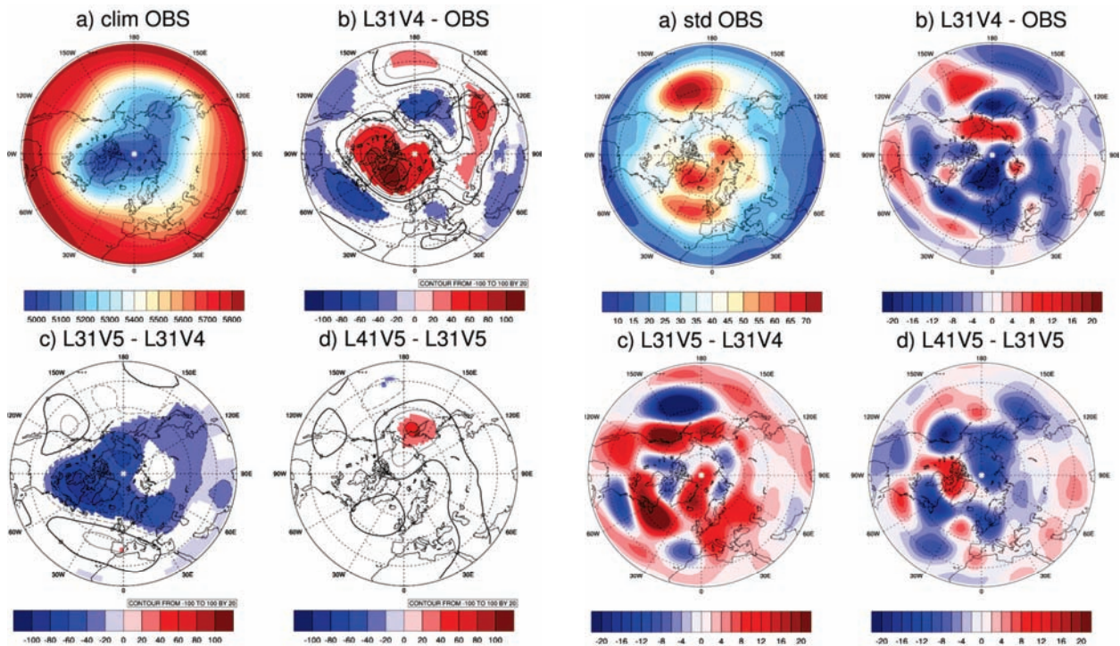
Figure 5: Erreur sur la moyenne du géopotentiel à 500hPa dans l'hémisphère nord - Climatologie DJF . Test de significativité à 99% .
