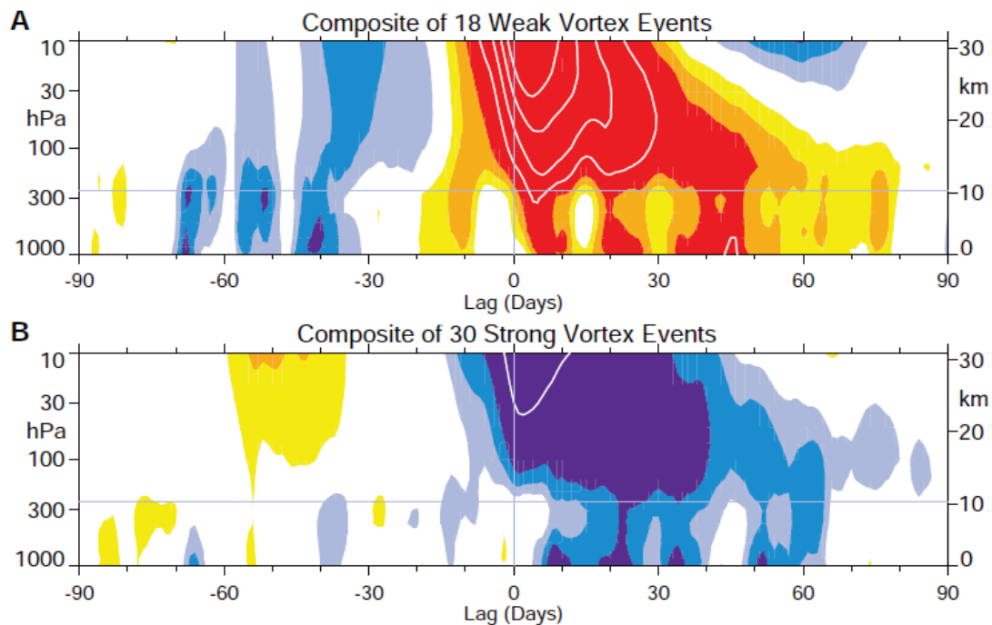
Figure 15: Coupes temps-pression des composites du mode annulaire pour (A) 18 événements "vortex faible" et (B) 30 événements "vortex fort". Les événements sont déterminés par les dates pour lesquelles le mode annulaire à 10 hPa dépasse les écart-types 3.0 et 11.5, respectivement. Les indices sont adimensionnalisés; l'intervalle de contour pour les plages colorées est de 0.25, et de 0.5 pour les contours blancs. Les valeurs entre 20.25 et 0.25 ne sont pas tracées. La ligne horizontale indique la limite approximative entre la troposphère et la stratosphère (d'après Baldwin et Dunkerton 2001).
