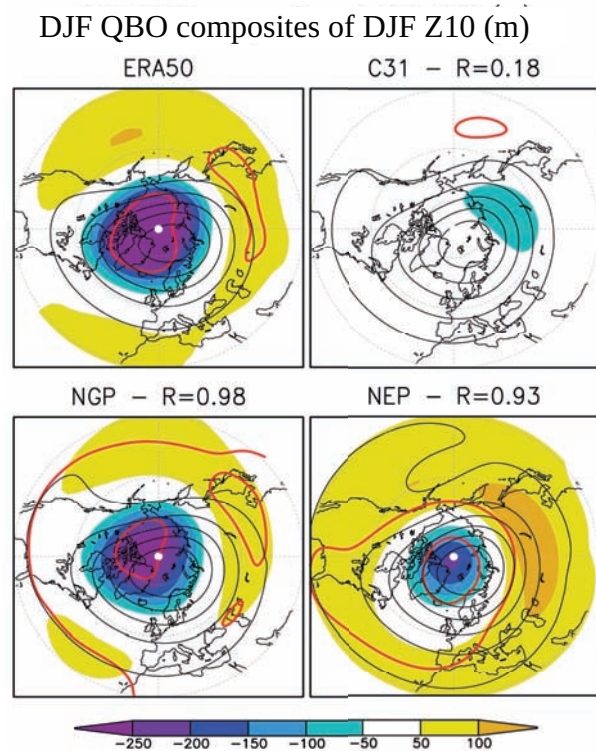
Figure 20: Composites DJF du géopotentiel à 10 hPa pour les réanalyses et les moyennes d'ensemble des expériences C31, NGP et NEP. La climatologie est représentée en contours noirs. Les anomalies significatives à 90 % sont délimitées par un contour rouge épais. R est le coefficient de corrélation entre les ensembles et les réanalyses.
