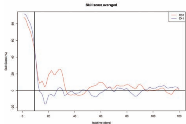
Figure 10: Skill score quotidien (en %) tel que défini par Roff et al. (2011) pour les expériences C41 (en bleu) et C31 (en rouge) par rapport au skill score climatologique, calculé sur le géopotential à 10 hPa sur le domaine "North Polar Cap", en fonction des jours.
