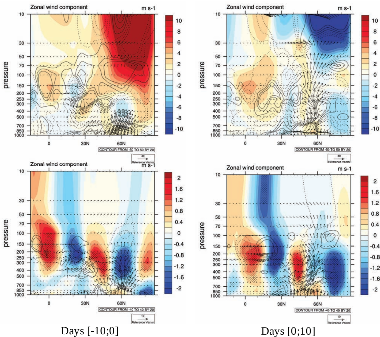
Figure 16: En haut : Flux d'Eliassen-Palm pour les membres « propagatifs » en moyenne 10 jours avant le RSS (à gauche) et 10 jours après le RSS (à droite). En bas : Différence de flux d'EP entre les membres "propagatifs" et "non propagatifs". Différence de vent zonal en plages colorées, significativité à 90% en pointillés.
