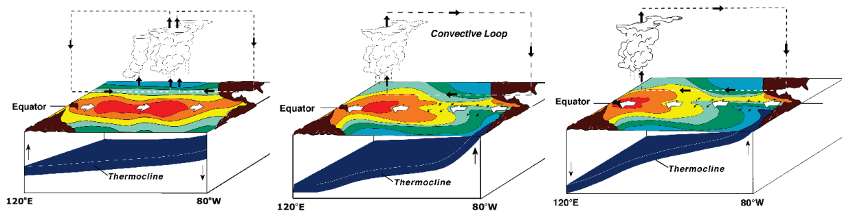
Figure 1: Représentation schématique des différentes phases de l'ENSO.
