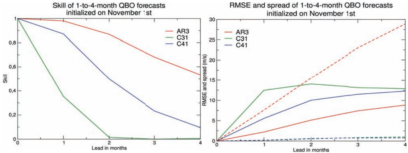
Figure 19: Scores sur l'indice QBO basé sur le vent zonal à 30 hPa moyennée sur la boîte [5^{\circ}\text{S}-5^{\circ}\text{N};180^{\circ}\text{W}-180^{\circ}\text{E}] de 1 à 4 mois d'échéance à partir du premier novembre pour le schéma auto-régressif d'ordre 3 (AR3) et les prévisions dynamiques low-top (C31) et high-top (C41): a) Corrélation avec les réanalyses du CEPMMT, b) RMSE et dispersion (en pointillés).
