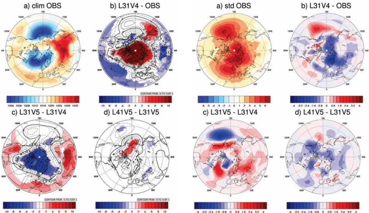
Figure 7: Erreur sur la Pmer dans l'hémisphère nord - Climatologie DJF . Test de significativité à 99% .
