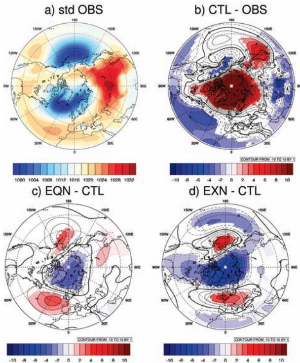
Figure 24: Biases de Pmer dans l'hémisphère nord - Climatologie DJF. Test de significativité à 99% .
