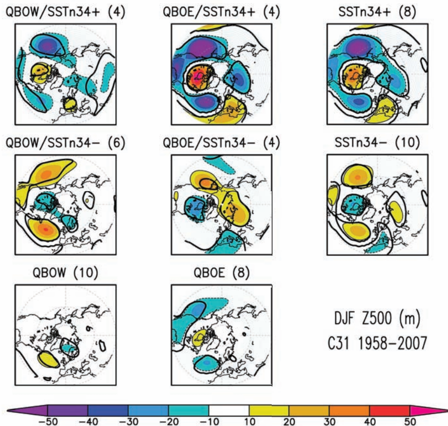
Figure 25: Double composites des anomalies hivernales (DJF) de géopotential à 500 hPa (en m) aux moyennes et hautes latitudes de l'hémisphère Nord pour l'ensemble C31, sur la base d'anomalies synchrones supérieures à un demi écart-type pour le vent zonal équatorial (5°S-5°N) à 30hPa comme indice de la QBO et les SST Niño3.4 comme indice de l'ENSO. Le trait noir épais délimite les anomalies significatives à 90%. Le nombre d'années utilisées pour chaque composite est indiqué entre parenthèses.
