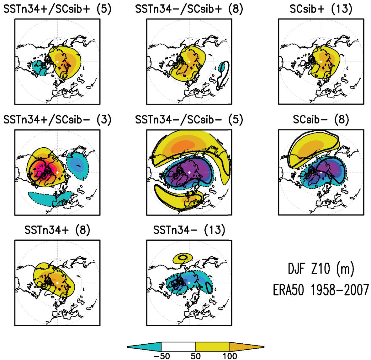
Figure 14: Double composites des anomalies hivernales (DJF) de géopotential à 10hPa (en m) aux moyennes et hautes latitudes de l'hémisphère Nord sur la base d'anomalies synchrones supérieures à un demi écart-type les SST Niño3.4 et l'étendue de la couverture neigeuse sur la Sibérie. A noter que les anomalies de SST et de neige sont moyennées sur l'automne (SON) précédent l'hiver sur lequel on moyenne le géopotential. Le trait noir épais délimite les anomalies significatives à 90%. Le nombre d'années utilisées pour chaque composite est indiqué entre parenthèses.
