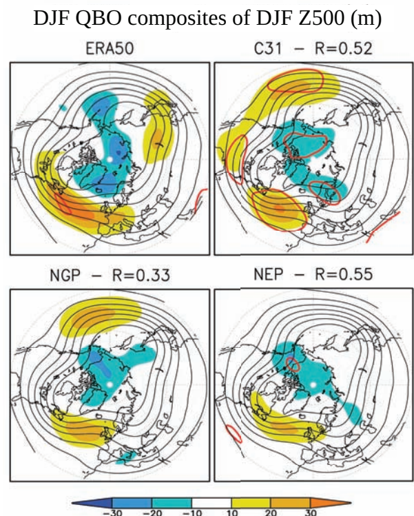
Figure 22: Composites DJF du géopotential à 500 hPa pour les réanalyses et les moyennes d'ensemble des expériences C31, NGP et NEP. La climatologie est représentée en contours noirs. Les anomalies significatives à 90 % sont délimitées par un contour rouge épais. R est le coefficient de corrélation entre les ensembles et les réanalyses.
