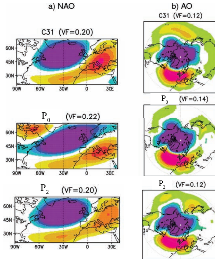
Figure 18: a) Première composante de l'EOF calculée sur la Pmer quotidienne, b) Première composante de l'EOF calculée sur le géopotential quotidien à 500 hPa, pour l'expérience de contrôle en haut, le profil P_0 au milieu, et le profil P_2 en bas.
