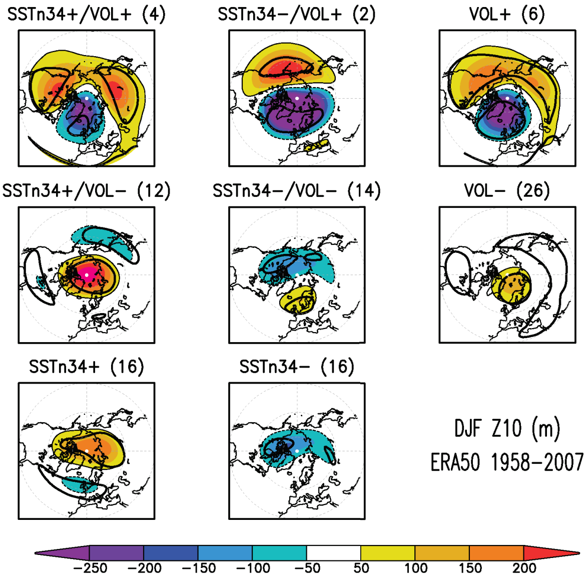
Figure 11: Double composites des anomalies hivernales (DJF) de géopotential à 10hPa (en m) aux moyennes et hautes latitudes de l'hémisphère Nord sur la base d'anomalies synchrones supérieures à un demi écart-type pour les SST Niño3.4 et selon la présence ou non d'une forte charge d'aérosols volcaniques. Le trait noir épais délimite les anomalies significatives à 90%. Le nombre d'années utilisées pour chaque composite est indiqué entre parenthèses.
