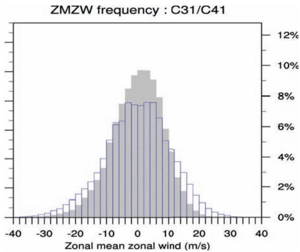
Figure 4: Distribution des anomalies quotidiennes centrées de vent zonal à 10hPa en moyenne zonale à 60°N sur la période NDJF. Expérience C31 en gris, C41 en bleu.
