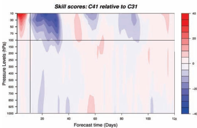
Figure 9: Skill score quotidien (en %) tel que défini par Roff et al. (2011) pour l'expérience C41 par rapport à C31, calculé sur le géopotential sur le domaine "North Polar Cap", tracé sur les niveaux pressions en fonction des jours.
