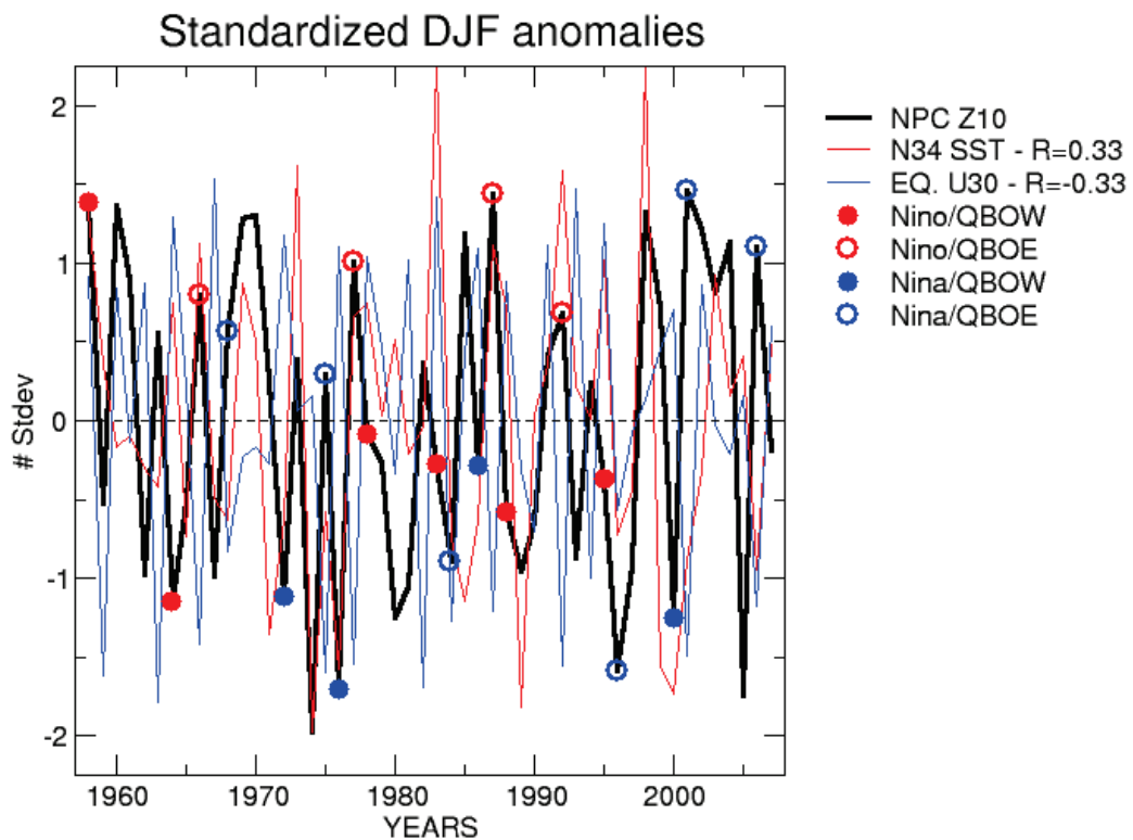
Figure 9: Anomalies hivernales (DJF) centrées et réduites (en nombre d'écart-type) pour différents indices climatiques : géopotential à 10hPa au nord de 60°N (en noir), SST Niño3.4 (en rouge), vent zonal à 30 hPa entre 5°S et 5°N (en bleu). Les symboles (cercles et disques de couleur) superposés à la courbe en noir montrent les hivers utilisés pour construire des composites du géopotential sur la base d'anomalies synchrones supérieures à un demi écart-type pour chacun des deux autres indices (ENSO et QBO).
