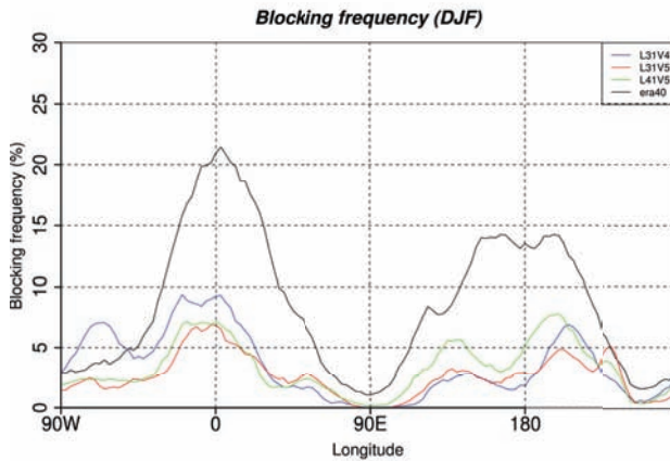
Figure 17: Fréquence de blocage (basée sur indice de Tibaldi et Molteni) en fonction des longitudes sur la période 1971-2000.
