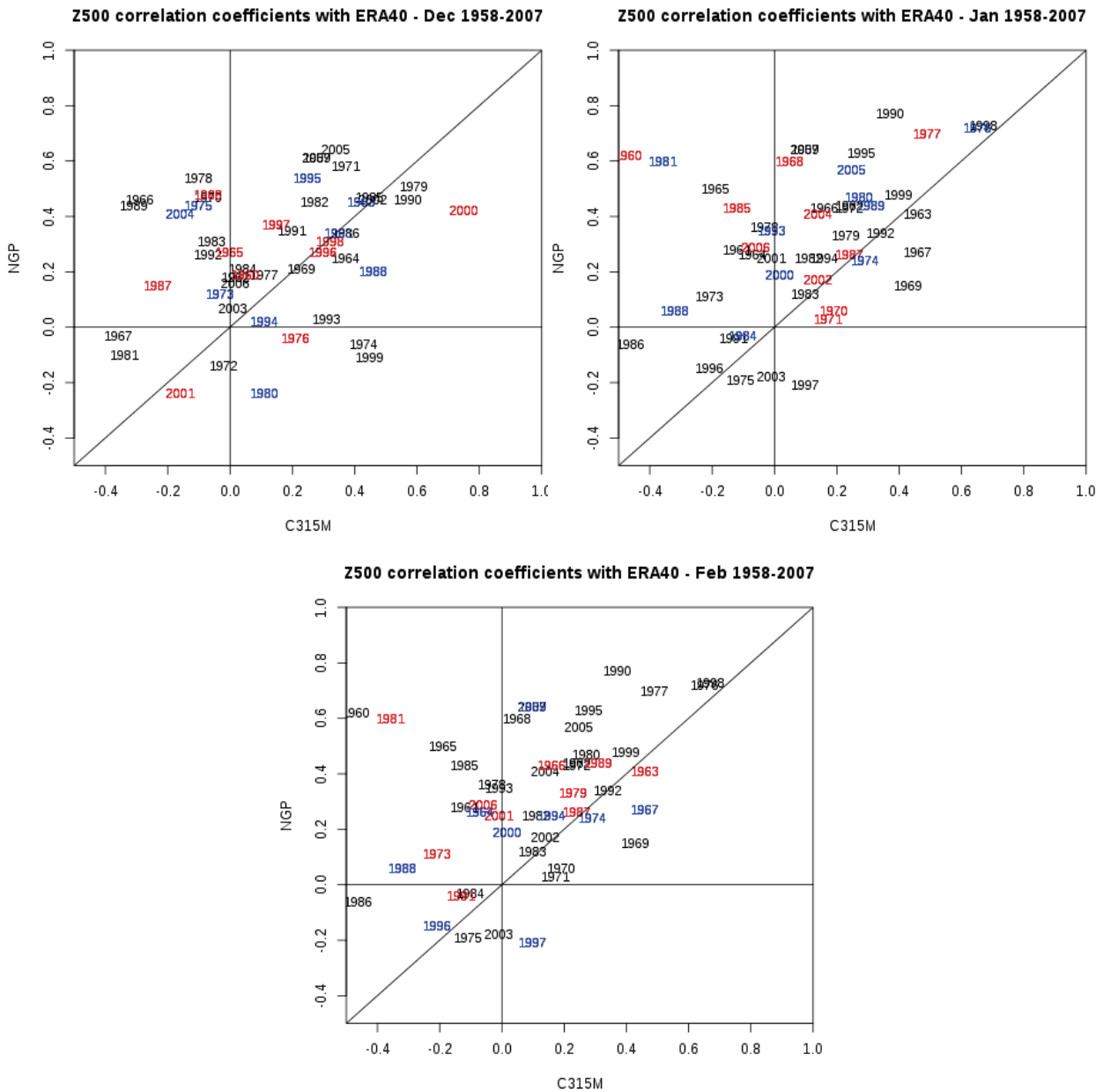
Figure 28: Scores troposphériques basés sur la corrélation entre les ensembles NGP/C31 (cinq membres chacun) et les réanalyses pour le géopotentiel à 500 hPa sur l'hémisphère nord extra-tropical, pour les mois de décembre, janvier et février sur la période 1958-2007. Les mois présentant un vortex polaire faible (tercile supérieur du géopotentiel à 10 hPa sur le domaine North Polar Cap) sont représentés en rouge, et les mois présentant un vortex polaire fort sont en bleu.
