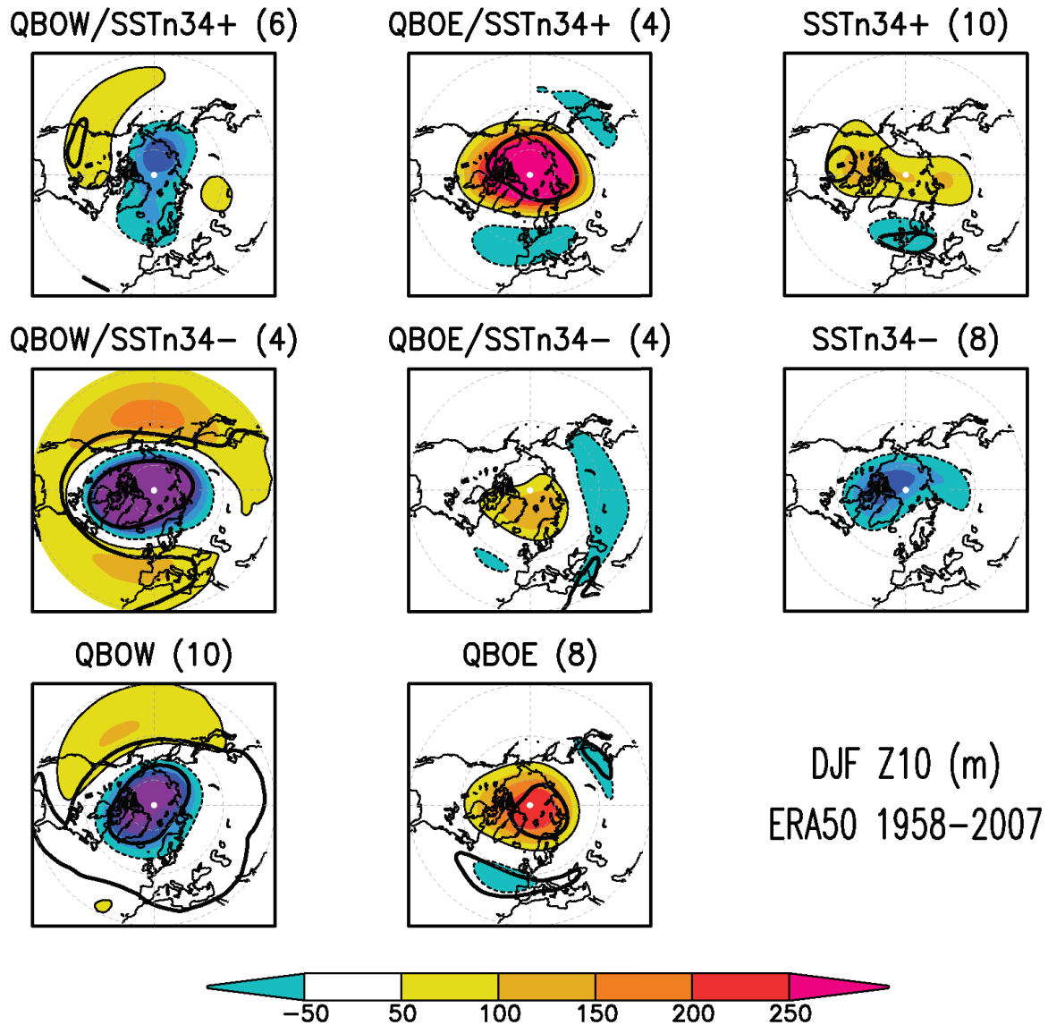
Figure 10: Double composites des anomalies hivernales (DJF) de géopotential à 10hPa (en m) aux moyennes et hautes latitudes de l'hémisphère Nord sur la base d'anomalies synchrones supérieures à un demi écart-type pour le vent zonal équatorial (5°S-5°N) à 30hPa comme indice de la QBO et les SST Niño3.4 comme indice de l'ENSO. Le trait noir épais délimite les anomalies significatives à 90%. Le nombre d'années utilisées pour chaque composite est indiqué entre parenthèses.
