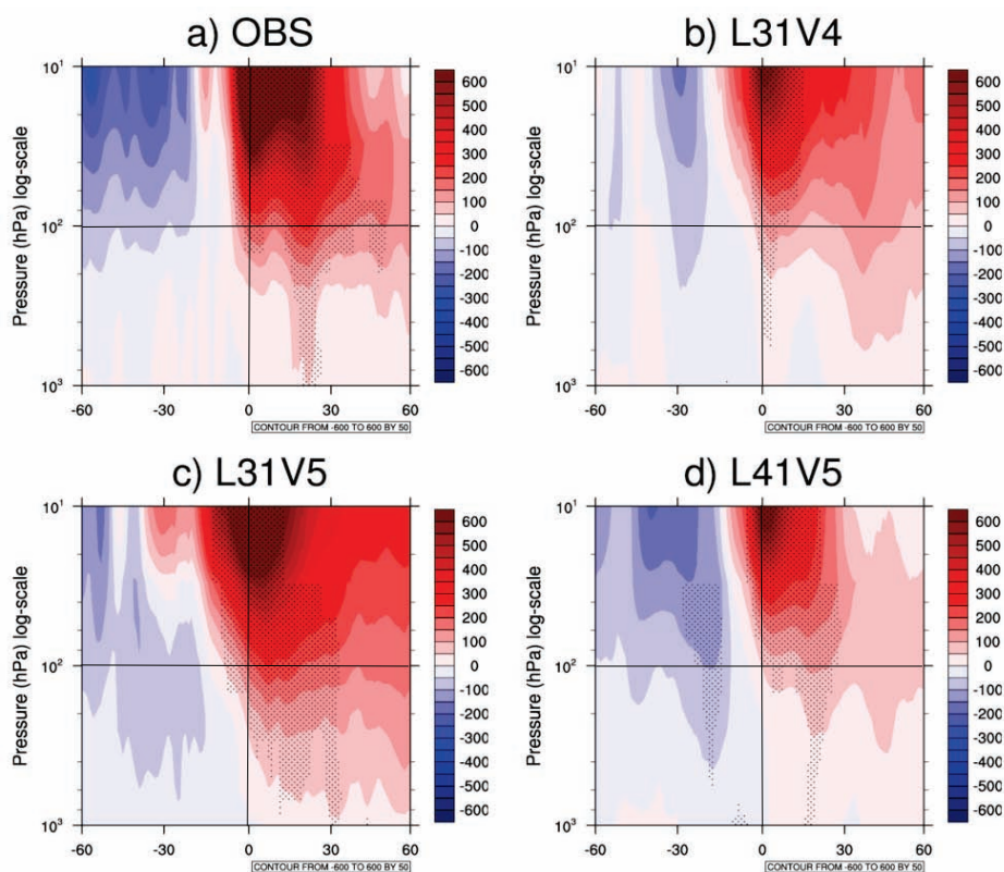
Figure 19: Coupes temps-pressure des anomalies quotidiennes de géopotential moyennées sur les épisodes de réchauffements stratosphériques, dans le domaine North Polar Cap ( > 60^\circ\text{N} ). Le jour 0 correspond à l'apparition d'un réchauffement stratosphérique, c'est à dire au renversement du vent zonal. Les pointillés représentent les anomalies significatives à 90 %.
