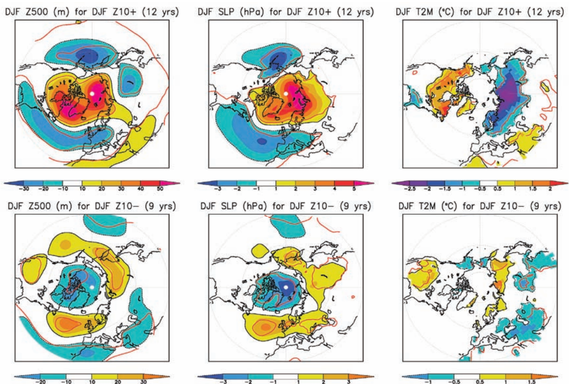
Figure 18: Analyse composite des anomalies hivernales (DJF) de géopotentiel à 500hPa (à gauche, en m), de pression au niveau de la mer (au milieu, en hPa), et de température de l'air à 2m (à droite, en °C) associées à un affaiblissement (en haut) ou un renforcement (en bas) du vortex polaire (anomalies DJF du géopotentiel à 10 hPa moyennées au nord de 60°N supérieures à un écart-type). Le trait rouge épais délimite les anomalies significatives à 90%. Le nombre d'années utilisées pour chaque composite est indiqué entre parenthèses.
