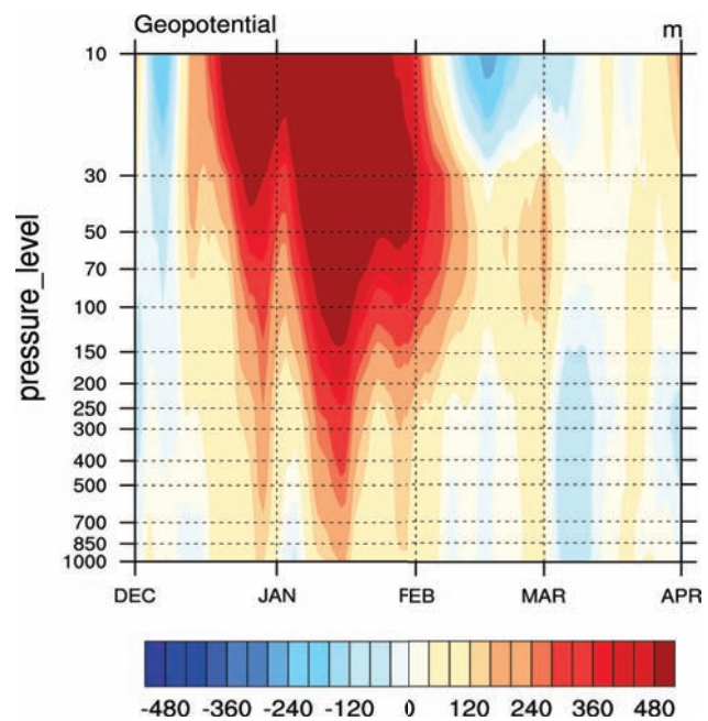
Figure 7: Coupe temps-pressure de l'anomalie quotidienne (par rapport à la climatologie ERA-40 1971-2000) de géopotential moyennée sur la bande 60°N-90°N, pour les mois de décembre 1976 à avril 1977. Données ERA-40.
