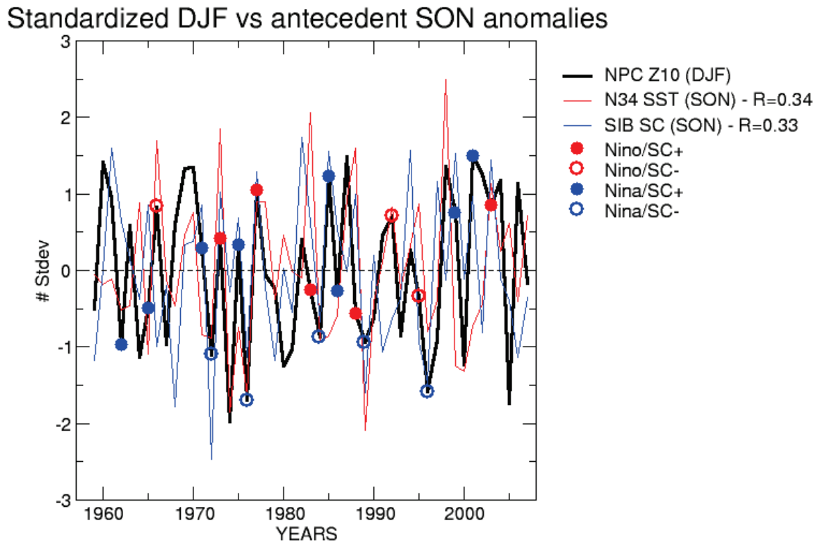
Figure 13: Anomalies hivernales (DJF) centrées et réduites (en nombre d'écart-type) pour différents indices climatiques : géopotential à 10hPa au nord de 60°N (en noir), SST Niño3.4 (en rouge), étendue de la couverture neigeuse sur la Sibérie (en bleu). A noter que les anomalies de SST et de neige sont moyennées sur l'automne (SON) précédent l'hiver sur lequel on moyenne le géopotential. Les symboles (cercles et disques de couleur) superposés à la courbe en noir montrent les hivers utilisés pour construire des composites du géopotential sur la base d'anomalies synchrones supérieures à un demi écart-type pour chacun des deux autres indices (ENSO et neige).
