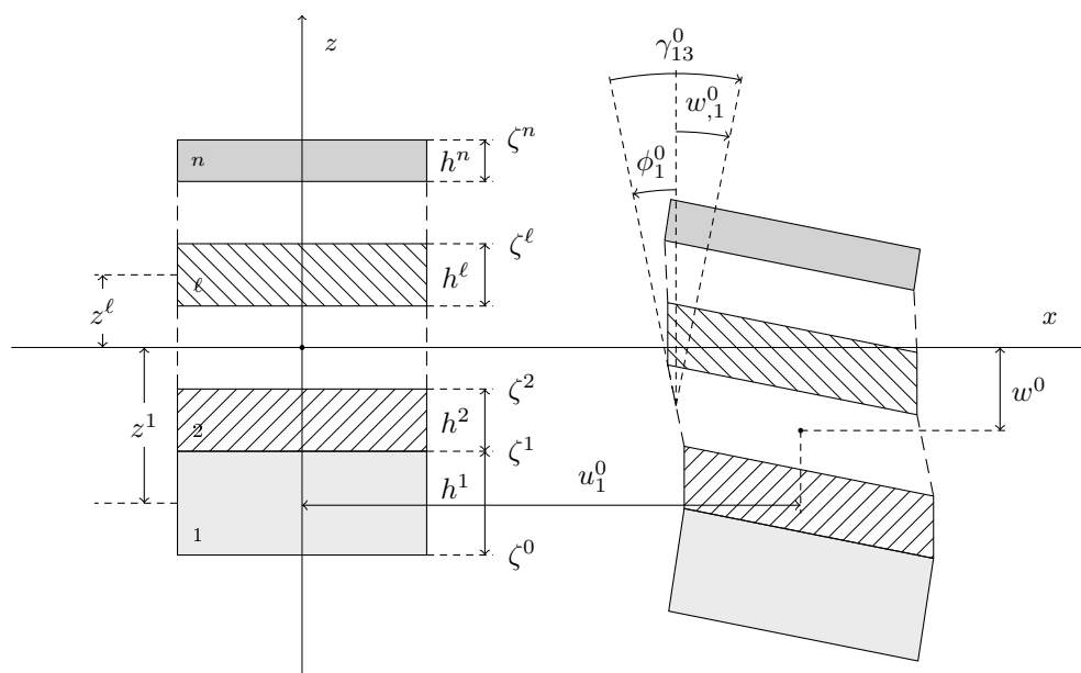
FIGURE 2.1 – Paramètres géométriques de la structure multicouche (présentée à gauche dans un état non déformé) et définition des déplacements.
