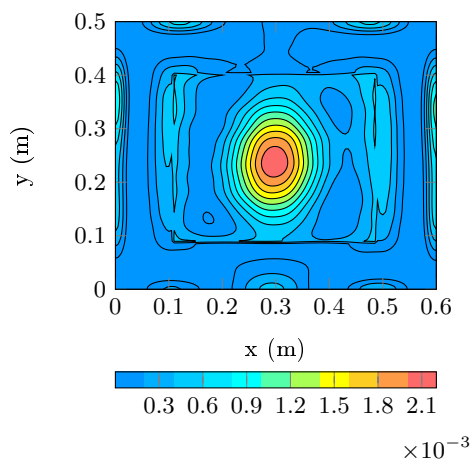
(c) Puissance dissipée \langle p_d^s(t) \rangle ( \text{W} \cdot \text{m}^{-2} )
