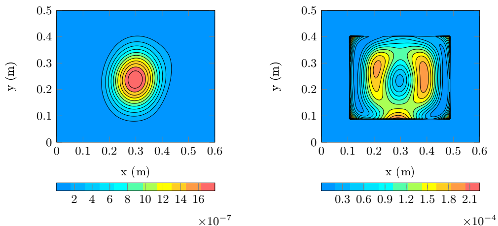
(a) Vitesse quadratique \langle i_3^2(t) \rangle ( \text{m}^2 \cdot \text{s}^{-2} ). (b) Energie de déformation puissance 2\omega \langle e_s^s(t) \rangle ( \text{W} \cdot \text{m}^{-2} )
