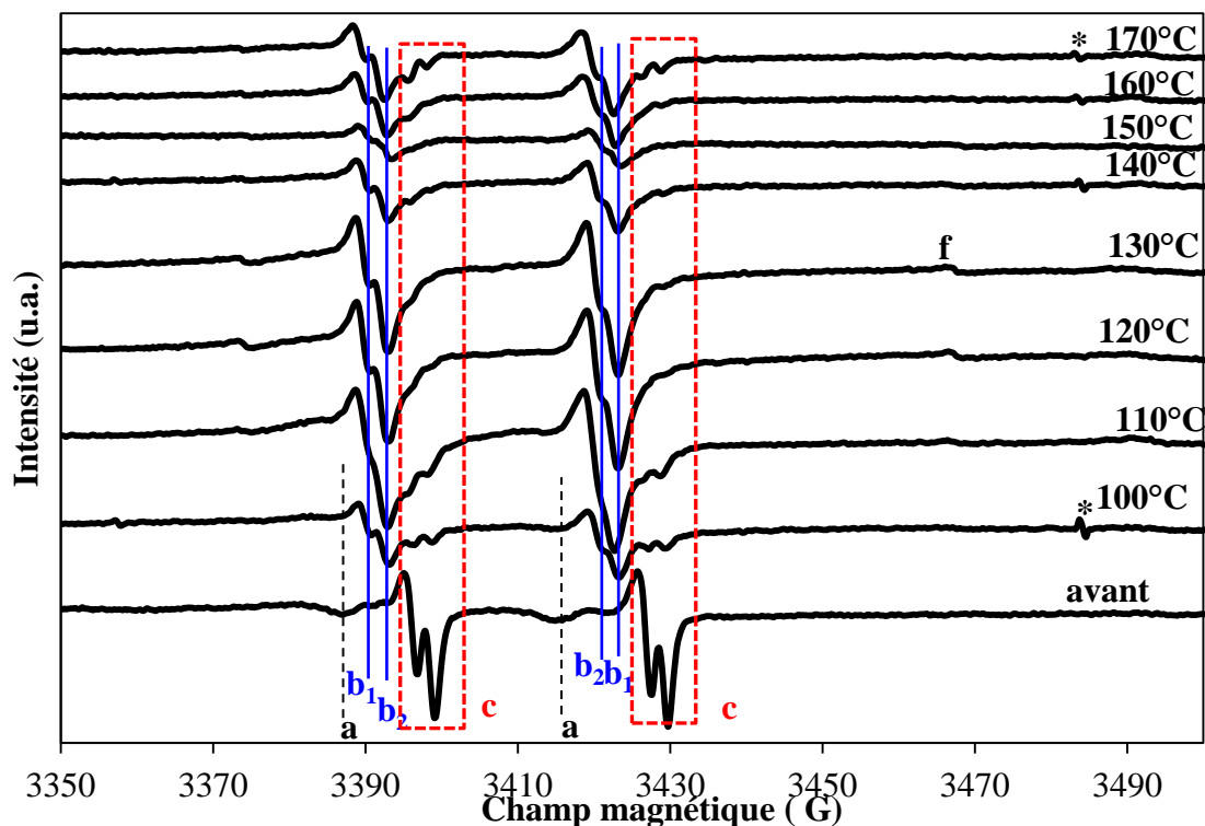
Figure III.16: Spectres RPE enregistrés à -196^{\circ}C obtenus en fonction de la variation de la température du déroulement de la réaction d'oxydation du propène en présence du catalyseur 10\%Ag/CeO_2(Imp)
