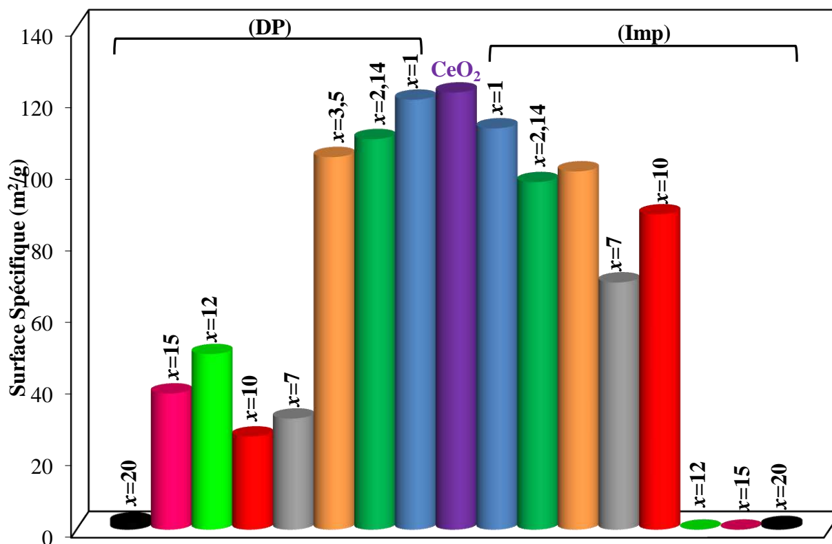
Figure II.3: Surfaces Spécifiques des catalyseurs x\%Ag/CeO_2 (Imp) et (DP)
