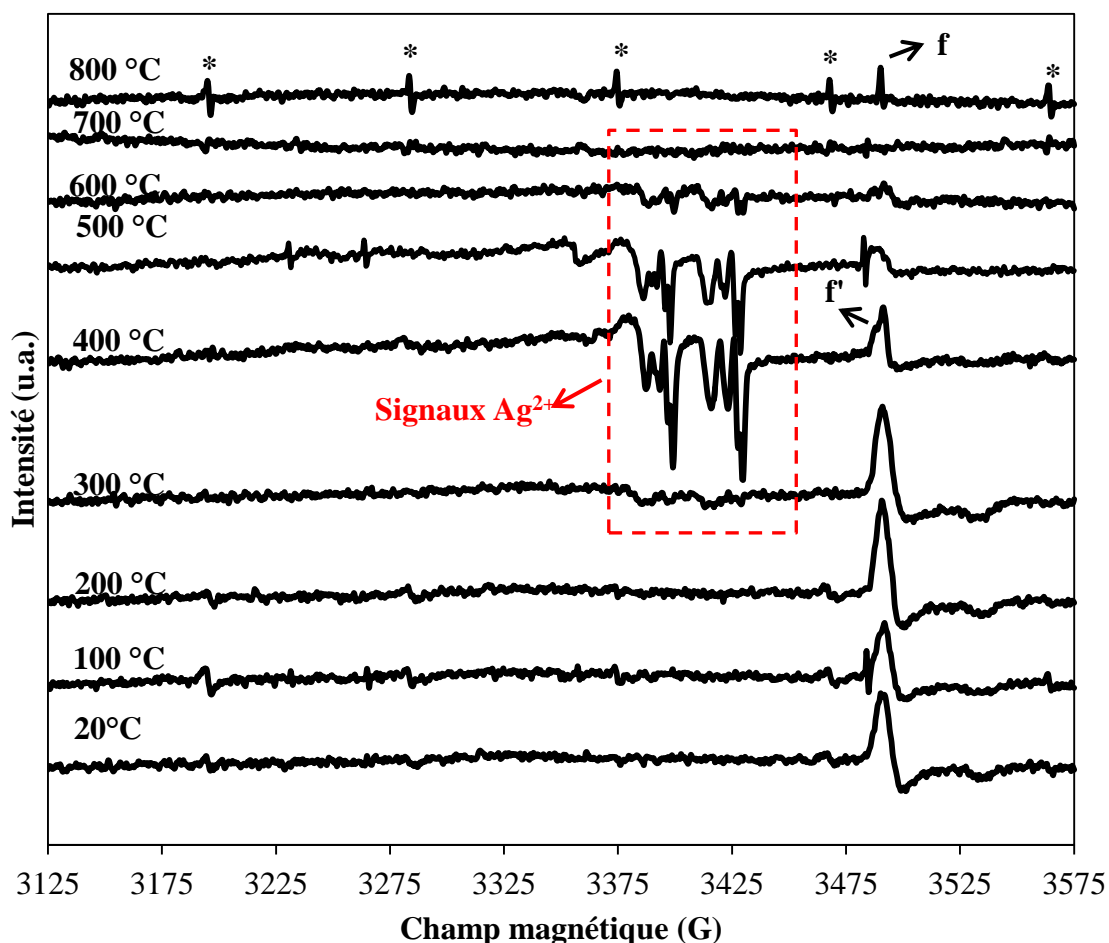
Figure II.21: Spectres RPE enregistrés à -196^{\circ}C pour l'échantillon 10\%Ag/CeO_2(Imp) sur différentes températures de calcination
