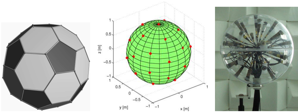
Figure 2: Gauche: géométrie d'un icosaèdre tronqué. Centre: distribution des points au centre de chaque face de l'icosaèdre tronqué. Droite: Antenne sphérique de rayon 14.5 cm avec 31 microphones conçue pour les validations expérimentales.
