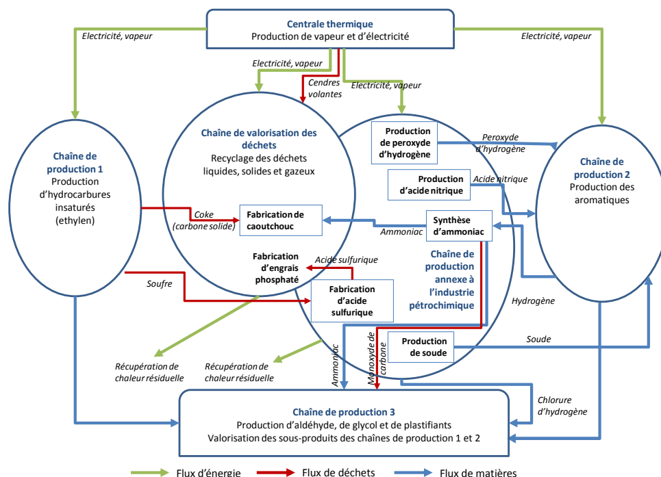
Figure 42 – La symbiose industrielle de Ningbo Chemical Industrial Zone (traduit et adapté de Wang M. F. et al. 2006)
