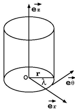
FIGURE 2.21 – Repère cylindrique utilisé pour décrire le comportement des cyclones tropicaux de l’hémisphère Nord. O est le centre du cyclone, r le rayon et λ l’angle. Tiré de Beucher (2010) .
