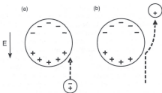
FIGURE 2.5 – Représentation schématisée des processus inductifs lors d'une collision entre deux hydrométéores. Placées dans un champ électrique dirigé vers le bas, les particules présentent un aspect dipolaire (les charges + vers le bas). Lors d'une collision, la petite particule va capter une charge positive provenant de la grosse particule. Tiré de MacGorman et Rust (1998) .
