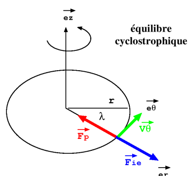
FIGURE 2.23 – Vue schématique de l'équilibre cyclostrophique dans un cyclone de l'hémisphère nord. Tiré de Beucher (2010) .
