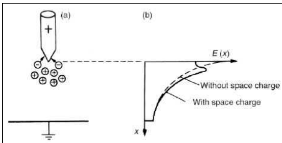
Figure 2.14. Influence de la charge d'espace sur la distribution du champ électrique inter-électrodes en polarité positive [96]
