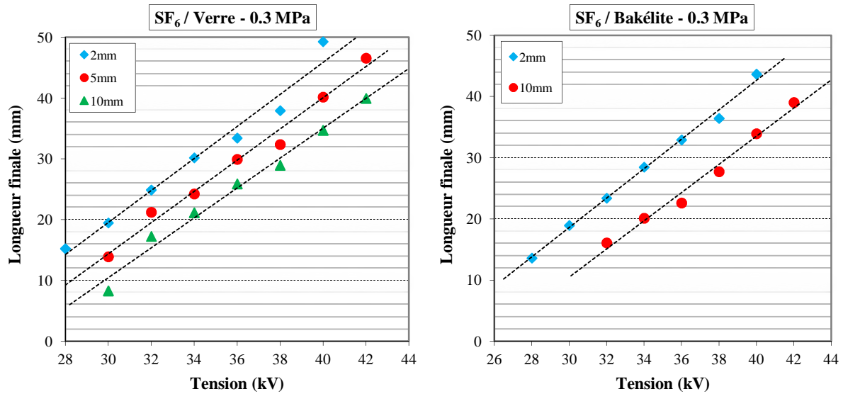
Figure 5.12. Variation de la longueur finale des décharges glissantes en fonction de l'épaisseur du solide dans le SF 6 à 0.3 MPa, sous tension continue, pour les deux matériaux ( e = 2 \text{ mm} ): Verre et Bakélite
