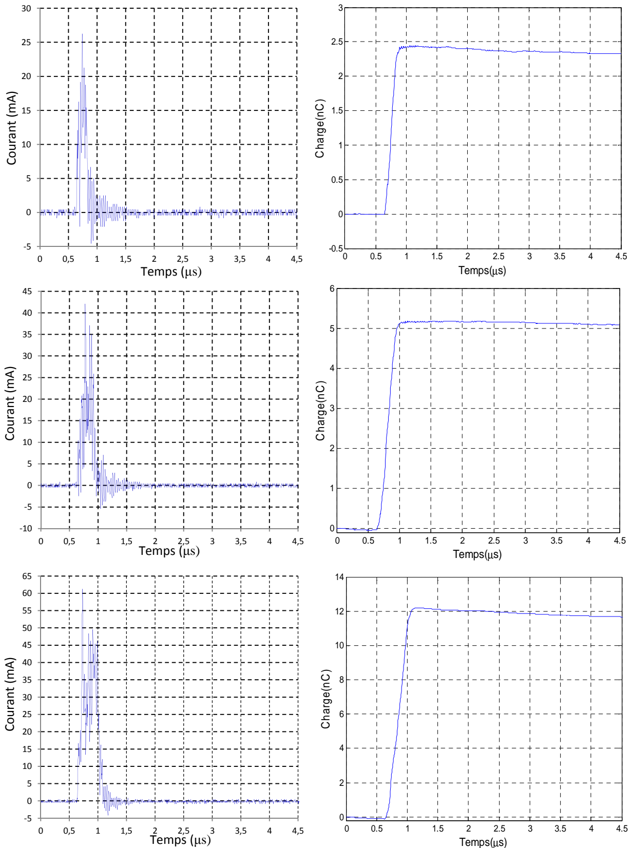
Figure 5. 14. Les courants et charges associés aux décharges glissantes obtenues avec des échantillons en verre de 2 mm d'épaisseur en présence de SF_6 à 0.3 MPa de pression pour différentes valeurs de tension 30, 34 et 38 kV
