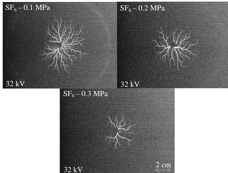
Figure 5.5. Influence de pression du gaz sur les décharges glissantes sous tension continue obtenues avec un échantillon en Bakélite de 2 mm d'épaisseur dans le SF 6
