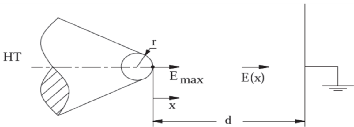
Figure 2.7. Système d'électrodes pointe - plan
