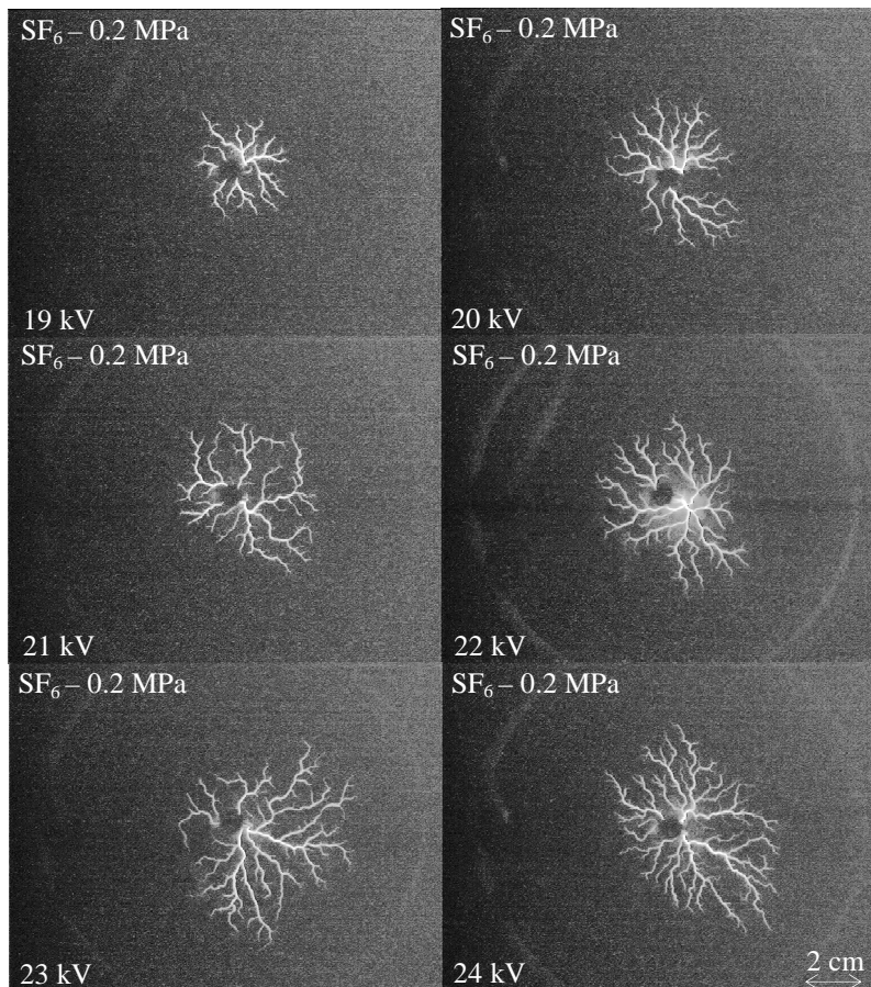
Figure 4.13. Influence de l'amplitude de la tension sur les décharges glissantes sous tension alternative avec une interface SF 6 /Bakélite ( e = 2 mm)
