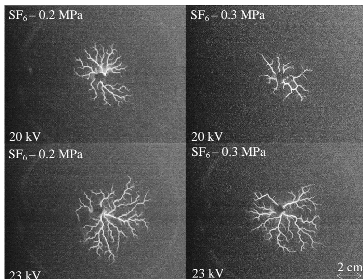
Figure 4.13. Influence de l'amplitude de la tension sur les décharges glissantes sous tension alternative avec une interface SF 6 /Bakélite ( e = 2 mm)
