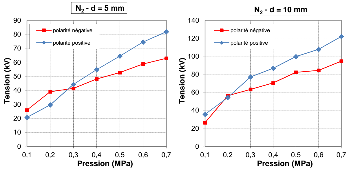
Figure 2.10. Tenue diélectrique du N_2 en champ quasi-uniforme (sphère - plan) pour deux distances inter-électrodes 5 et 10 mm, sous tension impulsionnelle (polarité positive et négative)
