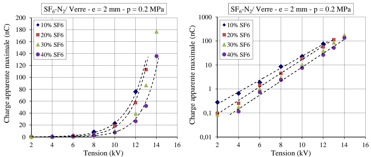
Figure 3.11. Evolution de la charge apparente maximale des décharges partielles en fonction de la tension appliquée et du pourcentage de SF_6 dans le N_2 , obtenue avec des échantillons en verre de 2 mm d'épaisseur, sous une pression de 0.2 MPa
