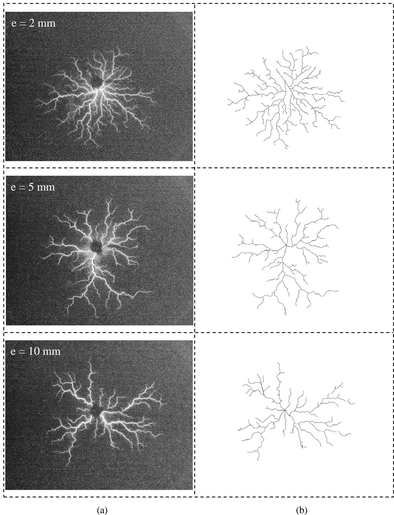
Figure 5.16. Images de décharges glissantes se propageant sur l'échantillon en verre en présence de SF_6 à 0.3 MPa sous tension continue pour différentes épaisseur: (a) image originale (b) image en binaire correspondante
