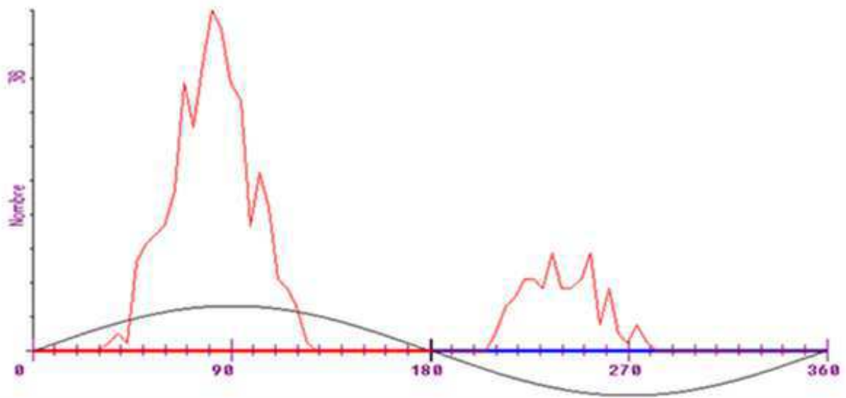
Figure 3.3. Répartition du nombre de décharges partielles par phase obtenue avec un échantillon solide en verre de 2 mm d'épaisseur en présence de SF 6 à 0.2 MPa de pression, sous tension alternative de 6 kV
