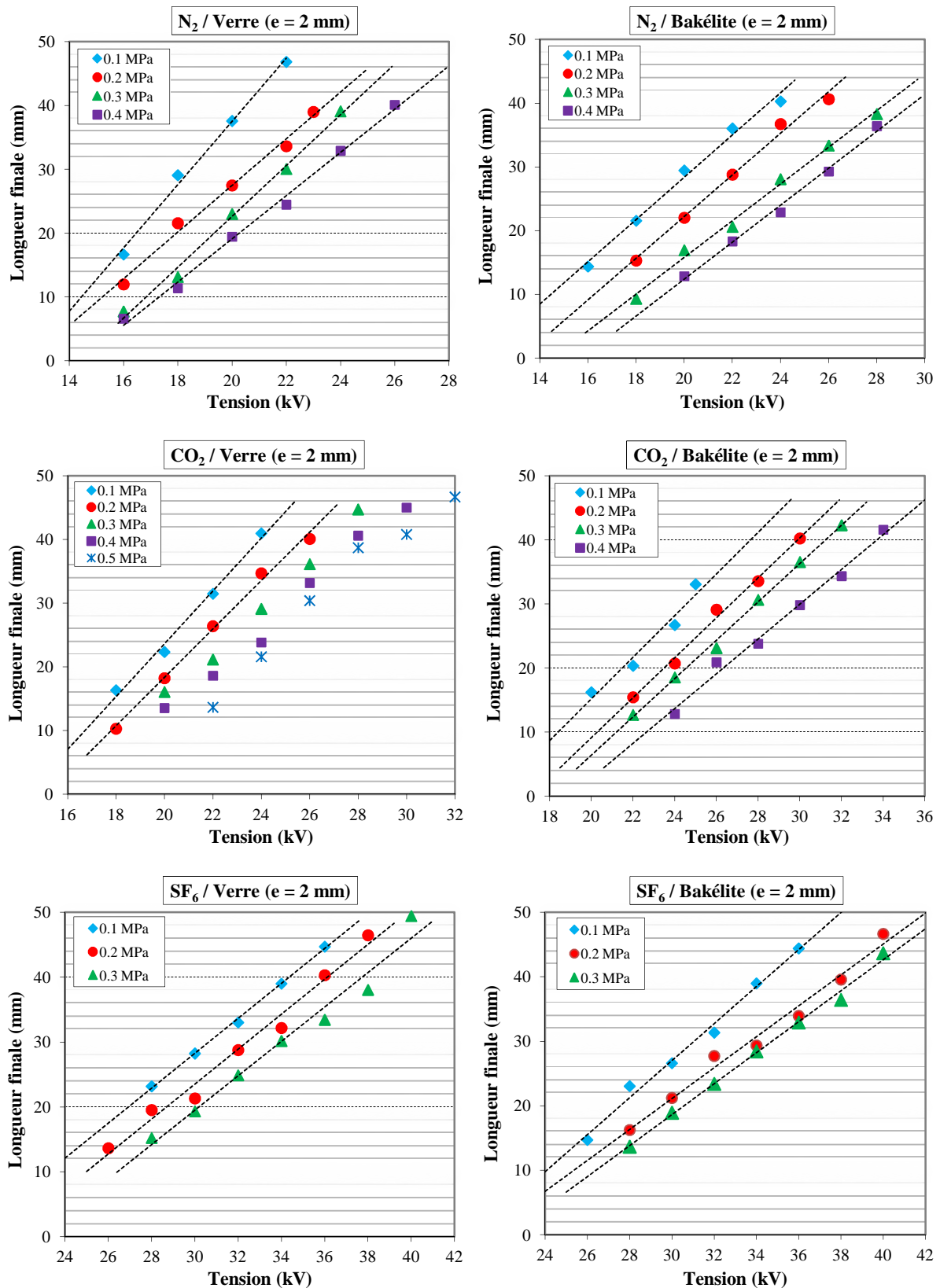
Figure 5.6. Variation de la longueur finale des décharges glissantes en fonction de la tension en présence des gaz N 2 , CO 2 et SF 6 sous différentes pressions pour les deux matériaux (e = 2 mm): Verre ( \epsilon_r = 5 ) et Bakélite ( \epsilon_r = 4.8 ), sous tension continue
