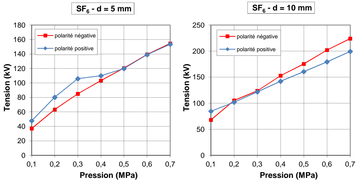
Figure 2.12. Tenue diélectrique du SF 6 en champ quasi-uniforme (sphère - plan) pour deux distances inter-électrodes 5 et 10 mm, sous tension impulsionnelle (polarité positive et négative)
