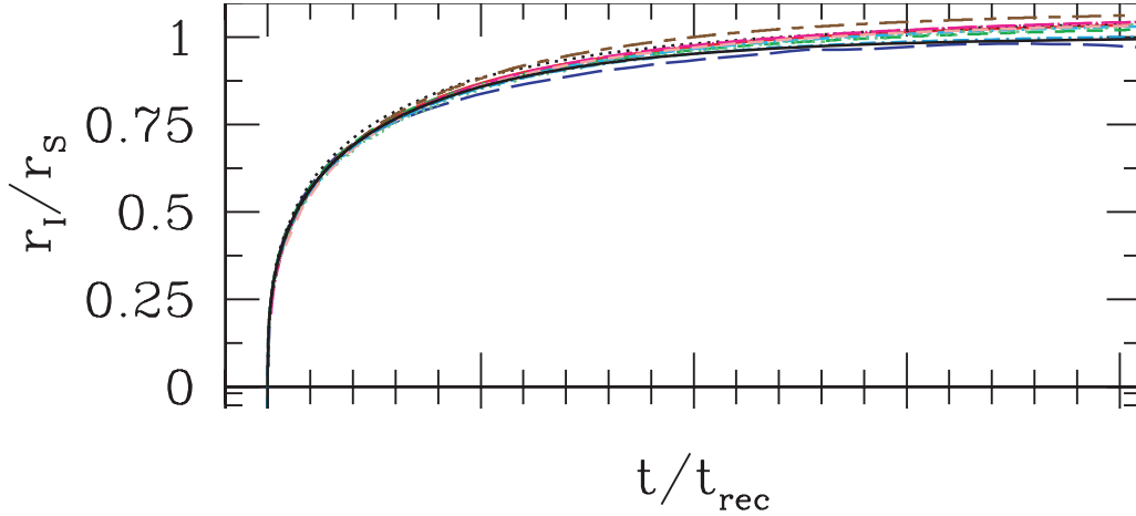
FIG. 1.8 – Evolution du rayon d’une sphère ionisée en expansion autour d’une source ionisante. Le rayon est exprimé en unité du rayon de Strömngren calculé au moyen de l’équation 1.24. La figure est extraite de Iliev et al. 2006a et montre la bonne correspondance entre l’évolution issue de différentes simulations de transfert du rayonnement et de la théorie exposée dans cette section (courbe noire en trait plein).
