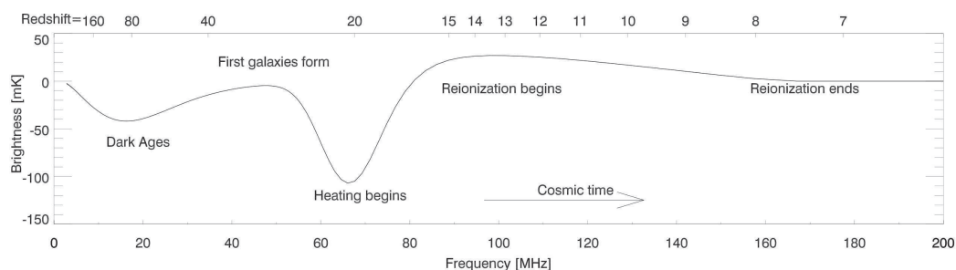
FIG. 1.17 – Evolution de la brillance de la raie à 21 cm moyennée sur tout le ciel des âges sombre (à z = 200 ) jusqu'à la fin de la période de réionisation un peu avant z = 6 . La ligne solide indique l'évolution du signal tandis que la ligne en tirets donne pour référence la valeur T_b = 0 . La figure est extraite de Pritchard & Loeb (2012).
