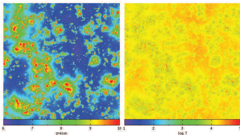
FIG. 2.5 – Exemple de cartes de redshifts de réionisation z_{reion} comparées aux champs de température pris au moment de la réionisation. La figure est extraite de Trac et al. (2008).
