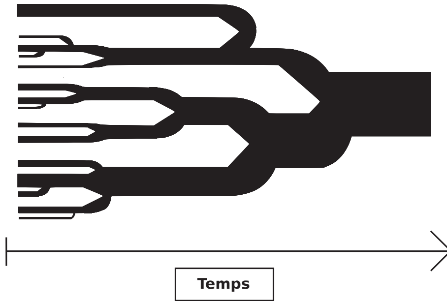
FIG. 3.1 – Schéma illustratif d'un arbre de fusion de halos de matière noire montrant la croissance en masse des halos par fusion successive. Le temps s'écoule de la gauche vers la droite et la taille des branches encode la masse des halos. (Figure inspirée de la figure 6 de Lacey & Cole 1993)
