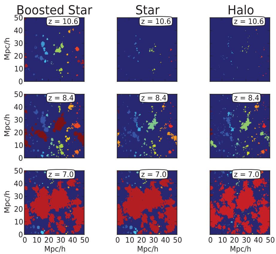
FIG. 4.5 – Cartes bidimensionnelles du champ d’ionisation pris à trois redshifts distincts dans les trois modèles de sources ionisantes pour les boîtes de 50 \text{ Mpc}/h .
