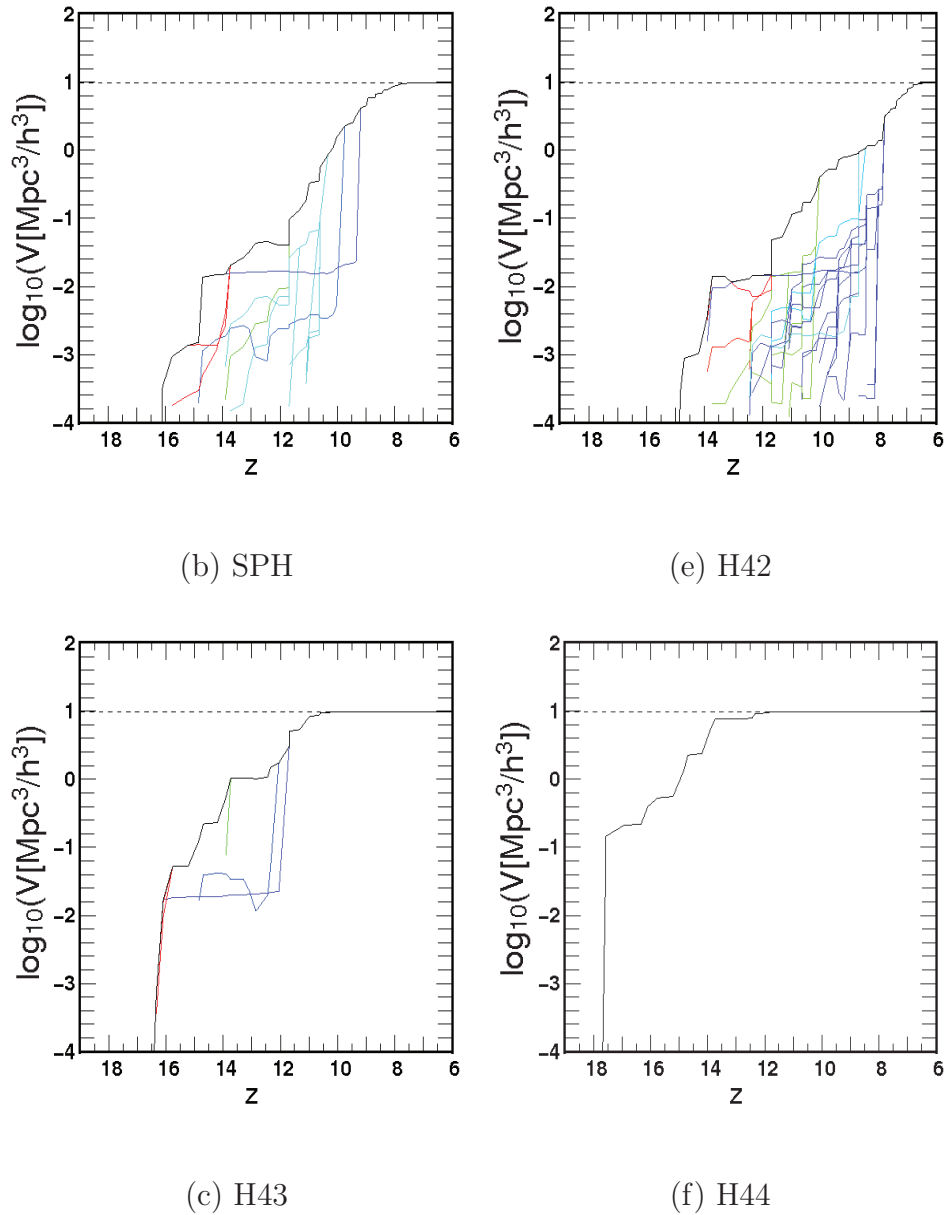
FIG. 8.3 – Evolution avec le redshift du volume des régions HII associées à M31. La ligne en trait plein noire représente l'évolution du volume de la région la plus grande. Les lignes en couleurs représentent les évolutions du volume des régions qui ont au moins atteint 10% du volume de la plus large à un moment dans la simulation. La ligne horizontale noire en tirets représente le volume total du cube contenant le progéniteur de M31. Les différentes couleurs encodent les différents redshifts de fusion des régions HII avec la région la plus large (rouge représente une fusion précoce et bleu une fusion tardive).
