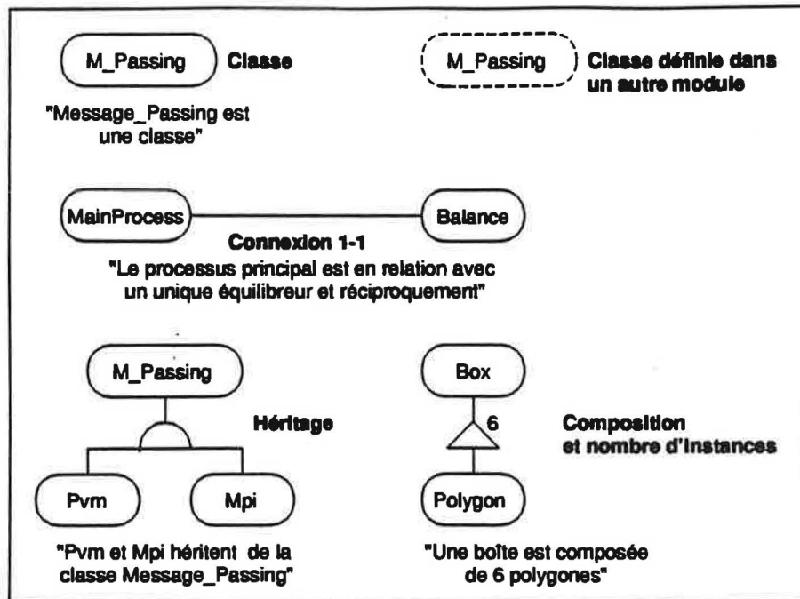
Figure 104 Conventions graphiques de représentation des diagrammes objets
