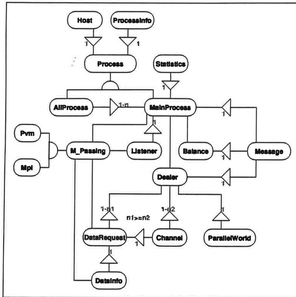
Figure 105 Diagramme objet du noyau parallèle
