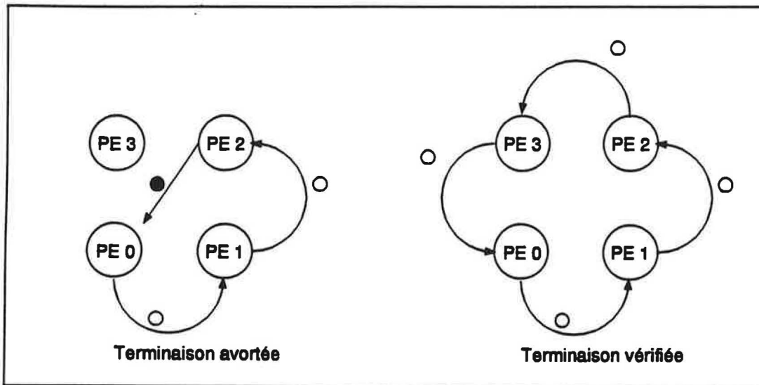
Figure 56 Algorithme de terminaison
