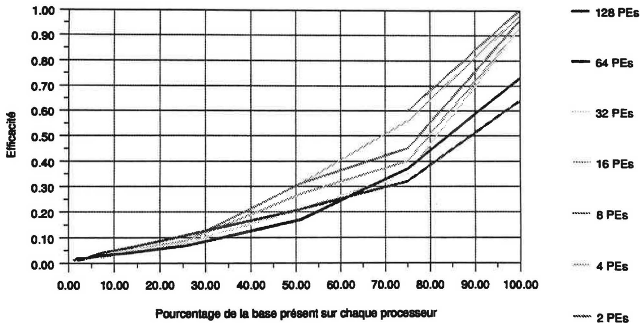
Figure 63 Efficacité en fonction de la distribution de la scène pour l'image M5.
