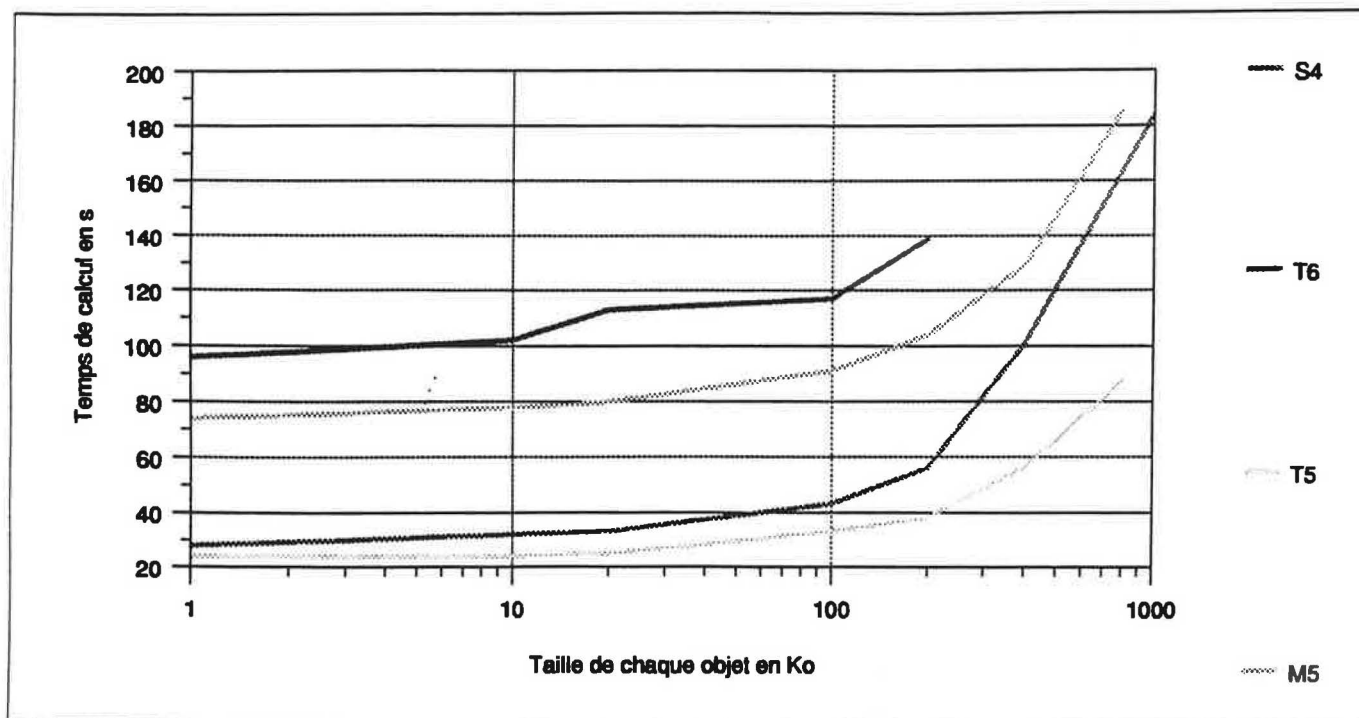
Figure 92 Temps de calcul pour 64 processeurs en fonction de l'augmentation de la taille des objets
