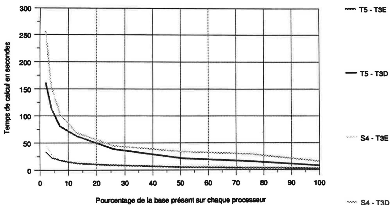
Figure 87 Comparaison des temps de calcul obtenus sur CRAY T3D et T3E avec 64 processeurs
