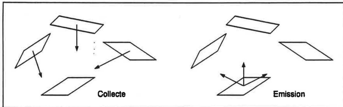
Figure 41 Radiosité par collecte et par émission
