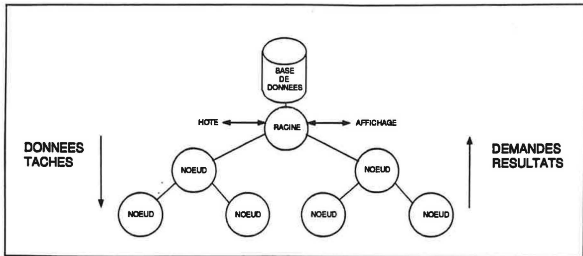
Figure 37 Architecture en forme d'arbre
