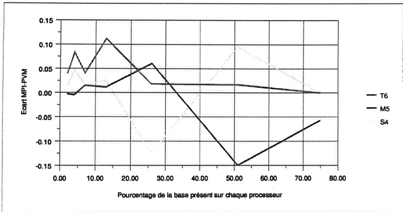
Figure 86 Ecart entre les temps de calculs avec MPI et PVM pour 64 processeurs
