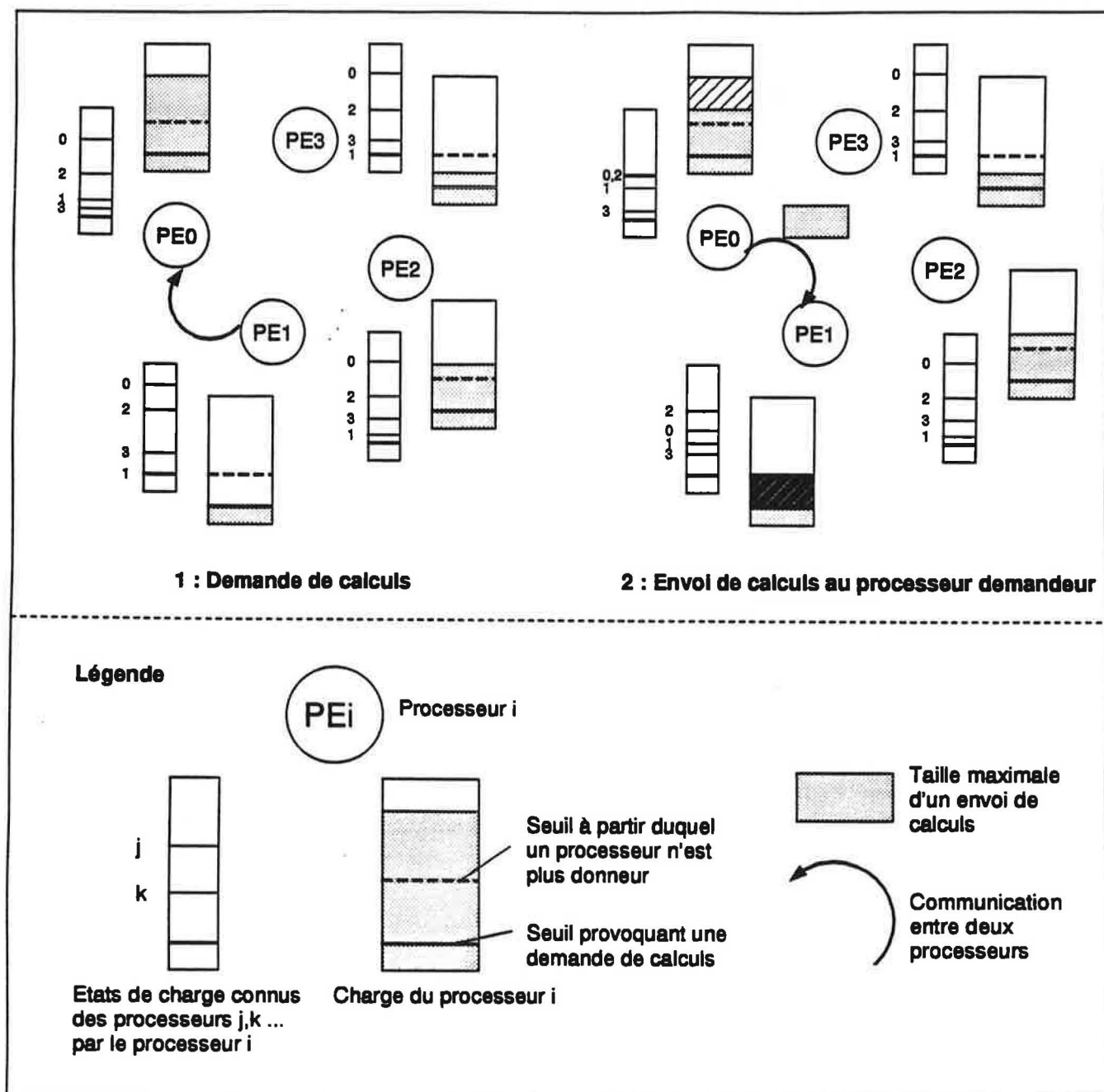
Figure 47 Nouvel équilibrage dynamique
