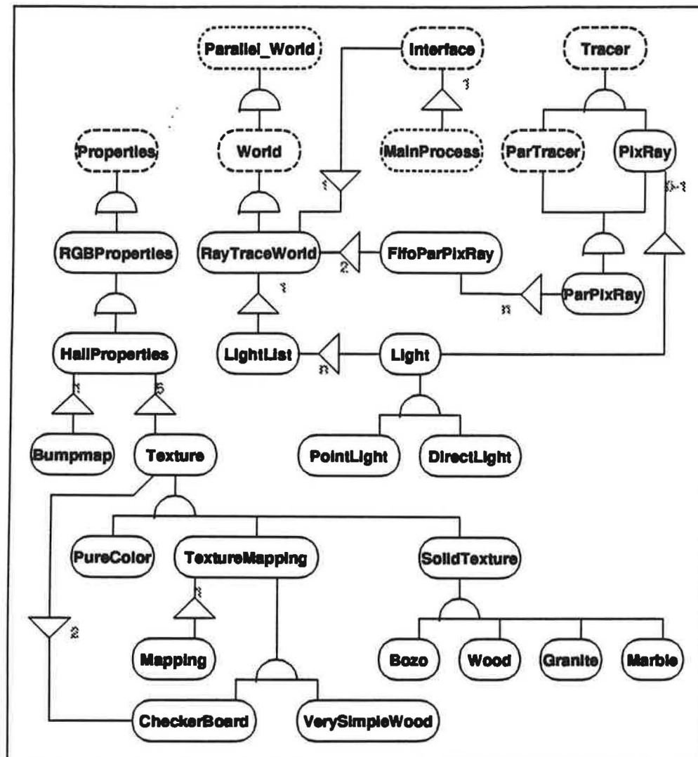
Figure 107 Diagramme objet du module optique
