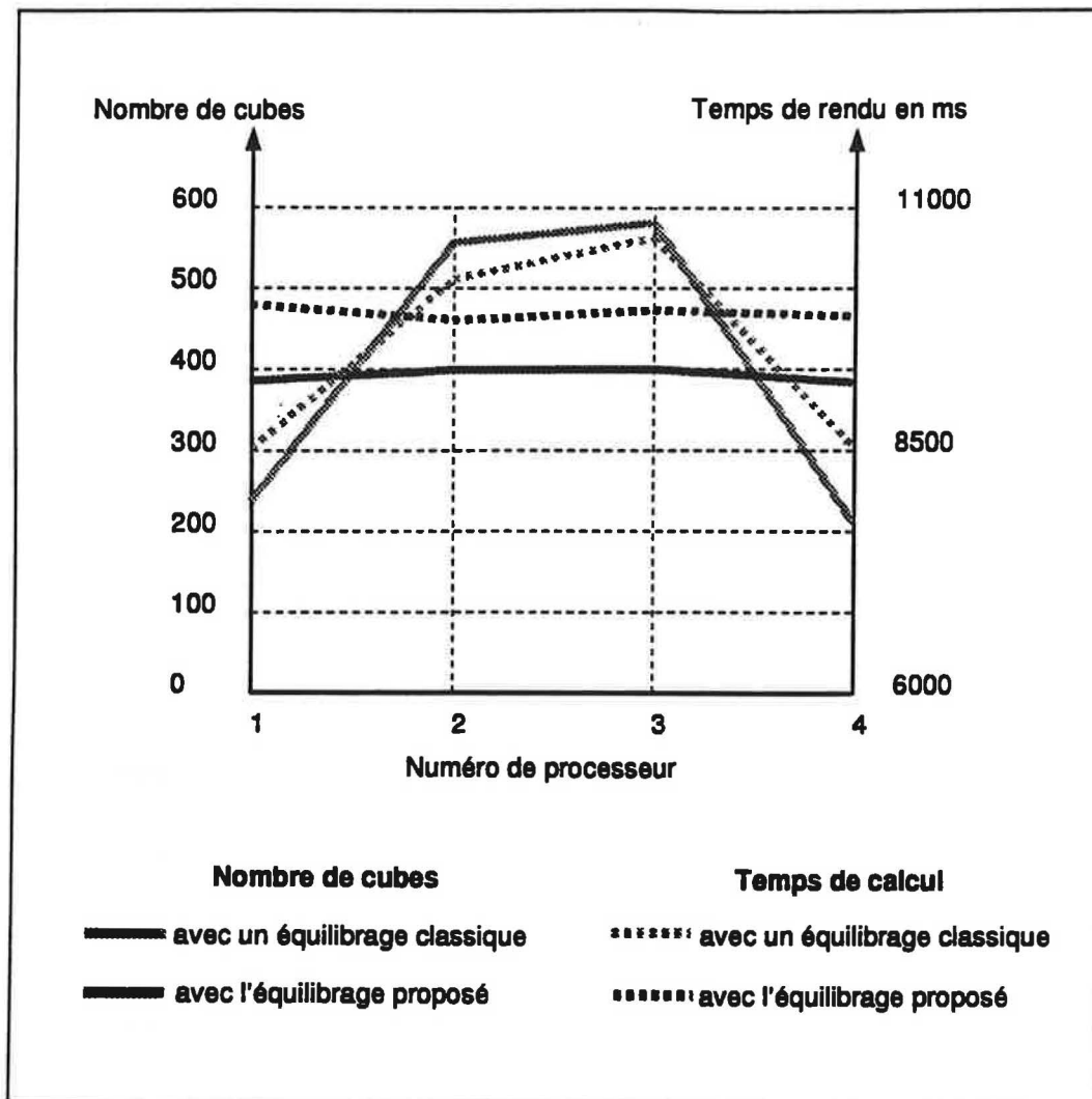
Figure 32 Comparaison de l'équilibrage des charges entre un découpage en tranches et celui proposé par Silva
