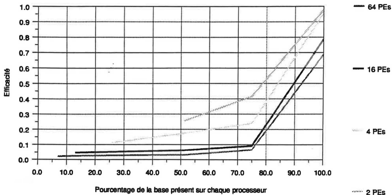
Figure 71 Efficacité pour l'image T5
