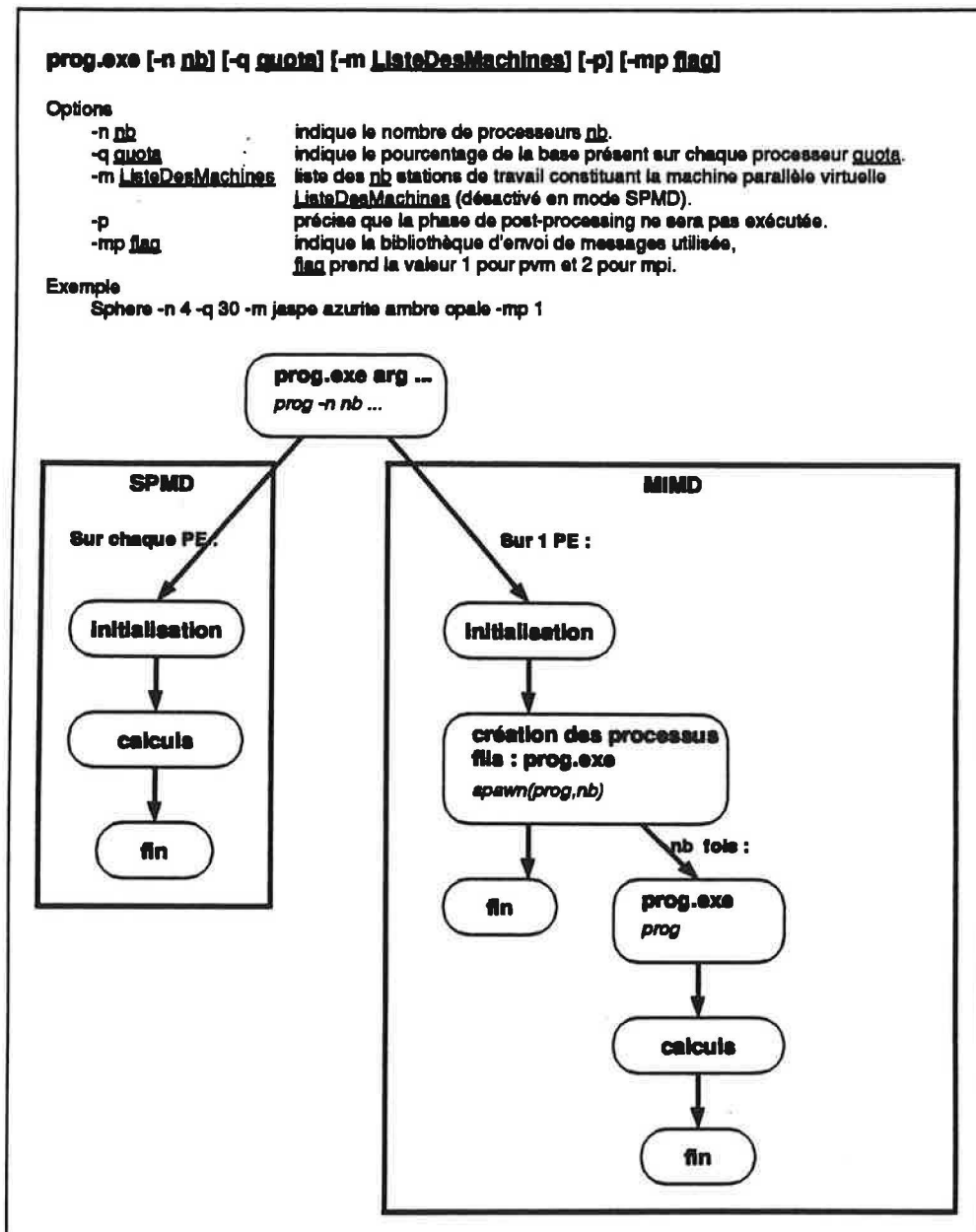
Figure 58 Procédure de lancement du logiciel
