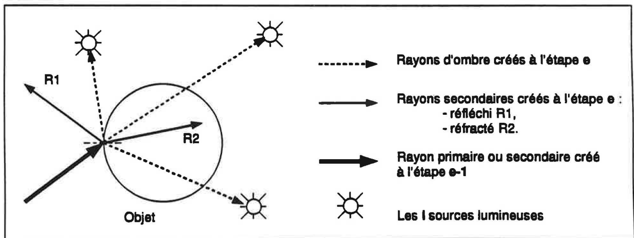
Figure 55 Création de rayons à chaque étape
