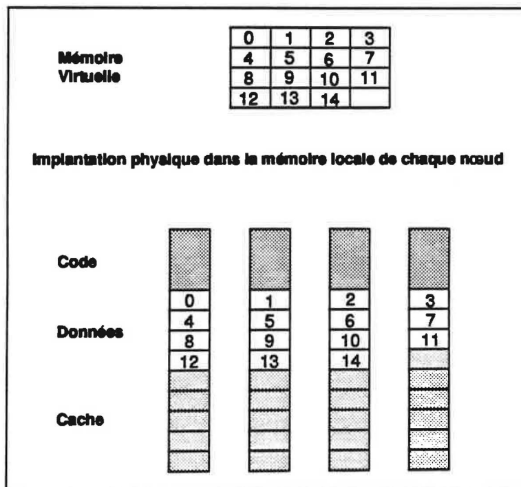
Figure 38 Implantation d'un mémoire partagée virtuelle
