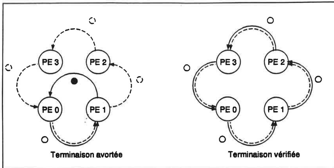
Figure 57 Trajets du jeton sur plusieurs parcours
