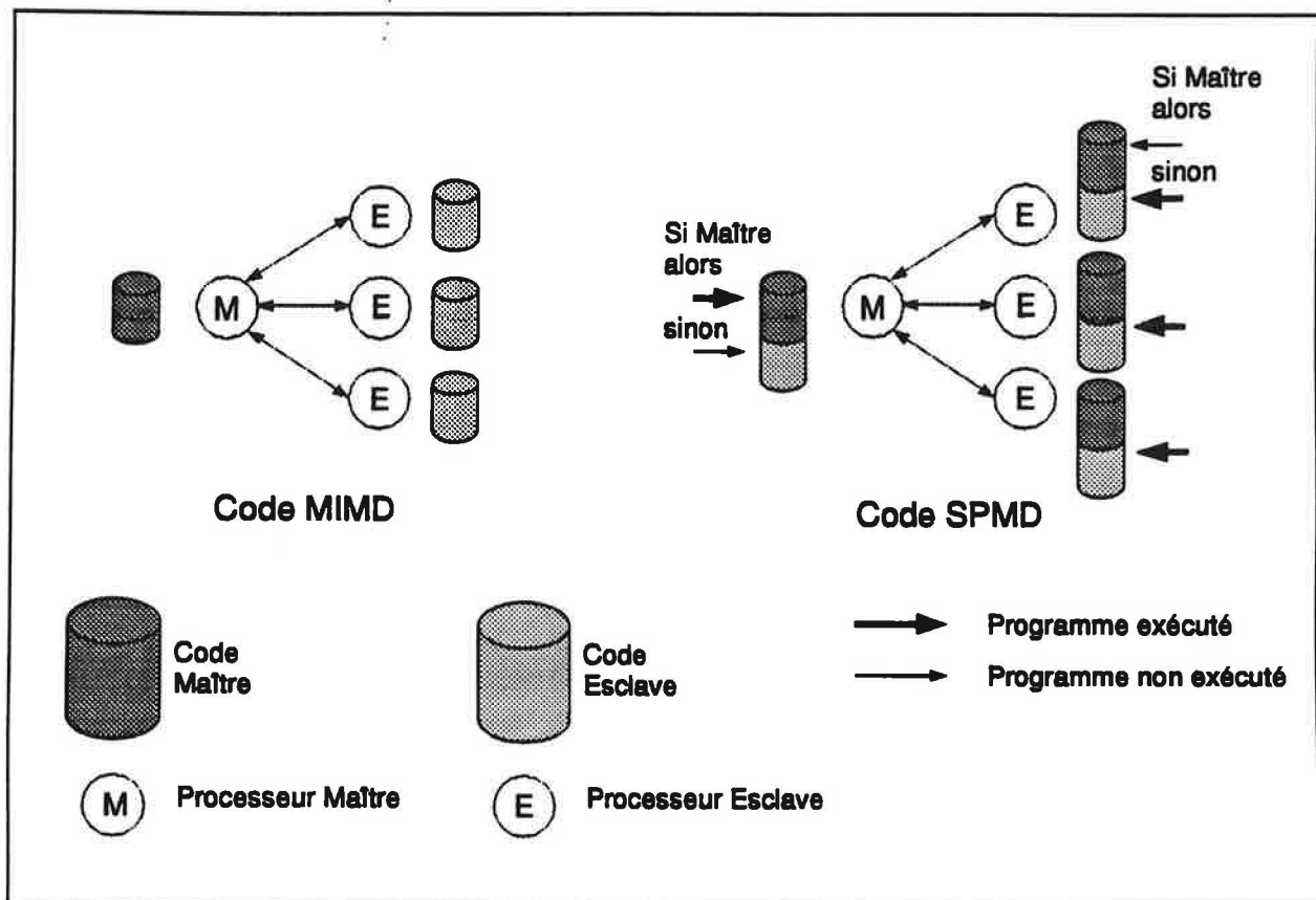
Figure 23 Différences entre codes MIMD et SPMD
