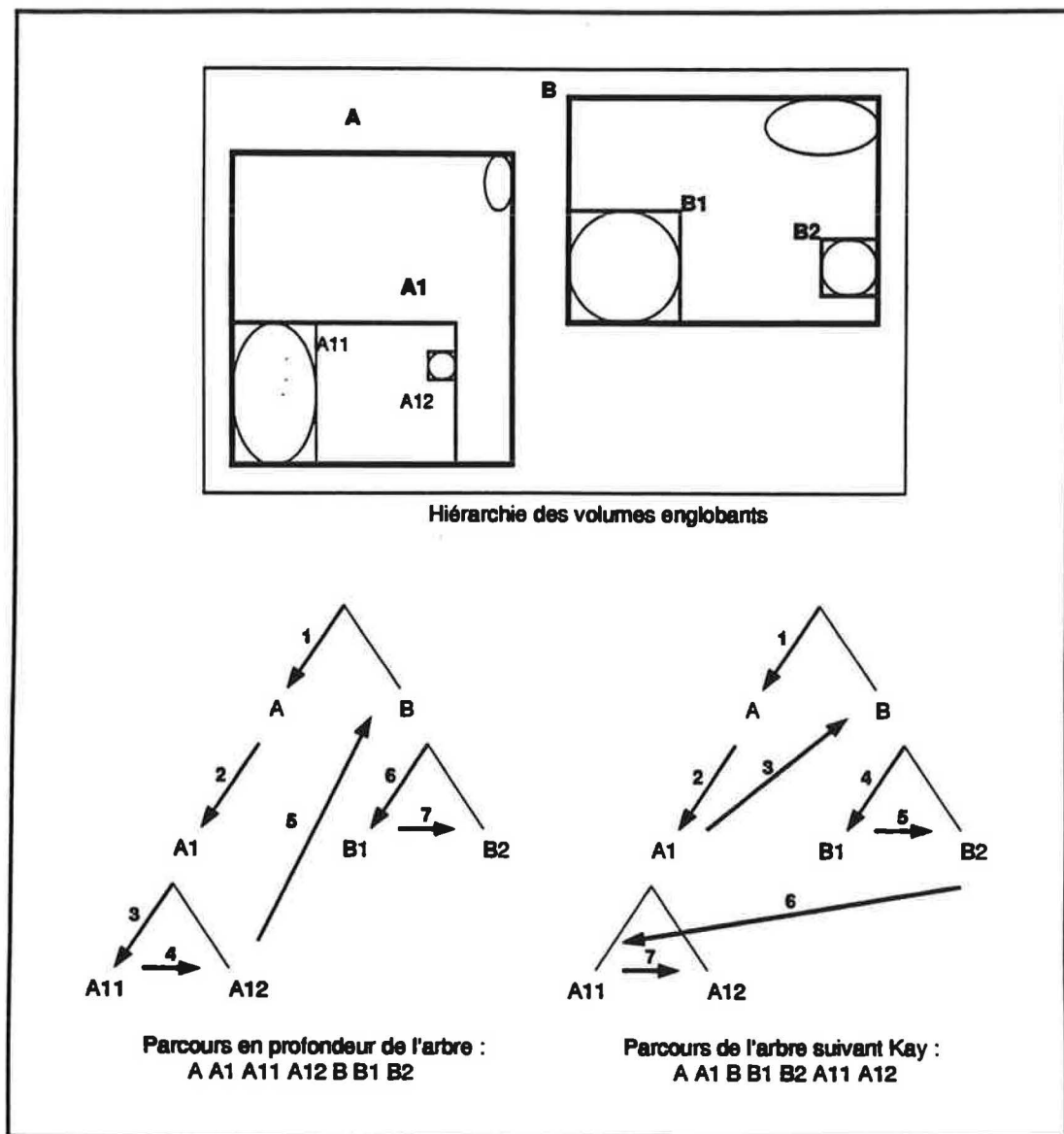
Figure 9 Accélération du parcours d'un arbre
