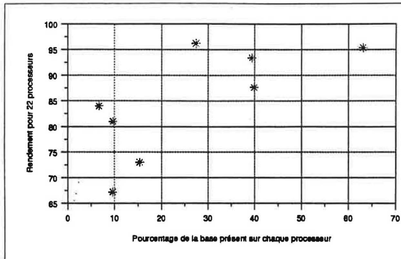
Figure 36 Rendement pour 22 processeurs sur différentes images en fonction du pourcentage de la base présent sur chaque processeur
