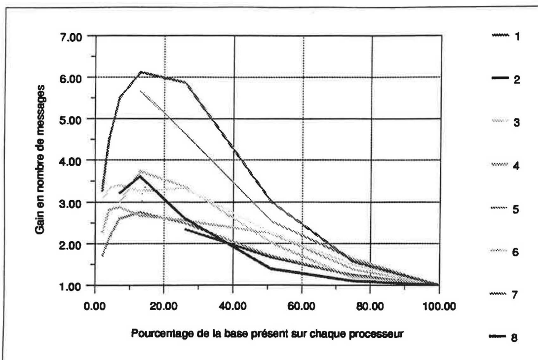
Figure 79 Gains en nombre de messages de l'algorithme à flots concurrents par rapport à l'algorithme à flots de données
