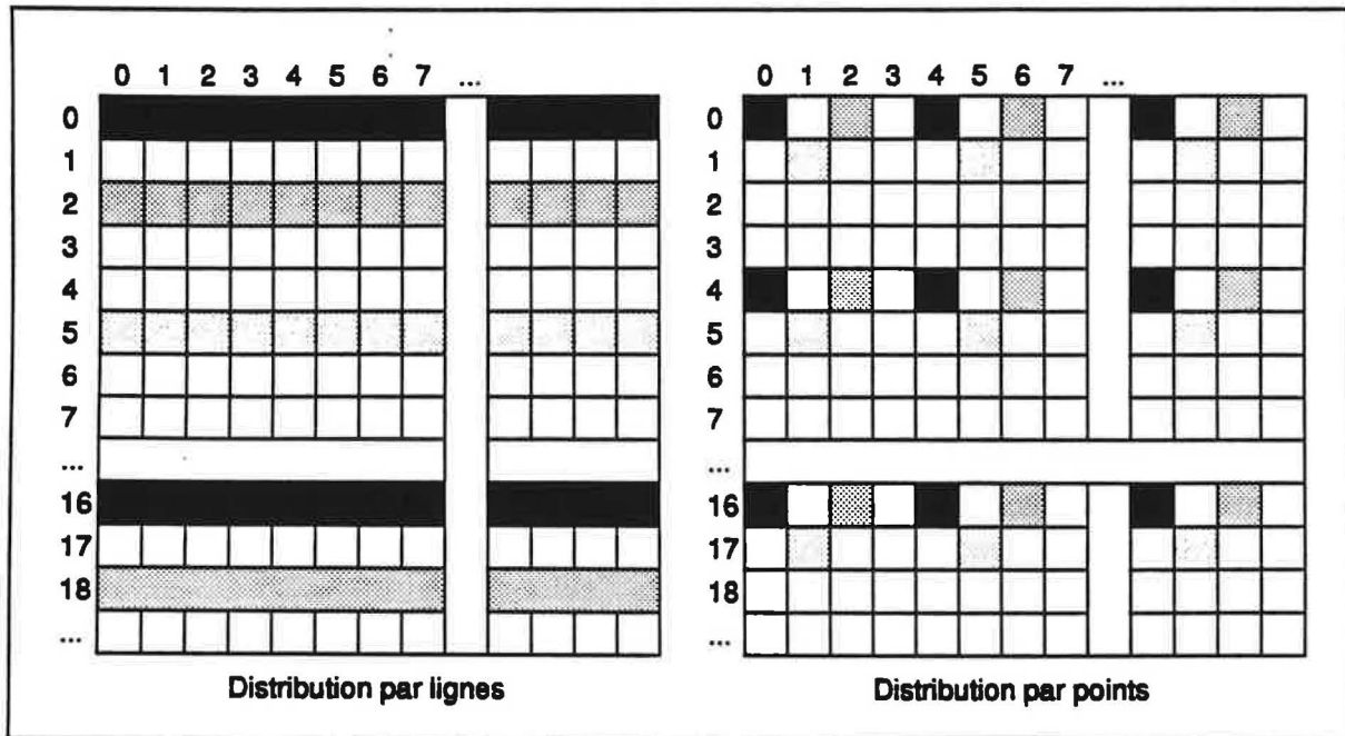
Figure 25 Distributions statiques de pixels sur 16 PEs
