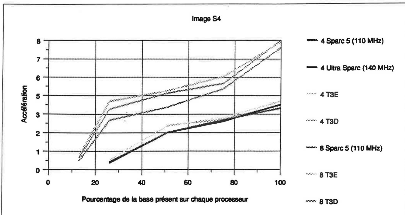
Figure 90 Comparaison de l'efficacité avec 4 et 8 processeurs sur des architectures variées (image S4)
