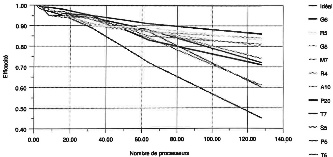
Figure 60 Efficacité avec base dupliquée
