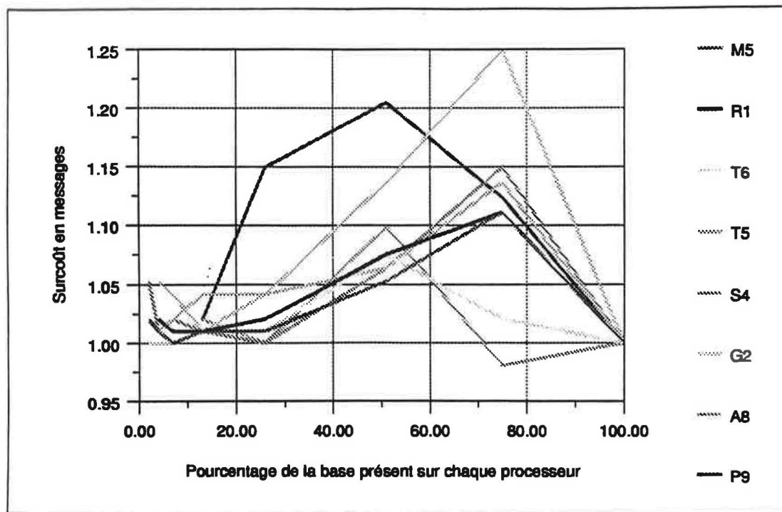
Figure 68 Surcoût en messages induit par l'équilibrage dynamique pour 64 processeurs
