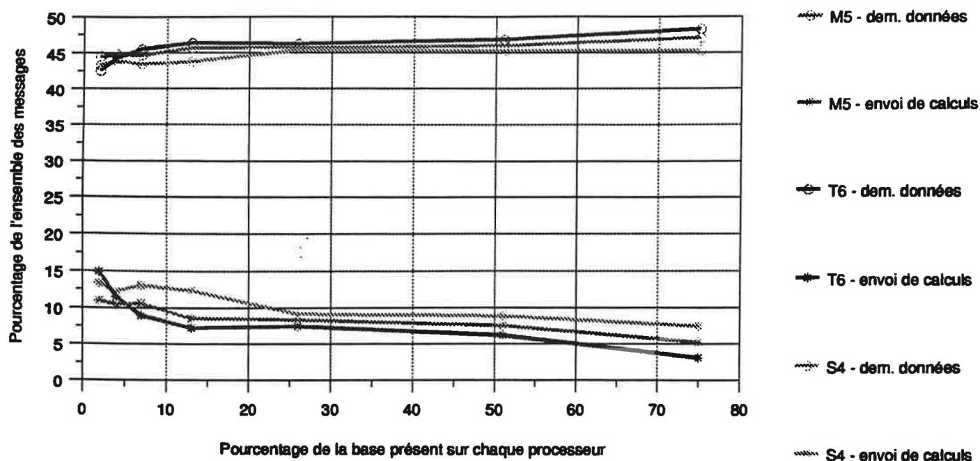
Figure 82 Comparaison du nombre de messages de chaque type pour l'algorithme à flots concurrents
