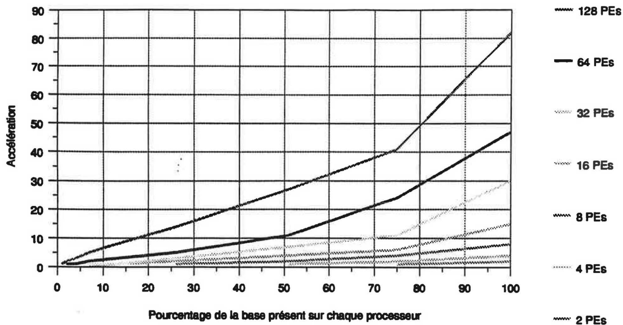
Figure 62 Accélération en fonction de la distribution de la scène pour l'image M5.
