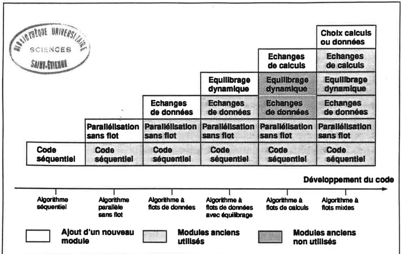
Figure 48 Etapes de développement de l'algorithme parallèle
