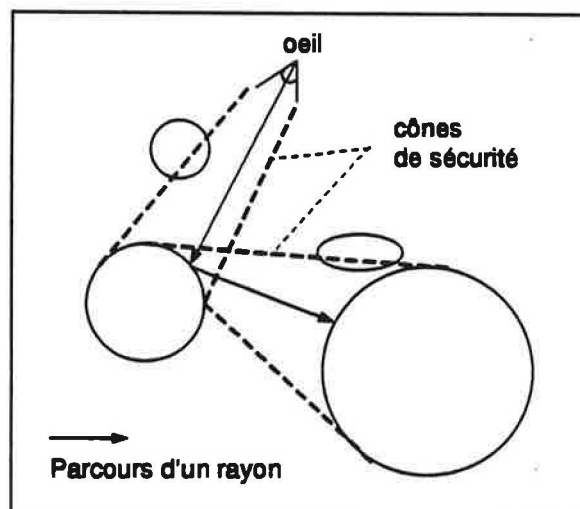
Figure 6 Cônes de sécurité
