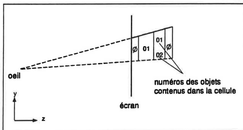
Figure 16 Obtention d'une cellule 3D à partir d'un rectangle de projection
