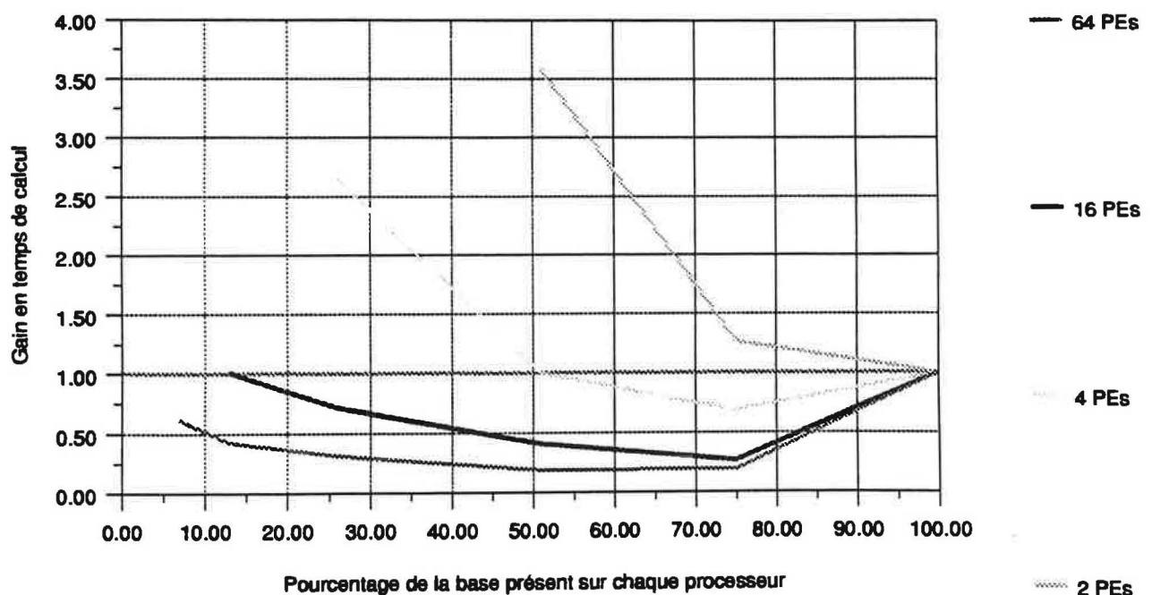
Figure 73 Gains en temps de l'algorithme à flots de calculs par rapport à l'algorithme à flots de données
