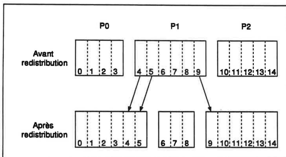
Figure 40 Redistribution de l'image
