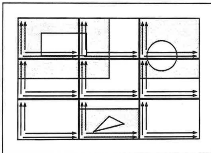
Figure 19 Parallélisation du raffinement des boîtes englobantes
