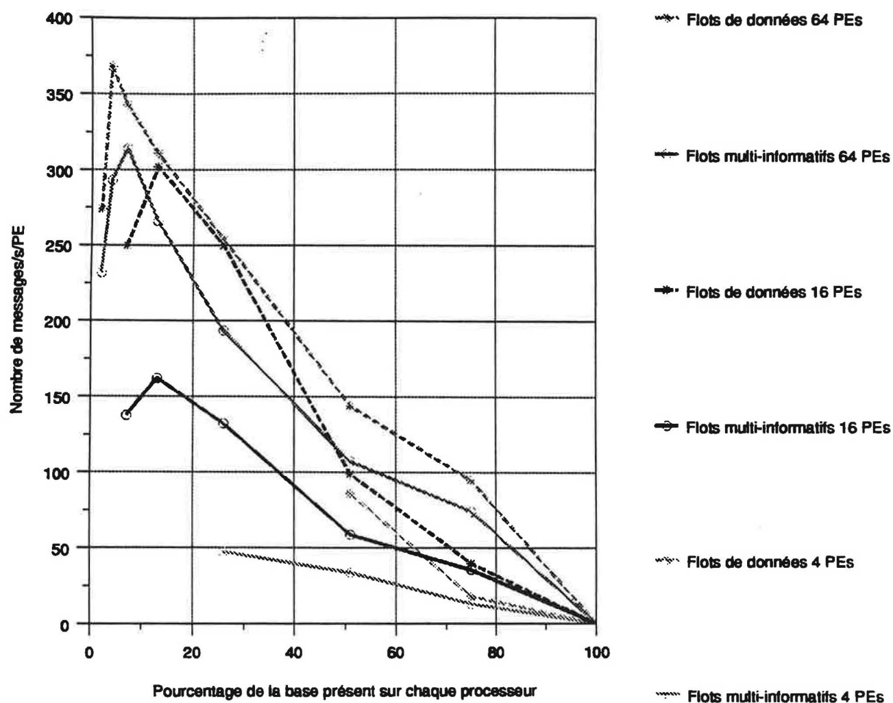
Figure 77 Comparaison du nombre de messages par seconde de l'algorithme à flots multi-informatifs et de l'algorithme à flots de données pour l'image M5
