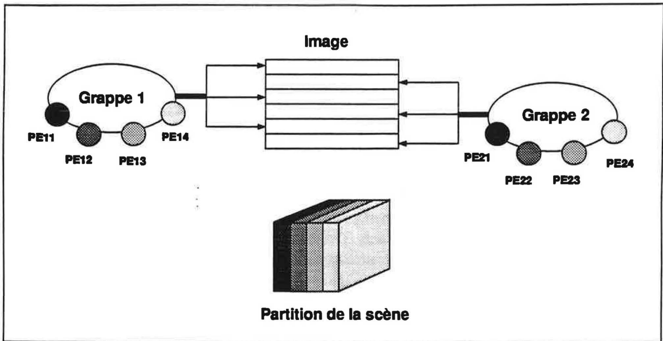
Figure 34 Architecture de la 'parallélisation hybride'
