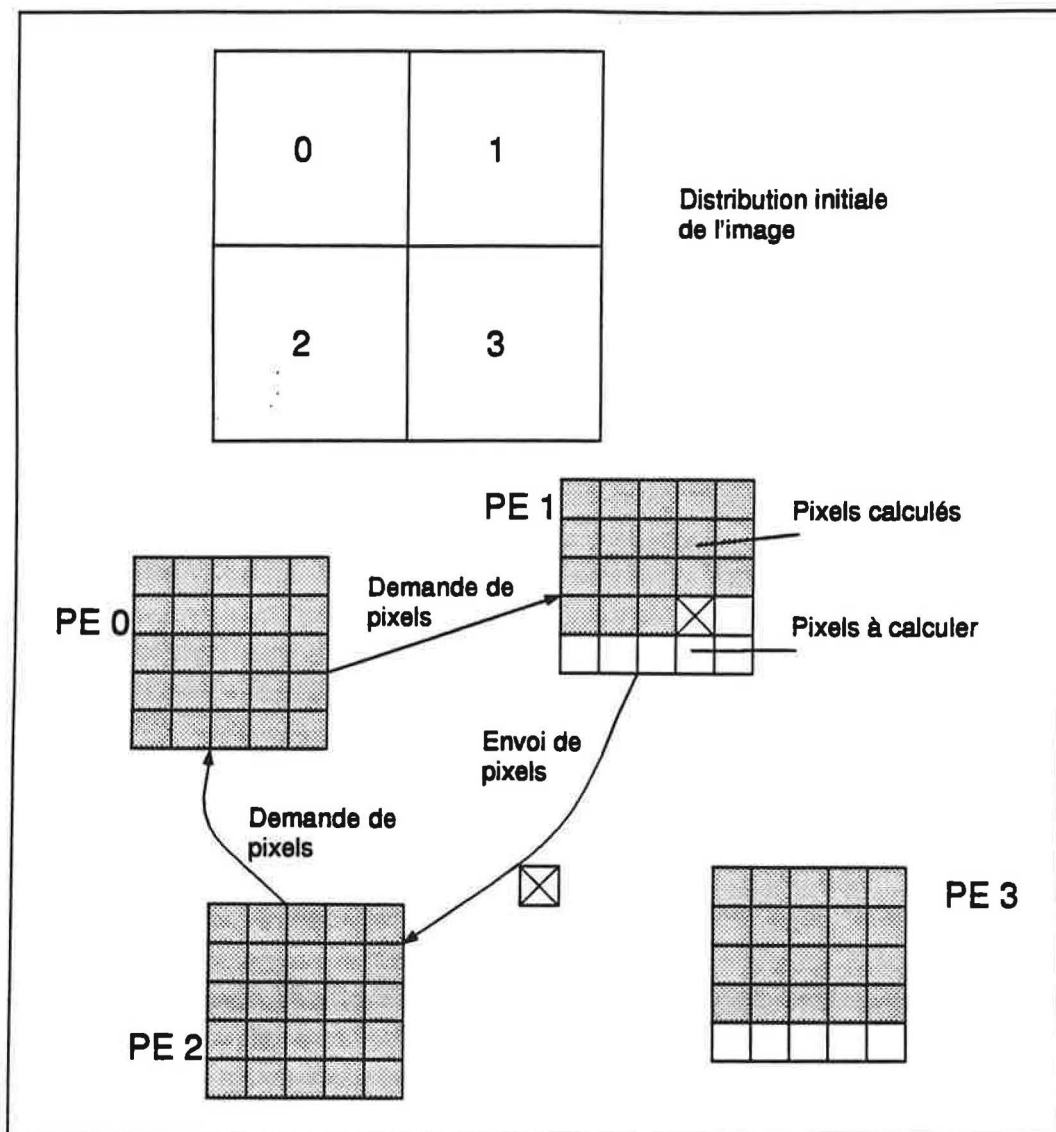
Figure 27 Distribution statique par blocs des pixels et équilibrage dynamique en anneau
