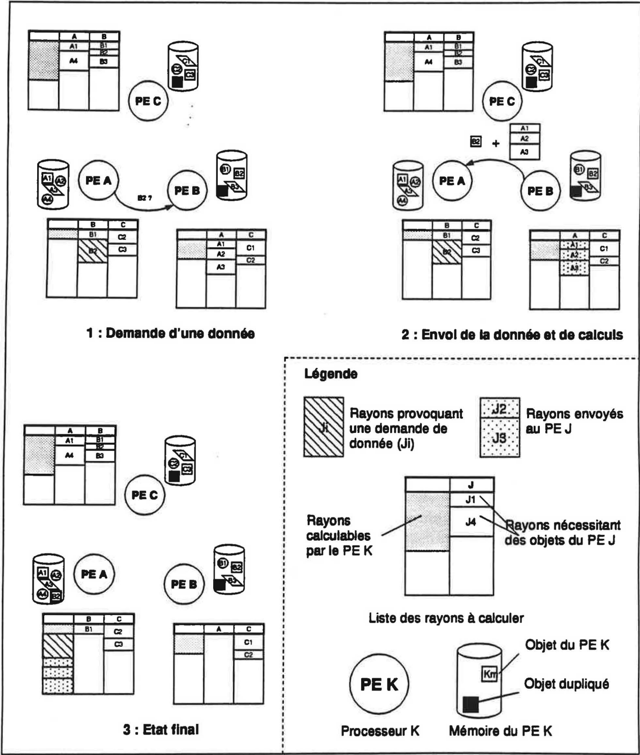
Figure 46 Schéma représentant l'envoi d'un message multi-informatif
