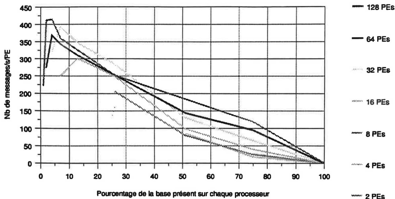
Figure 65 Nombre moyen de messages émis par PE par seconde pour M5
