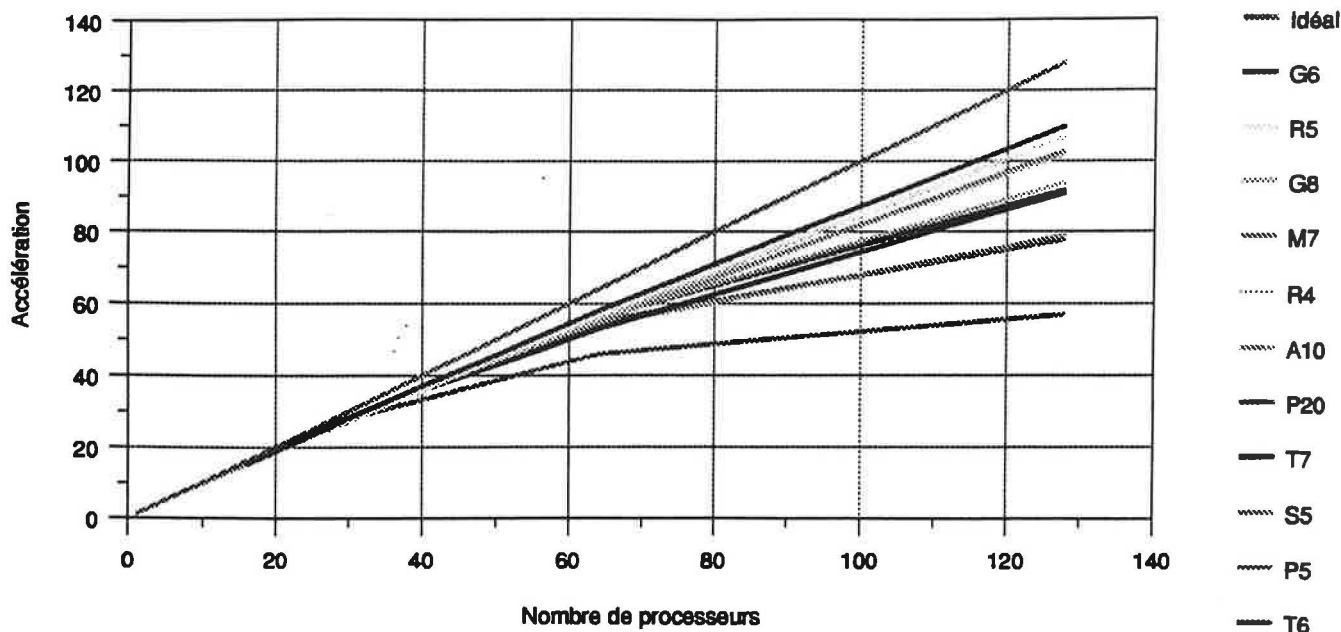
Figure 59 Accélération avec base dupliquée
