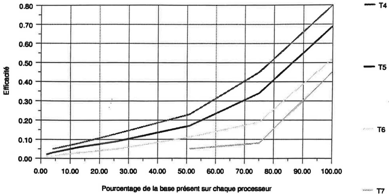
Figure 66 Efficacité pour 64 processeurs en fonction de la taille du cache pour l'image Tetrahedron avec des nombres de récursion différents.
