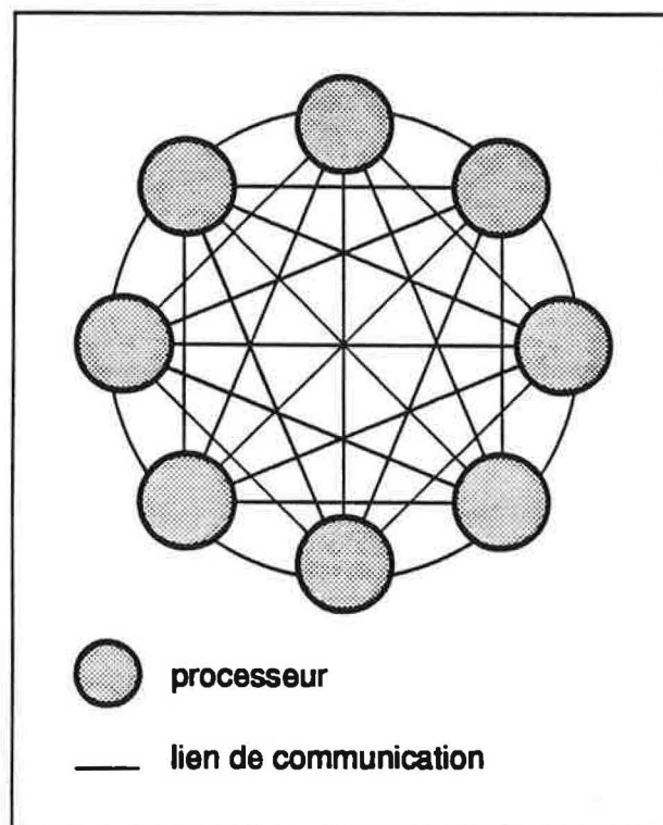
Figure 45 Réseau complètement connecté
