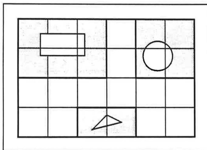
Figure 17 Construction de boîtes englobantes grossières à partir de voxels
