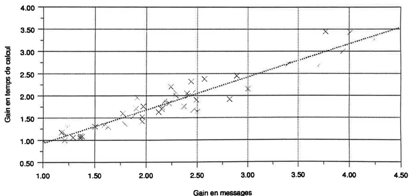
Figure 76 Relation entre gain en temps et gain en messages
