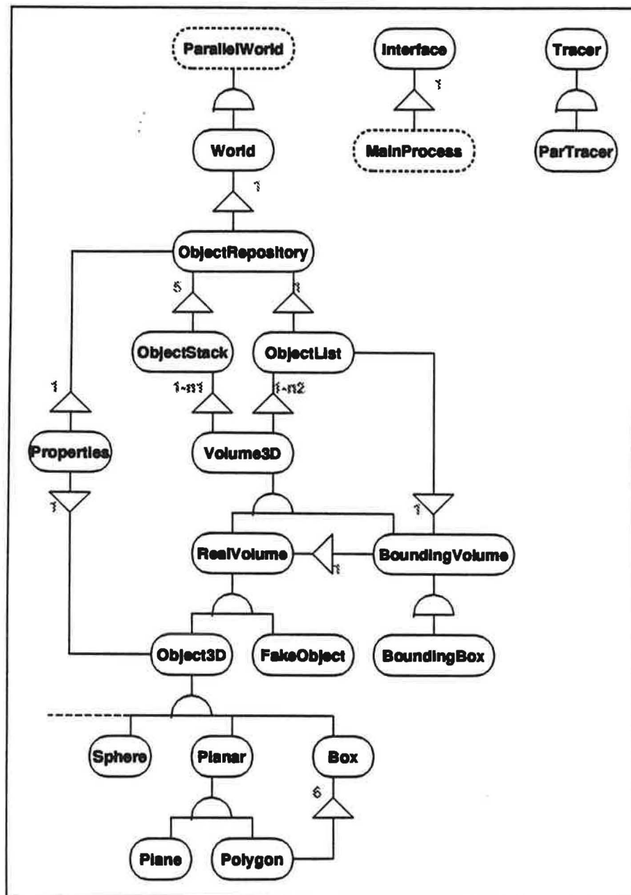
Figure 106 Diagramme objet du moteur d'intersection
