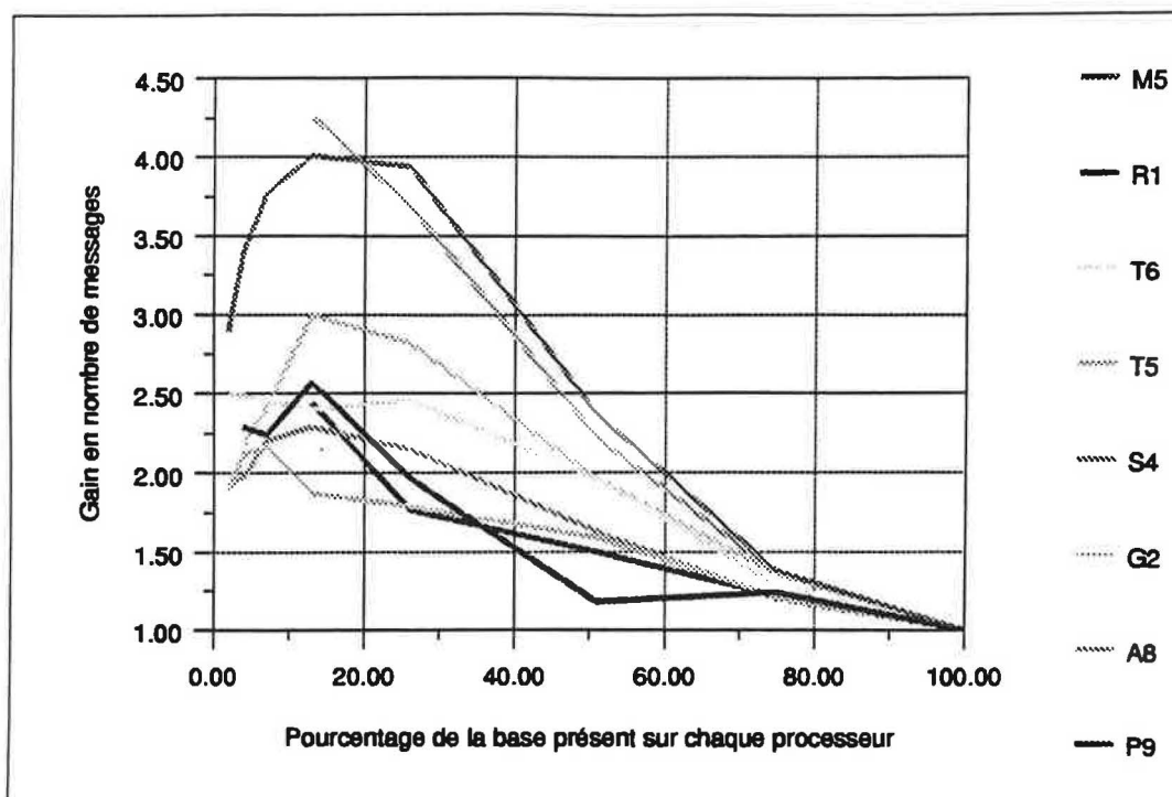
Figure 75 Gains en nombre de messages de l'algorithme à flots multi-informatifs par rapport à l'algorithme à flots de données
