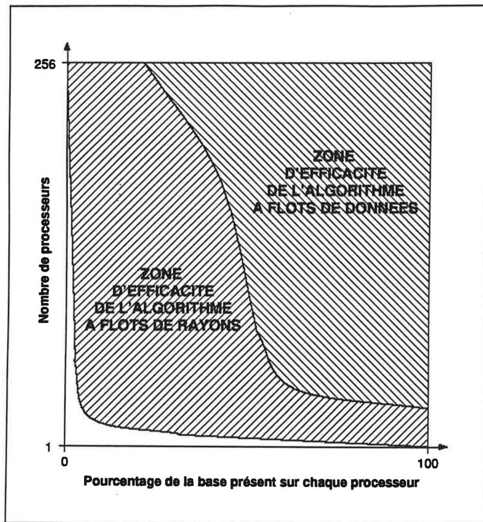
Figure 44 Zones d'efficacité des deux modèles
