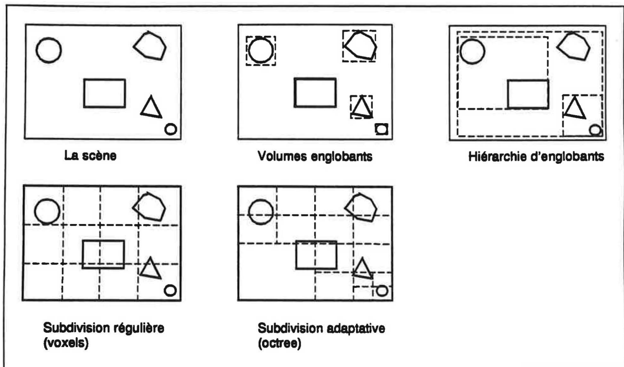
Figure 21 Les types d'accélération séquentielle les plus performants
