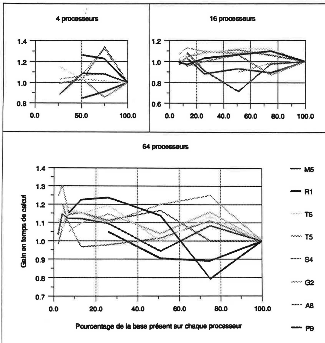
Figure 83 Gain en temps de l'algorithme à flots concurrents par rapport à l'algorithme à flots multi-informatifs
