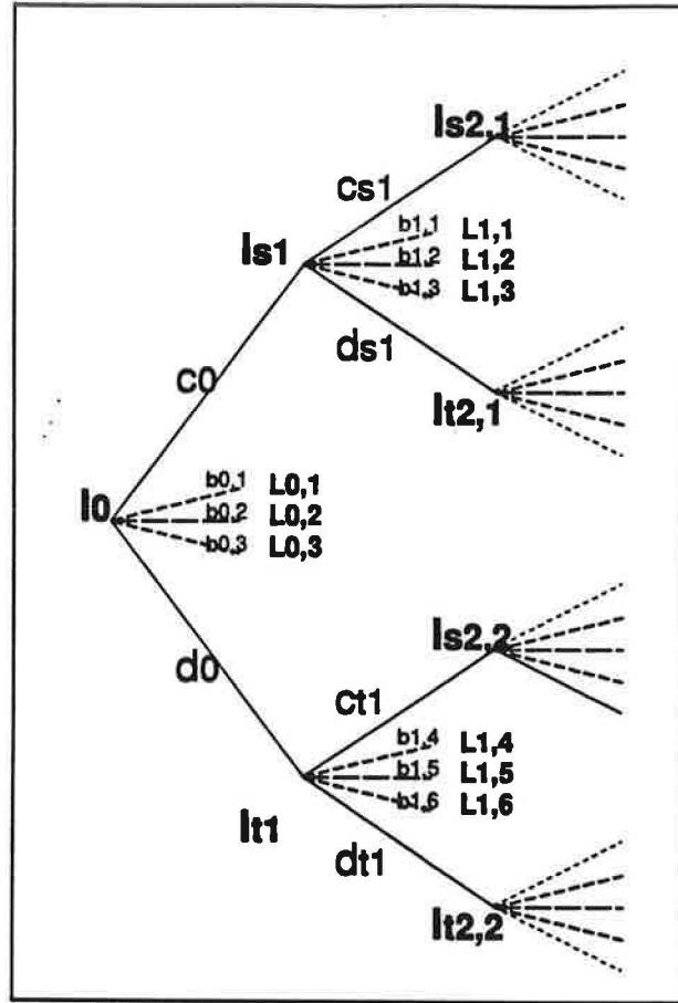
Figure 54 Arbre des rayons issus d'un pixel
