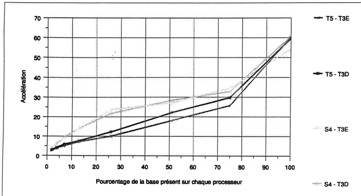
Figure 88 Accélération sur CRAY T3D et T3E avec 64 processeurs
