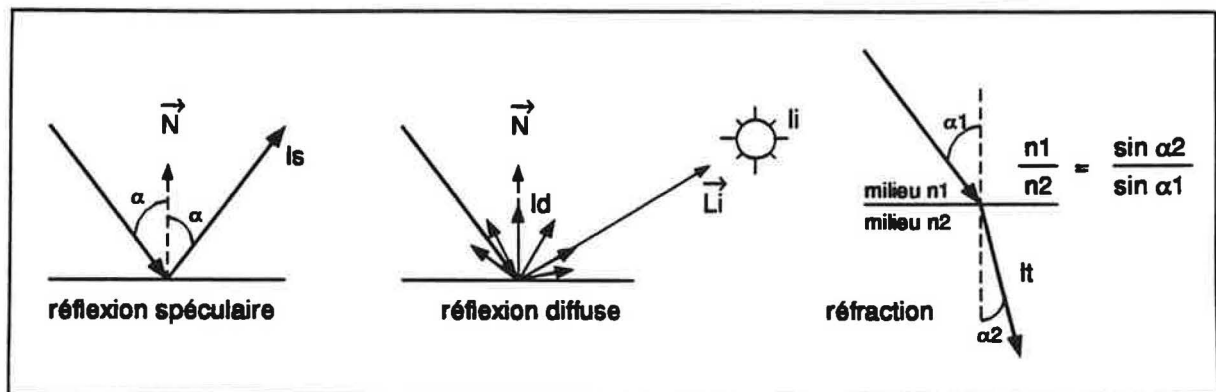
Figure 3 Réflexions et réfraction
