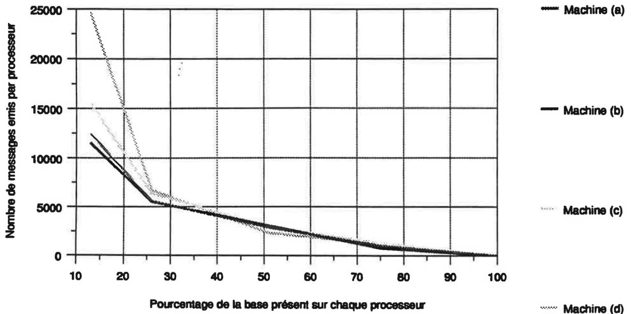
Figure 95 Nombre de messages émis sur les différentes machines
