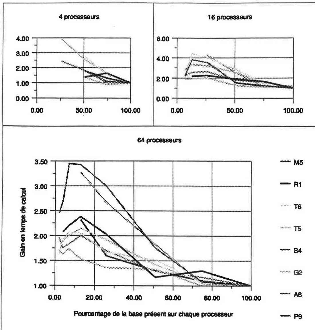
Figure 74 Gains en temps de l'algorithme à flots multi-informatifs par rapport à l'algorithme à flots de données
