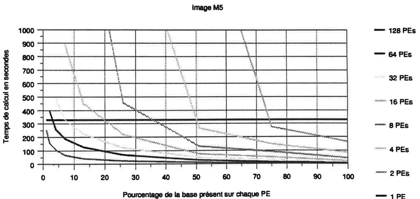
Figure 61 Temps de calcul en fonction de la distribution de la scène pour des images différentes pour des nombres de processeurs différents (Suite) ...
