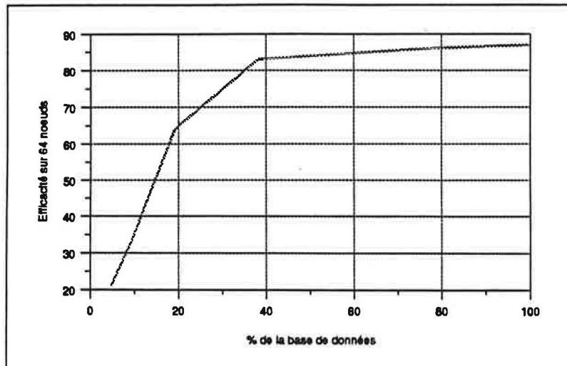
Figure 39 Mesures d'efficacité pour 64 processeurs données par Badouel pour l'image Mountain en fonction de la taille mémoire disponible pour chaque processeur
