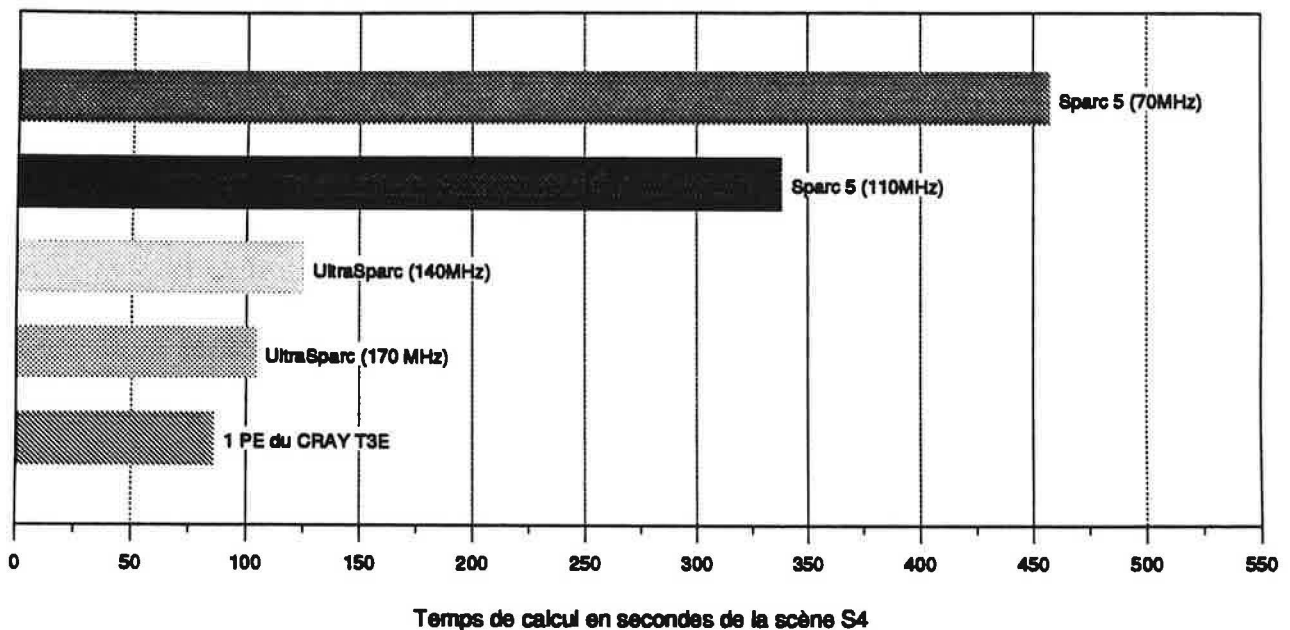
Figure 93 Temps de calcul de la scène S4 pour différents types de processeur
