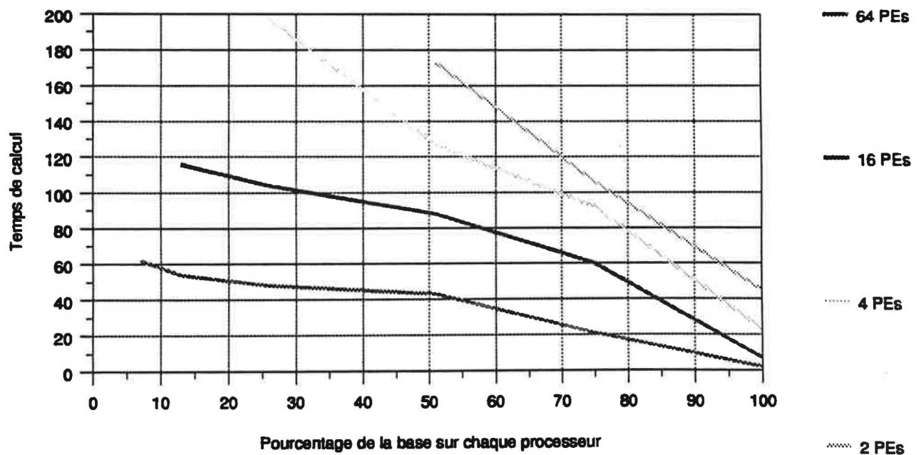
Figure 70 Temps de calcul pour l'image T5
