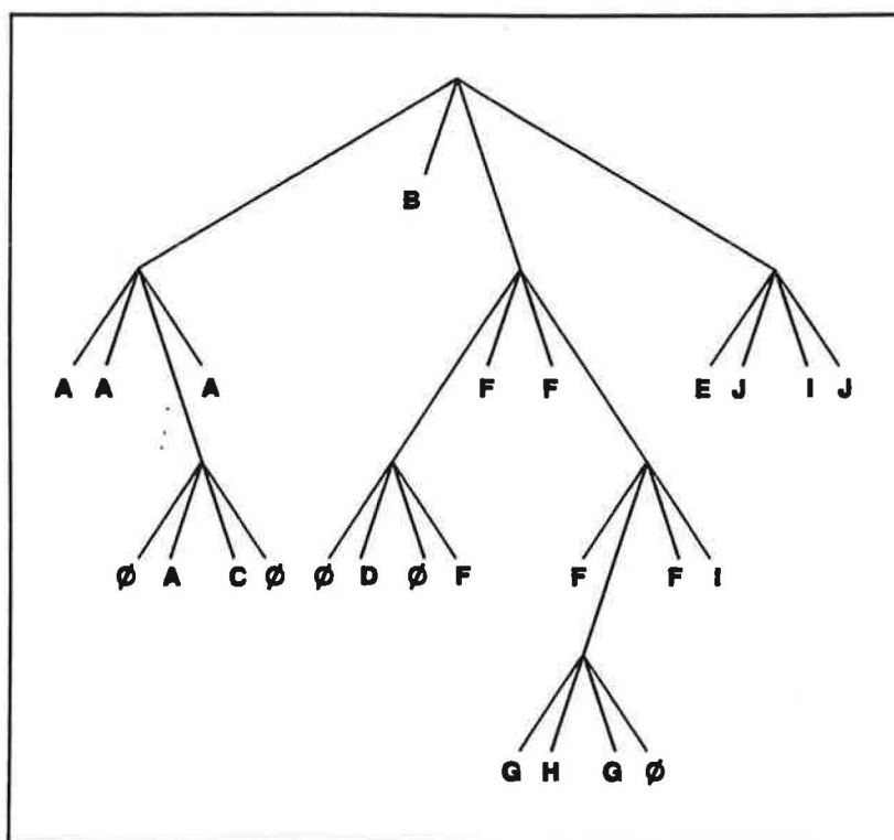
Figure 11 Arbre de découpage en quadtree d'une scène 2D
