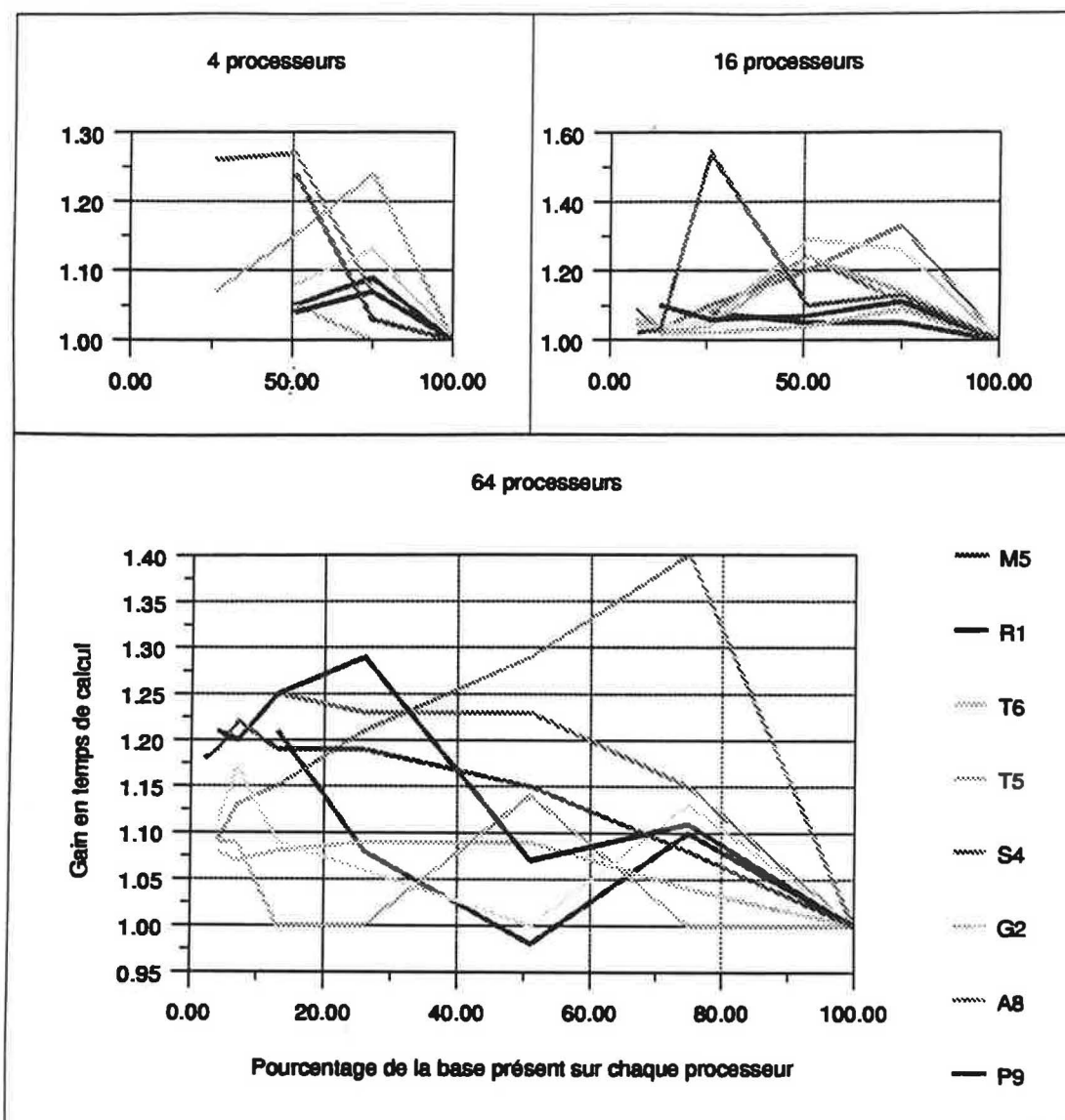
Figure 67 Gains en temps de l'algorithme à flots de données avec équilibrage par rapport à l'algorithme à flots de données sans équilibrage
