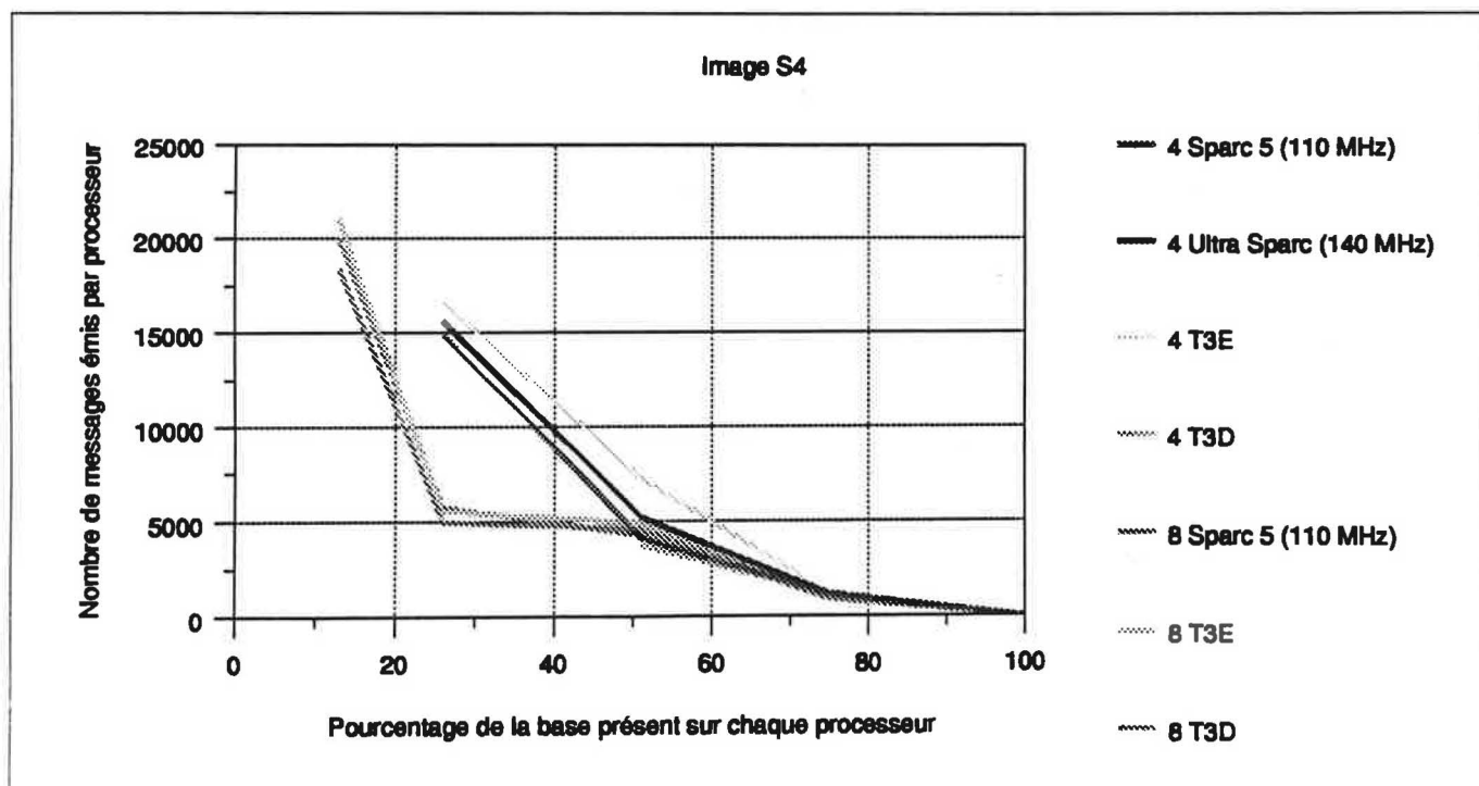
Figure 91 Comparaison du nombre de messages émis avec 4 et 8 processeurs sur des architectures variées (image S4)
