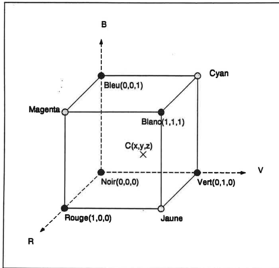
Figure 50 Modèle de couleur RVB
