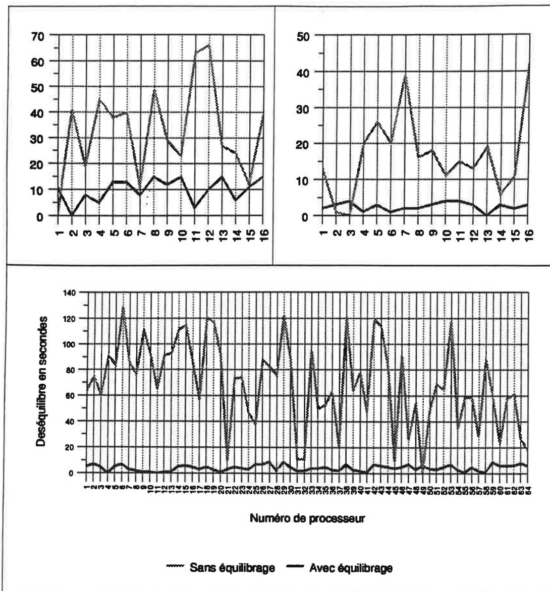
Figure 69 Ré-équilibrage de la charge de chaque processeur
