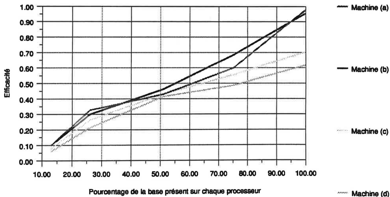
Figure 94 Efficacité des différentes machines
