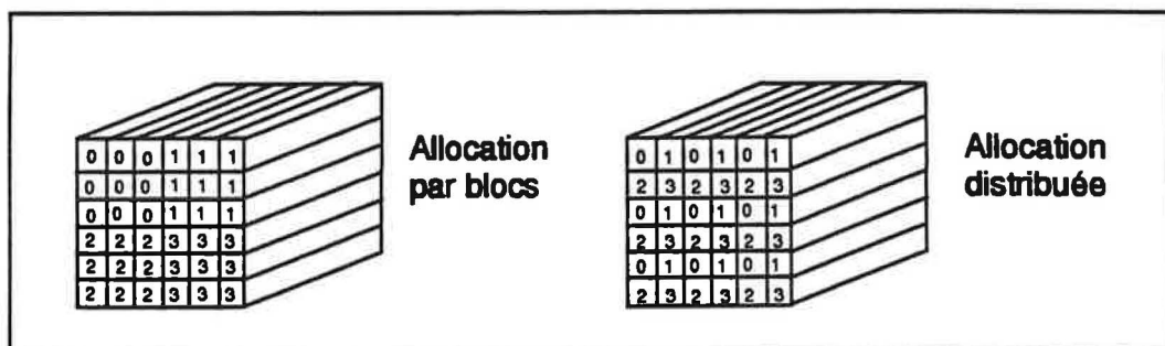
Figure 30 Allocation distribuée et allocation par blocs
