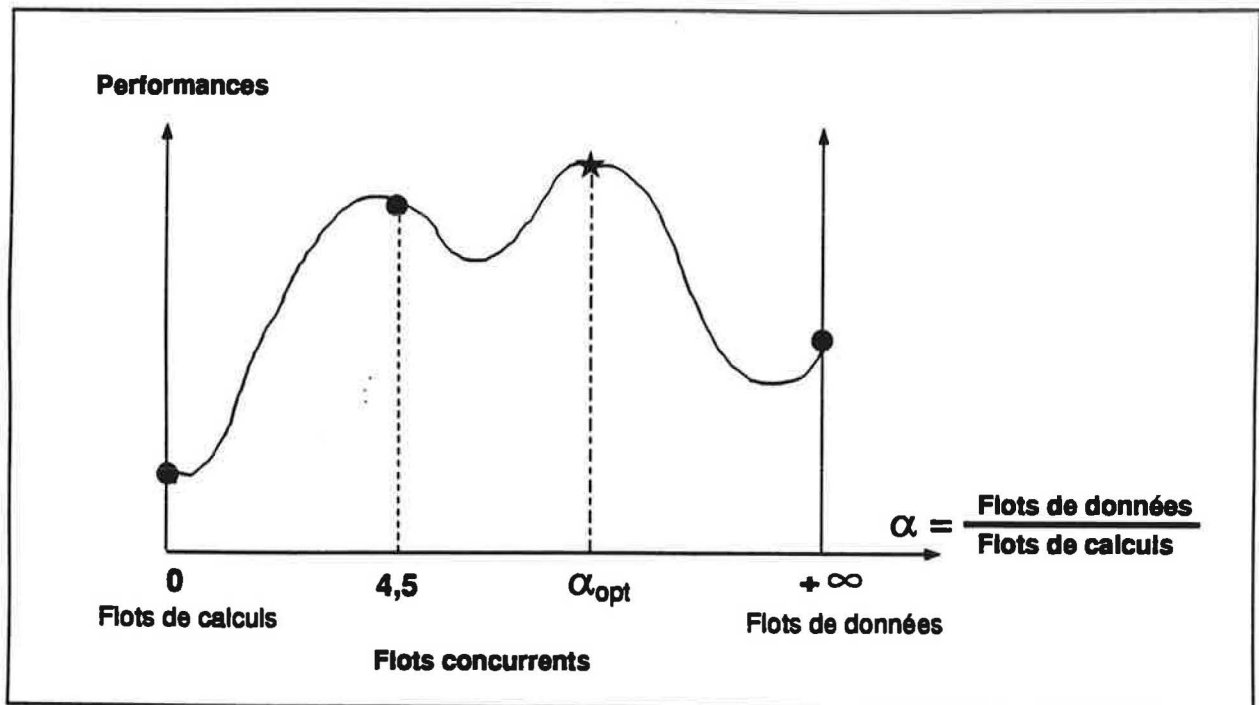
Figure 85 Etude des performances de l'algorithme à flots concurrents en fonction du rapport entre le nombre de messages d'envoi de données et le nombre de messages d'envoi de calculs.
