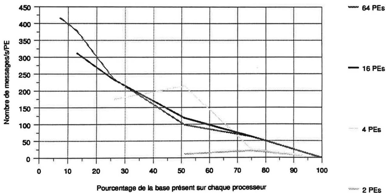
Figure 72 Nombre de messages
