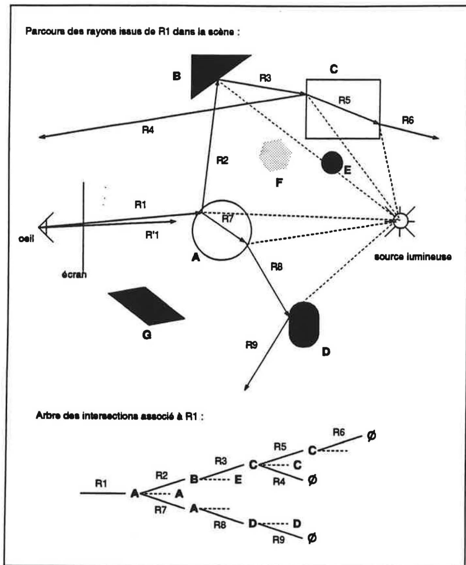
Figure 4 Arbre des intersections d'un rayon
