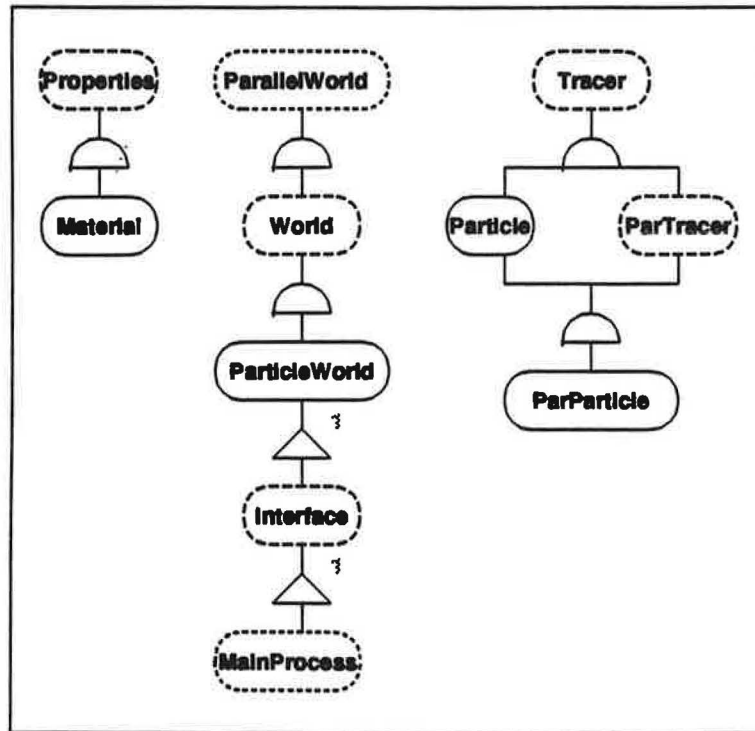
Figure 108 Diagramme objet du module particulaire
