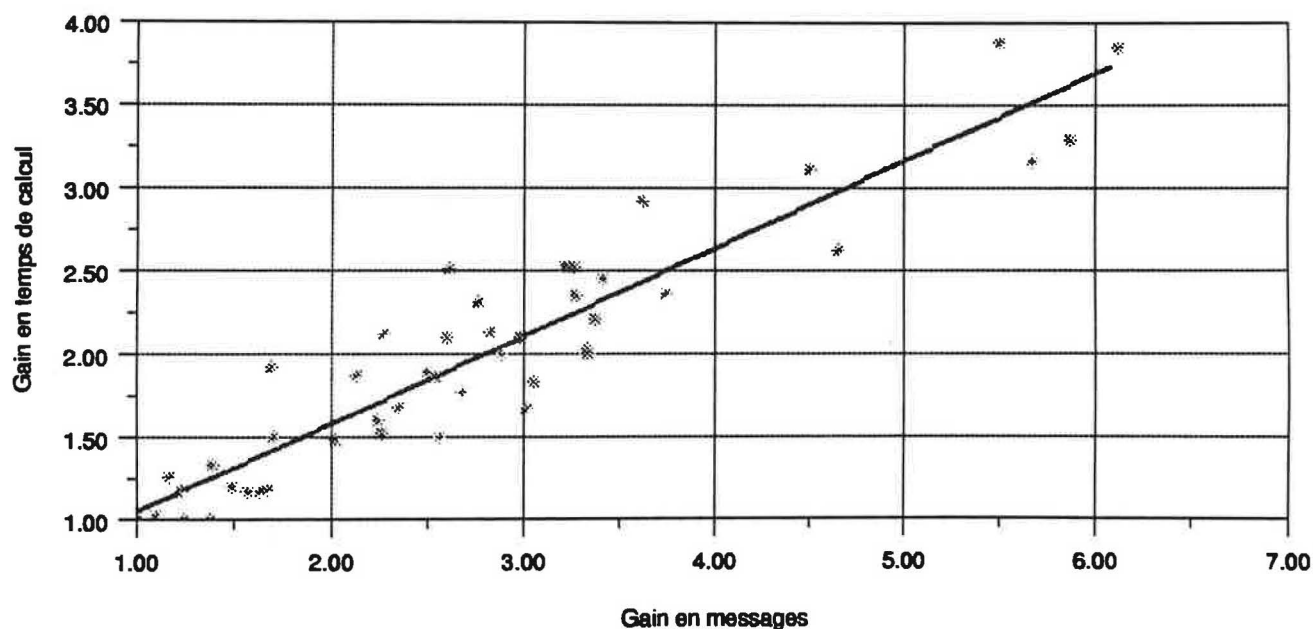
Figure 80 Relation entre gain en temps et gain en messages
