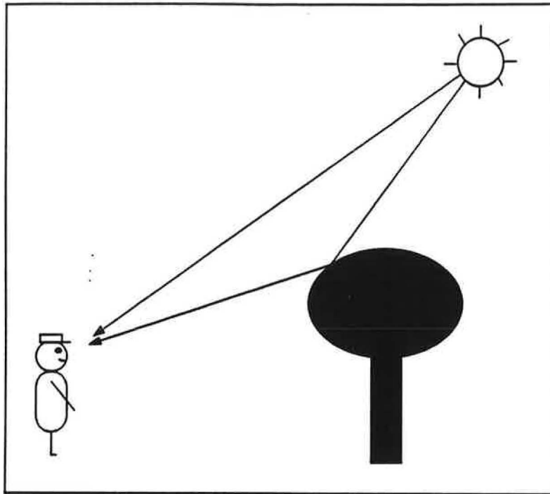
Figure 1 Parcours des photons permettant la formation d'une image pour un observateur
