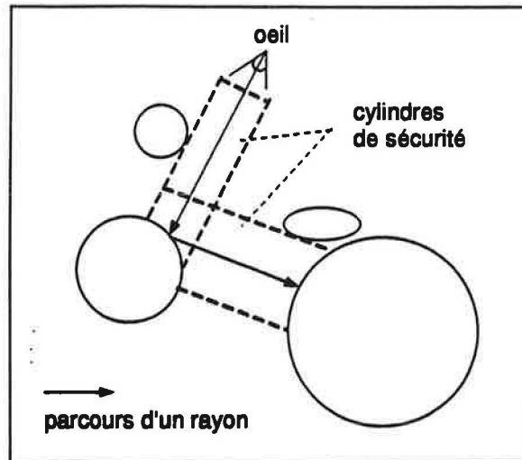
Figure 5 Cylindres de sécurité
