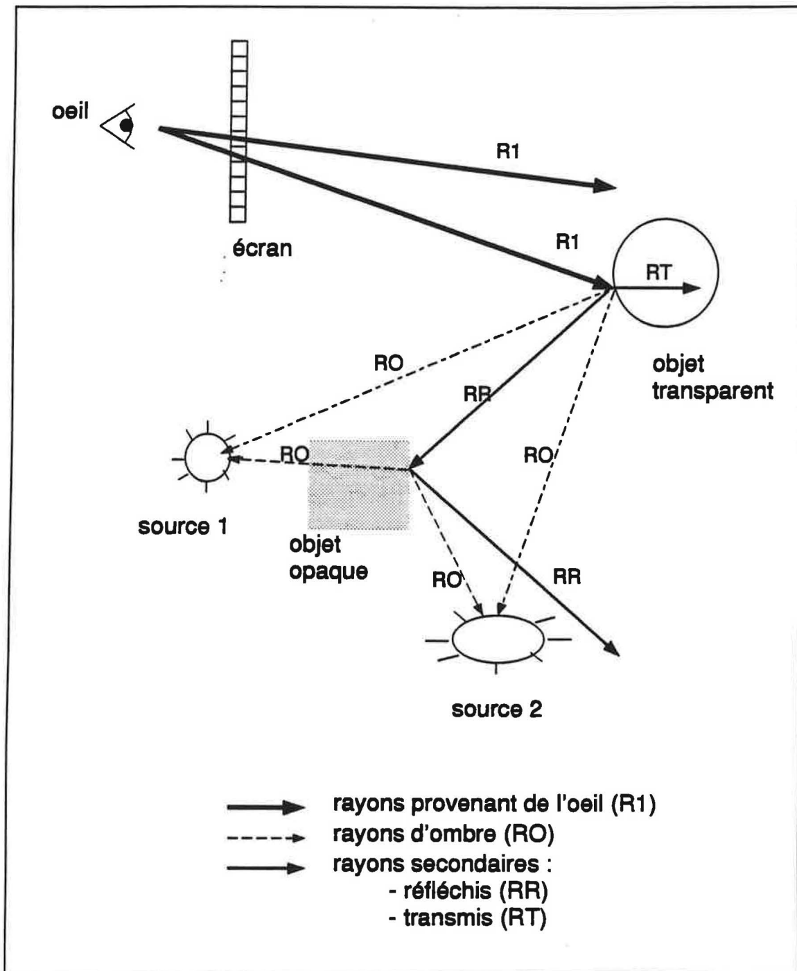
Figure 2 Parcours des rayons lumineux pendant l'algorithme de lancer de rayon
