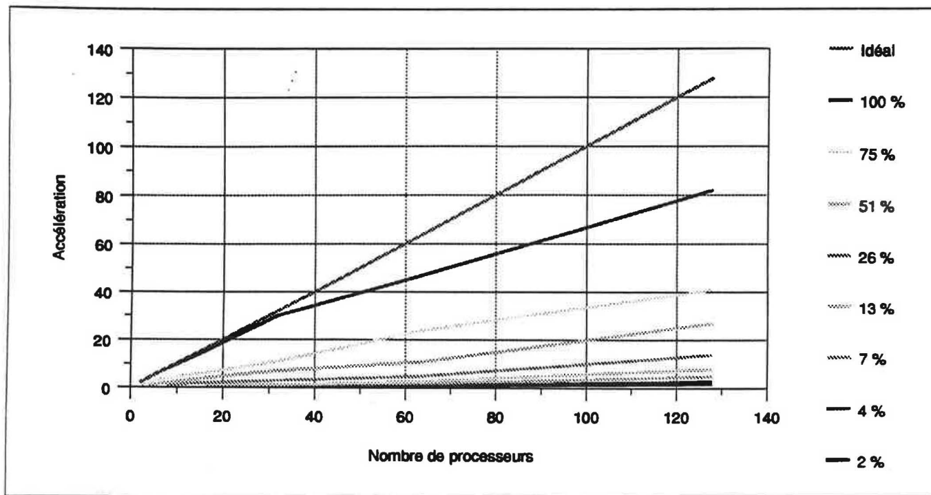
Figure 64 Accélération pour une distribution donnée en fonction du nombre de processeurs pour l'image M5.
