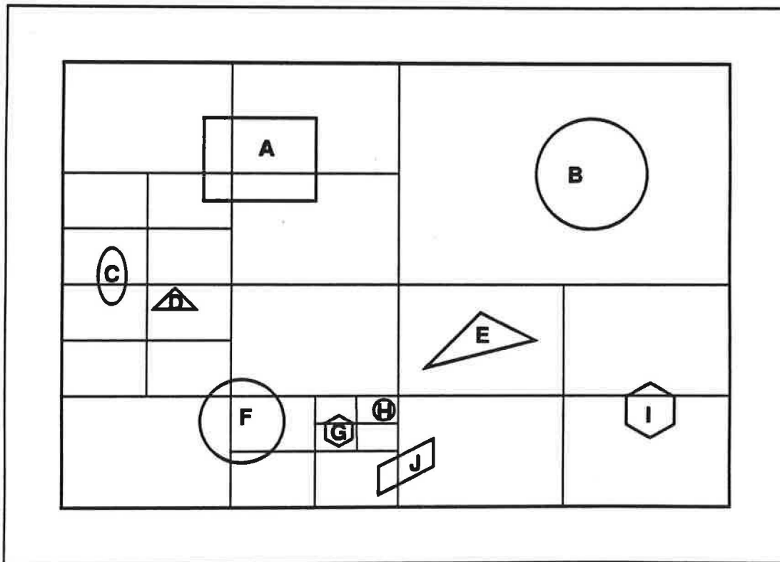
Figure 10 Découpage en quadtree d'une scène 2D
