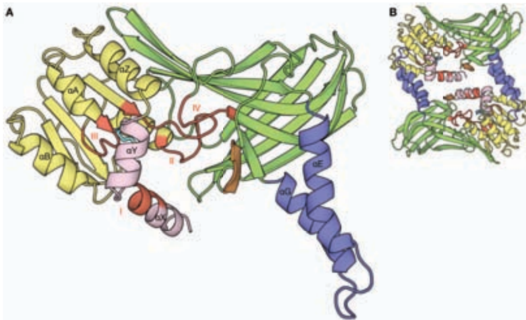
Figure 10 - Structure du domaine catalytique de la protéine CARM1 de souris (PDB : 3B3F) [153]
