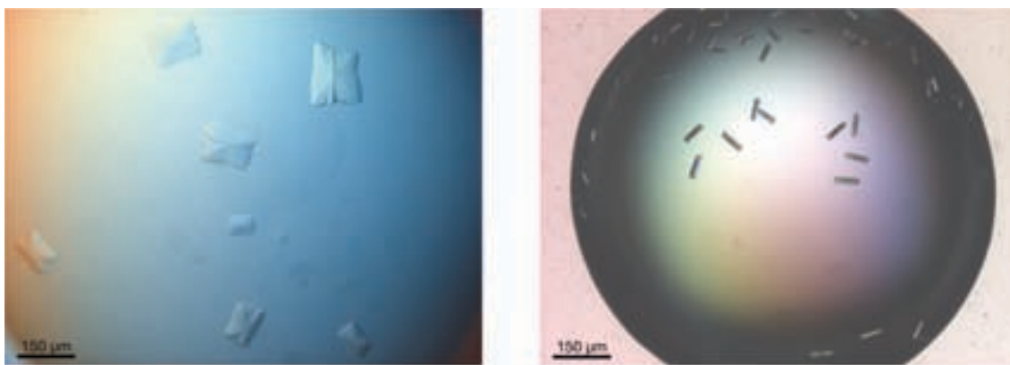
Figure 22 - Cristaux classiques de mCARM1 130-487
