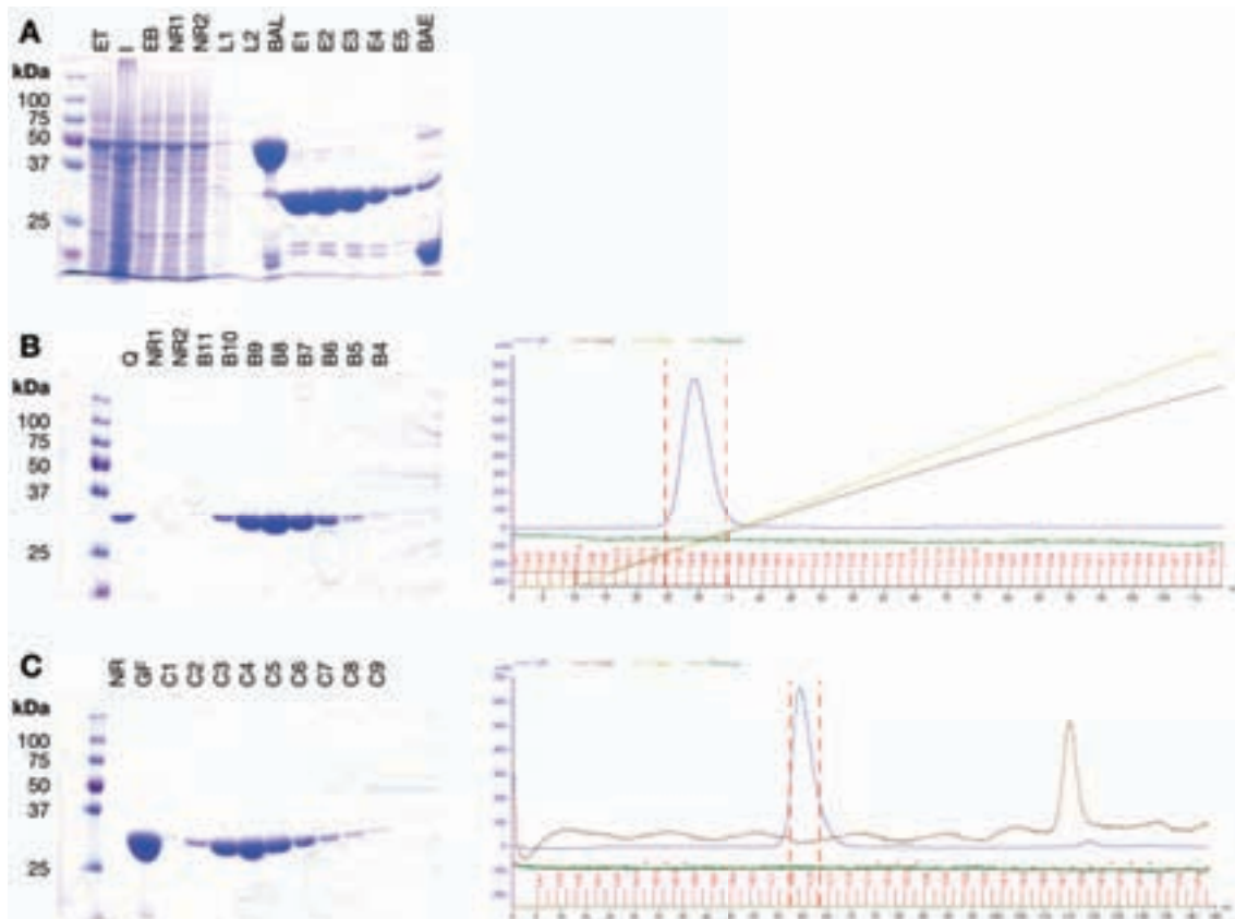
Figure 16 - Gels et chromatogrammes pour les différentes étapes de purification de mCARM1 130-507
