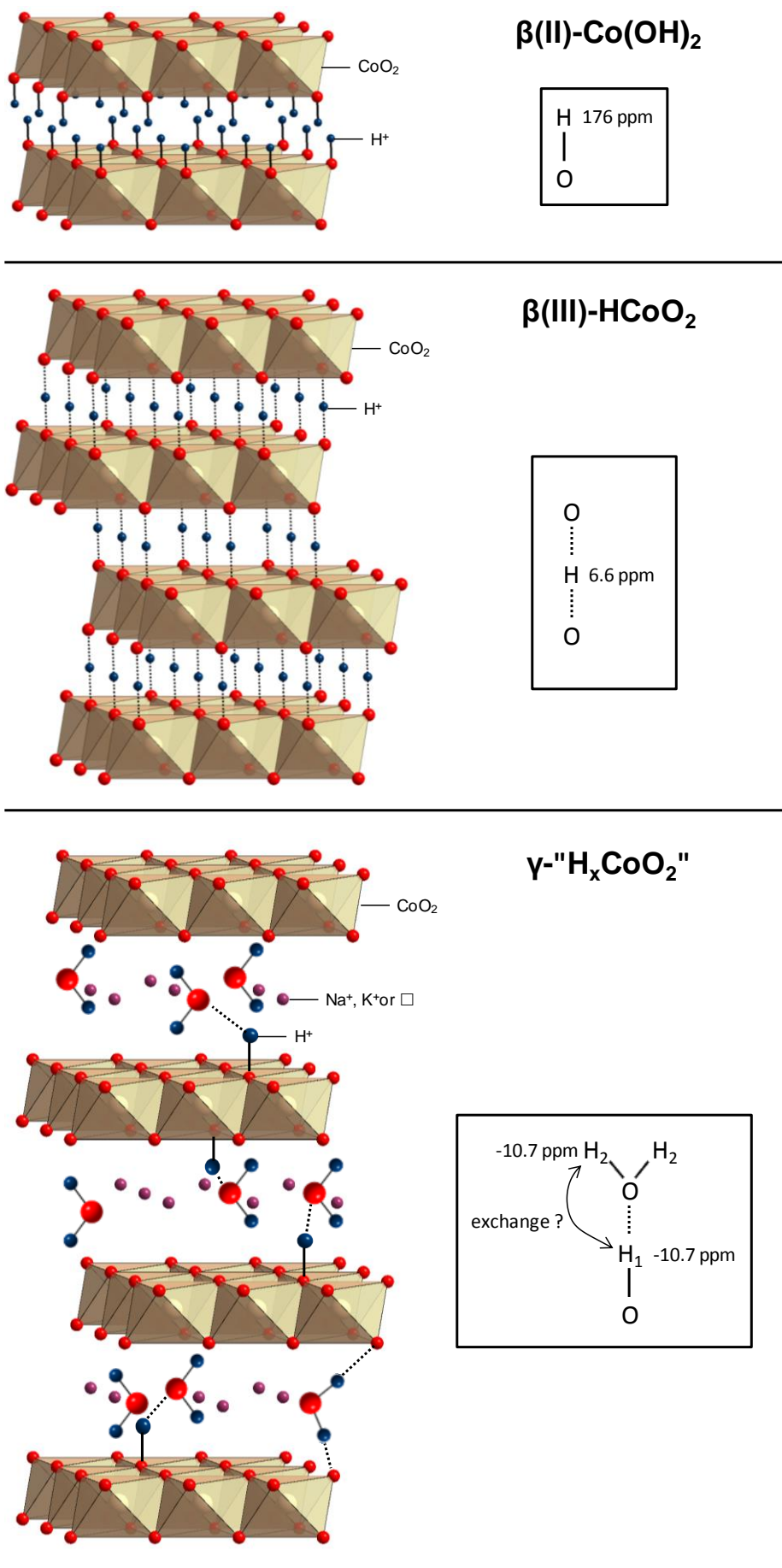
Figure III-22 : Représentations schématices des structures des phases \beta(\text{II})\text{-Co(OH)}_2 , \beta(\text{III})\text{-HCoO}_2 et \gamma\text{-}^{\text{H}}\text{CoO}_2 . Dans les liaisons O-H, les traits pleins traduisent des liaisons chimiques (essentiellement covalentes), alors que les traits pointillés illustrent des liaisons physiques (liaisons hydrogène). La représentation de l'espace interfeuillet de \gamma\text{-}^{\text{H}}\text{CoO}_2 est arbitraire. M. Butel a montré la présence d'ions \text{Na}^+ , \text{K}^+ et d' \text{H}_2\text{O} , mais nous n'avons pas d'information sur leur répartition, pas plus que sur l'orientation des molécules d'eau [41].
