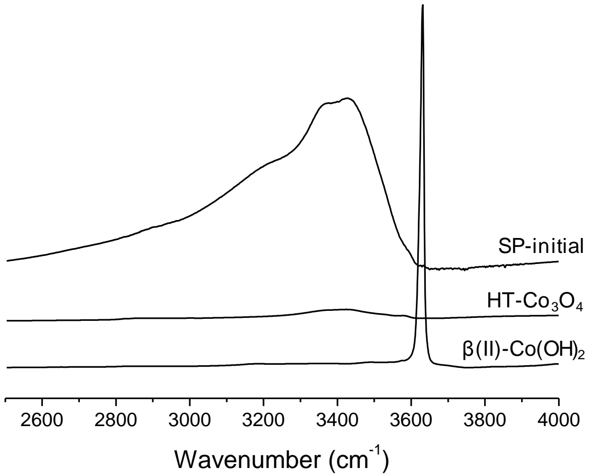
Figure III-14 : Comparaison des spectres IR haute fréquence des matériaux \beta(\text{II})\text{-Co}(\text{OH})_2 , \text{HT-Co}_3\text{O}_4 et SP-initial. Les spectres ont été normalisés par rapport à l'intensité intégrée de la bande Co-O basse fréquence vers 568 \text{ cm}^{-1} (non représentée ici).
