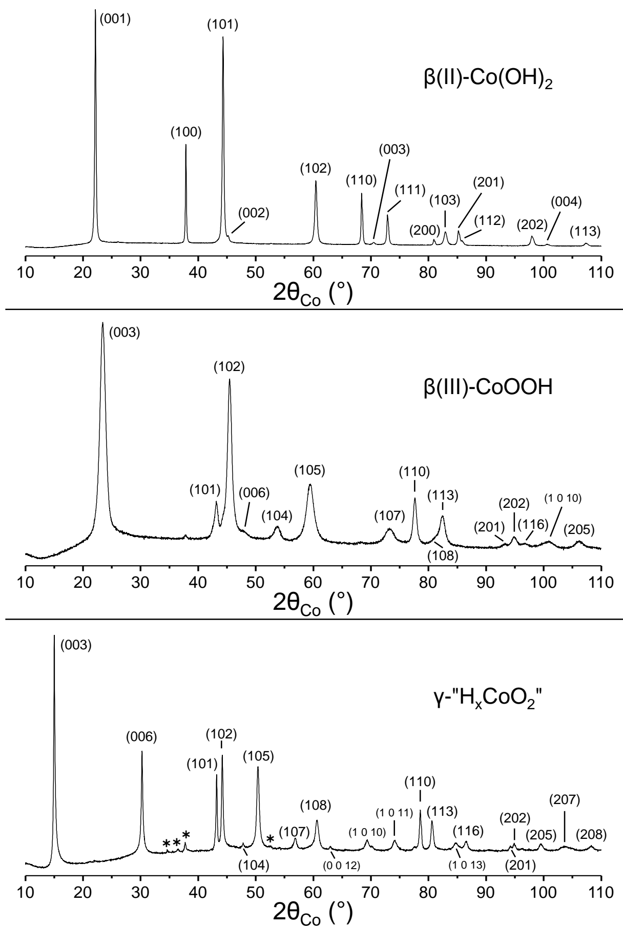
Figure I-8 : Diagrammes de diffraction des rayons X des principales phases au cobalt indexées dans le système hexagonal. Les astérisques (*) marquent les raies correspondant à une phase résiduelle Na_2CO_3 .
