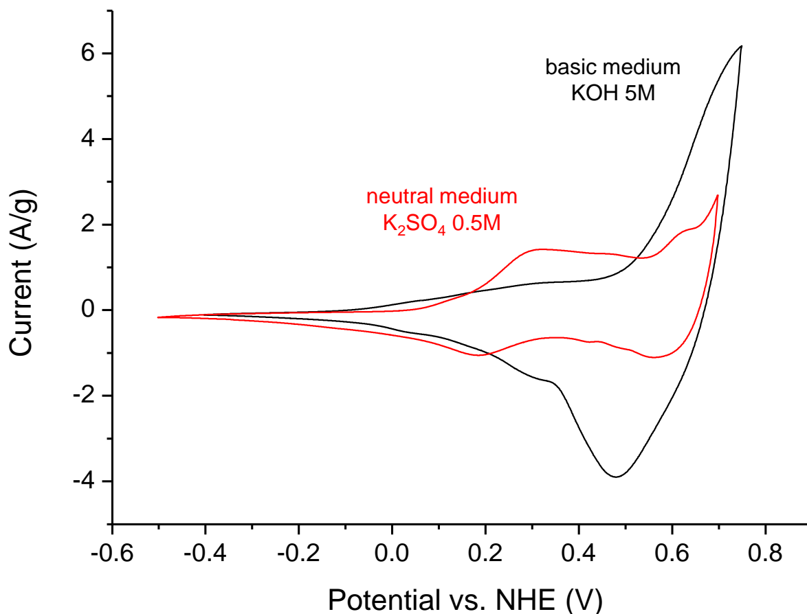
Figure IV-19 : Voltammogrammes, d'une électrode préparée à partir de SP-initial et contenant de 5% de noir de carbone, enregistrés à 5 mV/s dans deux électrolytes différents : KOH 5M et \text{K}_2\text{SO}_4 0,5M.
