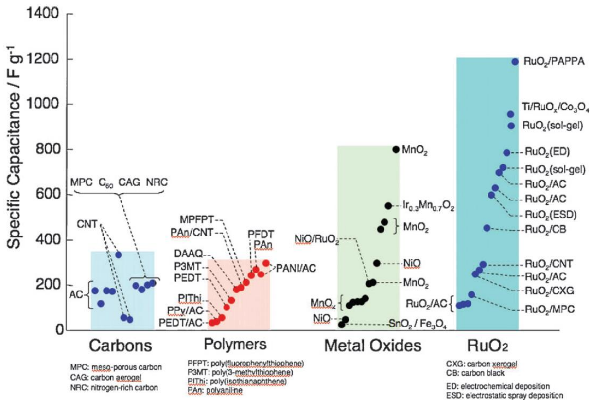
Figure 1-3 : Comparaison des capacités des principaux systèmes de supercondensateurs [14].
