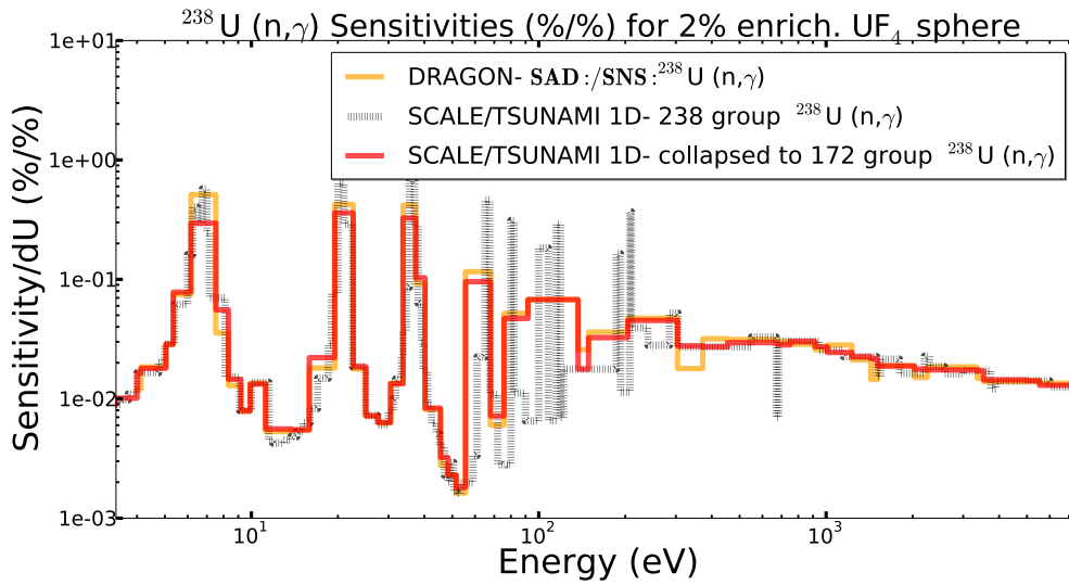
Figure 2.5: composante négatif de la sensibilité du k_{eff} pour l' ^{238}\text{U} U(n,e) dans la région de résonance (en % / %).
