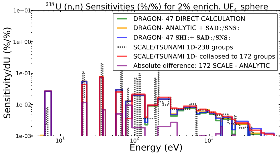
Figure 2.4: composante positive de la sensibilité du k_{eff} pour l' ^{238}\text{U} U(n,e) dans la région de résonance (en % / %).
