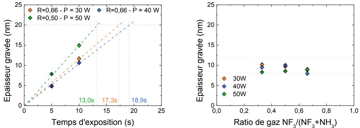
a) b) Figure 5.7 : a) Extrapolation du régime linéaire jusqu'à 20 nm pour des conditions de gravure à faible E_{crit} ; b) Epaisseurs gravées sur plaque avec motifs pour toutes les conditions plasma, après ajustements du temps d'exposition des conditions de gravure non-linéaire.
