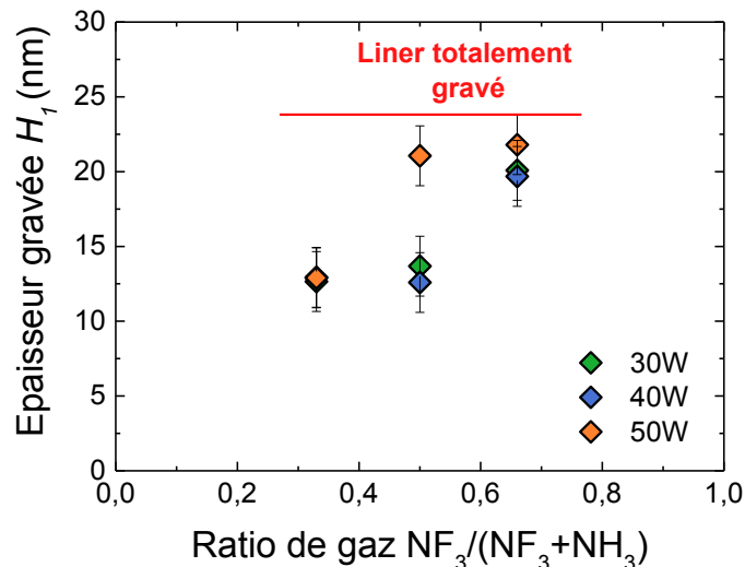
Figure 5.33 : Epaisseur gravée au-dessus du masque dur ( H_1 ) en fonction du ratio de gaz, pour des petites zones actives et des STI étroites, une gravure visée de 20 nm sur pleine plaque et différentes puissances plasma.
