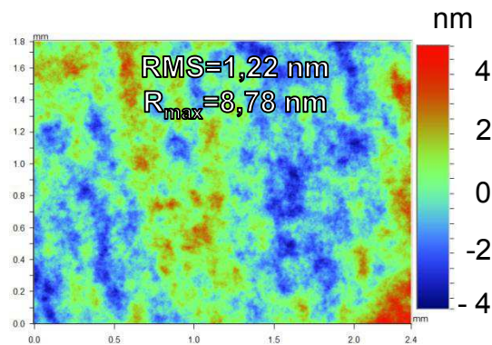
Figure 2.24 : Cliché réalisé par profilométrie optique d'un film de \text{SiO}_2 déposé par SACVD TEOS/ \text{O}_3 puis gravé par le procédé Siconi (surface de 1,8x2,4 mm 2 ).
