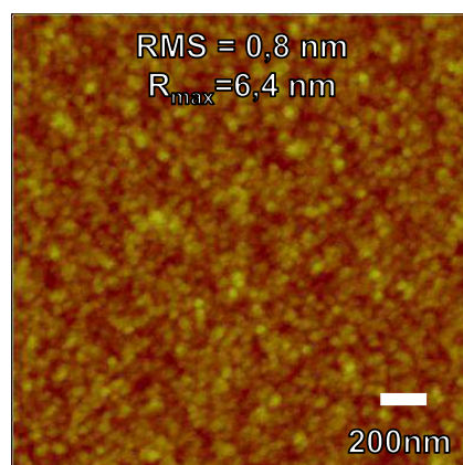
Figure 2.22 : Cliché AFM d'un film de SiO 2 de 40 nm d'épaisseur déposé par SACVD TEOS/O 3 (surface de 2x2 μm 2 ).
