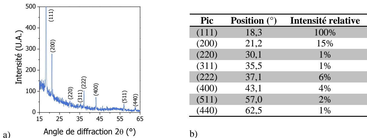
Figure 4.8 : a) Spectre XRD de la couche de sels fluorés (NH 4 ) 2 SiF 6 générée durant l'exposition au plasma ; b) Tableau des caractéristiques des différents pics observés (identification, position et intensité relative).
