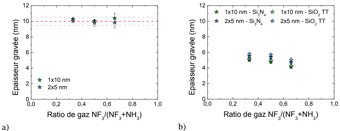
Figure 5.1 : a) Epaisseur gravée sur pleine plaque en fonction du ratio de gaz pour des gravures de 1x10 nm et 2x5 nm et une puissance de 50 W ; b) Epaisseur gravée sur plaque avec motifs pour les mêmes gravures.
