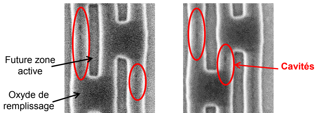
Figure 5.43 : Clichés MEB en vue de dessus réalisés dans les SRAM de la technologie CMOS 14 nm pour un remplissage avec un procédé SACVD TEOS/O 3 standard.
