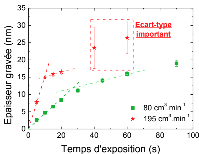
Figure 4.35 : Cinétique de gravure pour un débit total de gaz réactif \text{NF}_3+\text{NH}_3 de 80 et 195 \text{ cm}^3.\text{min}^{-1} avec un ratio de gaz de 0,50 et une puissance de 50 W.
