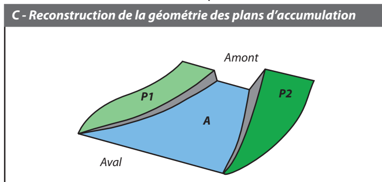
Figure M8 - Reconstruction des profils et de la géométrie des plans d'accumulation
