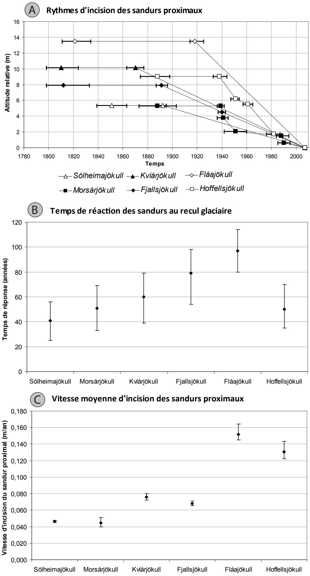
Figure R24 - L'incision des sandurs proximaux
