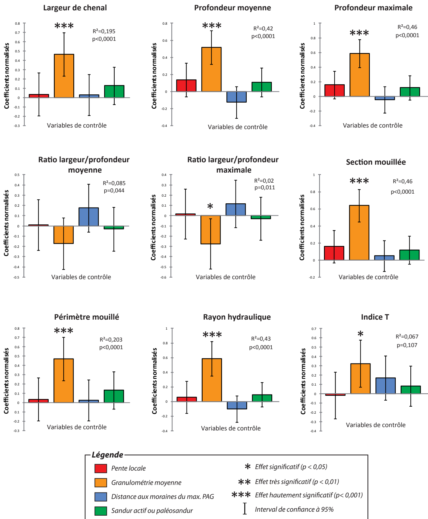
Figure R32 - Coefficients de régression normalisés issus des analyses de covariance
