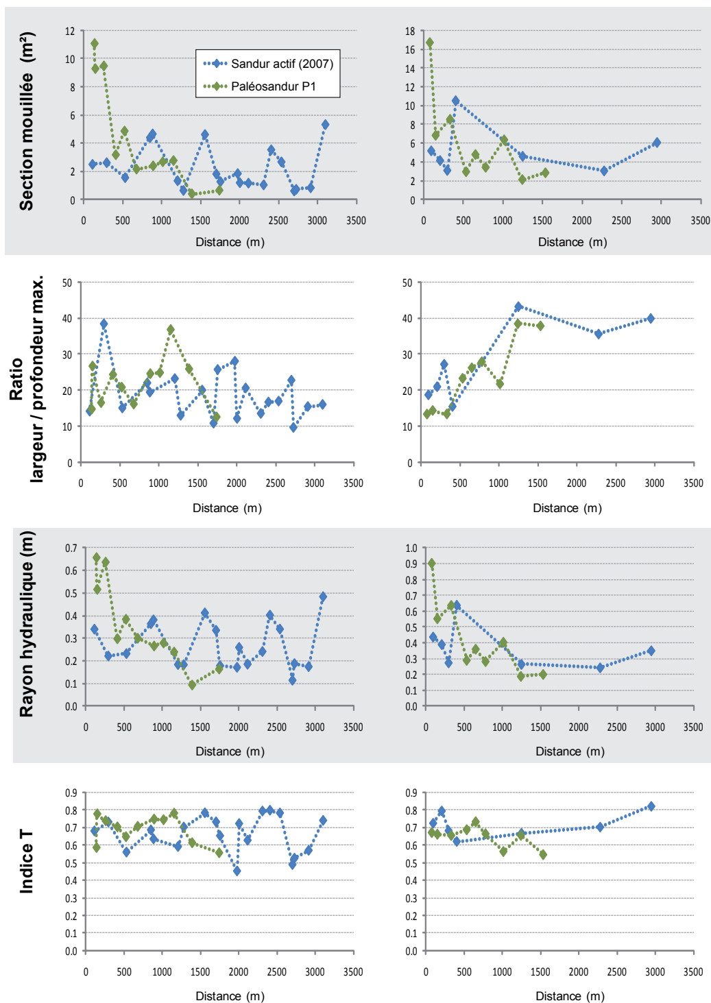
Figure R31 - Ajustement post-PAG de l'évolution amont-aval de la géométrie de chenal
