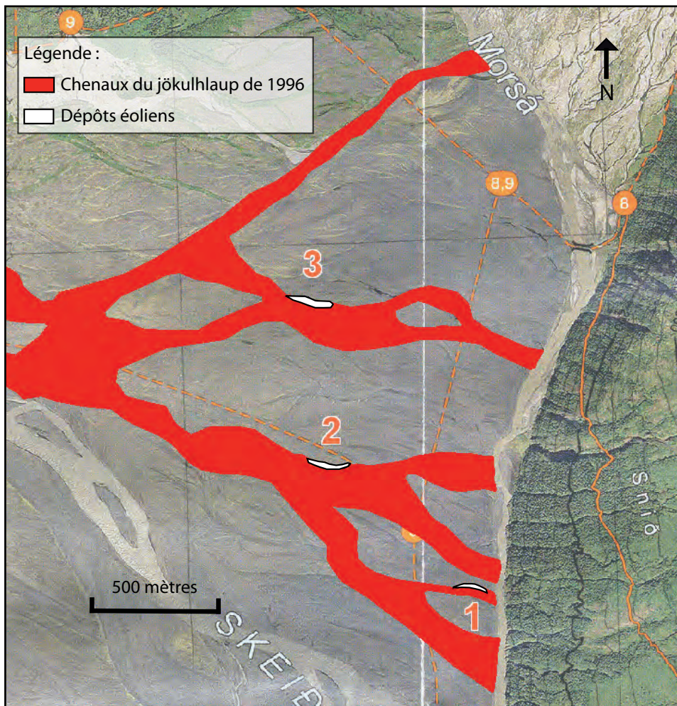
Figure A3 - Carte de localisation des dépôts éoliens échantillés
