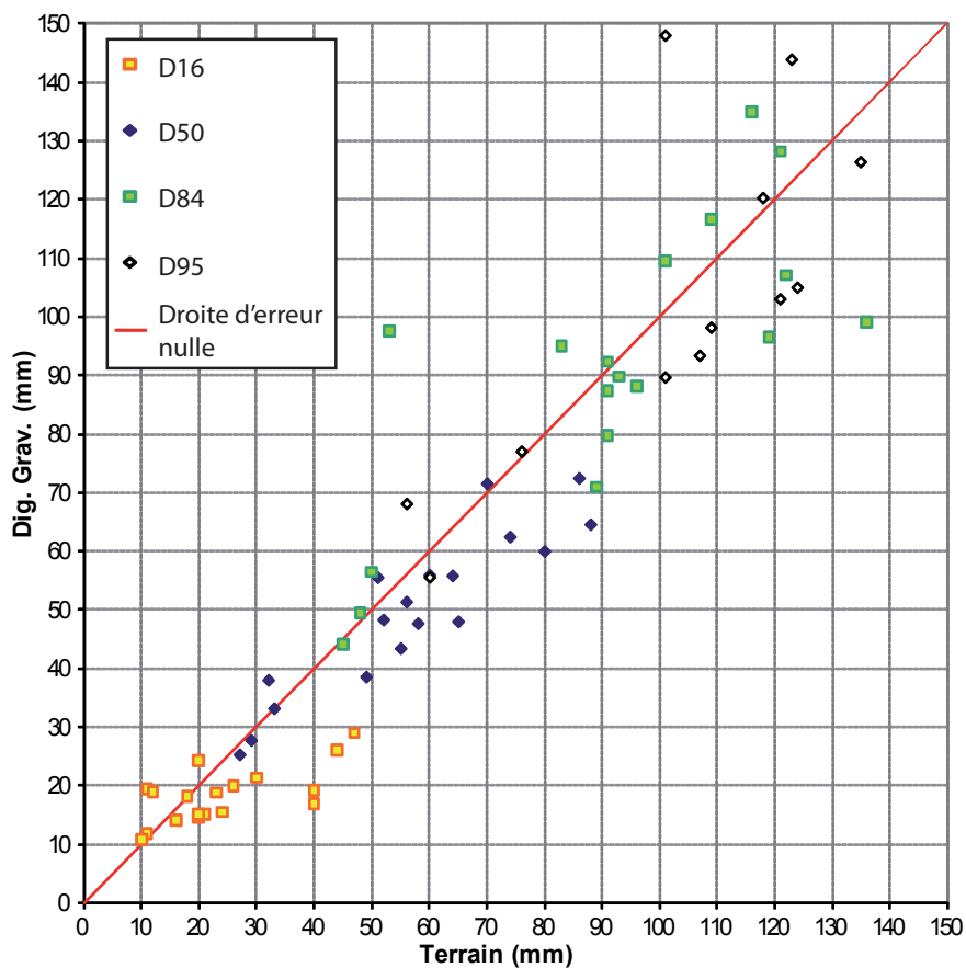
Figure M11 - Test d'une méthode de mesure automatisée de la granulométrie sur la rivière Allier
