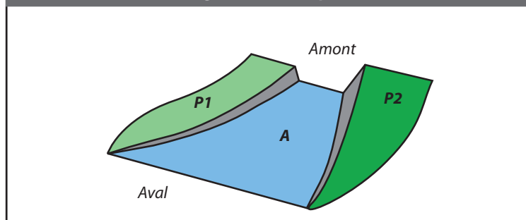
Figure M8 - Reconstruction des profils et de la géométrie des plans d'accumulation
