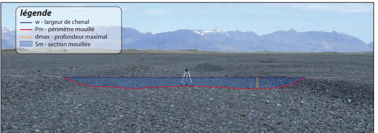
Figure M10 - Les paramètres de la géométrie de chenal mesurés
