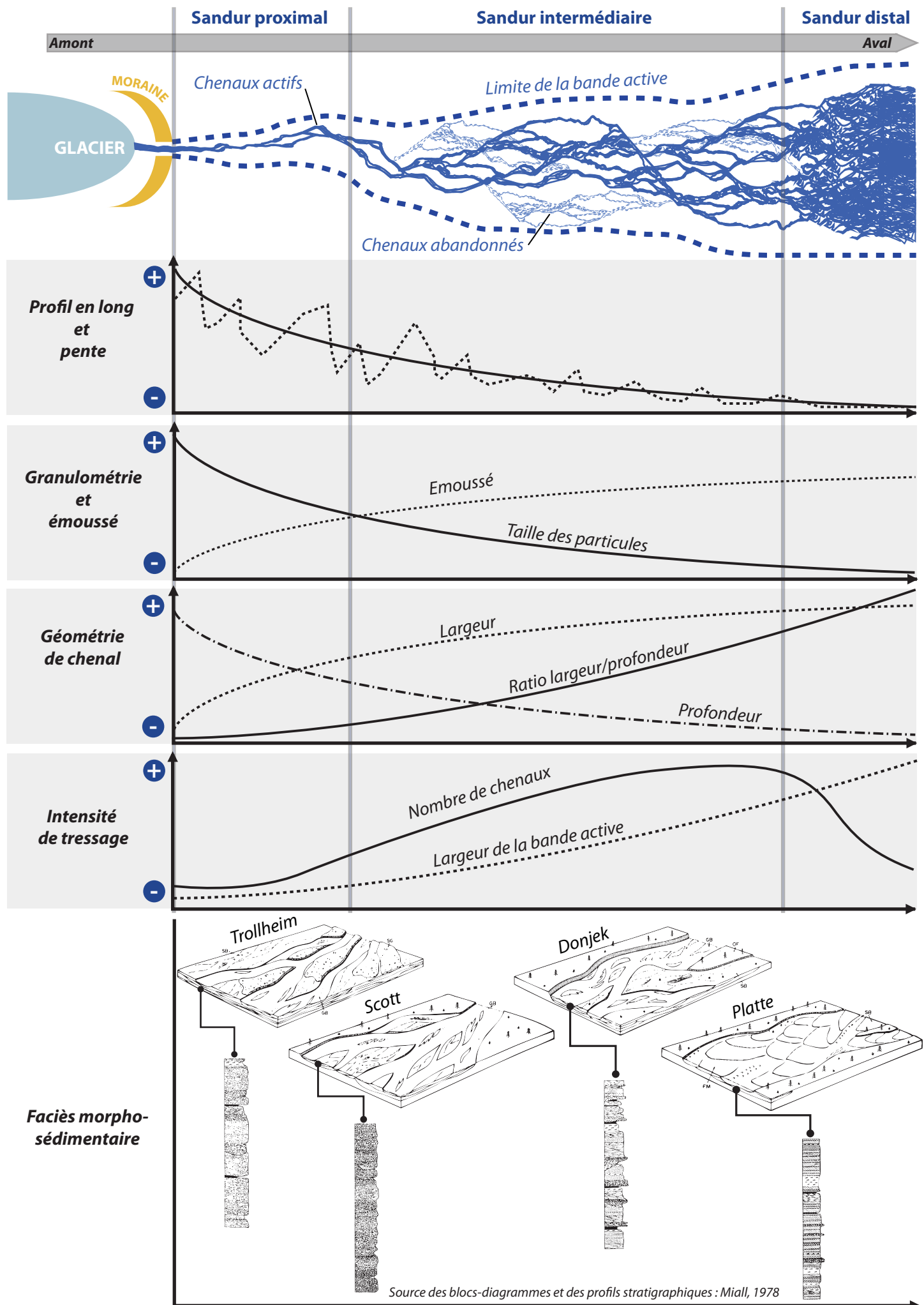
Figure B12 - Variation amont-aval des caractéristiques morphosédimentaires
