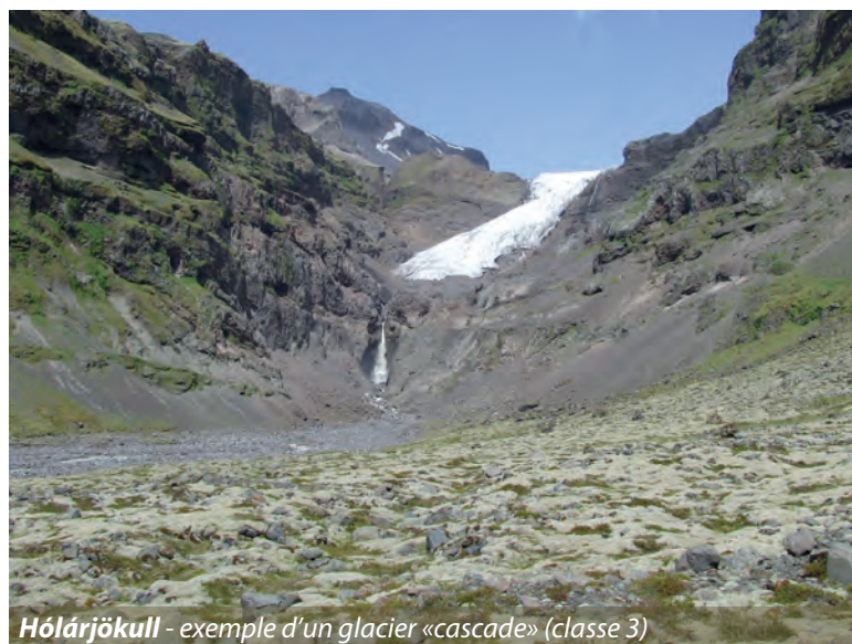
Figure R18 - Aperçu photographique des types de glacier
