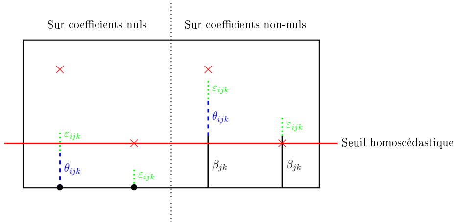
FIGURE 9.1 – Schéma simplifié comparant les seuillages homoscedastique et heteroscedastique dans les configurations A et B et en presence ou non d'effets aleatoires.
