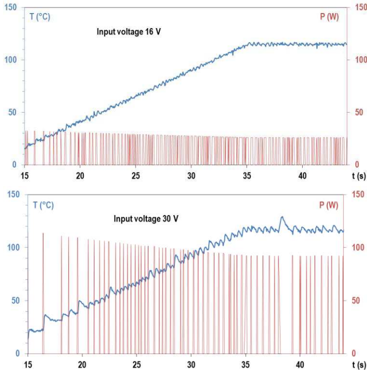
Fig. 118: illustration of the influence of input voltage choice for chip heating; T amb =30°C.
