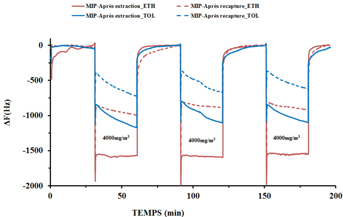
Fig. 4-16: Variations de fréquence d'un capteur avec une couche de MIP-DMSO (après extraction et recapture de la molécule empreinte) soumis à 4000 \text{ mg/m}^3 d'éthanol et de toluène (répétabilité)
