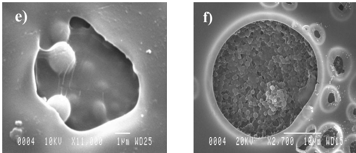
Fig. 3-16: Clichés MEB de couches MIP-DMSO après extraction de la molécule empreinte, en fonction de l'épaisseur : a, c et e) 200 nm, b, d et f) 1,4 μm
