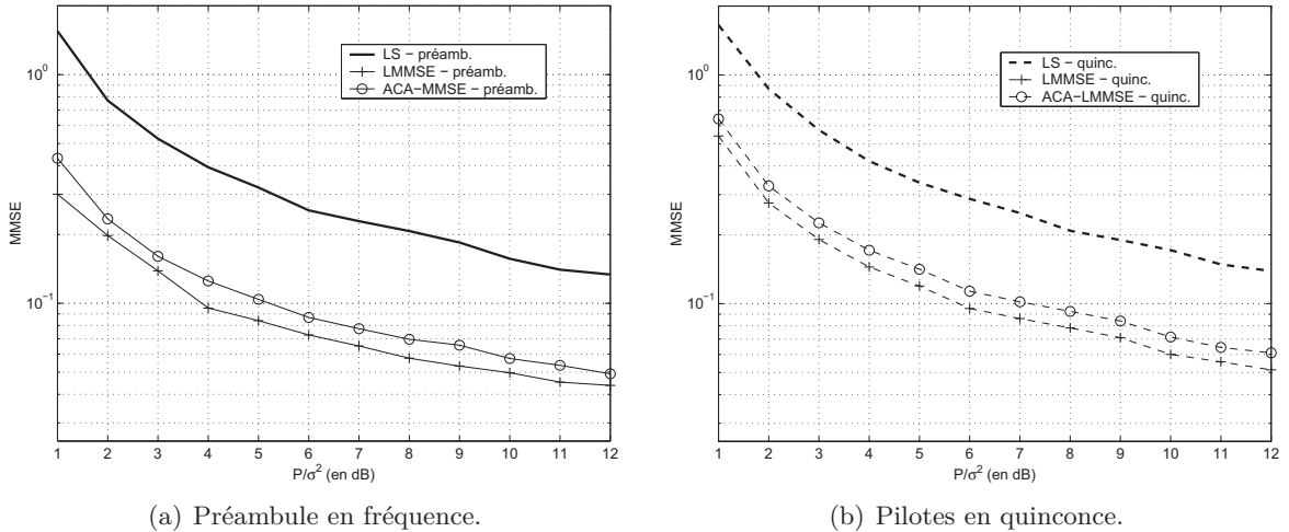
FIGURE r.6 – Erreur quadratique moyenne de ACA-LMMSE comparée à LS et LMMSE.
