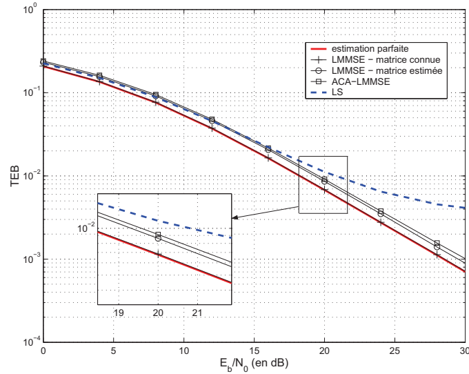
FIGURE r.7 – TEB de ACA-LMMSE comparé à LMMSE et LS en fonction de E_b/N_0 .
