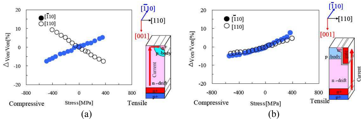
Figure 2.8 Variation de Von suivant le sens de la contrainte appliquée : (a) Structure Planaire, (b) structure en Tranchée [Tana06]
