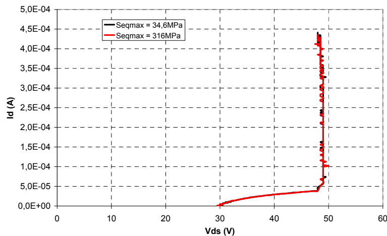
Figure 5.15 I_d(V_{ds}) suivant la contrainte mécanique appliquée à V_{gs} = 0 V « MOSFET »
