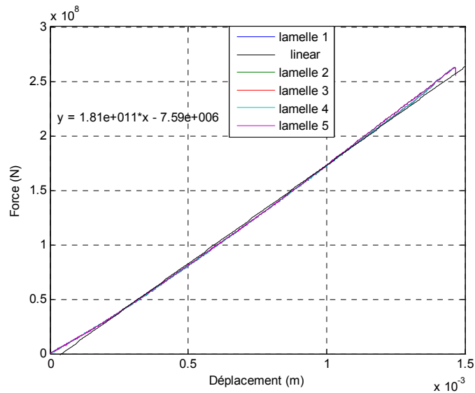
Figure 4.21 Courbes de variation de \bar{F} en fonction du déplacement « MOSFET »
