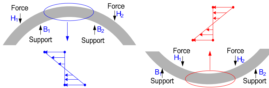
Figure 4.18 Configurations de mesure envisagées
