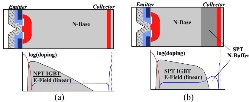
Figure 1.13 Structure à grille planaire : (a) NPT ;(b) SPT [ABB]
