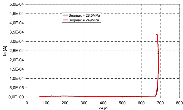
Figure 5.12 I_a(V_{ak}) suivant la contrainte mécanique appliquée à V_{gk} = 0 V « IGBT »
