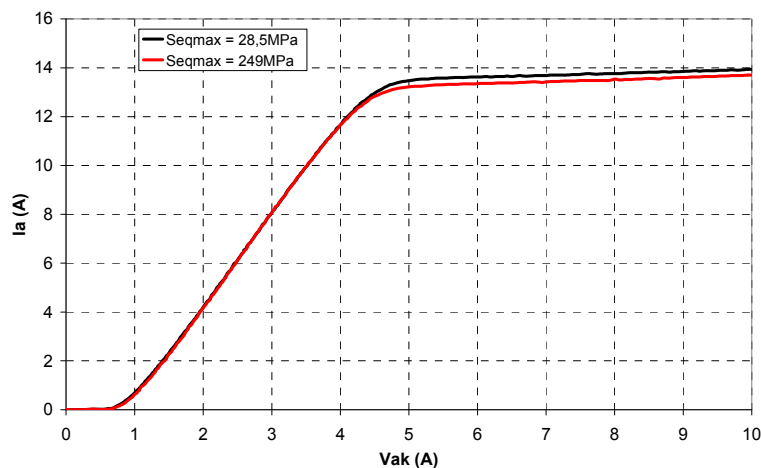
Figure 5.10 I_a(V_{ak}) suivant la contrainte mécanique à V_{gk} = 9\text{V} et T = 300^\circ\text{K} « IGBT »
