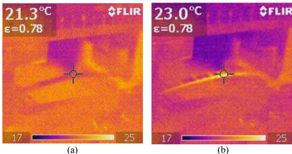
Figure 5.21 Distribution de la température sur la lamelle de transistors IGBT (a) Sans polarisation électrique (b) Polarisation électrique à 8Vet 3A
