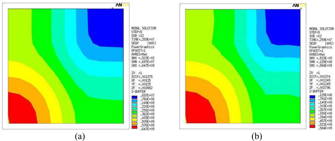
Figure 4.28 Distribution des contraintes de Von Mises en dessous de la puce en configuration partie haute en traction (a) IGBT (b) MOSFET
