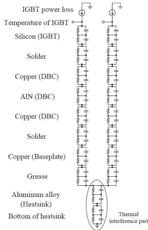
Figure 1.9 Modèle compacte thermique incluant deux IGBTs en parallèle [Taka04]
