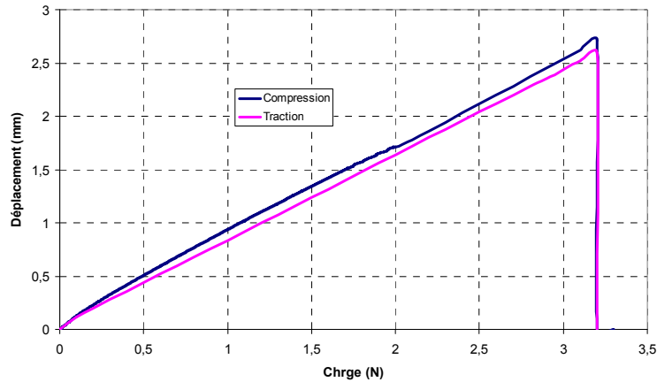
Figure 4.22 Courbes de variation du déplacement en fonction de la charge « MOSFET »
