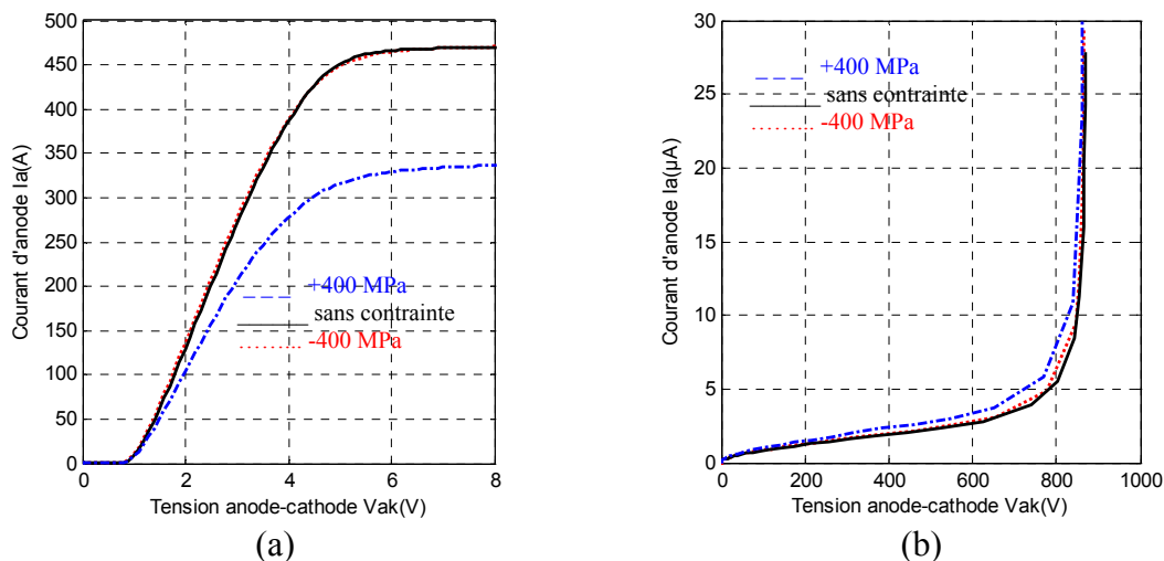
Figure 2.12 (a) Caractéristique de sortie, (b) Caractéristique de la tenue en tension, suivant la contrainte mécanique appliquée
