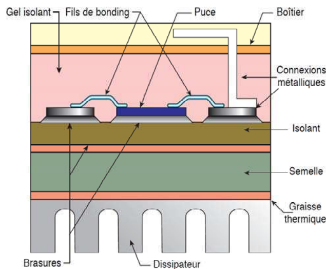
Figure 1.1 Assemblage classique de puissance monté sur son radiateur [Elec06]
