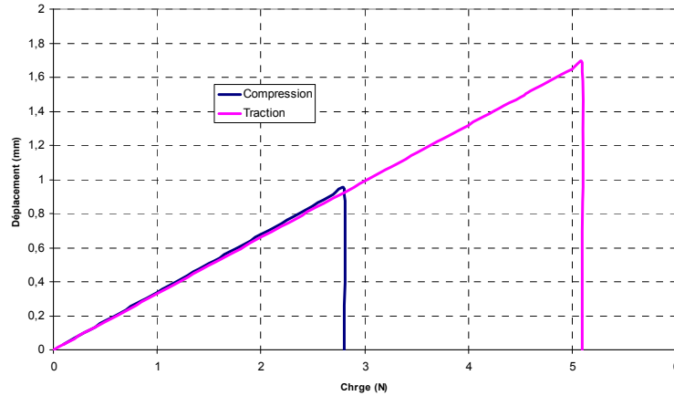
Figure 4.23 Courbes de variation du déplacement en fonction de la charge « IGBT »
