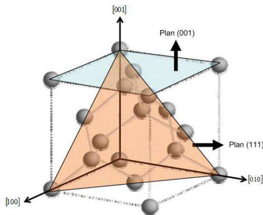
Figure 4.2 Structure cubique face centrées du silicium [Cho09]
