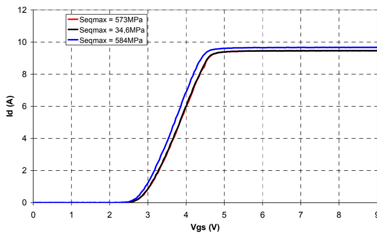
Figure 5.39 I_d(V_{gs}) suivant la contrainte mécanique appliquée à V_{ds} = 4 \text{ V} « MOSFET »
