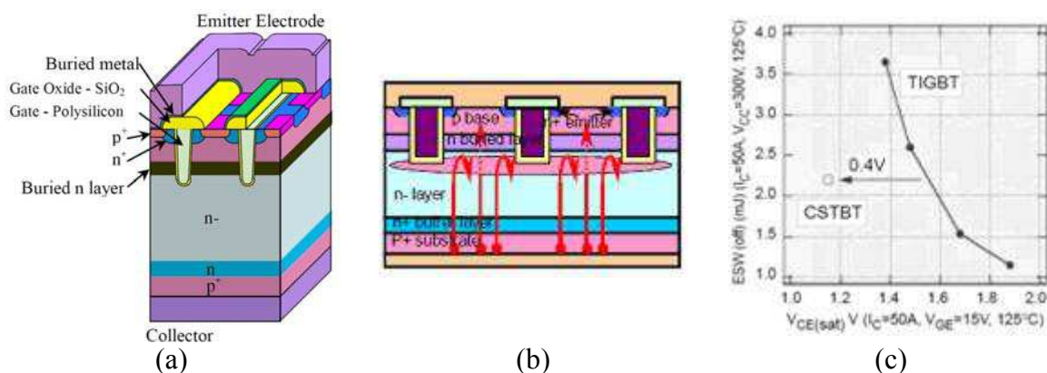
Figure 1.15 (a) Vue 3D de la structure PT-CSTBT ; (b) Déplacement des trous dans la structure CSTBT ; (c) Performances [Mits]
