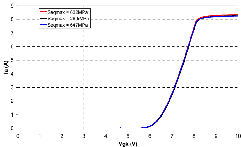
Figure 5.36 I_a(V_{gk}) suivant la contrainte mécanique appliquée à V_{ak} = 4 \text{ V} « IGBT »
