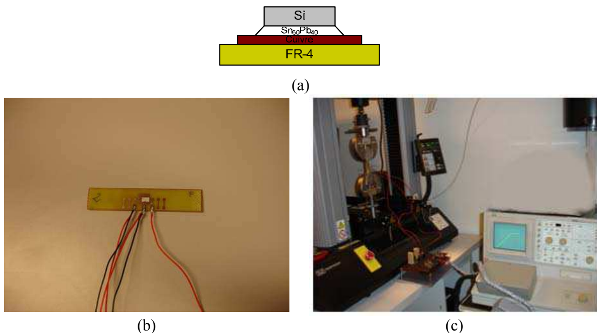
Figure 5.9 (a) Coupe 2D de l'assemblage, (b) Véhicule de test, (c) Banc de mesure expérimental
