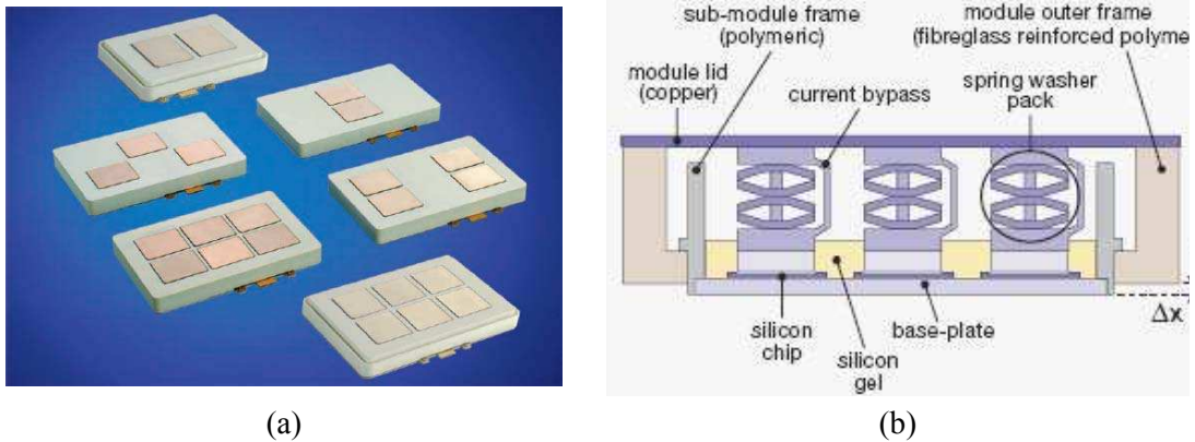
Figure 1.24 (a) Modules StakPak à boîtier press-pack ; (b) Coupe 2D de l'assemblage StakPak [ABB]
