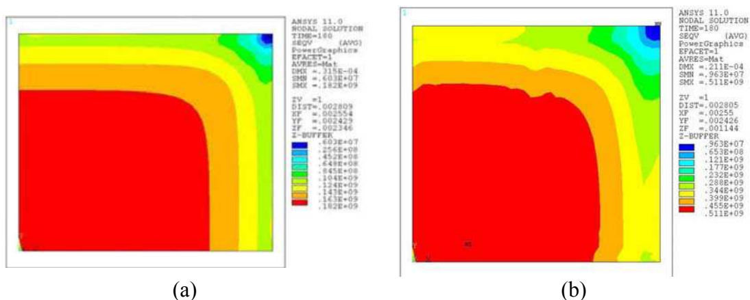
Figure 1.28 Distribution des contraintes de Von Mises : (a) DBC ; (b) l'assemblage à double face d'évacuation thermique [EPO06]
