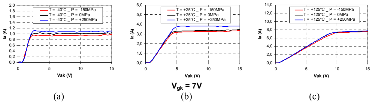
Figure 5.23 I_a(V_{ak}) suivant la contrainte mécanique à V_{gk} = 7\text{ V} (a) T = -40^\circ\text{C} , (b) T = +25^\circ\text{C} , (c) T = +125^\circ\text{C} « IGBT »
