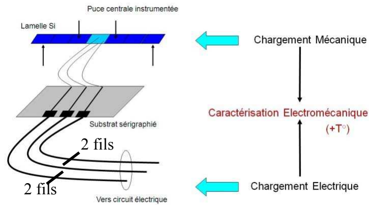
Figure 5.16 Instrumentation de la lamelle pour la caractérisation électromécanique
