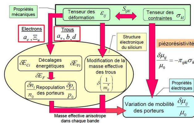
Figure 2.9 Représentation schématique du calcul électromécanique [Guil04]
