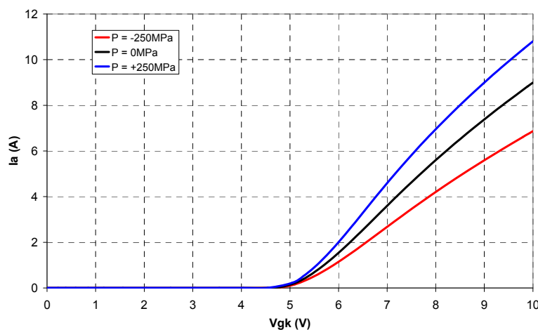
Figure 5.6 I_a(V_{gk}) suivant la contrainte mécanique uniaxiale appliquée à V_{ak} = 4V
