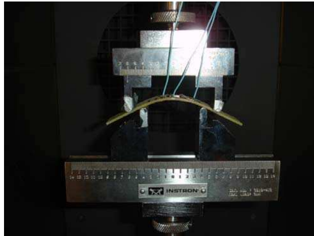
Figure 4.26 Test de flexion quatre points
