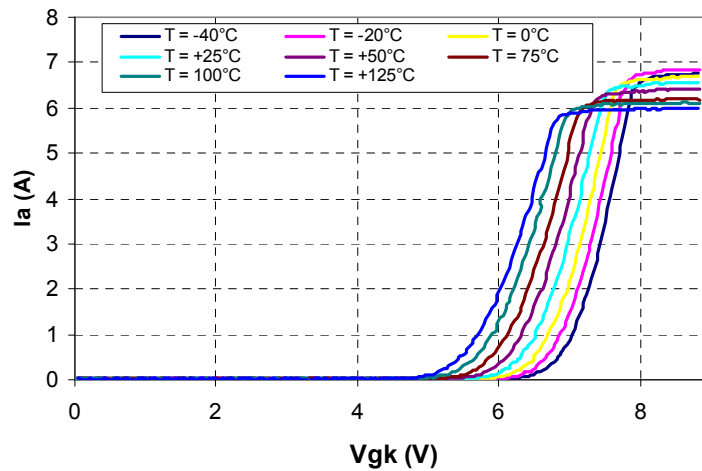
Figure 5.24 I_a(V_{gk}) suivant la température ambiante à V_{ak} = 4\text{ V} « IGBT »
