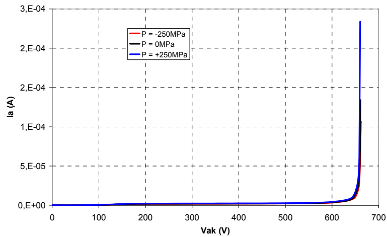
Figure 5.7 I_a(V_{ak}) suivant la contrainte mécanique uniaxiale appliquée à V_{gk} = 0V
