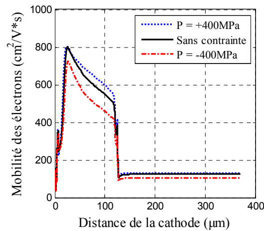
Figure 3.15 Distribution 1D de la mobilité des électrons le long de la ligne de coupe a-a' suivant la contrainte mécanique appliquée
