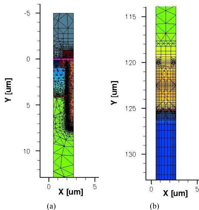
Figure 3.3 Modèle de simulation par éléments finis (a) partie haute, (b) partie basse du composant
