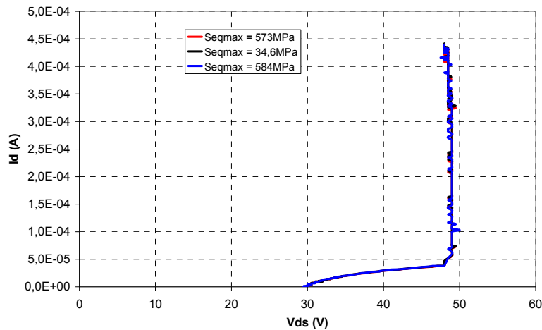
Figure 5.40 I_d(V_{ds}) suivant la contrainte mécanique appliquée à V_{gs} = 0V « MOSFET »
