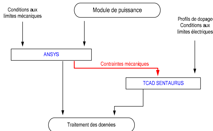
Figure 1.5 Liaison entre ANSYS et TCAD SENTAURUS
