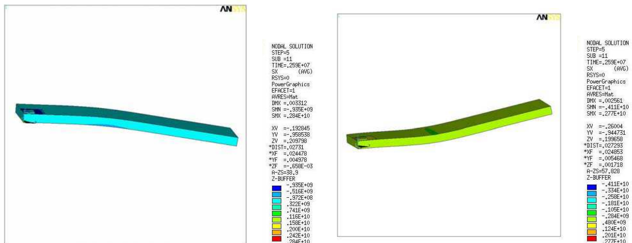
(a) Configuration partie haute en traction (b) Configuration partie haute en compression Figure 4.27 Distribution des contraintes uniaxiales S_{xx} sur l'assemblage
