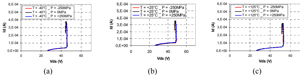
Figure 5.33 I_d(V_{ds}) suivant la contrainte mécanique à V_{gs} = 0V (a) T = -40^\circ C , (b) T = +25^\circ C , (c) T = +125^\circ C « MOSFET »
