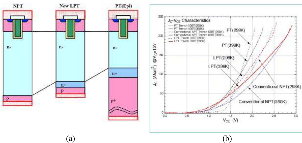
Figure 1.16 (a) Coupe 2D des structures NPT, New LPT et PT(Epi) ; (b) Caractéristique de sortie J_C - V_{CE} à 298°K et 398°K pour les structures NPT, PT et LPT [Mits]
