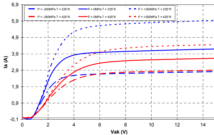
Figure 5.5 I_a(V_{ak}) suivant la contrainte mécanique uniaxiale appliquée pour T = 235^\circ\text{K} et T = 425^\circ\text{K}
