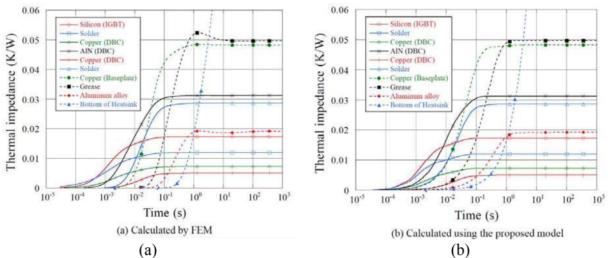
Figure 1.8 L'impédance thermique de chaque couche de l'assemblage : (a) Calcul éléments finis 'FEM' ; (b) Calcul avec le modèle RC [Taka04]
