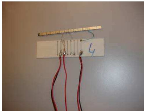
Figure 5.19 Lamelles de transistors MOSFET câblée à travers un substrat sérigraphié
