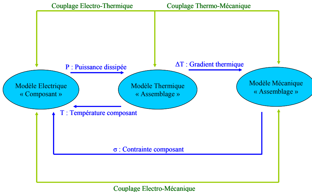
Figure 1.4 Diagramme de la modélisation électro-thermo-mécanique
