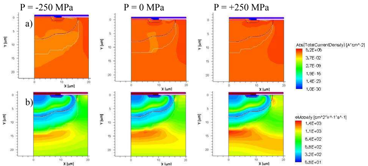
Figure 5.8 Distribution 2D suivant la contrainte mécanique appliquée (a) La densité du courant dans le canal du MOSFET, (b) La mobilité des électrons
