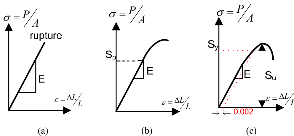
Figure 4.1 Diagrammes contrainte-déformation suivant le type de matériau (a) Fragile, (b) Semi-ductile, (c) Ductile
