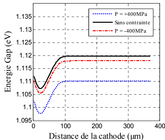
Figure 3.9 Distribution 1D de l'énergie Gap à t_1 = 12 \mu\text{s} le long de la ligne de coupe a-a' suivant la contrainte mécanique appliquée'
