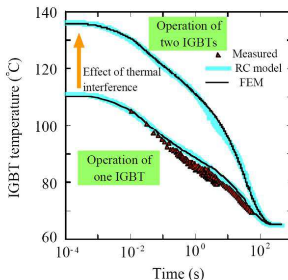
Figure 1.10 Comparaison des résultats de mesure, de simulation par FEM et du modèle compacte RC pour une puissance dissipée de 93,7 W [Taka04]
