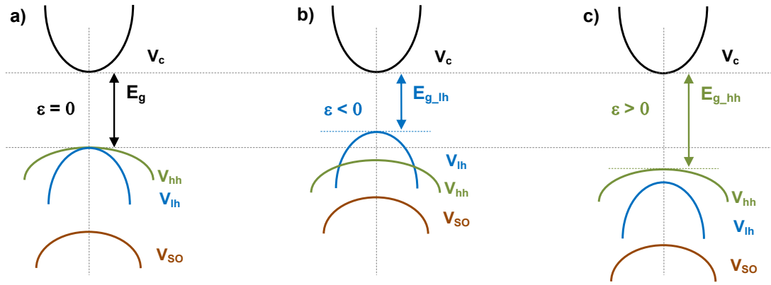
Figure 2.10 Représentation schématique de la structure de bande d'un matériau a) non contraint, soumis à une contrainte bi-axiale b) en traction, et c) en compression
