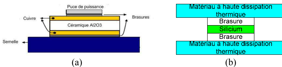
Figure 1.26 (a) Coupe2D de l'assemblage sur substrat SMI ; (b) Coupe2D de l'assemblage à double face d'évacuation thermique
