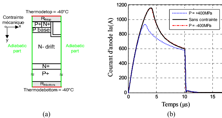
Figure 3.12 (a) Application de la température sur le modèle, (b) Résultat de simulation du mode court-circuit
