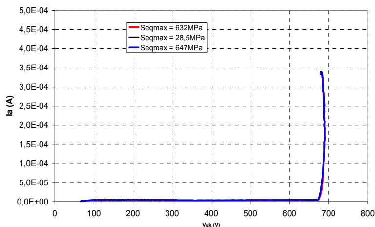
Figure 5.37 I_a(V_{ak}) suivant la contrainte mécanique appliquée à V_{gk} = 0V « IGBT »
