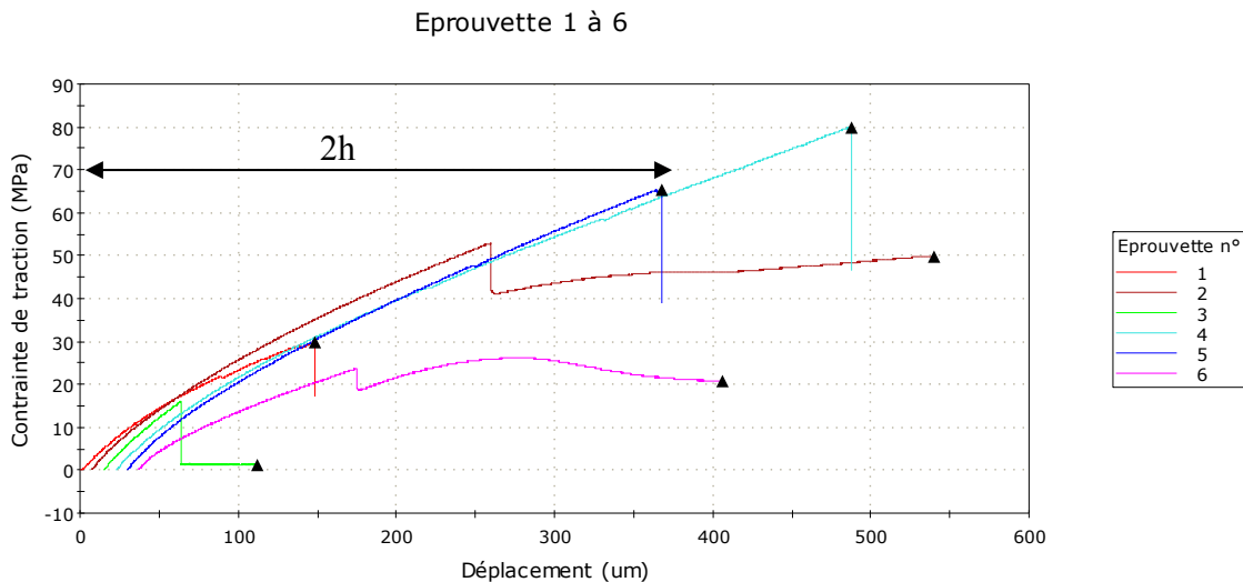
Figure 4.8 Courbes contrainte-déplacement dans la direction [110]
