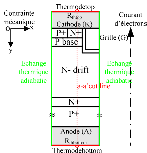
Figure 3.2 Modèle 2D IGBT asymétrique à grille en tranchée
