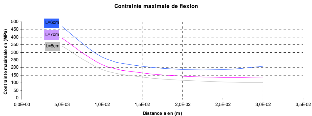
Figure 4.19 Contraintes maximales suivant les distance a et L
