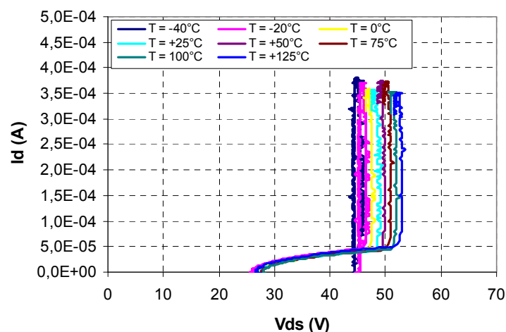
Figure 5.32 I_d(V_{ds}) suivant la température ambiante à : à V_{gs} = 0 V « MOSFET »
