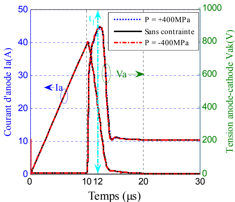
Figure 3.8 Courant d'anode (à gauche) et tension anode-cathode (à droite) suivant la contrainte mécanique appliquée en mode UIS
