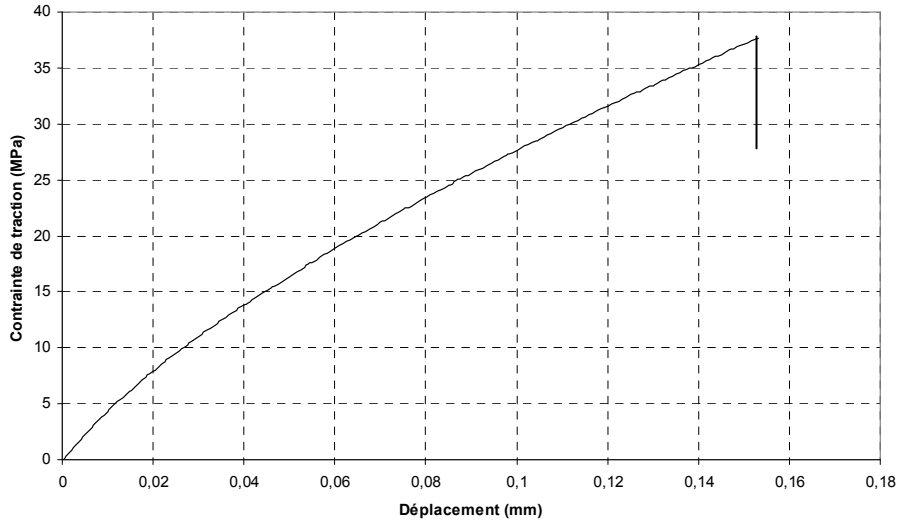
Figure 4.10 Courbe contrainte-déplacement « lamelle IGBT »
