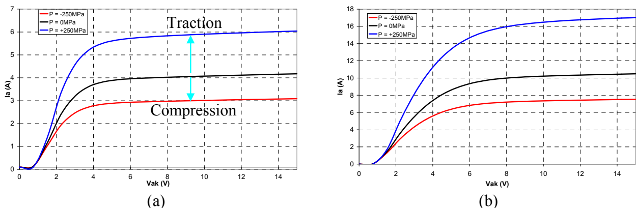
Figure 5.4 I_a(V_{ak}) dans le cas de l'application d'une contrainte mécanique uniaxiale (a) V_{gk} = 7\text{V} , (b) V_{gk} = 9\text{V}
