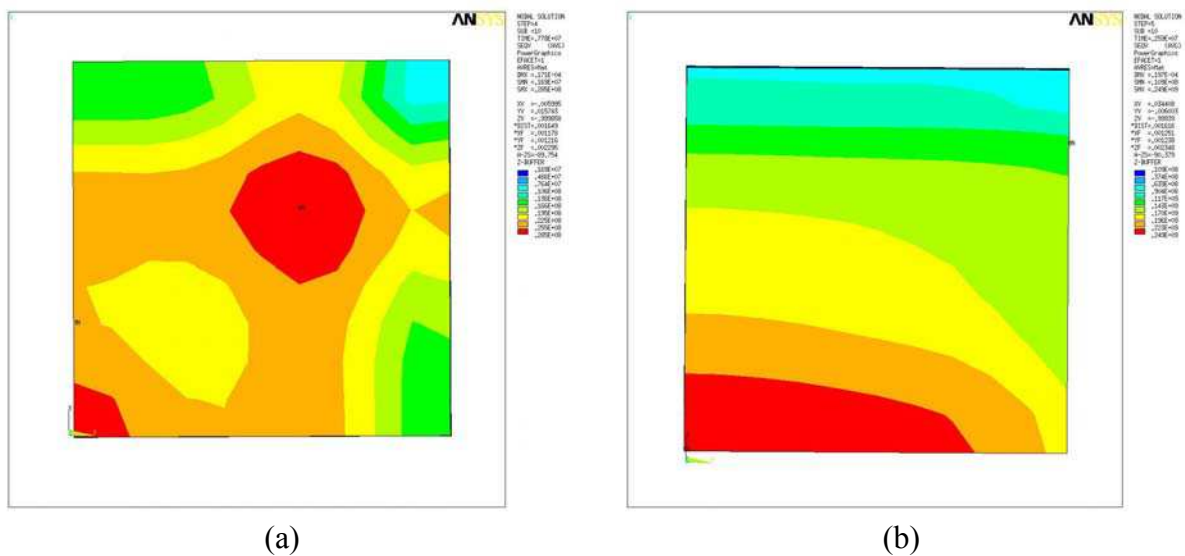
Figure 4.15 Distribution des contraintes de Von Mises en dessous de la puce (a) Avant chargement de traction (b) Après chargement de traction
