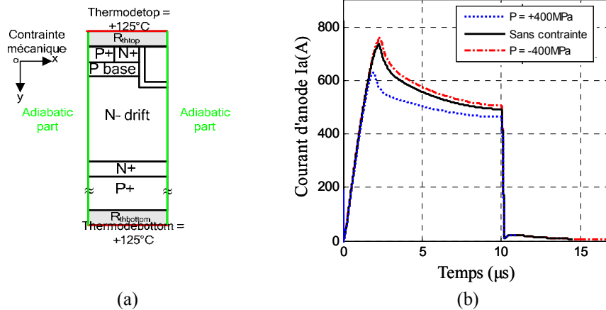
Figure 3.13 (a) Application de la température sur le modèle, (b) Résultat de simulation du mode court-circuit
