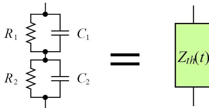
Figure 1.7 Cellule de base du modèle compact [Taka04]
