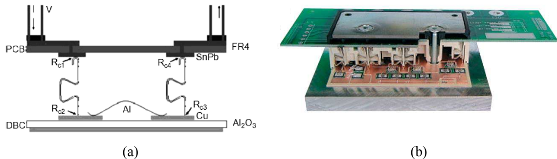
Figure 1.25 (a) Coupe 2D de l'assemblage avec contact ressort pressé ; (b) Vue d'un module MiniSKIIP avec ses contacts ressorts [Semi]
