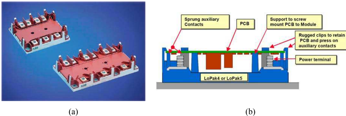
Figure 1.23 (a) Modules LoPak ; (b) Coupe 2D de l'assemblage du PCB sur les modules LoPak [ABB]
