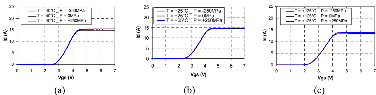
Figure 5.31 I_d(V_{gs}) suivant la contrainte mécanique à V_{ds} = 4V (a) T = -40^\circ C , (b) T = +25^\circ C , (c) T = +125^\circ C « MOSFET »
