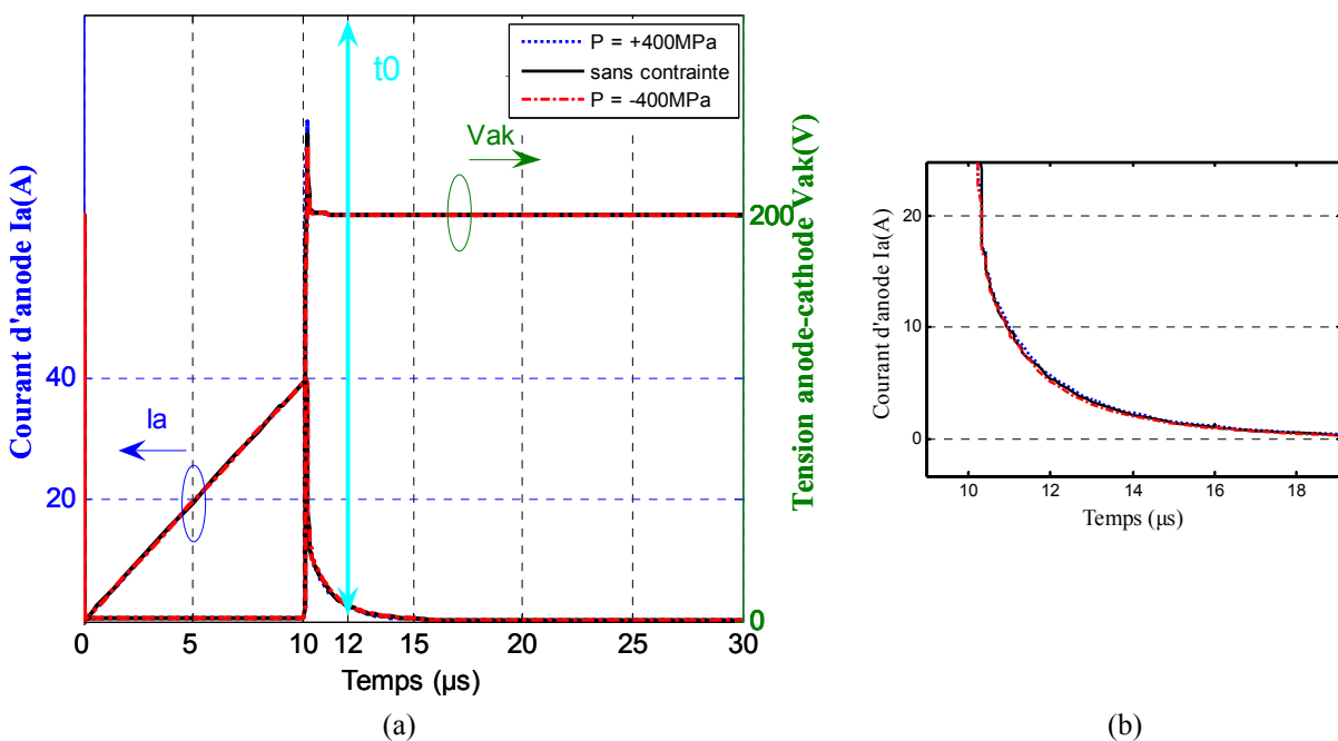
Figure 3.5 (a) Courant d'anode (à gauche) et tension anode-cathode (à droite) suivant la contrainte mécanique appliquée en mode CIS, (b) Zoom sur la queue de courant
