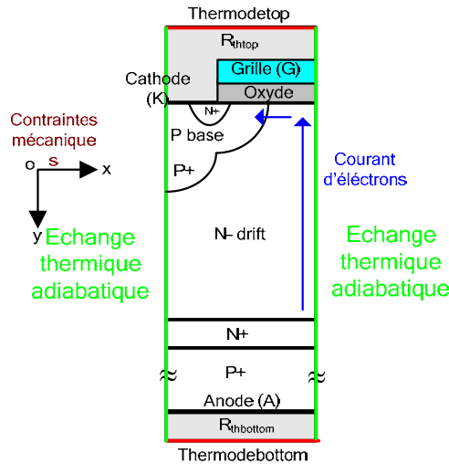
Figure 5.2 La structure de l'IGBT simulé
