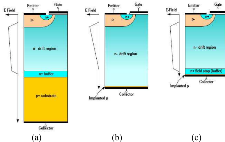
Figure 1.11 Structures de base avec grille planaire [Micr] : (a) PT ; (b) NPT ; (c) FS
