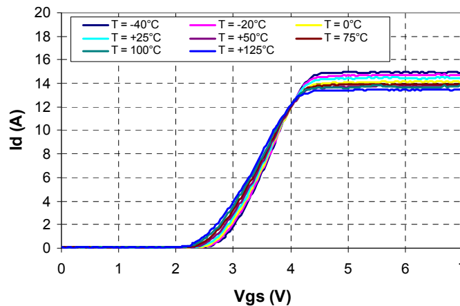
Figure 5.30 I_d(V_{gs}) suivant la température ambiante à V_{ds} = 4 \text{ V} « MOSFET »
