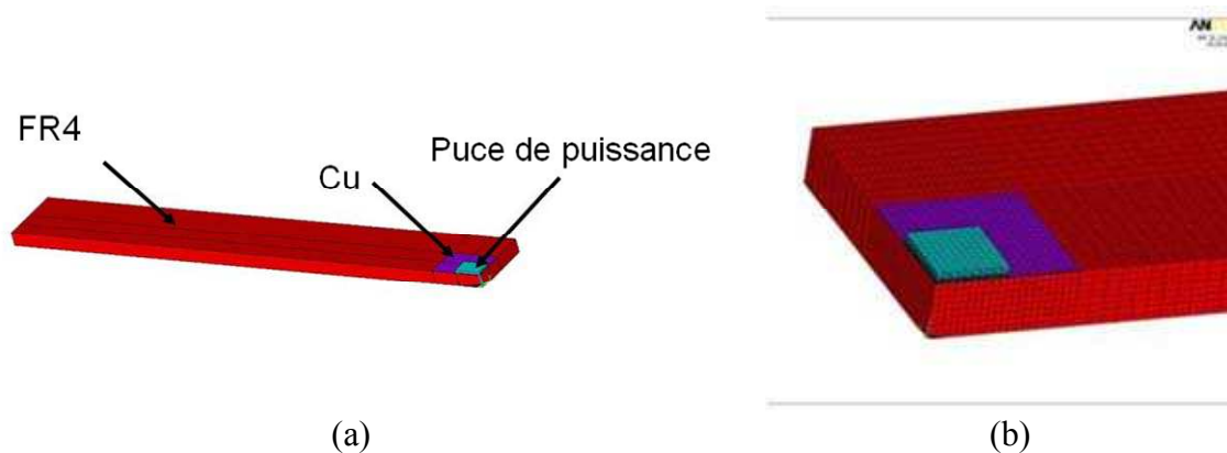
Figure 4.14 (a) Modèle simulé avec ANSYS, (b) Zoom sur la partie active
