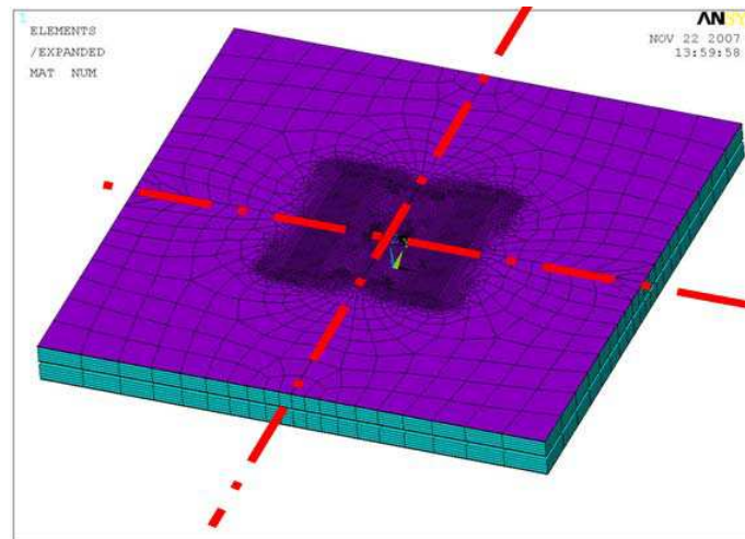
Figure 1.27 Modélisation 3D de ¼ de l'assemblage de puissance
