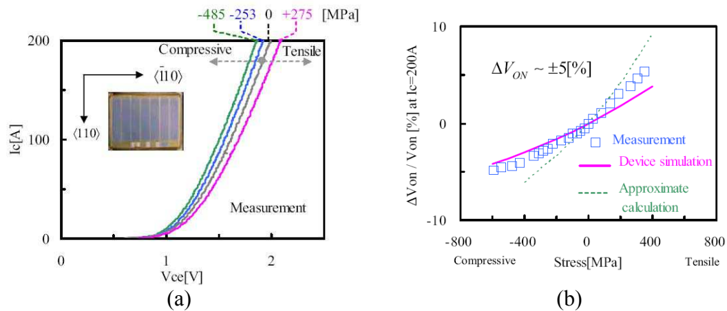
Figure 2.6 (a) Caractéristiques de sortie I_c = f(V_{ce}) , (b) Variation du V_{on} en fonction de la contrainte [Usui05]
