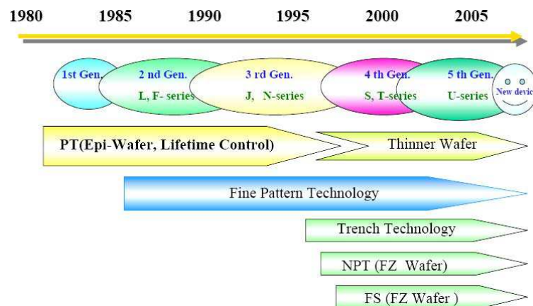
Figure 1.12 Développement de la technologie IGBT de FUJI ELECTRIC [Fuji]
