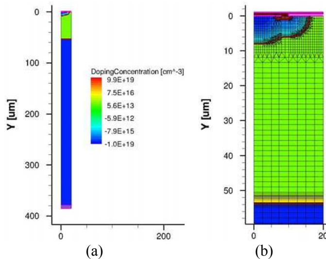
Figure 5.3 (a) Modèle simulé, (b) Maillage des différentes zones
