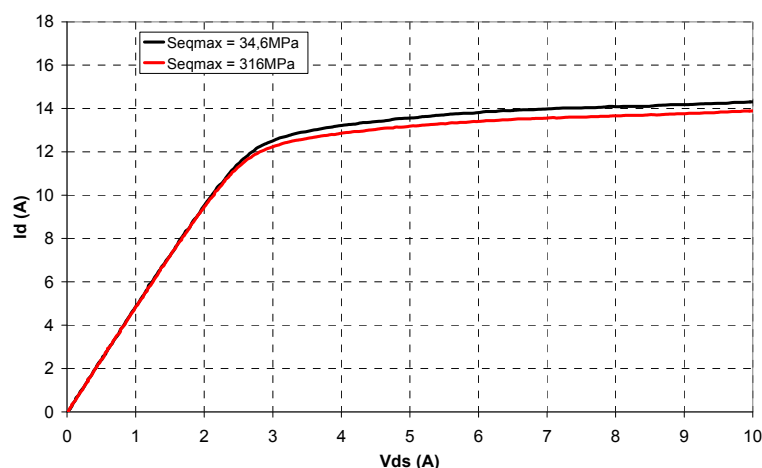
Figure 5.13 I_d(V_{ds}) suivant la contrainte mécanique à V_{gs} = 5\text{ V} et T = 300^\circ\text{K} « MOSFET »
