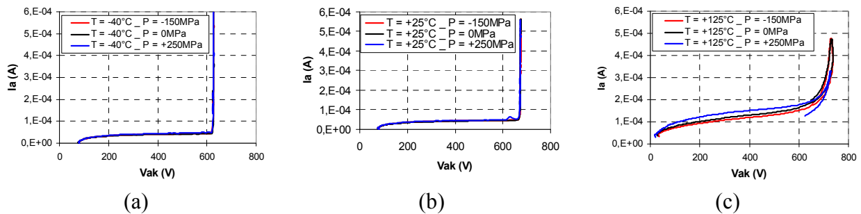
Figure 5.27 I_a(V_{ak}) suivant la contrainte mécanique à V_{gk} = 0 V (a) T = -40^\circ\text{C} , (b) T = +25^\circ\text{C} , (c) T = +125^\circ\text{C} « IGBT »
