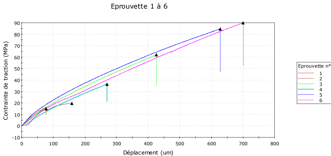
Figure 4.9 Courbes contrainte-déplacement dans la direction [1\bar{1}0]
