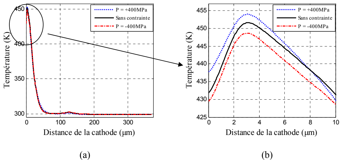
Figure 3.16 (a) Distribution 1D de la température le long de la ligne de coupe a-a' (b) Zoom à 10 \mu\text{m} de la partie haute du composant
