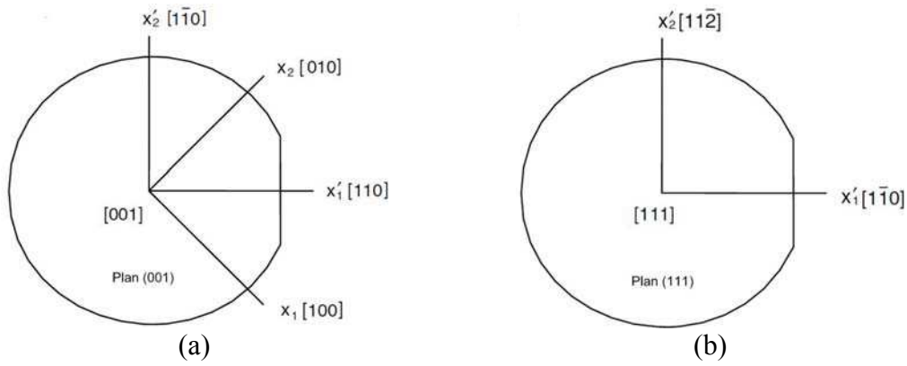
Figure 4.3 (a) Orientations dans le plan (001), (b) Orientations dans le plan (111)
