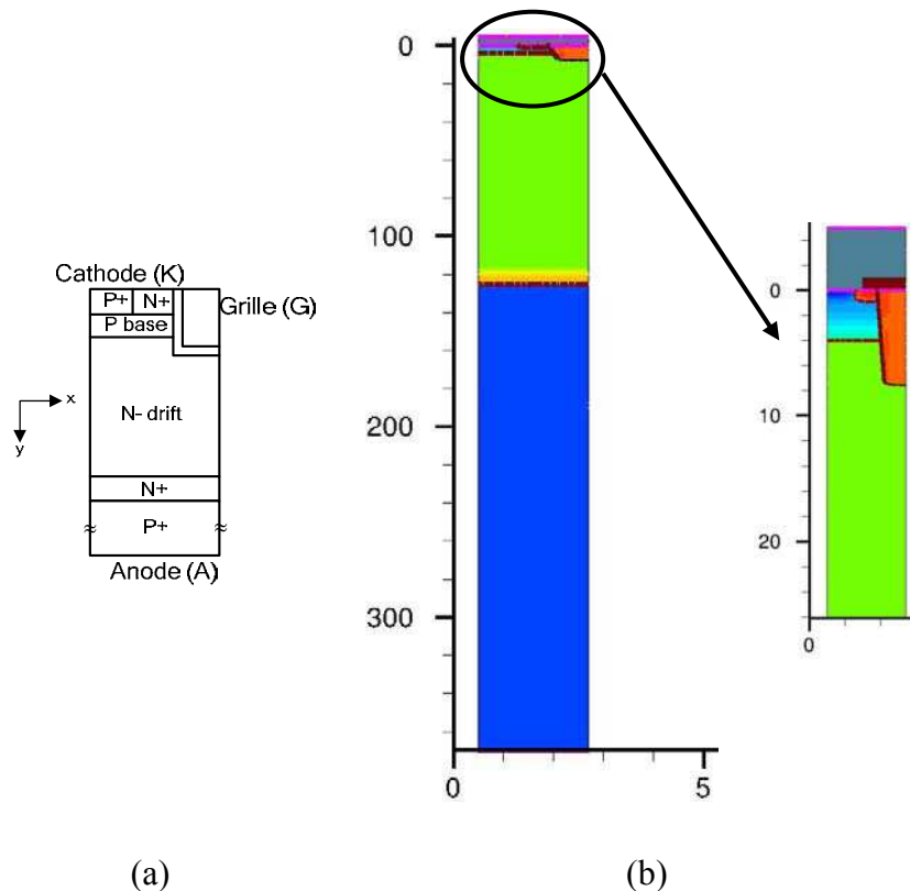
Figure 2.11 (a) Modèle de l'IGBT, (b) Le composant et le zoom sur la partie haute
