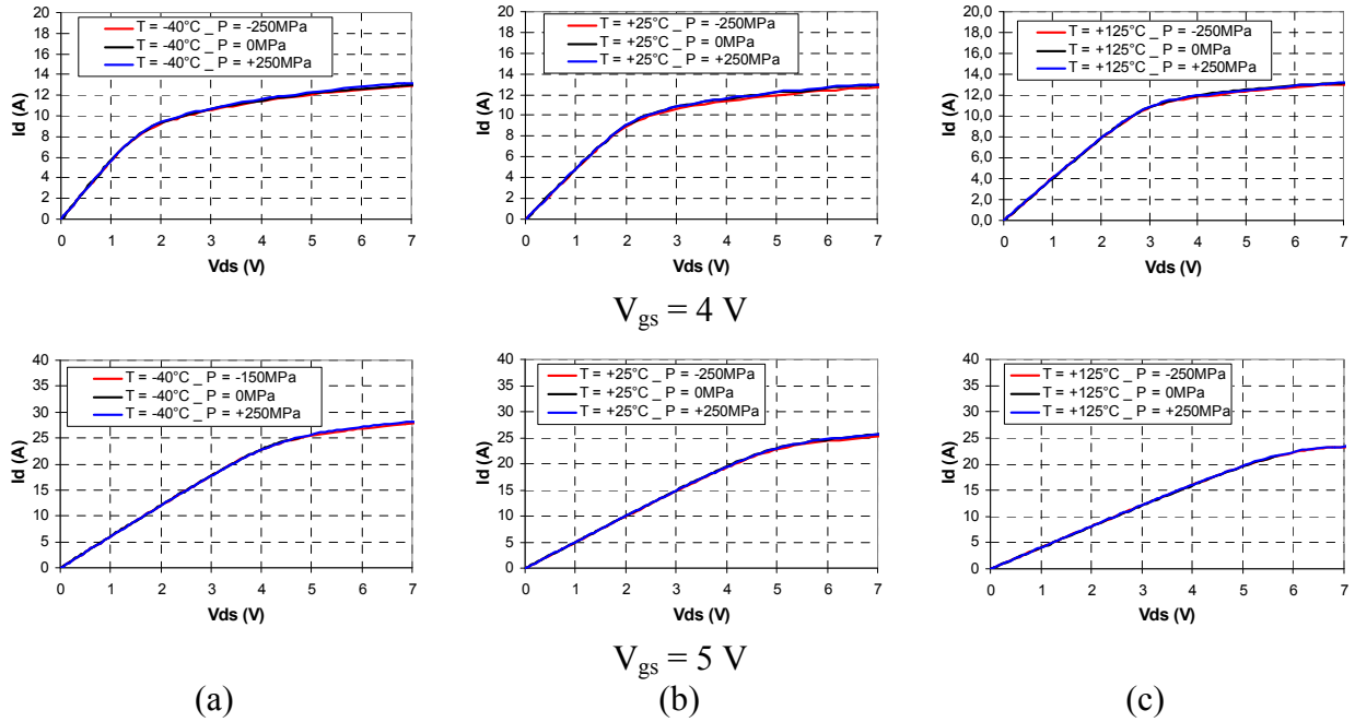
Figure 5.29 I_d(V_{ds}) suivant la contrainte mécanique à V_{gs} = 4 \text{ V} et à V_{gs} = 5 \text{ V} (a) T = -40^\circ\text{C} , (b) T = +25^\circ\text{C} , (c) T = +125^\circ\text{C} « MOSFET »
