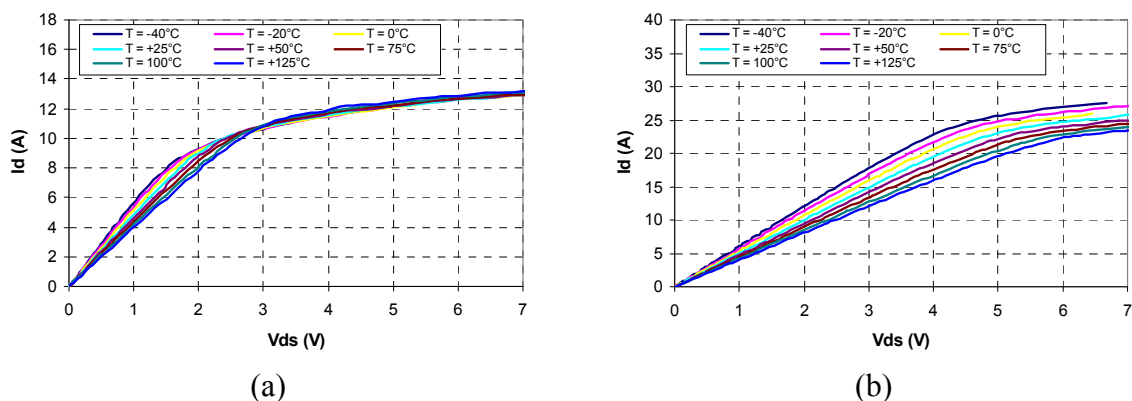
Figure 5.28 I_d(V_{ds}) suivant la température ambiante à : (a) V_{gs} = 4 V, (b) V_{gs} = 5 V « MOSFET »
