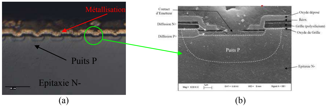
Figure 5.1 (a) Vues optiques en section de la structure du transistor, (b) Vue MEB détaillée
