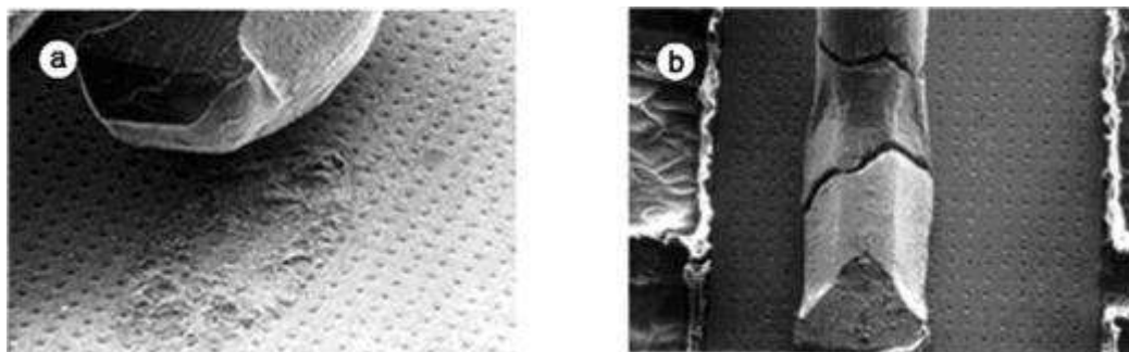
Figure 1.2 (a) Levée du fil de câblage, (b) fracture du pied du fil de câblage [Cia02]
