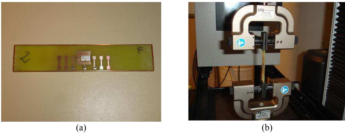
Figure 4.12 (a) Véhicule de test, (b) Test de traction uniaxiale
