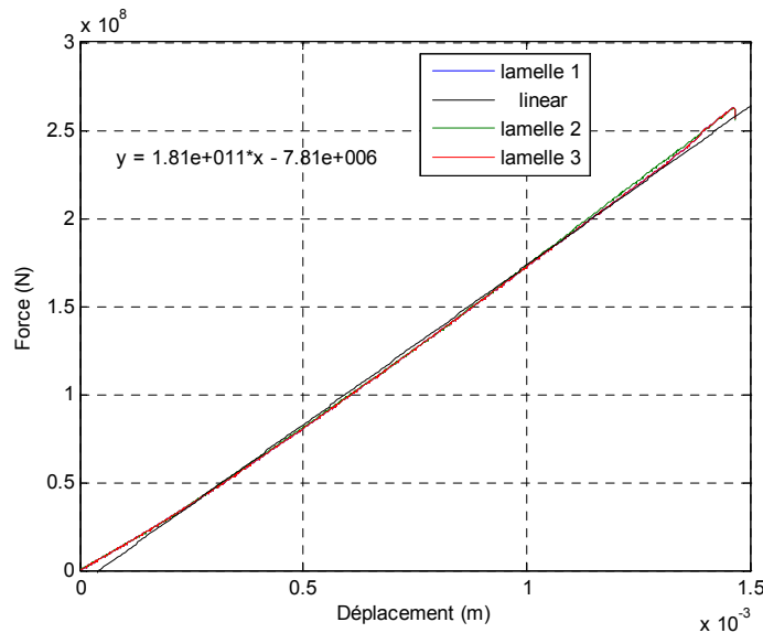
Figure 4.20 Courbes de variation de \bar{F} en fonction du déplacement « IGBT »
