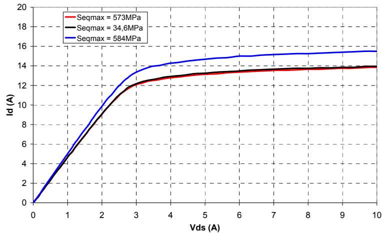
Figure 5.38 I_d(V_{ds}) suivant la contrainte mécanique pour V_{gs} = 5 \text{ V} et T = 300^\circ\text{K} « MOSFET »
