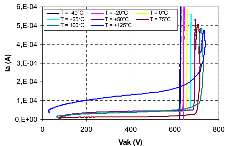
Figure 5.26 I_a(V_{ak}) suivant la température ambiante à : à V_{gk} = 0\text{ V} « IGBT »
