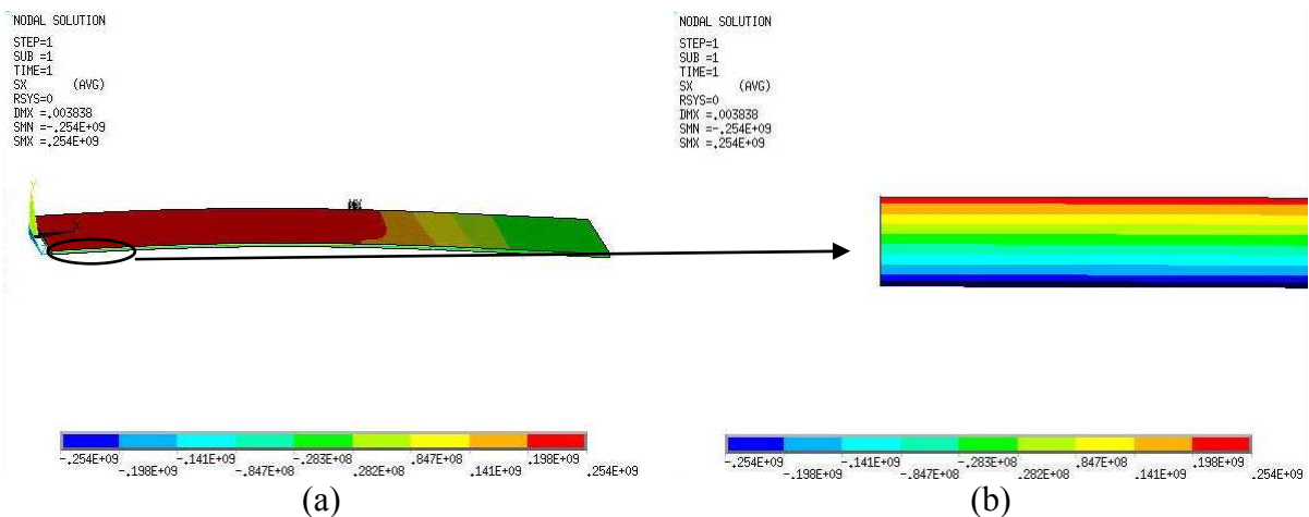
Figure 4.24 Distribution de la contrainte uniaxiale S_{xx} en traction, (a) Quart de la lamelle, (b) Zoom sur l'épaisseur
