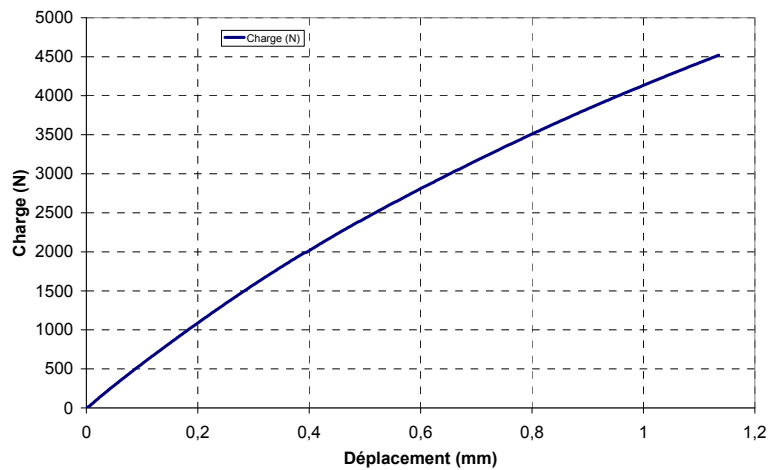
Figure 4.13 Courbe charge-déplacement du substrat FR-4
