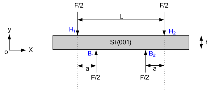
Figure 4.17 Application du chargement en mode de flexion 4 points
