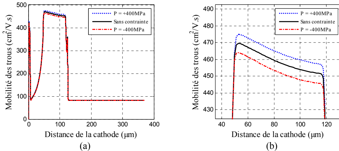
Figure 3.6 (a)Distribution 1D des trous à t_0 = 12\mu s le long de la ligne de coupe a-a' suivant la contrainte mécanique appliquée, (b) zoom entre 48 \mu m et 118 \mu m
