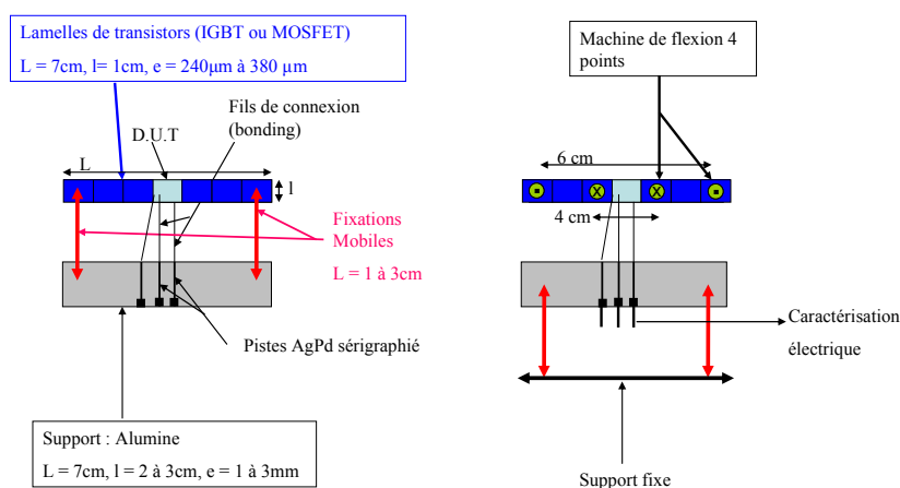
Figure 5.18 Proposition du véhicule de test
