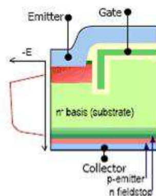
Figure 1.19 Coupe 2D de la structure IGBT 3 du fabricant INFINEON [Infi]
