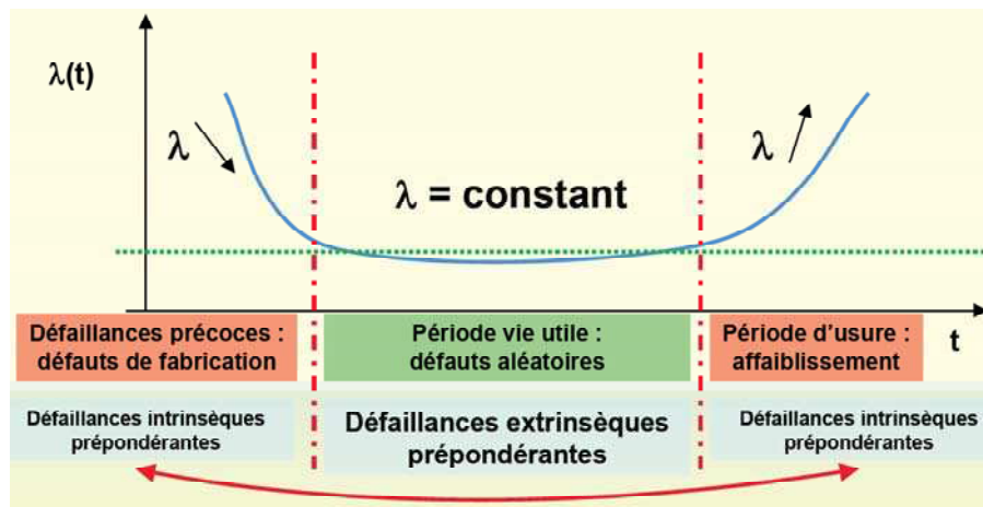
Figure 1.3 Allure de la fonction taux de défaillance \lambda en fonction du temps
