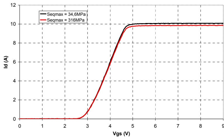
Figure 5.14 I_d(V_{gs}) suivant la contrainte mécanique appliquée à V_{ds} = 4 V « MOSFET »
