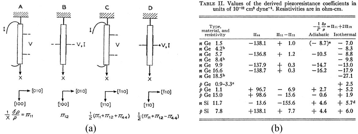
Figure 2.3 (a) Extraction expérimentale des coefficients piézorésistifs ; (b) Tableau de mesure des coefficients piézorésistifs [Smit54]
