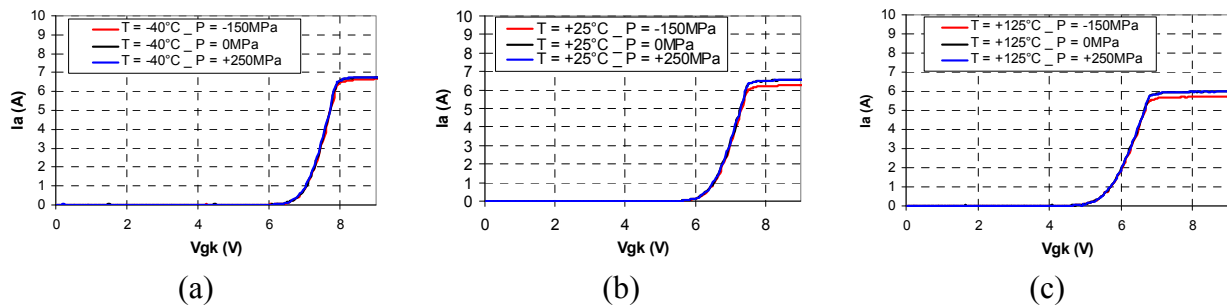
Figure 5.25 I_a(V_{ak}) suivant la contrainte mécanique à V_{ak} = 4\text{ V} (a) T = -40^{\circ}\text{C} , (b) T = +25^{\circ}\text{C} , (c) T = +125^{\circ}\text{C} « IGBT »
