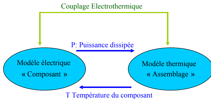
Figure 1.6 Diagramme de la modélisation électrothermique
