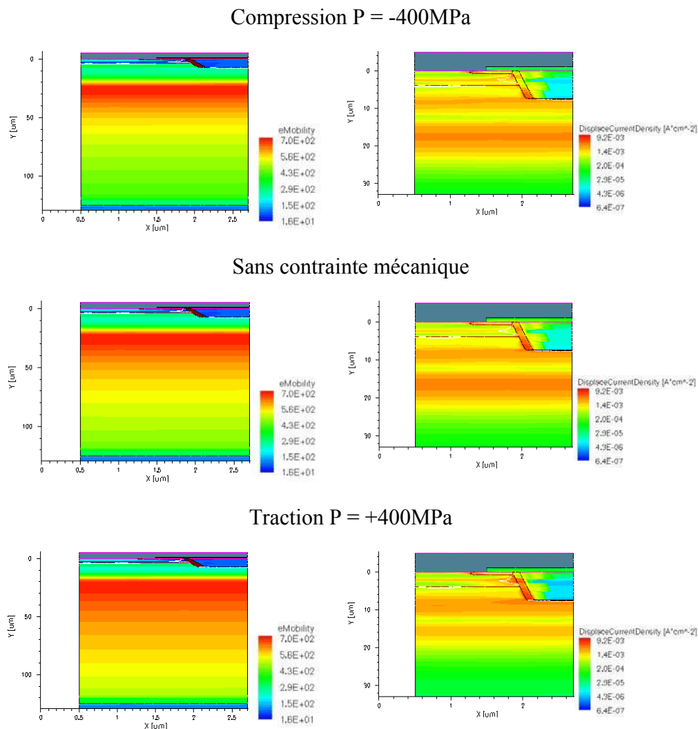
Figure 3.14 Distribution bidimensionnelle de la mobilité des électrons (à gauche) et de la densité du courant (à droite) durant le court-circuit au temps t_2 suivant la contrainte mécanique appliquée
