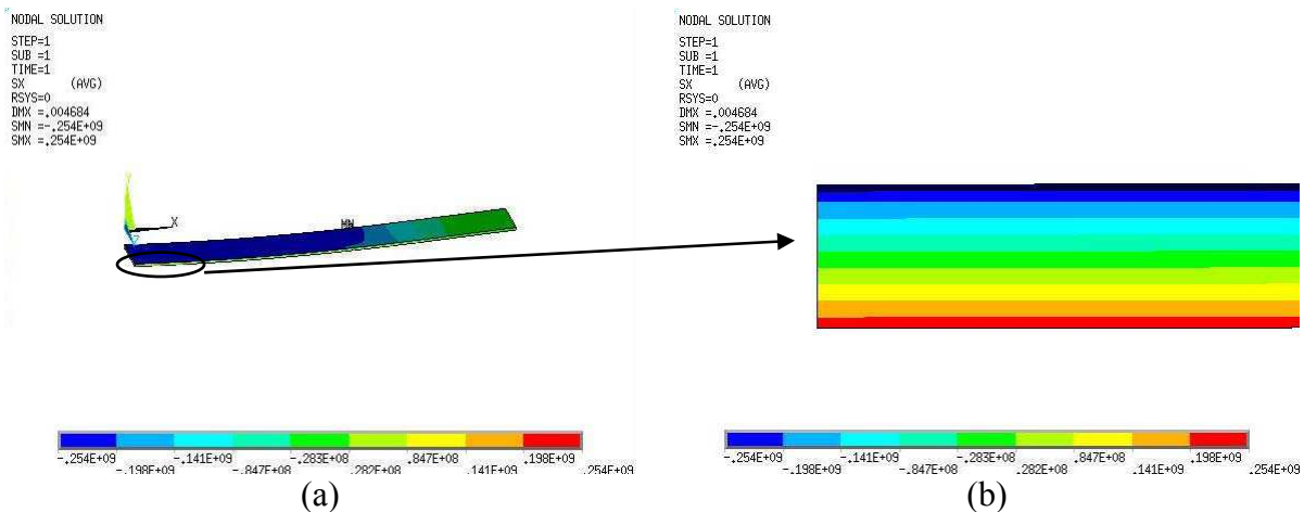
Figure 4.25 Distribution de la contrainte uniaxiale S_{xx} en compression, (a) Quart de la lamelle (b) Zoom sur l'épaisseur
