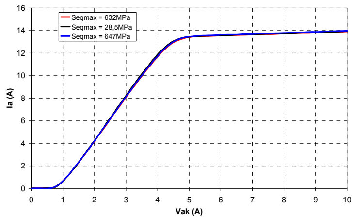
Figure 5.35 I_a(V_{ak}) suivant la contrainte mécanique pour V_{gk} = 9 \text{ V} et T = 300^\circ\text{K} « IGBT »
