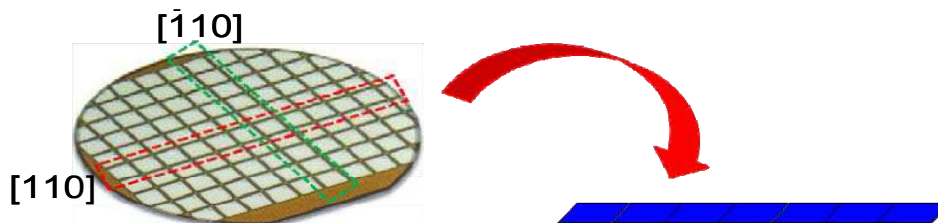
Figure 5.17 Lamelles IGBT obtenues à partir d'un wafer (découpes suivant les deux axes cristallographiques)
