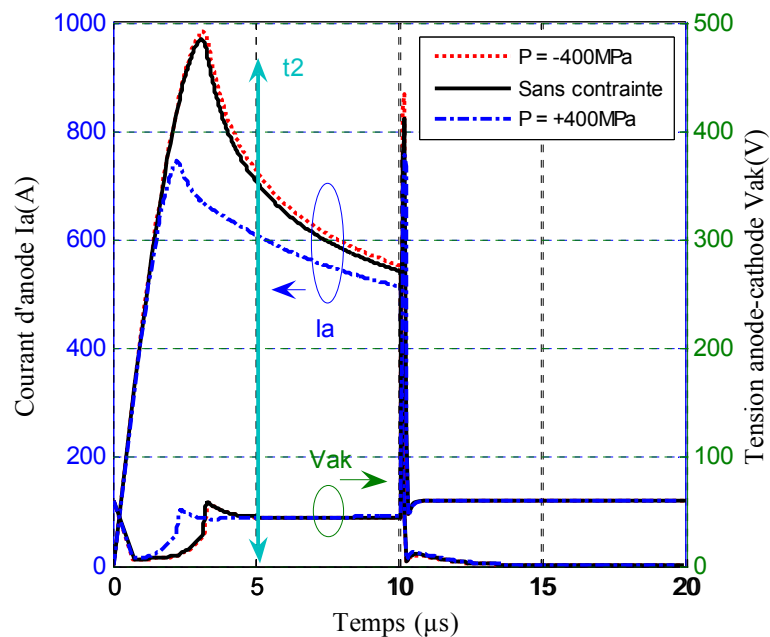
Figure 3.11 Courant d'anode (à gauche) et tension anode-cathode (à droite) suivant la contrainte mécanique appliquée
