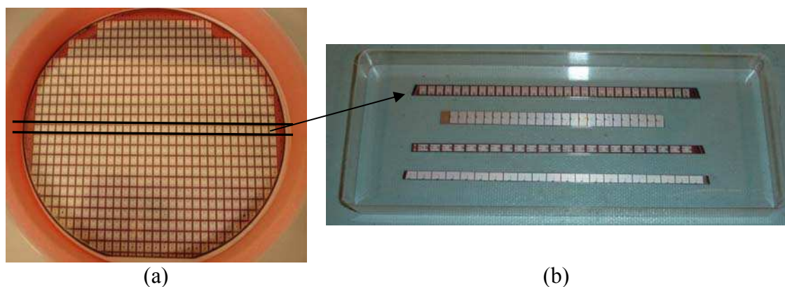
Figure 4.5 (a) Plaquette transistors IGBT, (b) Lamelles de MOSFET et d'IGBT
