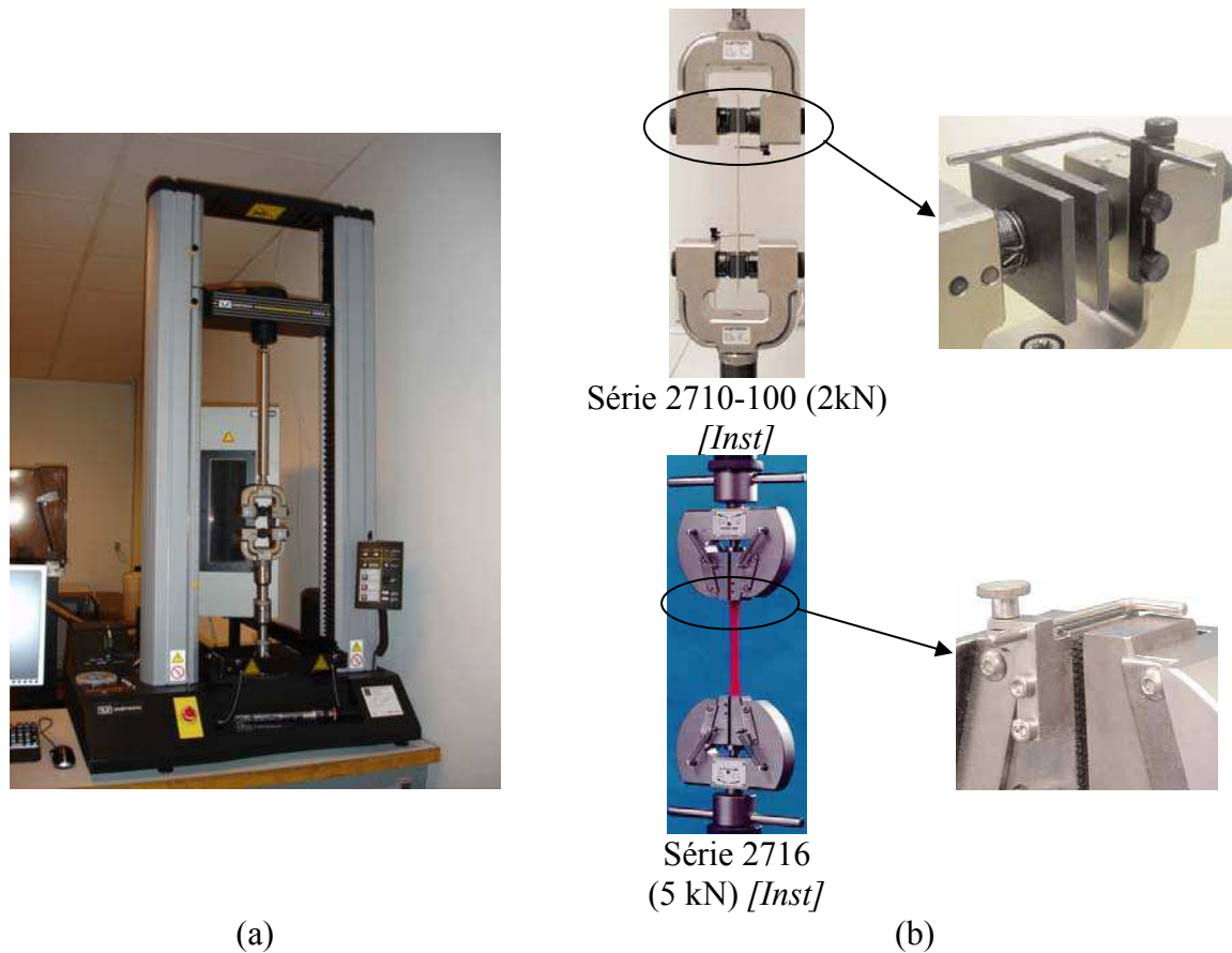
Figure 4.4 (a) Machine de caractérisation mécanique bi-colonnes INSTRON 5565, (b) Mors
