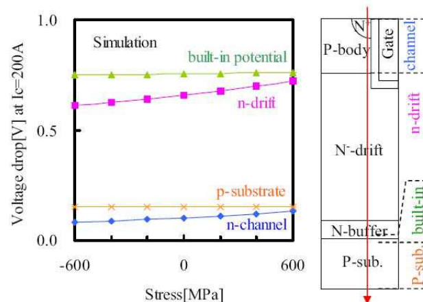
Figure 2.7 Variation de la tension des différentes régions de la structure en tranchée [Usui05]
