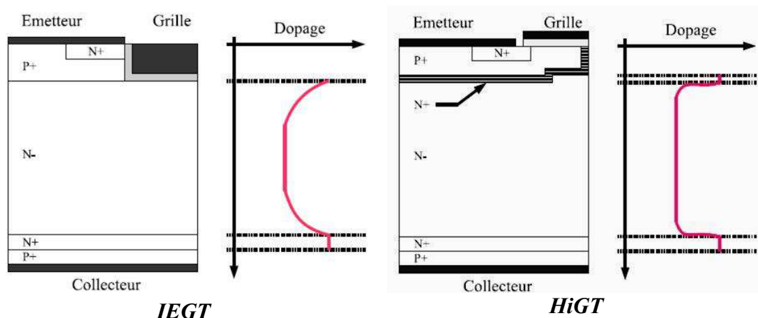
Figure 1.20 Coupe schématique des structures IEGT et HiGT et profil de dopage de la zone N-N +
