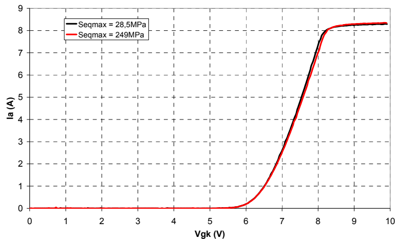
Figure 5.11 I_a(V_{gk}) suivant la contrainte mécanique appliquée à V_{ak} = 4 V « IGBT »
