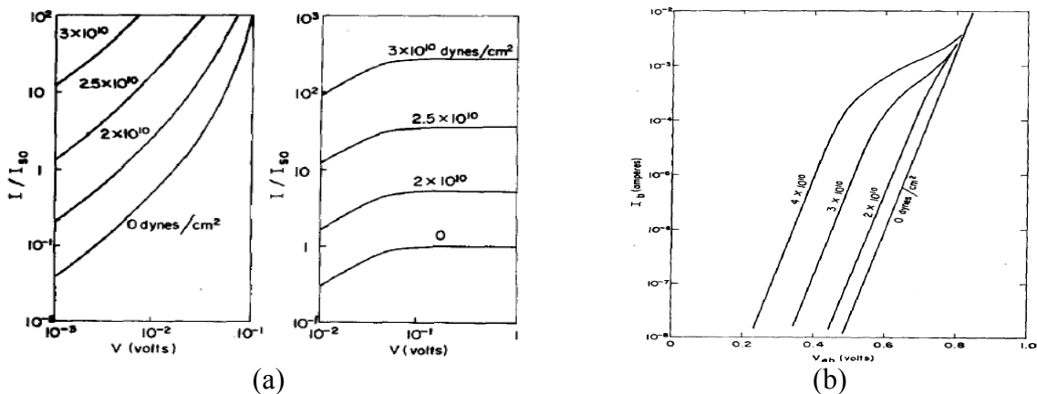
Figure 2.4 (a) I_d = f(V_d) d’une diode polarisée en direct et en inverse, (b) I_b = f(V_{be}) d’un transistor bipolaire [Wort64]
