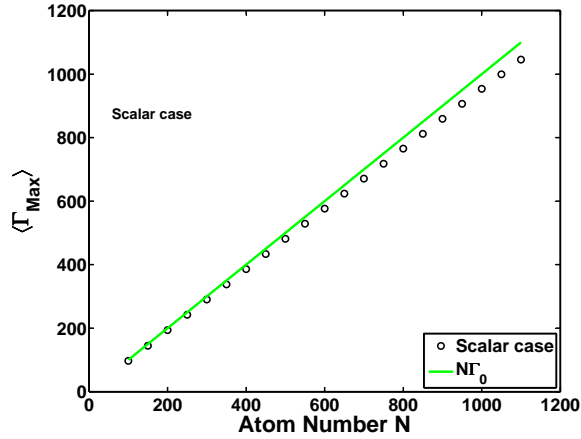
FIGURE 3.33 – Evolution de la largeur de mode associée à l'état superradiant en fonction du nombre d'atomes N dans le cas scalaire pour un nuage dont la densité est \rho\lambda^3 = 1.36.10^6 . On remarque clairement une déviation à la convergence de cette largeurs vers la valeur N\Gamma_0 .
