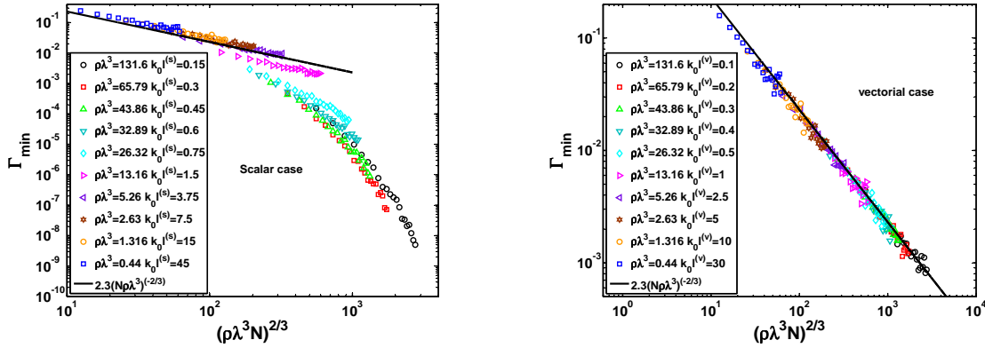
FIGURE 3.11 – Evolution de la valeur minimum moyenne des largeurs des modes \Gamma_{min} en fonction de (\rho\lambda^3 N)^{-2/3} dans les cas scalaire (figure de gauche) et vectoriel (figure de droite) pour des densités allant de \rho\lambda^3 = 0.44 à \rho\lambda^3 = 131.1 . Comme nous l’avons prévu à partir des distributions des valeurs propres de H_{eff} dans le plans complexe, que ce soit dans le régime dilué ou dans le régime dense le moment d’ordre 1 de la valeur minimum de largeur des modes est dominée par les paires sousradiantes dans le cas vectoriel alors que nous observons une nette rupture de pente dans le cas scalaire. Cette rupture de pente dans le cas scalaire apparaît aux grandes densités ( \rho\lambda^3 \simeq 26.32 ) et correspond à l’apparition de la concentration des valeurs propres ayant un long temps de vie autour d’une énergie bien précise ( E_{at} \simeq 1 ). Les traits pleins représentent l’équation (3.48) sur les deux graphiques.
