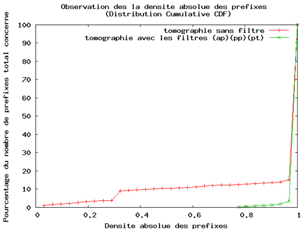
(a) Apparitions temporelles des différents préfixes avant et après application du filtre préfixe-temps (pt) et des filtres (pp)(ap) sur la tomographie T_{2005-01}
