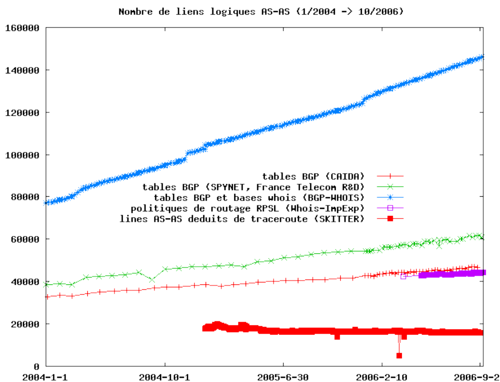
(b) Evolution du nombre de liens inter-AS en fonction du temps
