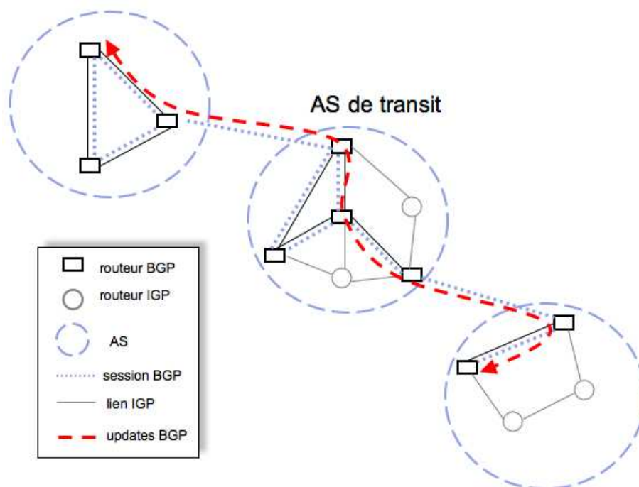
(b) Exemple d'un AS d'un opérateur de transit. Un AS de transit transmet des messages d'update BGP entre différents AS.
