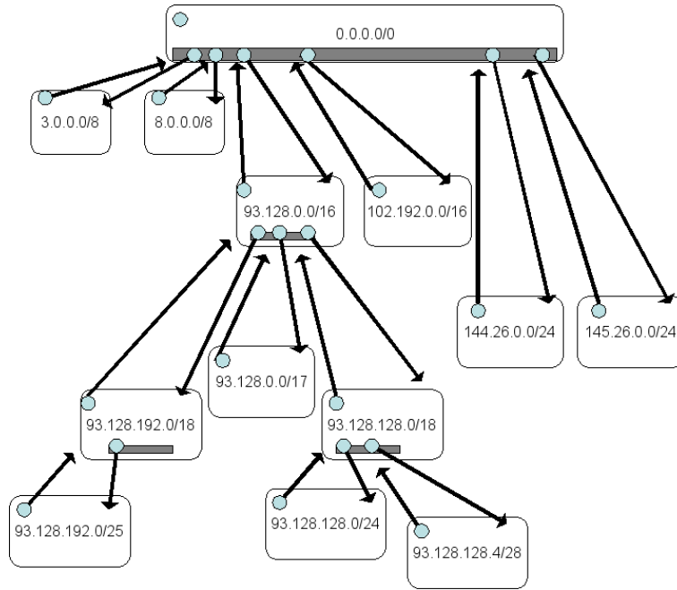
FIG. D.2 – Exemple d'arbre de préfixe
