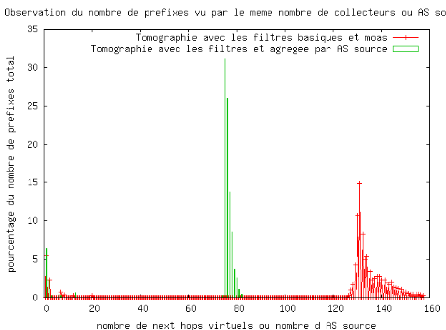
FIG. B.7 – Préfixes observés par le même nombre de collecteurs (next hop virtuels) ou le même nombre d’AS sources
