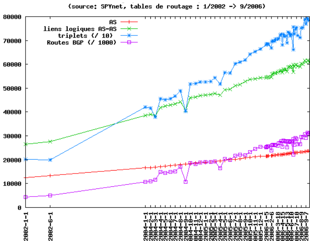
(a) Evolution des nombres d'AS, de liens AS-AS, de triplets d'AS et de routes BGP. La légende indique le cas échéant le facteur d'échelle qui a été utilisé pour chaque indicateur.
