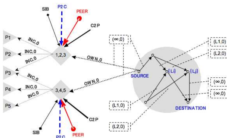
(b) un noeud du graphe étendu des AS-préfixe. D'une part le nombre de Local Pref clients est propre à chaque AS. D'autre part, les différents agrégats de préfixes sont aussi propres à chaque AS. Le poids des arcs d'inclusion et des arcs d'accès est égal à e .
