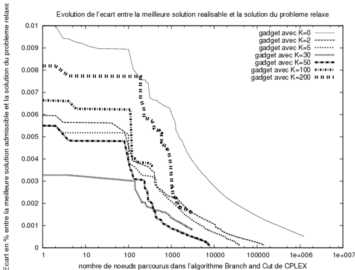
FIG. 3.16 – Évolution de la valeur du gap de résolution au cours de l’algorithme Branch & Cut en fonction du nombre d’itérations de CPLEX et de différents valeurs du nombre de K-plus-courts chemins pour l’énumération des coupes gadget
