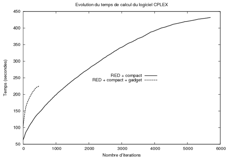
FIG. 3.17 – Effet de l'utilisation des coupes gadget sur le temps d'exécution du logiciel CPLEX.
