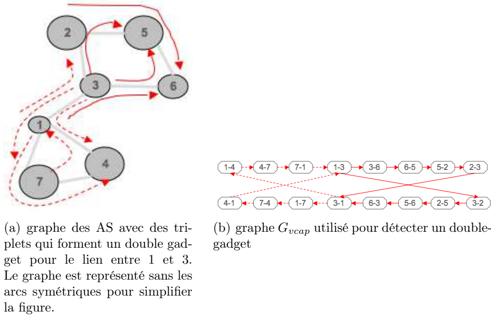
FIG. 3.11 – Double contrainte gadget, appelée chestnut
