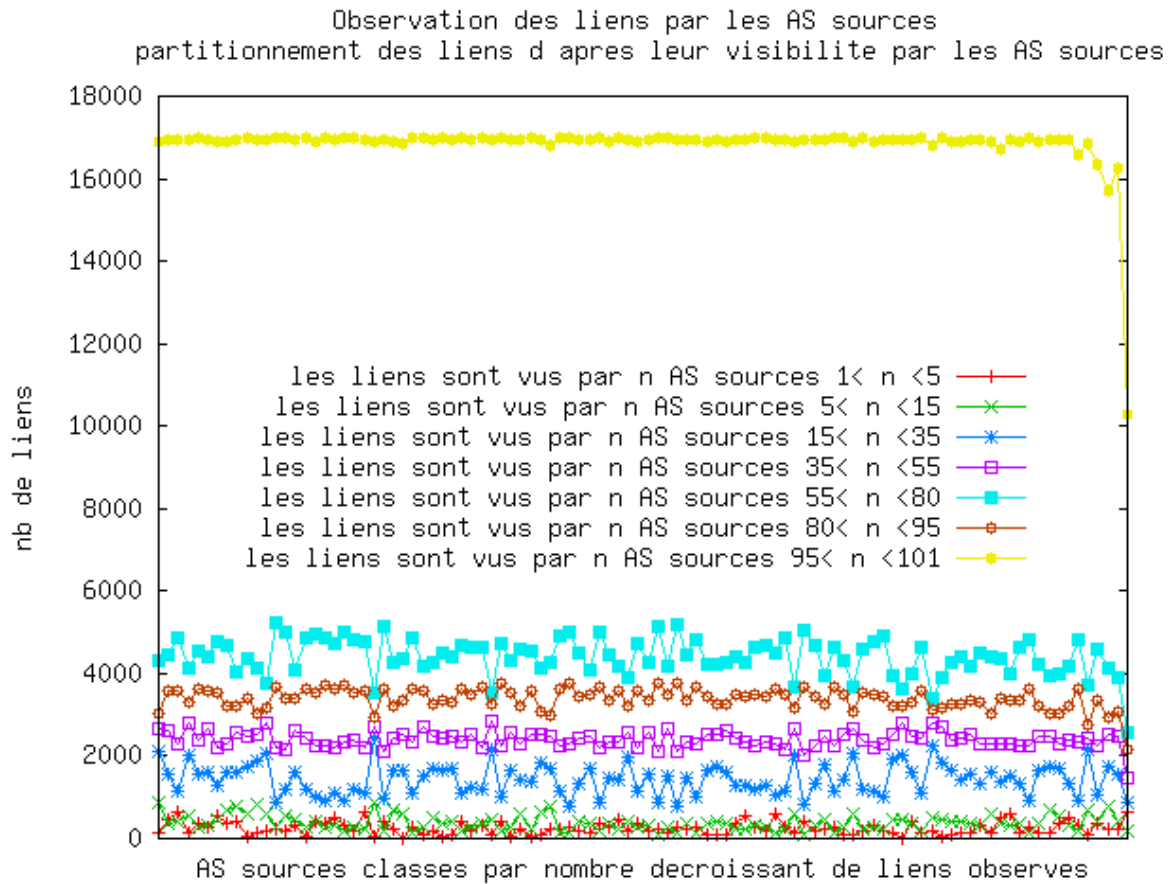
(a) tomographie T_{2006-08}
