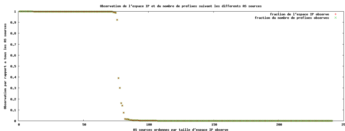
FIG. B.8 – Nombre de préfixes et fraction de l’espace d’adresses IP visible par chaque AS source. Les AS sources sont classés par fraction d’espace d’adresses IP visible
