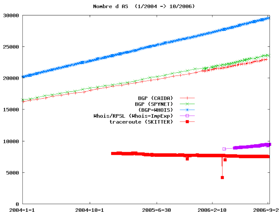
(a) Evolution du nombre d'AS en fonction du temps
