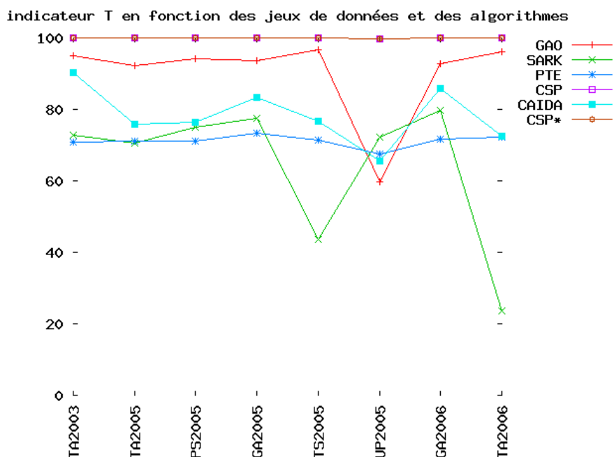
FIG. 3.19 – Valeurs de l'indicateur T pour les différentes solutions des algorithmes en fonction des jeux de test
