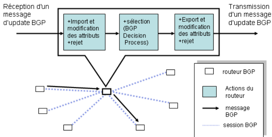
(b) Le traitement d'un message d'update BGP par un routeur. La sélection et l'acceptation d'une route BGP reçue par une session est fonction de la politique de routage. La sélection de la meilleure route BGP est effectuée par le BGP Decision Process. L'export de la meilleure route modifiée pour un préfixe dépend de la session BGP de sortie et des attributs de la route.
