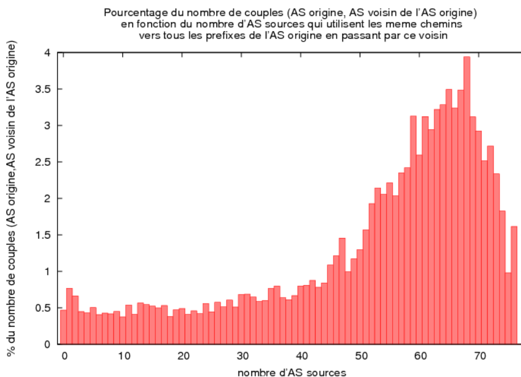
FIG. 2.20 – Nombre de couples (AS origine, AS voisin de l'AS origine) dont le même nombre d'AS sources observe exactement les mêmes chemins vers les différents préfixes de l'AS origine en passant par l'AS voisin de l'AS origine.
