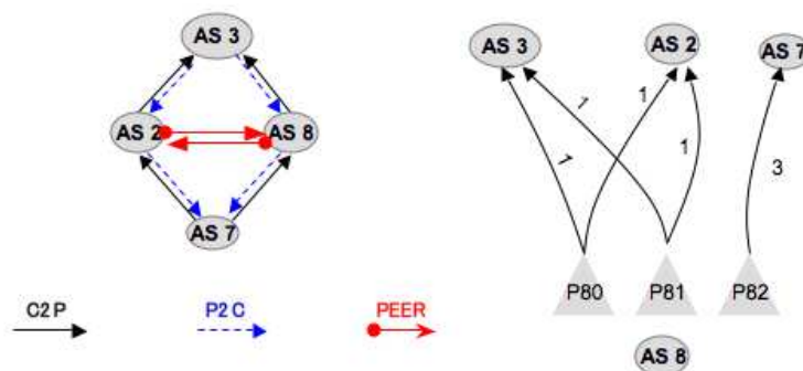
(a) exemple de graphe des AS avec l'illustration de la matrice de politique d'annonce de l'AS 8.
