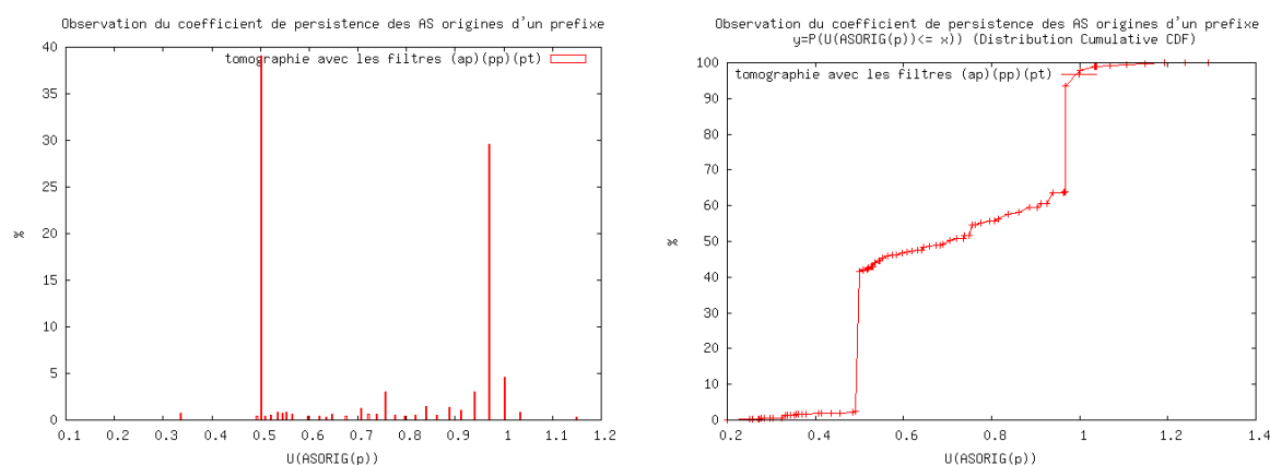
(a) U(ASORIG(p)) pour la tomographie T_{2005-01}
