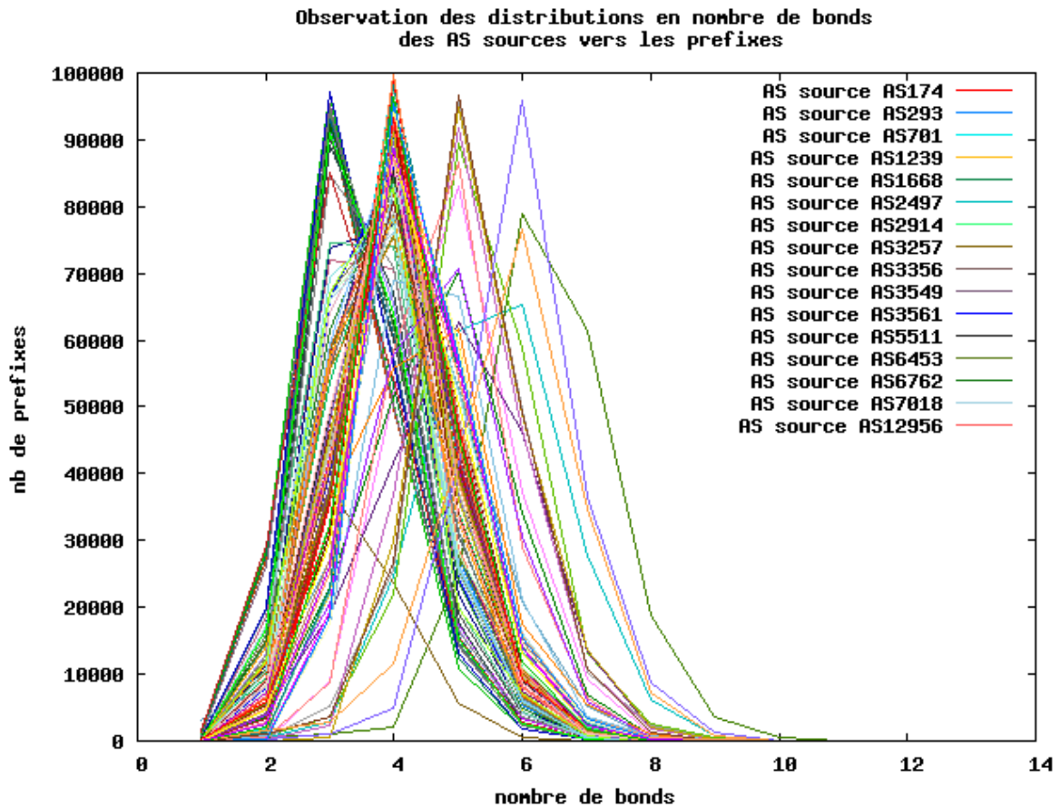
(a) Les AS de la légende sont ceux dont les distributions ont un pic à 3 bonds.
