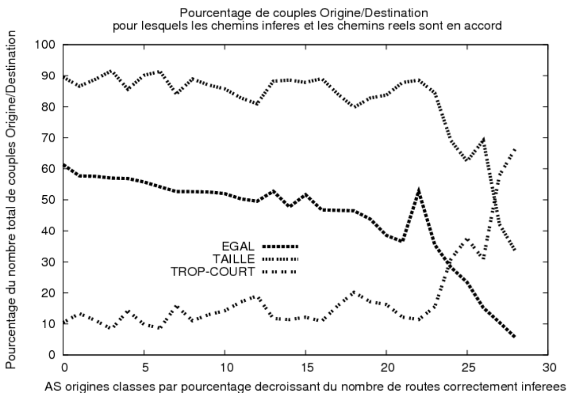
(a) modèle G-AS utilisé avec la tomographie P_{2003}
