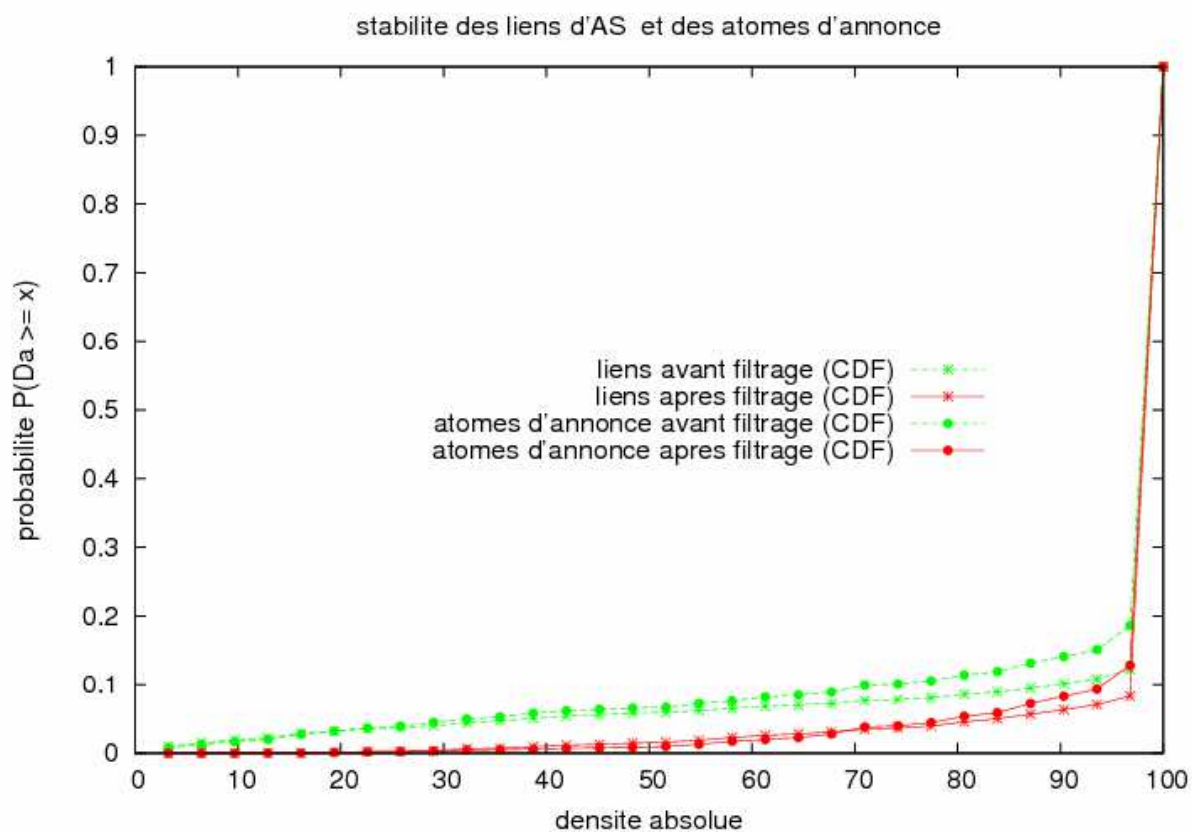
FIG. 2.6 – Filtrage des atomes d’annonce et des liens en fonction de la densité absolue
