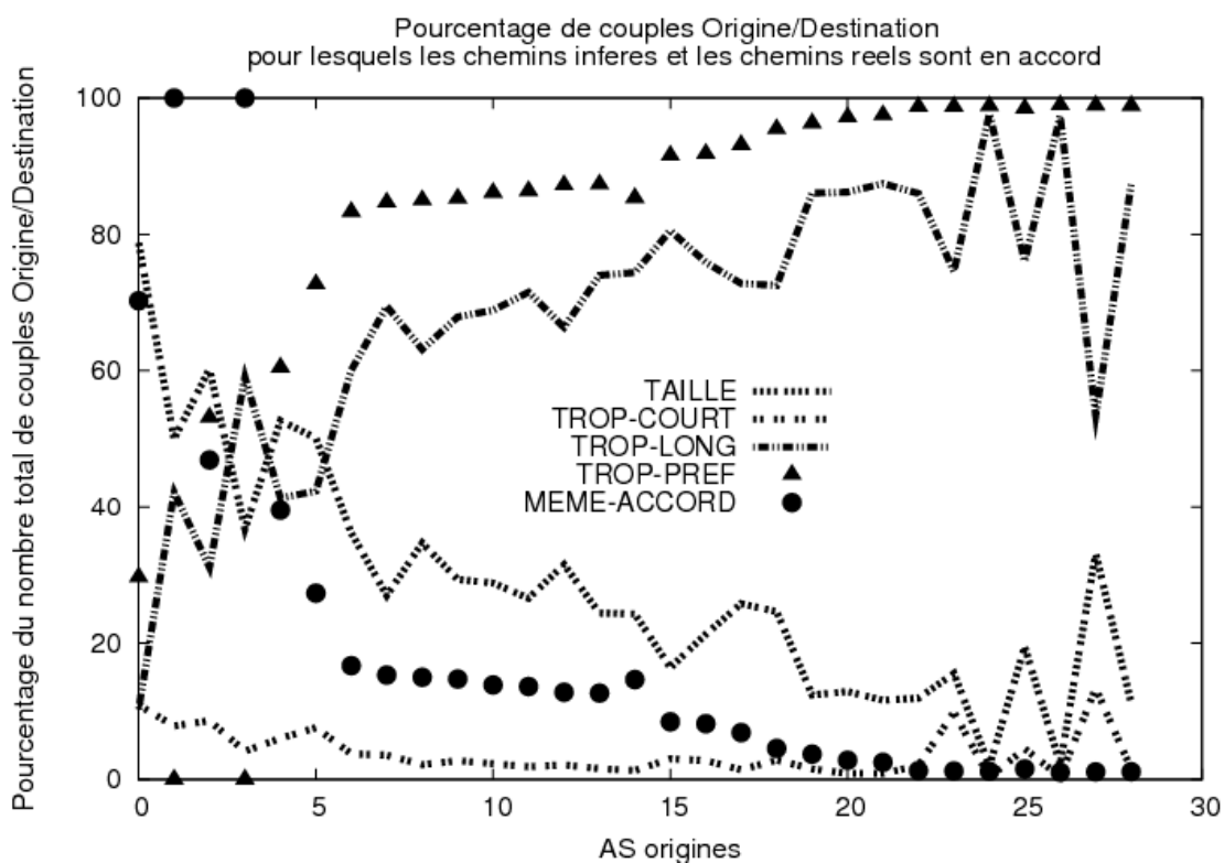
(a) modèle G - LP utilisé avec la tomographie P_{2003}
