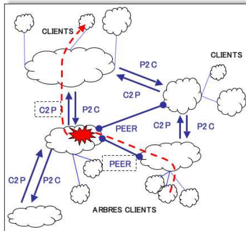
(d) Cheminement invalide (1)
