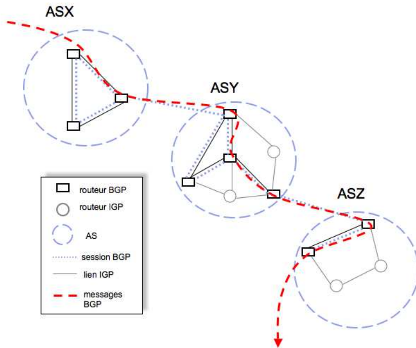
(a) Un atome de politique de transit correspond à un chemin d'AS de taille 3 déduit d'un attribut AS Path d'un message BGP.
