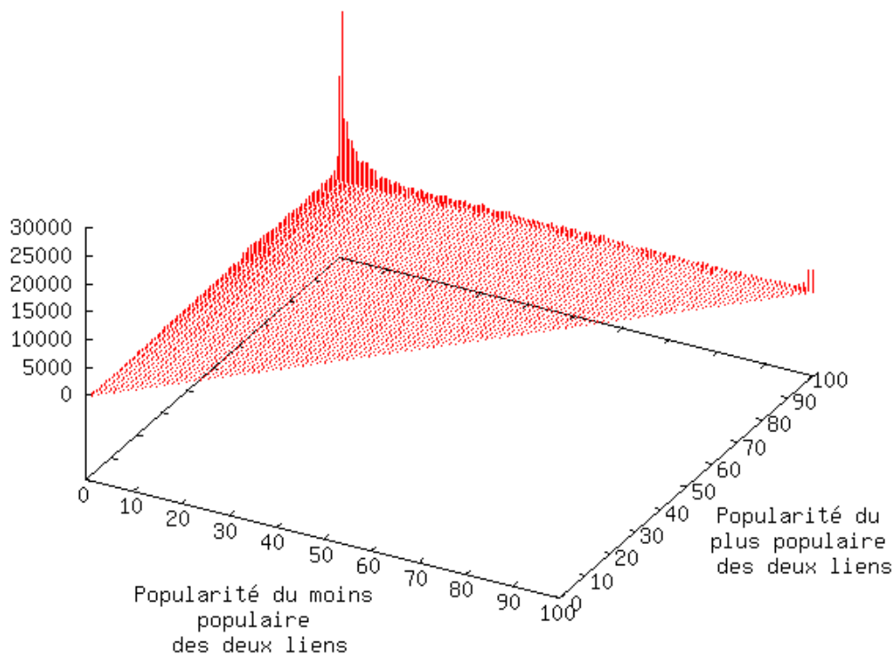
(a) tomographie T_{2006-08}
