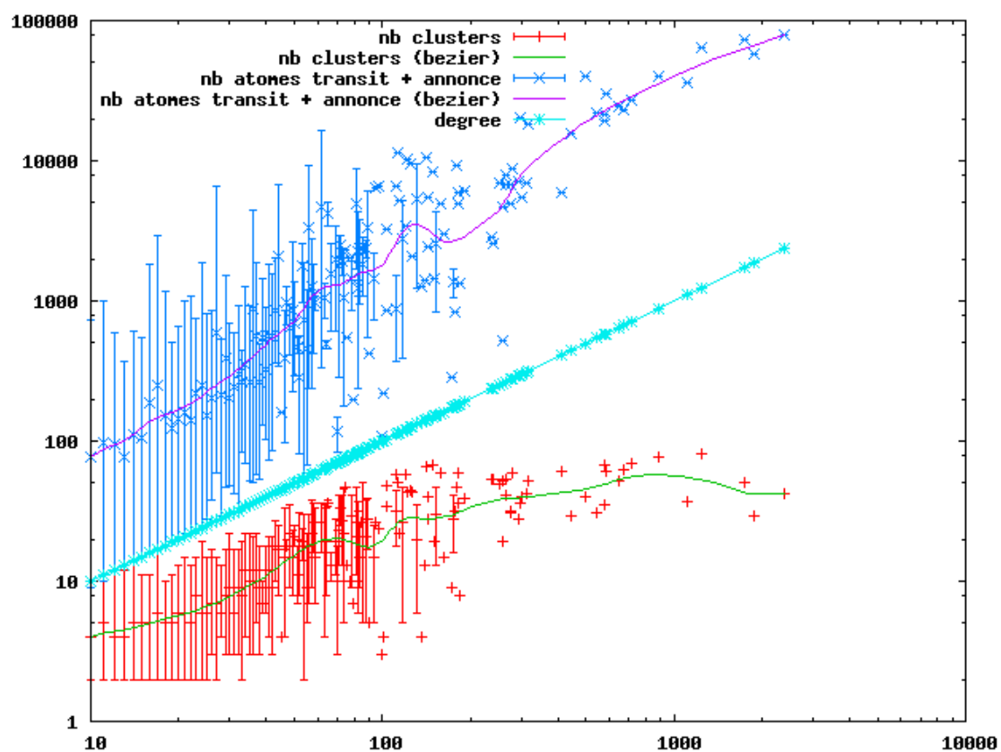
FIG. 2.22 – Nombre de clusters et nombre d’atomes de politique de routage d’un AS en fonction de son degré
