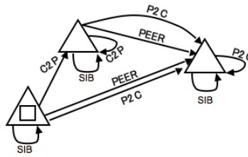
FIG. 3.3 – Automate de construction des labels de chemins valides
