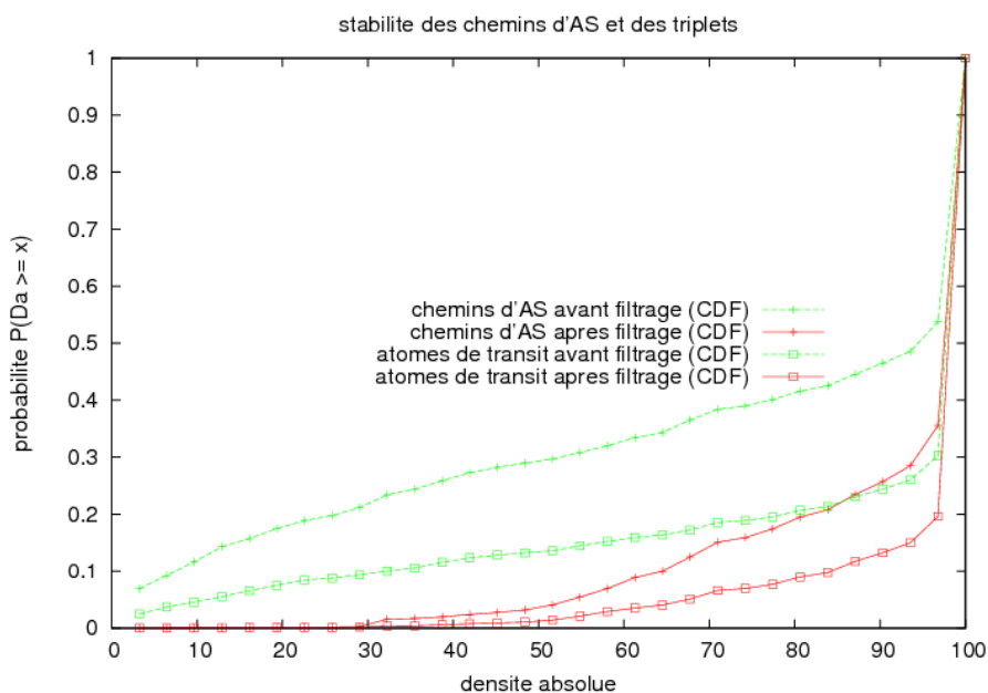
FIG. 2.7 – Impact des filtres (lt) et (aat) sur la densité absolue des chemins et des préfixes
