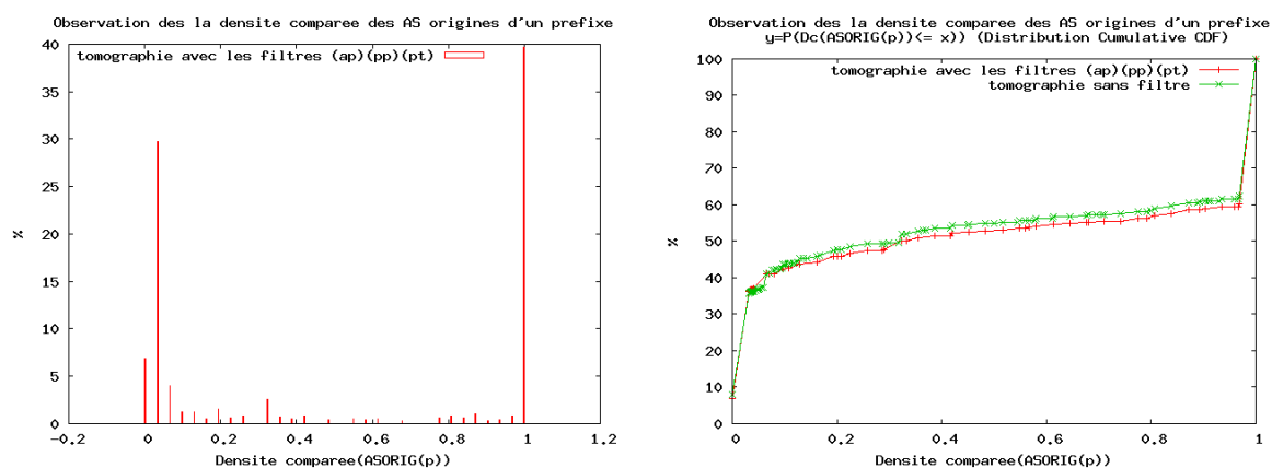
(a) D_c(ASORIG(p)) pour la tomographie T_{2005-01}
