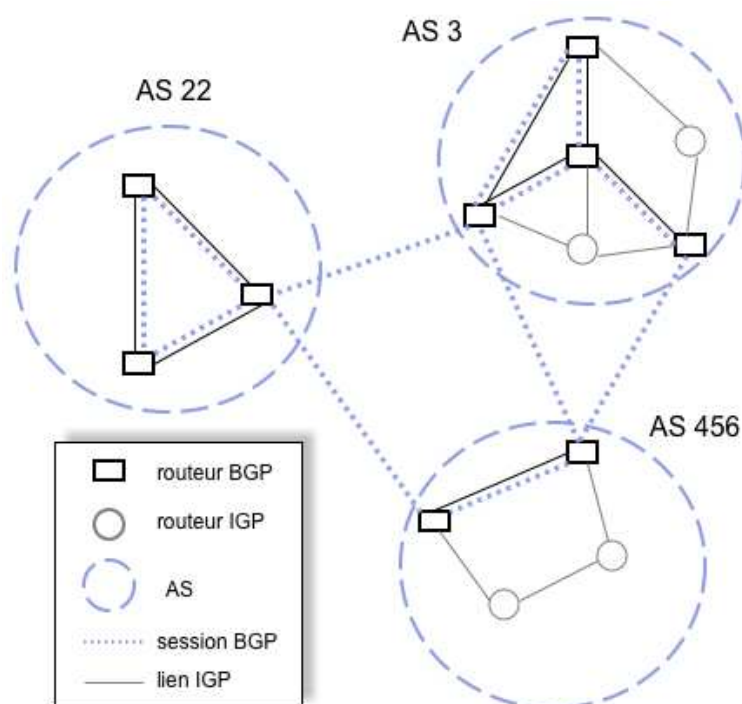
FIG. 1.4 – Un exemple de réseau BGP formé de 3 AS.
