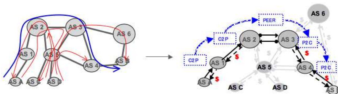
FIG. 3.4 – Exemple de problème d'inférence des accords d'interconnexion
