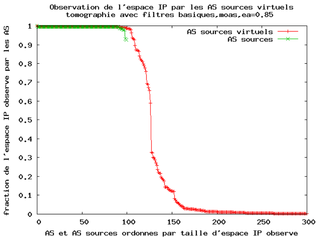
(b) tomographie T_{2006-08}
