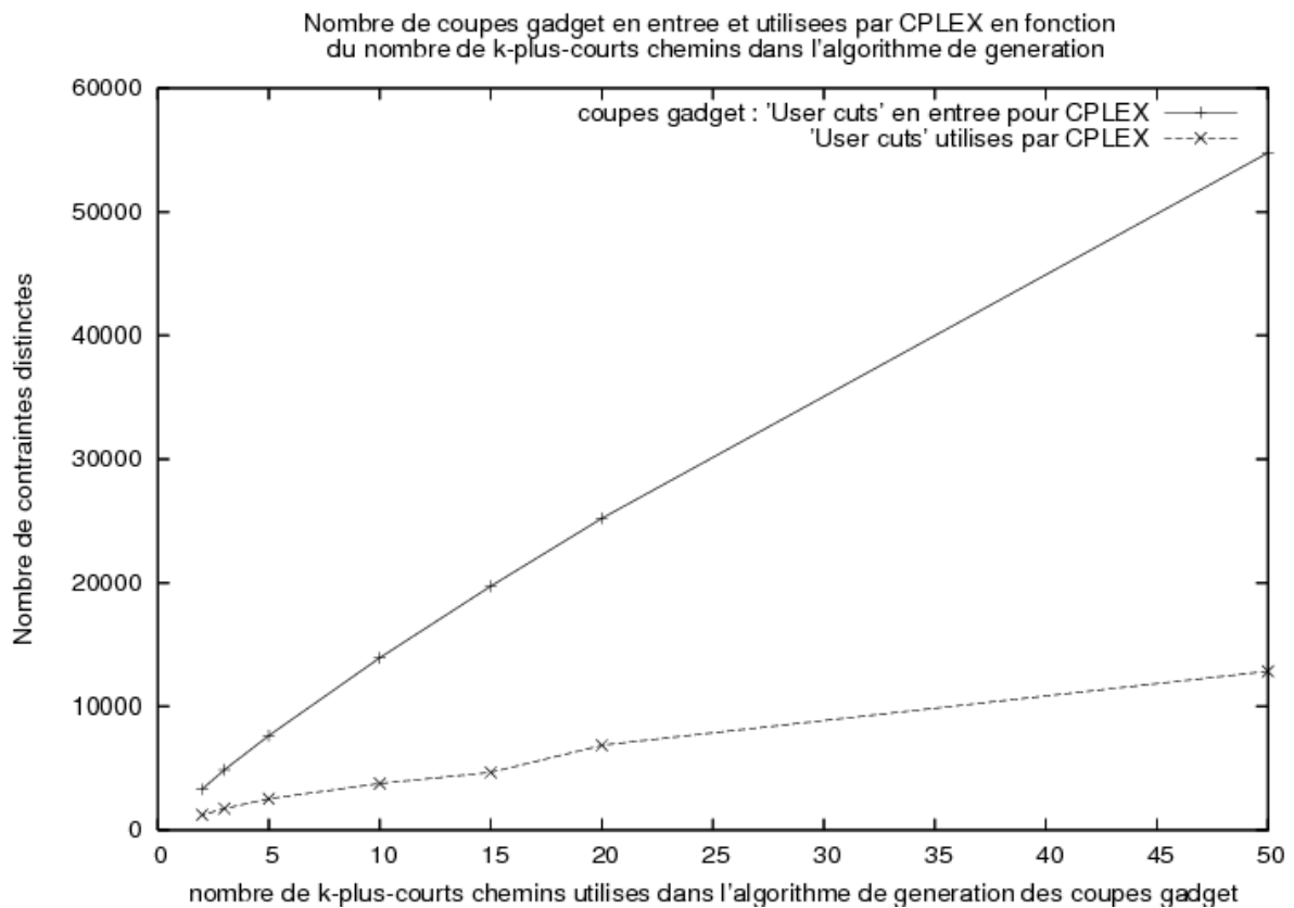
FIG. 3.14 – Nombre de coupes gadget utilisées pour le jeu de test
