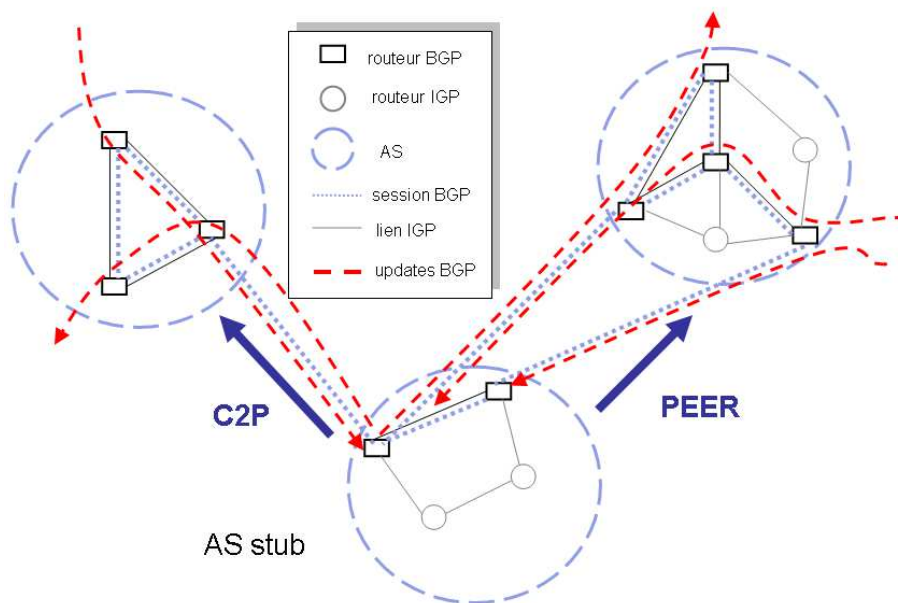
(a) Exemple d'un AS stub. Les AS stub sont des clients finaux et ne transmettent pas les messages BGP entre leurs AS voisins (fournisseurs ou peer).
