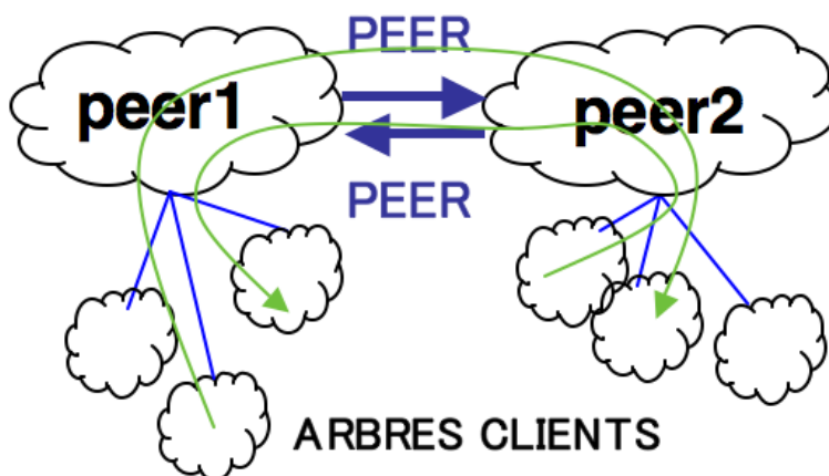
(b) Relation de Peering : deux opérateurs partagent gratuitement les communications entre leurs clients (et les clients des clients...). Les relations de peering sont notés PEER.
