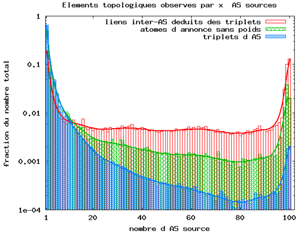
(a) tomographie T_{2006-08}
