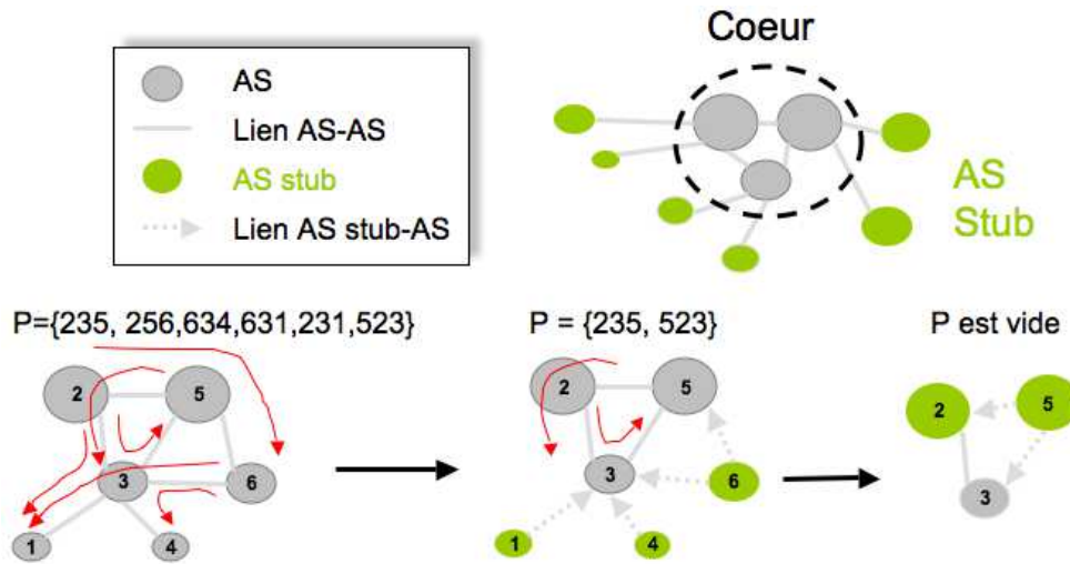
FIG. 2.23 – Illustration de la hiérarchie simple induite par les triplets
