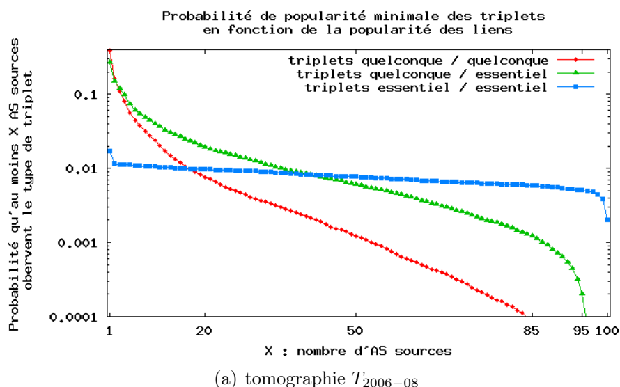
FIG. 2.17 – Répartition des différentes popularités de triplets d’AS en fonction de la popularité des liens.
