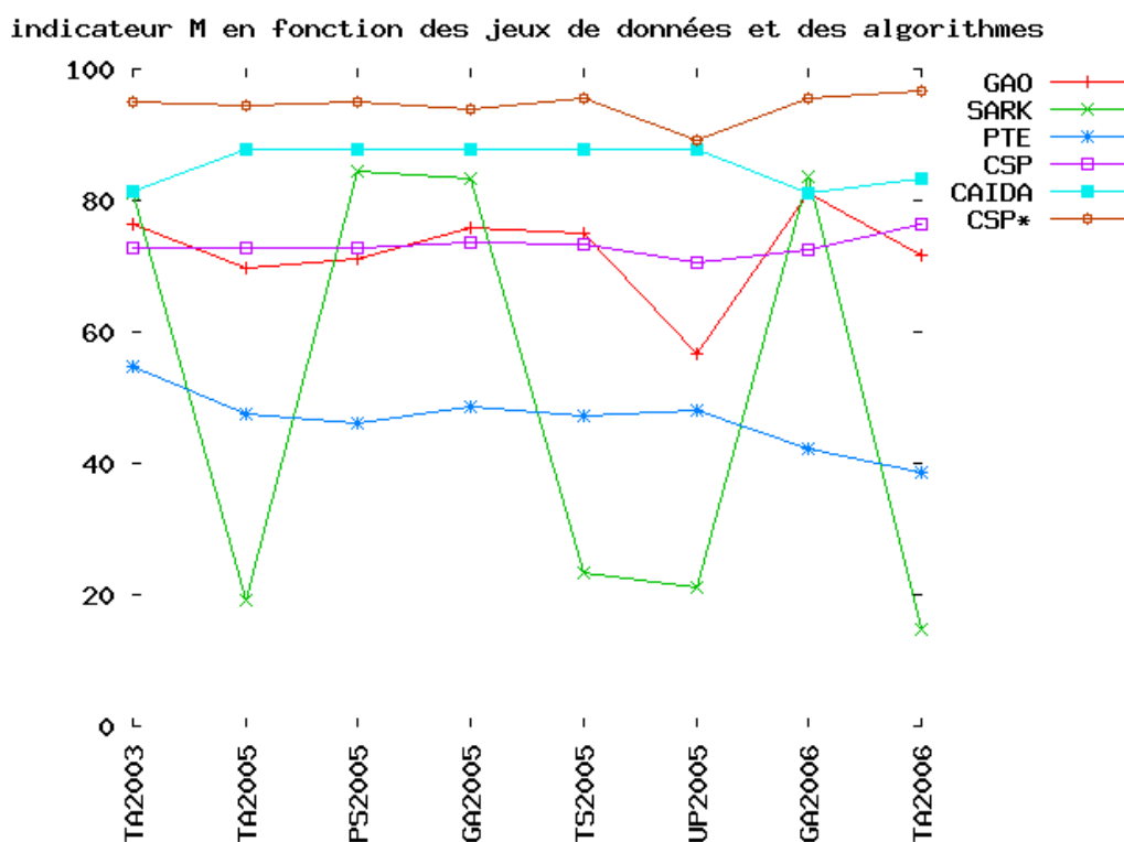
FIG. 3.20 – Valeurs de l’indicateur M pour les différentes solutions des algorithmes en fonction des jeux de test
