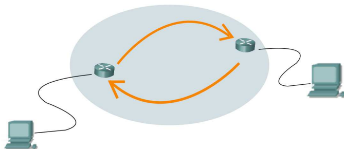
FIG. 1.1 – Asymétrie des chemins dans le réseau Internet
