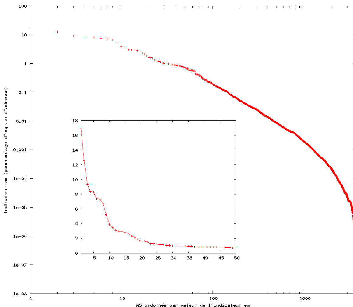
FIG. 2.24 – Pourcentages des espaces d'adresses transitées moyen par AS source pour la tomographie T_{2006-08}
