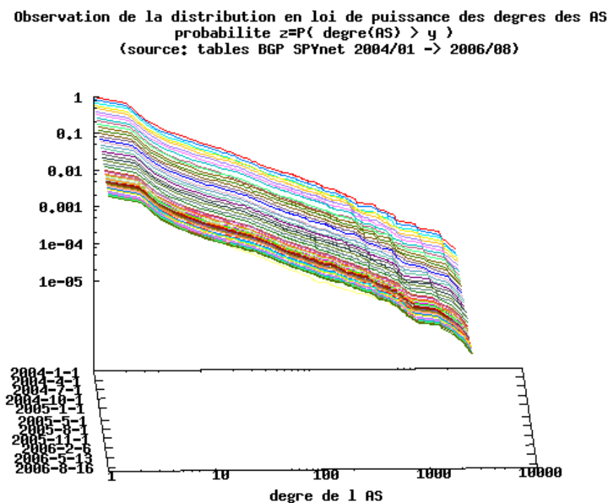
FIG. 2.4 – Loi de distribution des degrés des AS pour les topologies interdomaines dans l'application SpyNET
