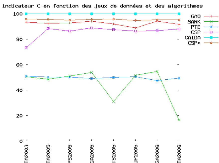
FIG. 3.21 – Valeurs de l'indicateur C pour les différentes solutions des algorithmes en fonction des jeux de test
