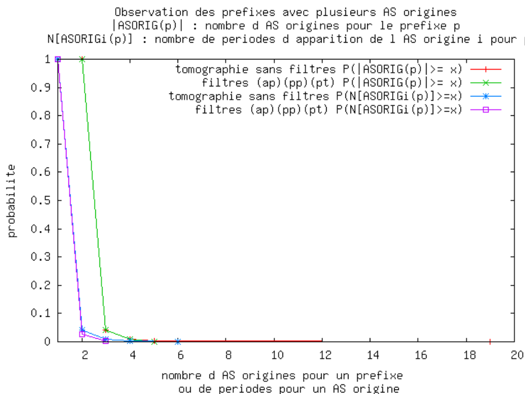
FIG. B.4 – Répartition des valeurs M(ASORIG(p)) et N(ASORIG(p)) avant et après filtrage (pp), (ap) et (pt = 0.75)
