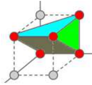
(a) Sur cette figure, la dimension est n = 3 . Les points rouges correspondent aux m = 5 éléments (\phi_1, \dots, \phi_m) \in \{0, 1\}^3 \times \dots \times \{0, 1\}^3 . L'enveloppe convexe correspond au volume dessiné. Les points gris sont les éléments de l'ensemble \{0, 1\}^n \setminus (\phi_1, \dots, \phi_m) .
