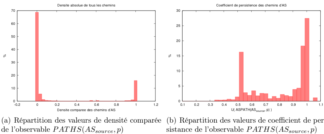
FIG. 2.10 – Répartition des valeurs de densité comparée et de coefficient de persistance pour l'observable PATHS(AS_{source}, p) .
