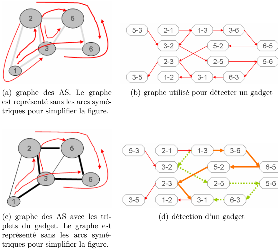
FIG. 3.10 – Détection d'une contrainte gadget
