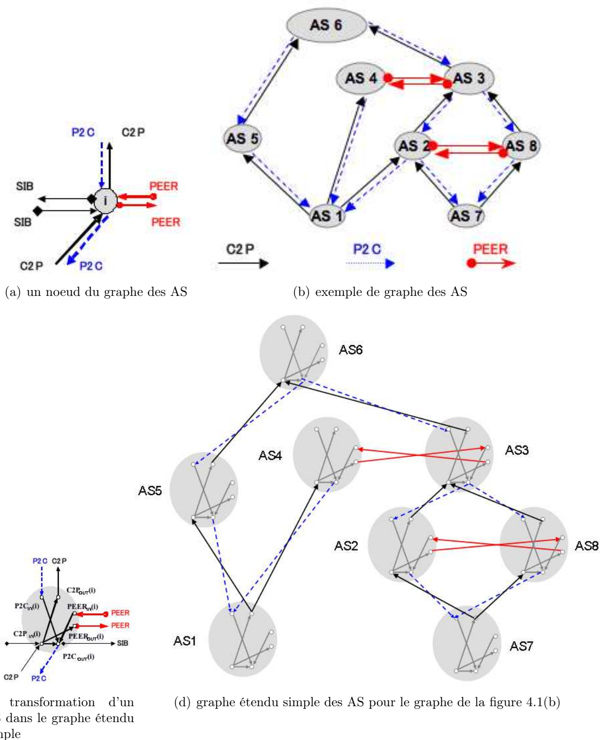
FIG. 4.1 – Exemple de transformation d'un graphe des AS en graphe étendu simple des AS
