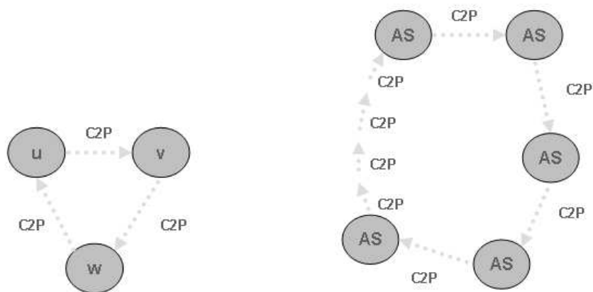
(a) Cycle de relations C2P de taille 3. (b) Cycle de relations C2P de taille quelconque.
