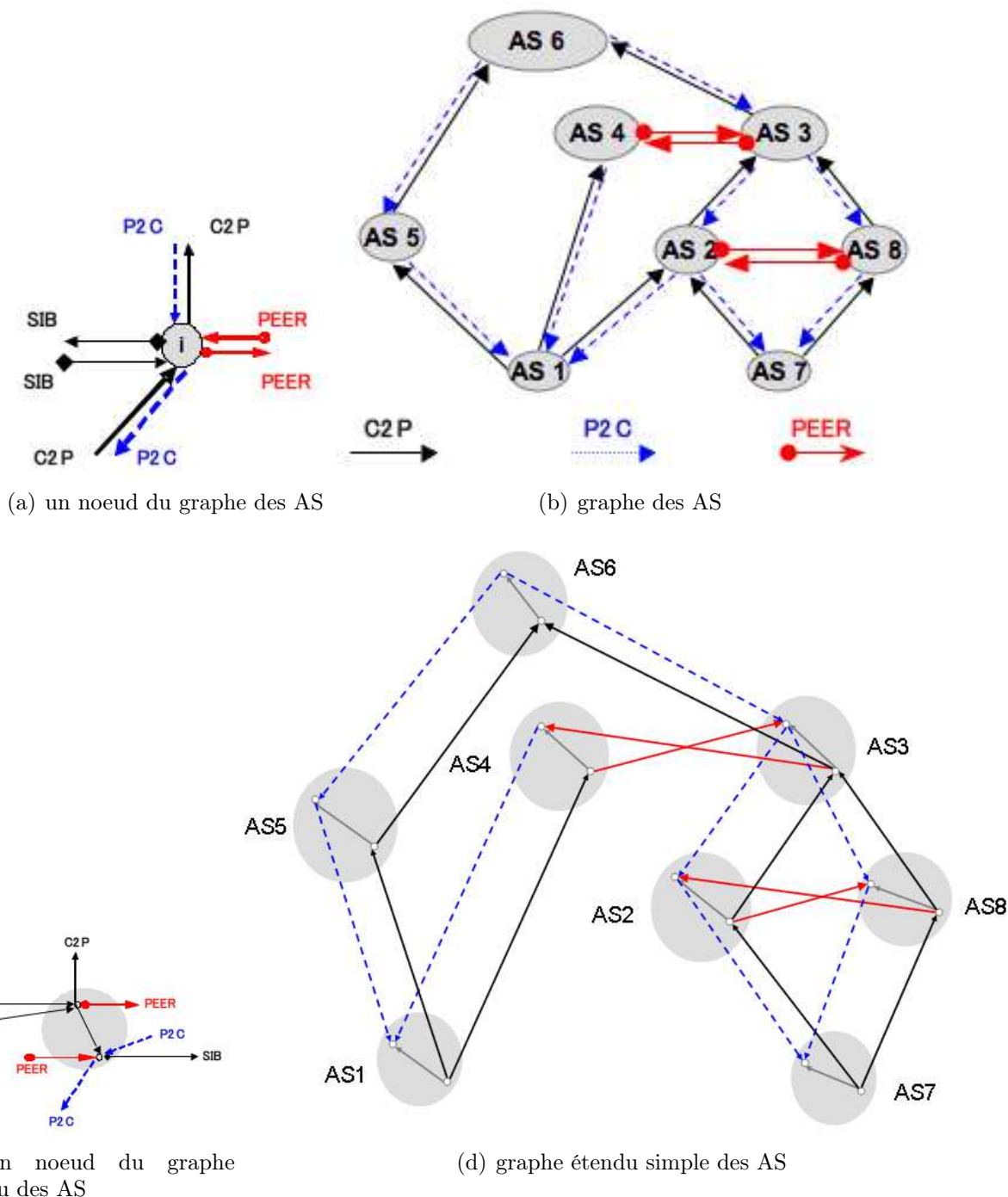
FIG. 4.3 – Transformation du graphe des AS en graphe étendu des AS
