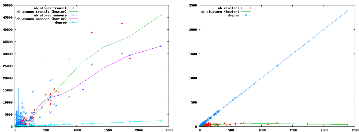
(a) Nombre d’atomes de transit et d’annonce en fonction du degré d’un AS (b) Nombre de clusters en fonction du degré d’un AS
