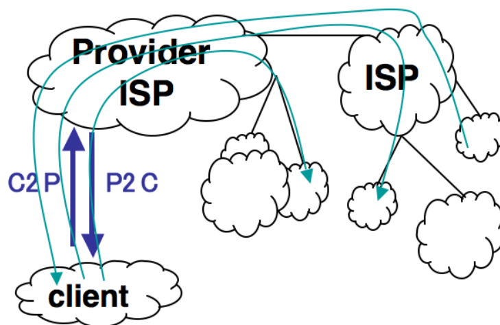
(a) Relation de Transit : un opérateur client paye un fournisseur pour pouvoir communiquer avec ses partenaires peering, clients et fournisseurs dans les deux sens. La relation d’un client vers un fournisseur est notée C2P, et la relation d’un fournisseur vers un client est notée P2C.
