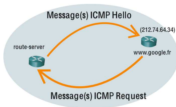
(a) Illustration d'une commande ping du routeur "route-server" vers l'adresse 212.74.64.34
