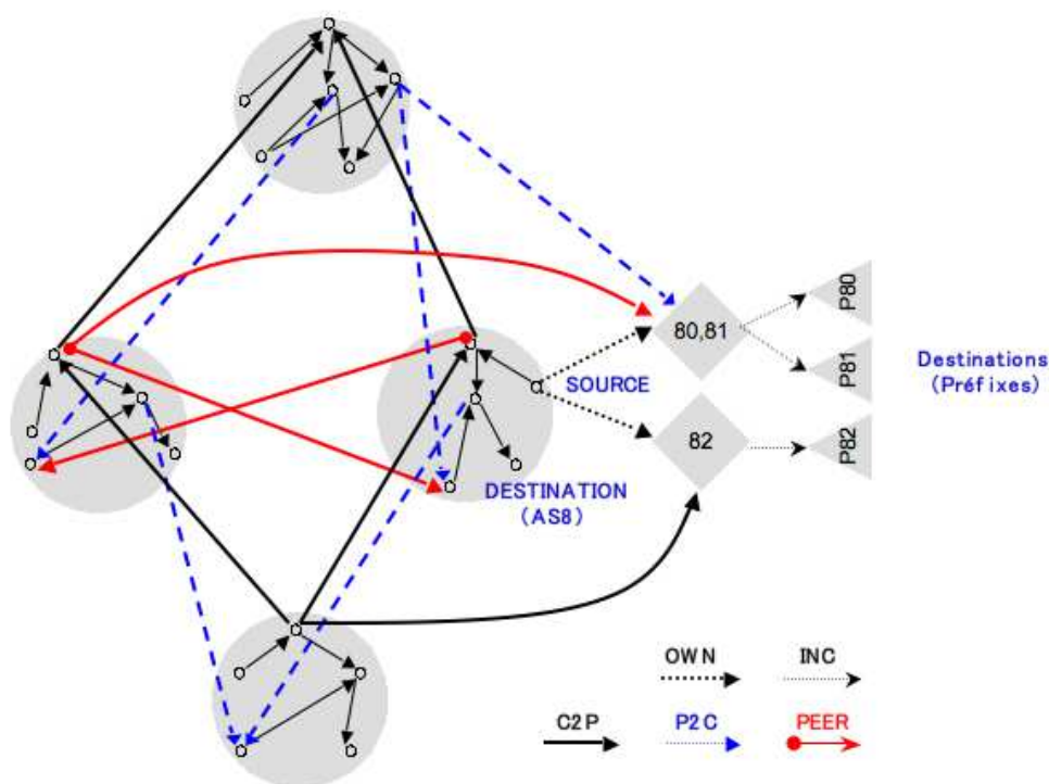
(c) transformation du graphe de la figure 4.8(a) en graphe étendu AS-préfixe.
