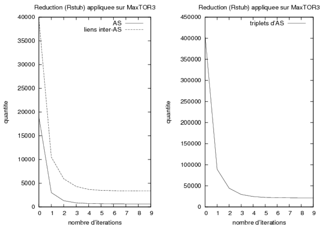
FIG. 3.13 – Effet de l’algorithme de réduction ( R_{stub} ) sur le jeu le test.
