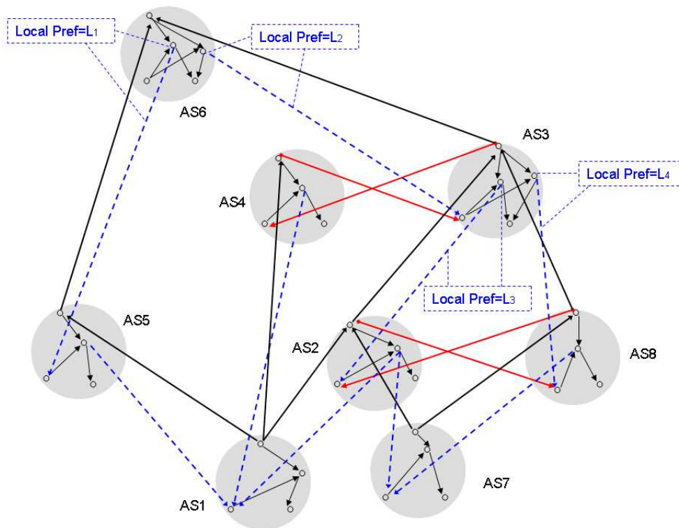
(b) graphe étendu des AS avec prise en compte de différentes valeurs de Local Pref pour les clients d'un même AS. Les valeurs de Local Pref indiquées avec des cadres en pointillés désignent des sommets internes ou des poids sur les liens.
