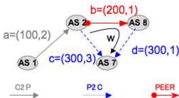
FIG. 4.4 – Non distributivité à gauche pour la structure algébrique des poids
