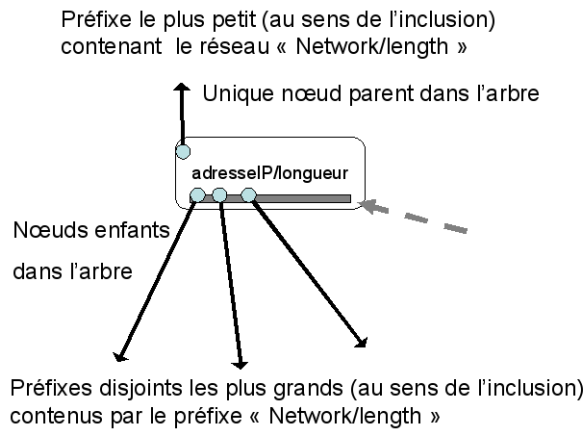
FIG. D.3 – Un noeud dans l'arbre de préfixes
