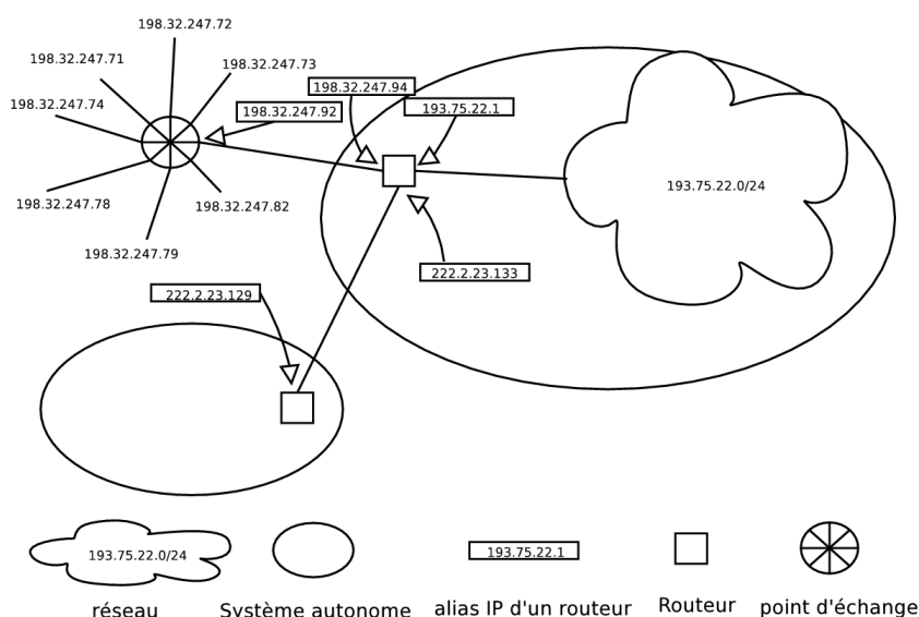
FIG. 1.7 – Exemple où un routeur a plusieurs interfaces IP dans des plans d’adressage différents
