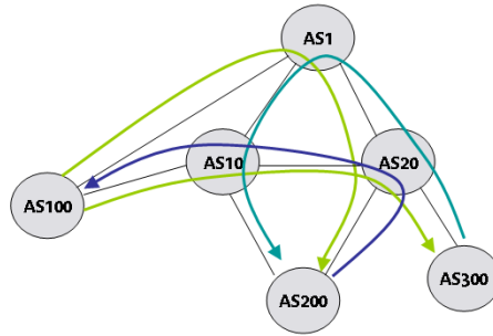
(a) Une topologie interdomaine avec 4 AS_PATH
