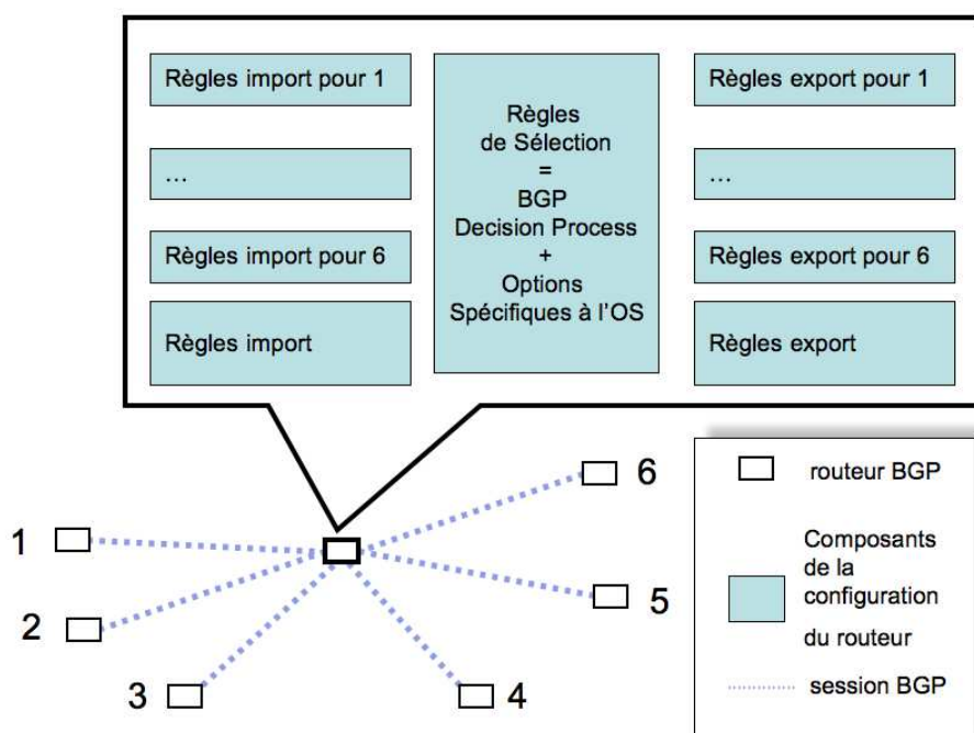
(a) Règles issues de la politique de routage d'un routeur BGP. Une route est traitée d'après la session BGP d'entrée, ses attributs BGP et la session BGP de sortie.
