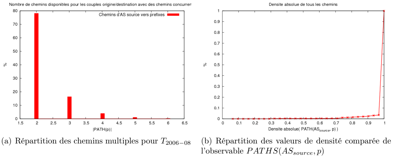
FIG. 2.9 – Loi de répartition des densité absolues des chemins multiples pour les AS sources vers les préfixes
