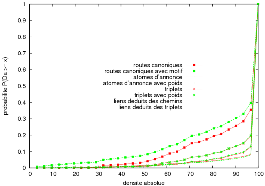
FIG. 2.8 – Répartition des éléments topologiques fonction de la densité absolue
