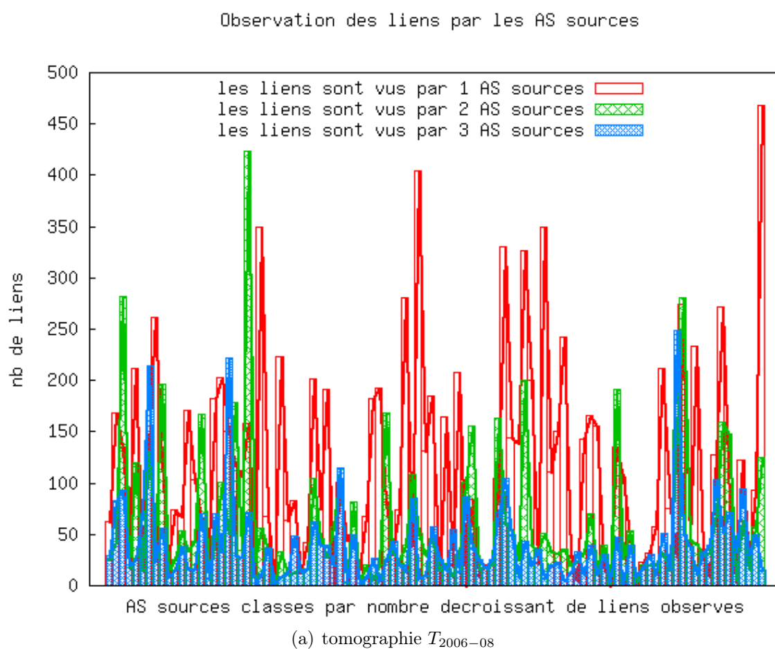
FIG. 2.12 – Liens inter-AS observés par un, deux ou trois AS sources seulement
