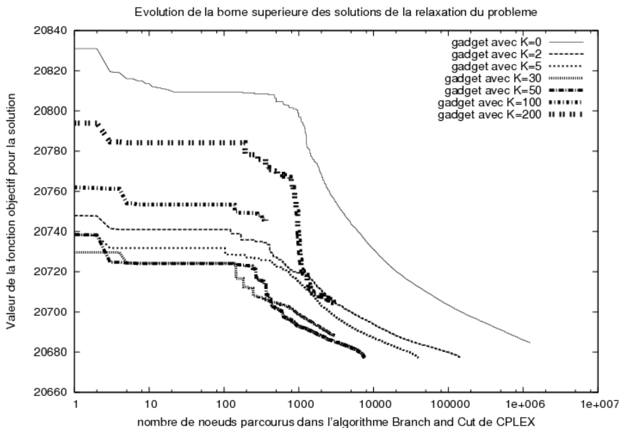
FIG. 3.15 – Évolution de la borne supérieure des solutions du problème relaxé en fonction du nombre d'itérations de CPLEX et du nombre de K-plus-courts chemins utilisés pour l'énumération des coupes gadget
