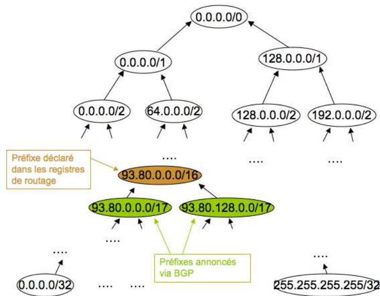
FIG. 2.26 – Découpage des préfixes déclarés dans les registres de routage pour les annonces via le protocole BGP
