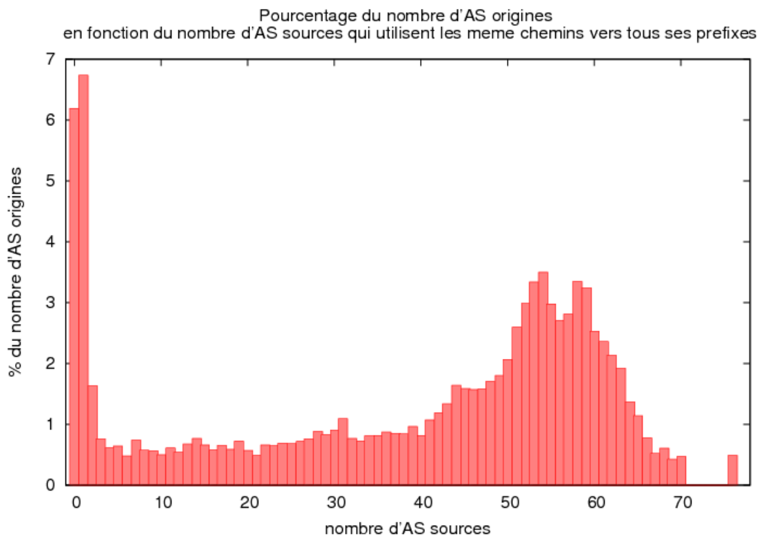
FIG. 2.19 – Nombre d'AS origines dont le même nombre d'AS sources observe exactement les mêmes chemins vers les différents préfixes de l'AS origine.
