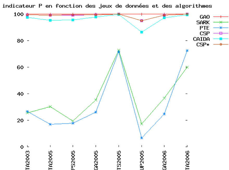
FIG. 3.18 – Valeurs de l'indicateur P pour les différentes solutions des algorithmes en fonction des jeux de test
