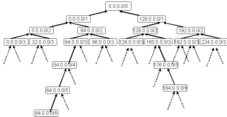
FIG. D.1 – Arbre binaire contenant tous les préfixes réseaux
