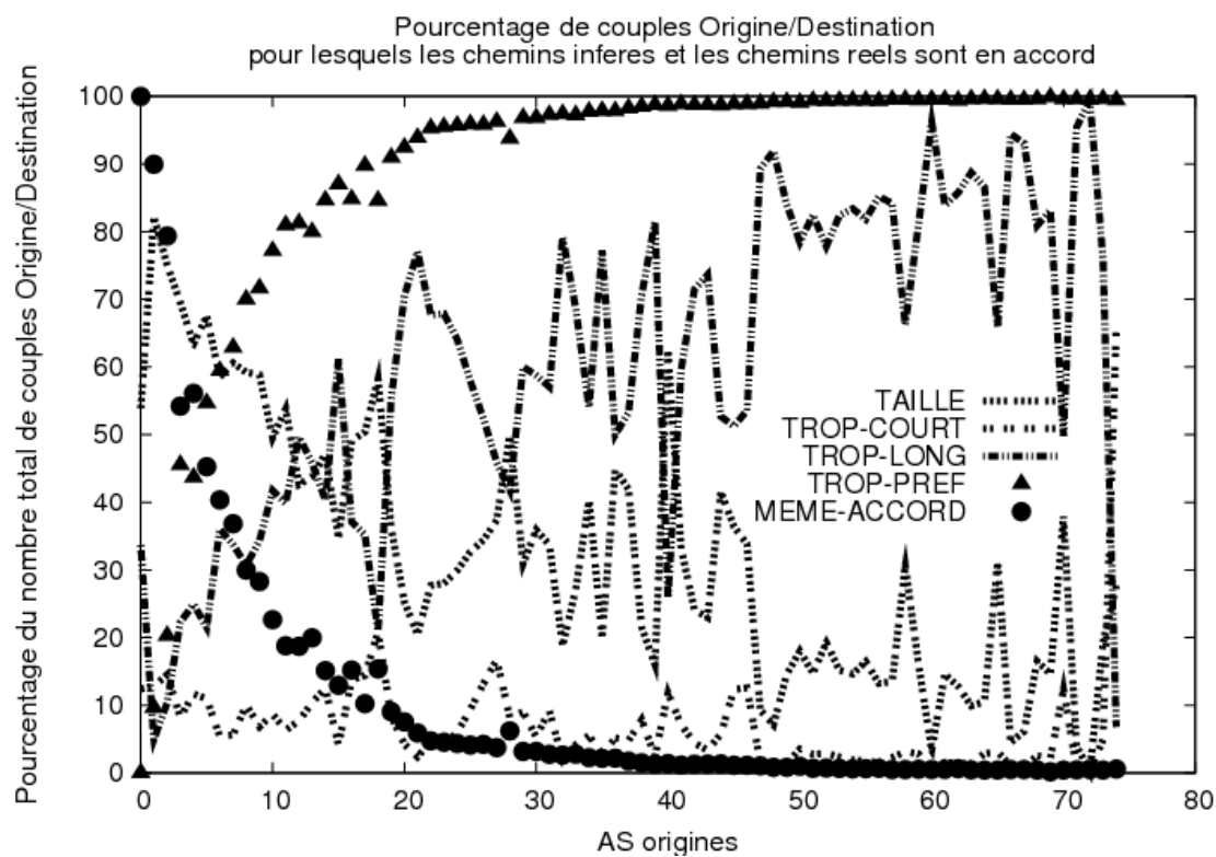
(b) modèle G - LP utilisé avec la tomographie P_{2005}
