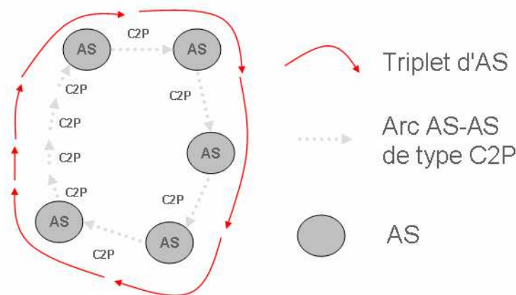
(a) Cycle de relations C2P cumulé avec un cycle de triplets. Dans ce cas précis, l'interdiction de cycles de relations C2P oblige au moins un triplet du cycle à être invalide.
