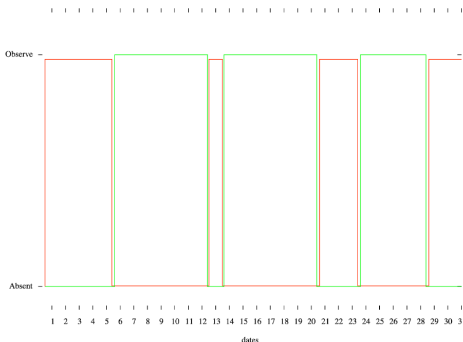
(a) Observation des deux routes du next hop BGP 198.32.176.177 de la sonde route - views - palo - alto(usa) pour le NLRI 193.54.79/24 pour 31 dates. Dans cet exemple, l'observable \alpha est la route d'un collecteur vers un préfixe. Les valeurs de l'observable sont les deux routes observées : M(\alpha) = 2 . Pour la route 1 : N(1) = 2, d_1 = 30, D_a(1) = \frac{22+4}{31} = D_r(1/\alpha), D_r(1) = \frac{22+4}{30} . Pour la route 2 : N(1) = 2, d_1 = 8, D_a(1) = \frac{1+4}{31} = D_r(2/\alpha), D_r(1) = \frac{1+4}{8} . On a U = \frac{8+30}{31} . Ici, il n'y jamais deux routes différentes pour le même collecteur vers le même préfixe. Donc D_c(1/\alpha) = D_c(2/\alpha) = D_c(\alpha) = 0 .
