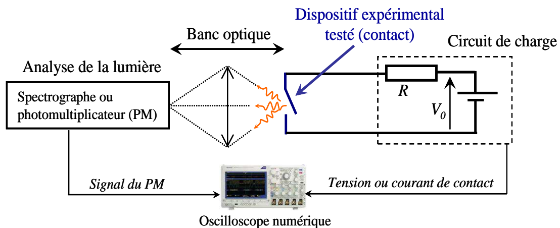
Figure 75 : Schéma de principe des expériences réalisées
