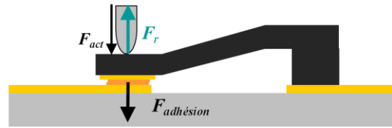
Figure 155 : Scénario proposé expliquant les rebonds de contact aux faibles vitesses d'actionnement
