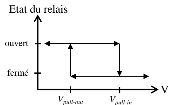
Figure 7 : Etat du relais en fonction de la tension d'actionnement
