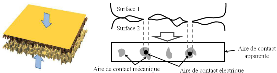
Figure 8 : Illustration des aires de contact apparente, mécanique et électrique [Duv11]
