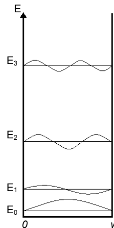
Figure 50 : Représentation de la fonction d'onde des électrons dans un puits de potentiel infini
