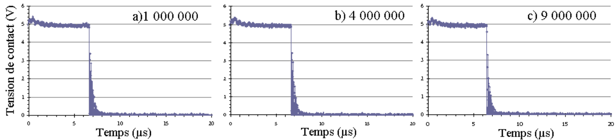
Figure 141 : Evolution de la tension de contact à la fermeture d'un relais Omron-2 pour a) 10^6 , b) 4 \cdot 10^6 et c) 5 \cdot 10^6 cycles ( f=10\text{Hz} )
