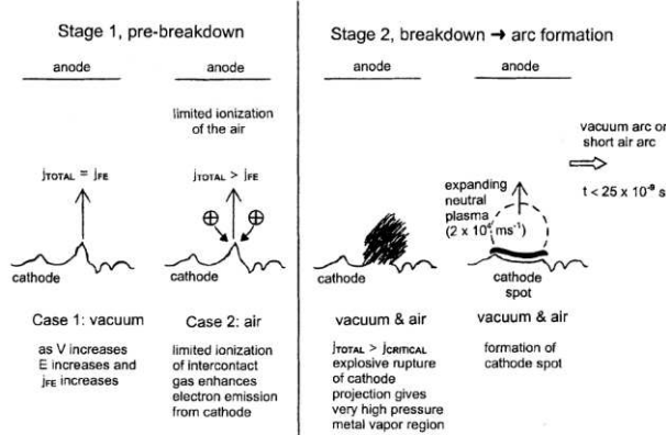
Figure 33 : Mécanisme de claquage pour un gap <4μm dans l'air ou <500μm dans le vide [Slade02]
