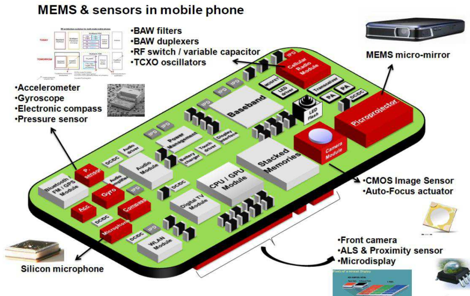
Figure 3 : Composants MEMS dans un téléphone mobile [Perk12]
