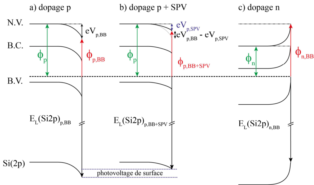
Figure V-18 : Diagramme d'énergie schématique présentant a) une forte courbure de bande dans le cas d'une surface dopée p et b) une compensation par un photovoltage de surface. c) représente un diagramme de bande d'un dopage n avec une courbure de bande importante amenant à un travail de sortie de type p.
