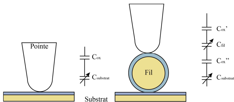
Figure II-32 : Représentation schématique d'une mesure SCM sur un substrat plan oxydé et sur un fil oxydé déposé sur substrat oxydé et équivalence électrique. Les parties oxydées sont représentées en bleu.
