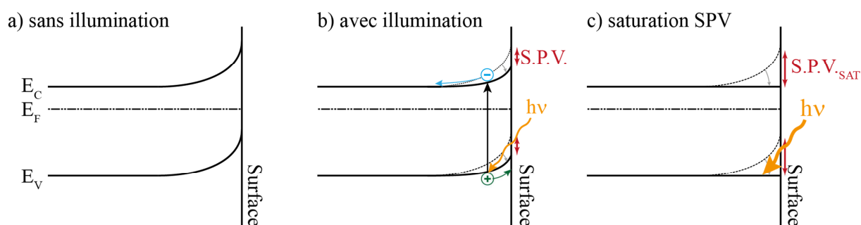
Figure II-8 : Diagramme de bande schématique illustrant l'effet du photovoltage de surface. a) courbure de bande dans un semiconducteur de type n, b) absorption de photon amenant à l'aplatissement partiel de la courbe de bande, c) saturation du photovoltage de surface conduisant à la condition de bande plate.
