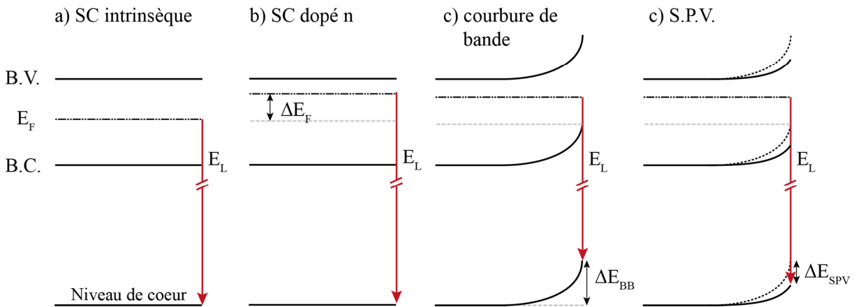
Figure II-7 : Diagramme schématique des différentes contributions influant sur l'énergie de liaison d'un niveau de cœur
