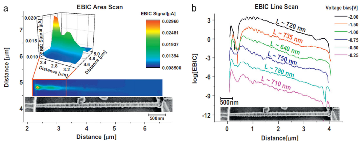
Figure I-18 : Mesure EBIC sur un nanofil de silicium p + -i [23] a) balayage EBIC de surface à un potentiel de -0,5 V, b) profils EBIC le long du fil (translation verticale des courbes pour meilleure lecture).
