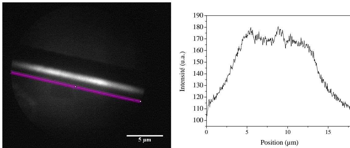
Figure IV-27 : Image XPEEM au seuil de photoémission à h\nu=161 eV du fil A-1 à E-E_F=7,2 eV et profil d'intensité au niveau de ligne rouge.
