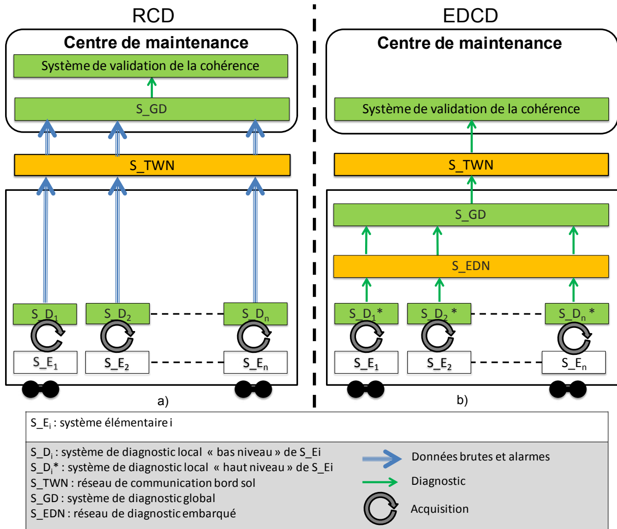
Figure 12 : Détail sur les architectures RCD et EDCD dans le transport ferroviaire
