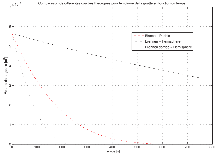
FIGURE 5.3 – Comparaison du volume de la goutte en fonction du temps pour différentes courbes théoriques proposées par Brennen [Brennen 05] (forme hémisphérique) et Bianca (et co-auteurs) [Bianca 03] (forme cylindrique).
