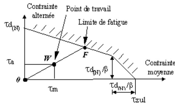
Figure III-54 : diagramme de Haigh
