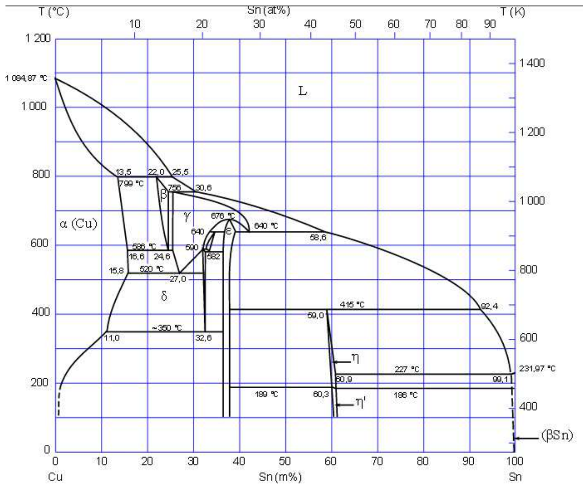
Figure II-10 : Diagramme de phase cuivre/étain (Cu/Sn) [JOH01]
