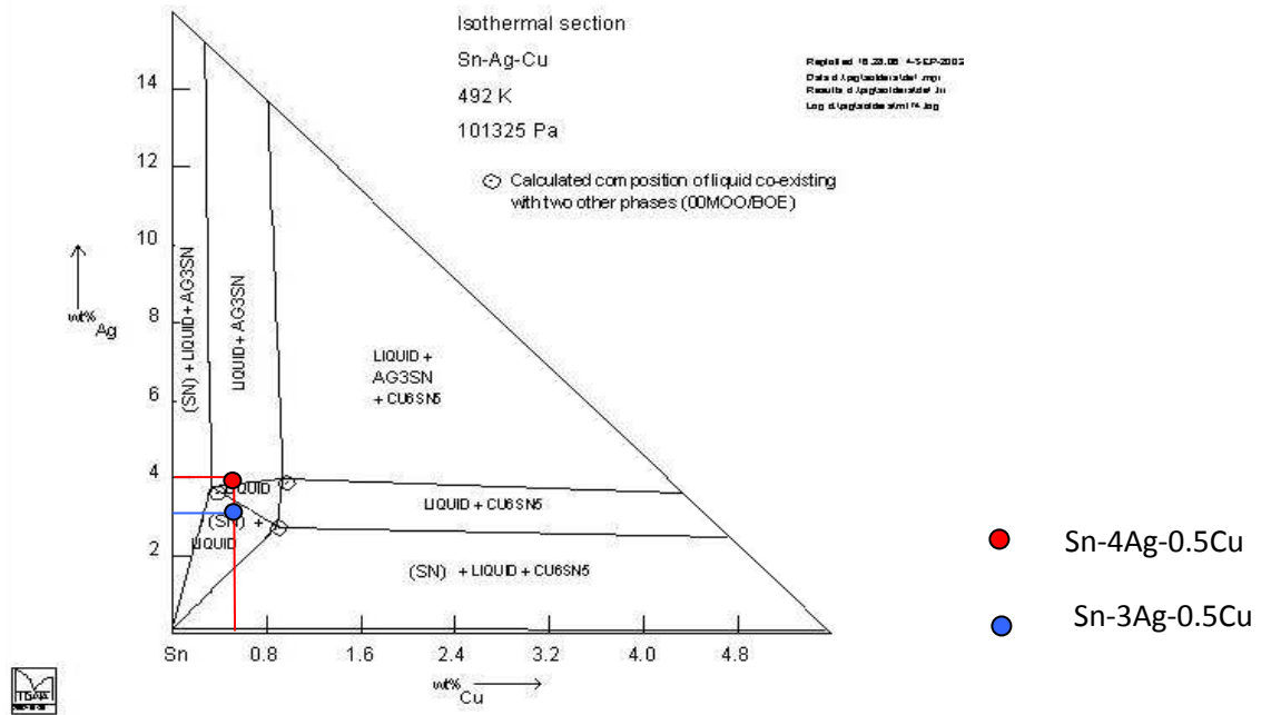
Figure I-11 : Section isotherme du diagramme ternaire à 219°C [SCH01]
