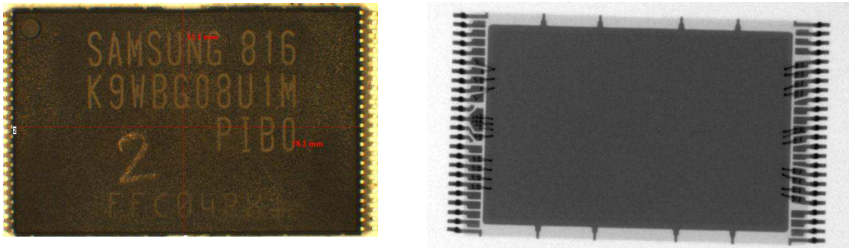
Figure IV-26 : Vue générale et vue RX d'un TSOP 48 type 1
