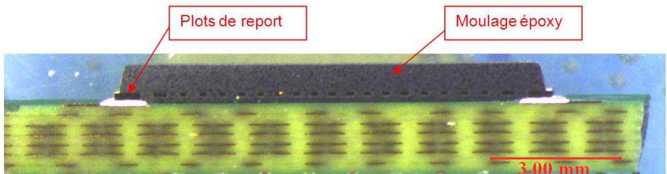
Figure III-52 : vue en coupe d'un QFN 68
