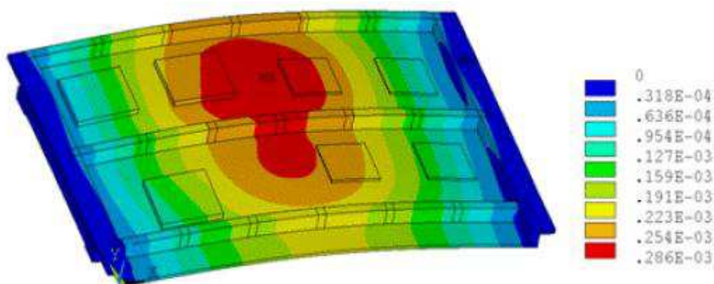
Figure III-45 : déformation de la carte soumise à des vibrations (GPa)
