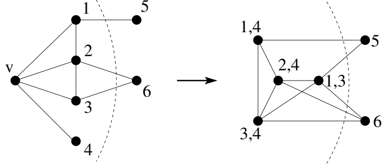
FIGURE 5.2: Exemple de pliage généralisé pour le sommet v , dont le voisinage contient un anti-triangle (1-3-4). Le sous-graphe induit à droite des pointillés est invariant. (5-6) est un indépendant maximum dans le graphe modifié, ce qui donne (v-5-6) comme un indépendant maximum pour le graphe initial.
