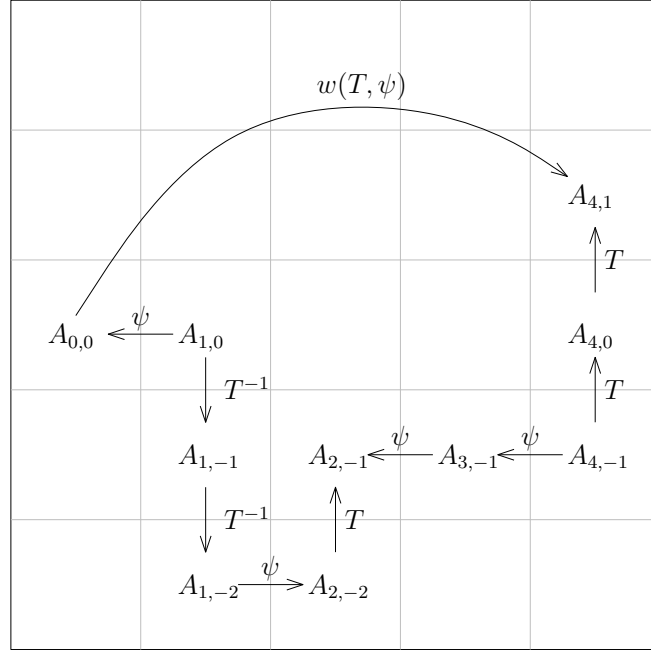
FIGURE 1. La construction de \psi pour w = t^2u^{-2}tut^{-2}u^{-1}
