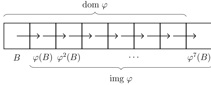
FIGURE 2. Une échelle \varphi de hauteur 8
