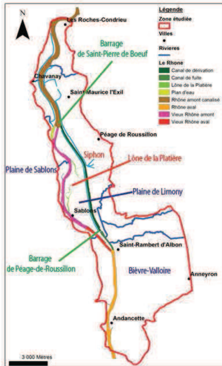
Figure 3: Schéma de la zone d'étude - Principales entités hydrauliques.
