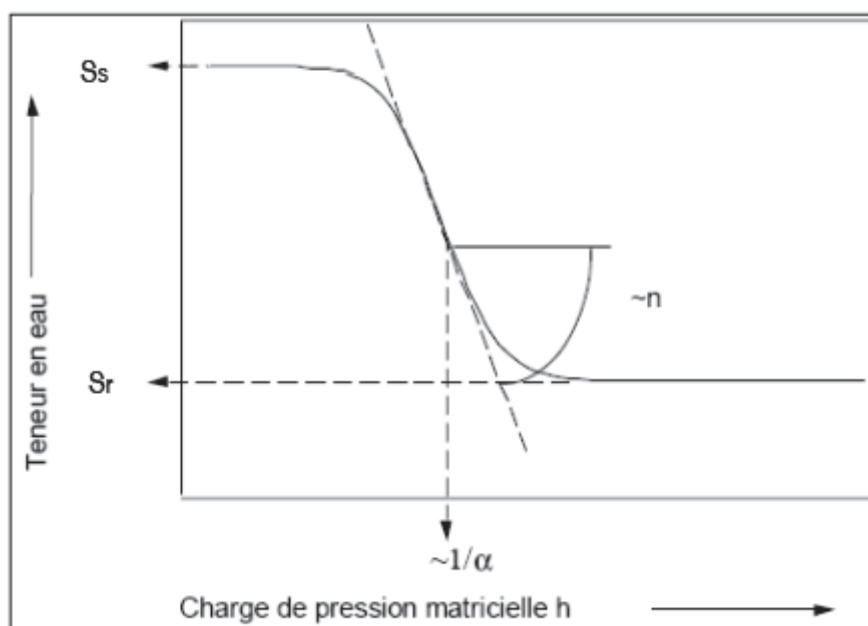
Figure 79 : Teneur en eau en fonction de la pression capillaire - Tirée de Ghoulil (2009), modifiée.
