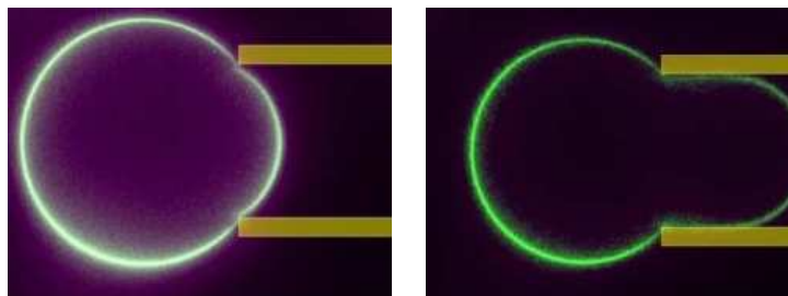
FIGURE 1.11 – Mesure d’excès d’aire par aspiration d’une vésicule unilamellaire par micropipette, observée en microscopie de fluorescence (issu de [42]).
