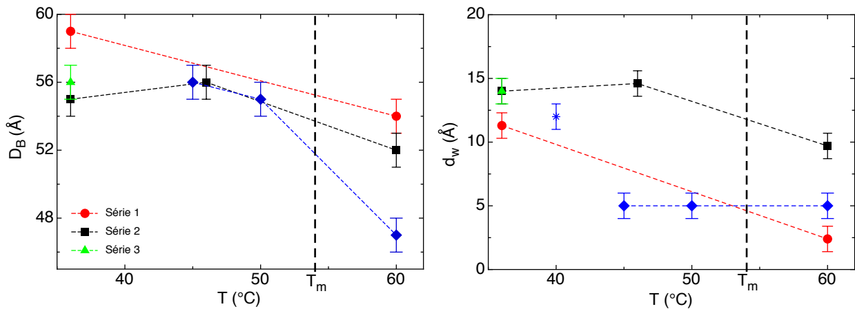
FIGURE 1.9 – A gauche : épaisseur de la bicouche flottante D_B en fonction de la température. ( \diamond ) et ( \star ) : résultats obtenus par réflectivité de neutrons respectivement par Rondelli et al. (non publiés) et Malaquin et al. [11]. A droite : épaisseur d'eau inter-bicouche d_w en fonction de la température. Les lignes sont des guides pour les yeux.
