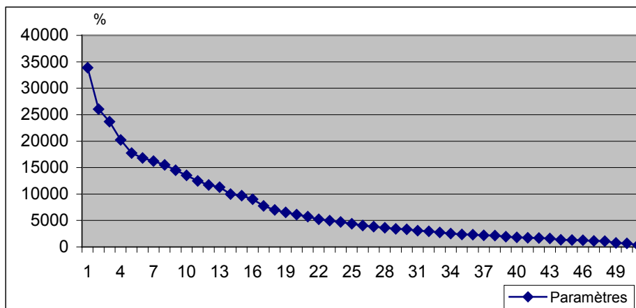
Figure 29 : Valeurs propres des vecteurs des 51 caractéristiques basées sur MFCCs
