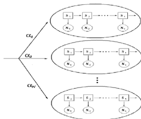
Figure 8 : Mélange des HMMs [Fernandez et al, 2003]
