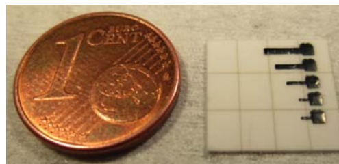
b) Poutres sérigraphiées en epoxy chargé au carbone de taille 1mmx220 \mu\text{m} x40 \mu\text{m} pour les plus petites
