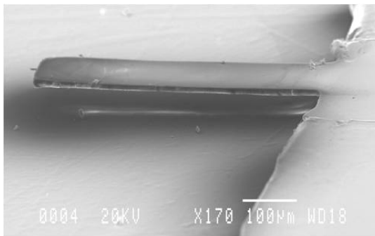
a) Poutre en SU8 de taille 400x100x5 \mu\text{m}^3
