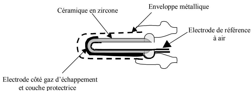
Figure III.18 : Coupe schématique d'une sonde lambda.
