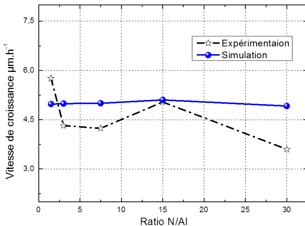
Figure 1 : évolution de la vitesse de croissance des couches d'AlN en fonction du ratio N/Al.
