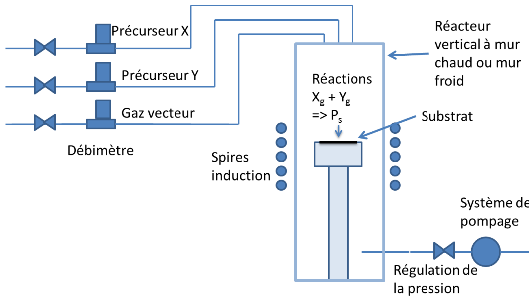
Figure 1. 17: représentation d'un réacteur CVD.
