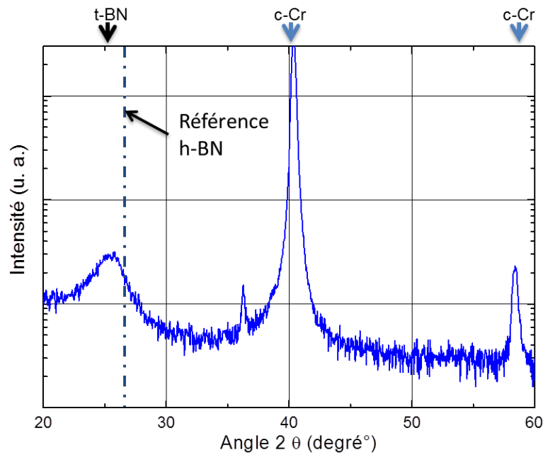
Figure 4.17 : spectre XRD incidence rasante de l'échantillon BN-51.
