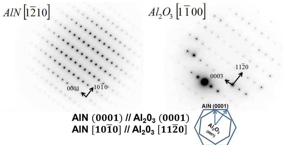
Figure 3.20 : cliché de diffraction MET de l'échantillon AIN-12.
