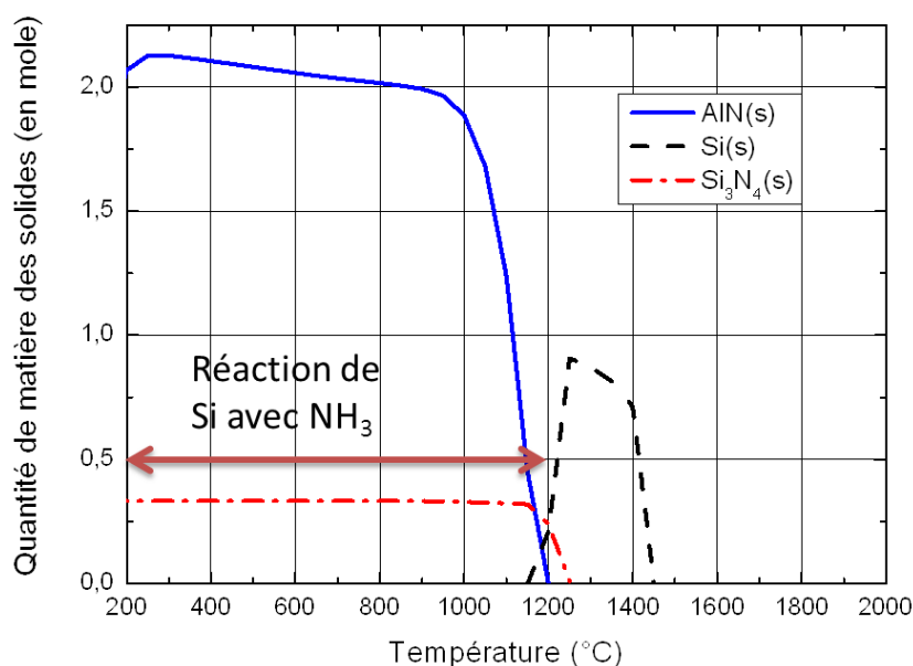
Figure 2.6 : équilibre thermodynamique du système \text{H}_2(\text{g})/\text{AlCl}_3(\text{g})/\text{NH}_3(\text{g})/\text{Si}(\text{s}) (quantité 1000/2.31/3.5/1 moles).
