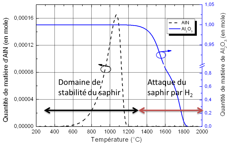
Figure 2.5 : équilibre thermodynamique du système H_2(g)/Al_2O_3(s)/NH_3(g) (quantité 1000/1/3.5 moles).
