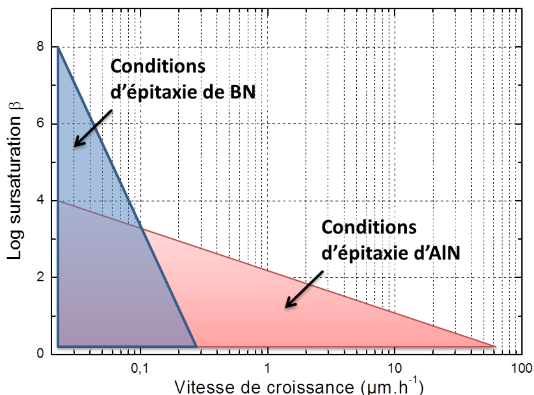
Figure 5.12 : Conditions d'épitaxie d'AlN et de BN observées expérimentalement
