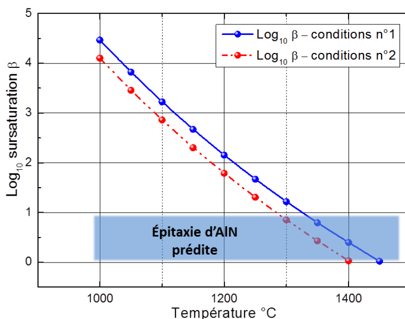
Figure 2.17 : \log_{10} de la sursaturation \beta de la croissance d'AlN calculée à une pression de 1333 Pa.
