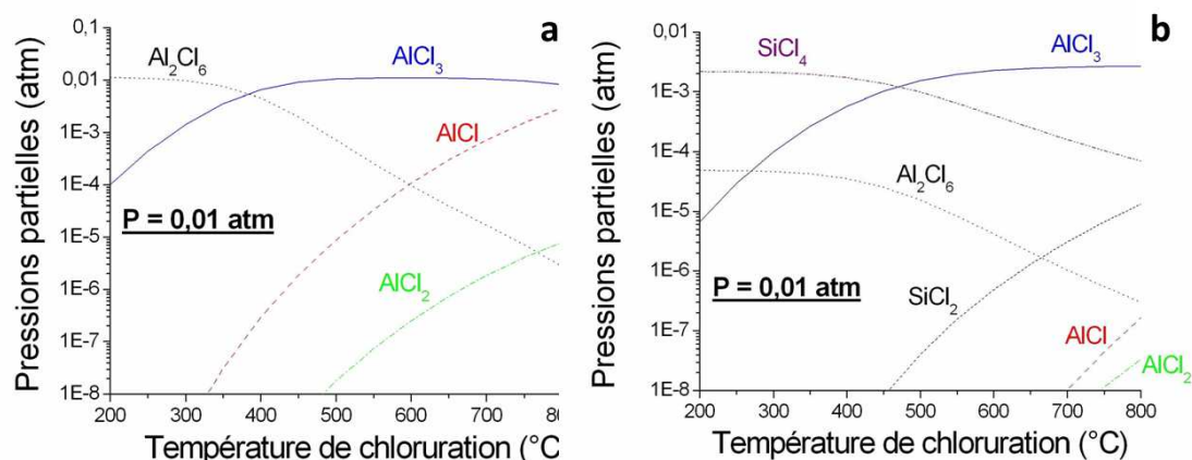
Figure 2.2 : simulation thermodynamique, a) de l'étape de chloruration d'Al(s) par \text{Cl}_2 , b) de la réaction entre \text{AlCl}_3 et \text{SiO}_2 [10].
