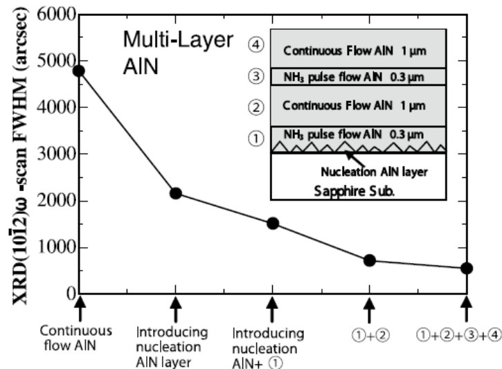
Figure 1.27: évolution de la FWHM de la raie (10-12) de w-AlN en fonction de l'empilement des couches réalisées par un apport continu et séquencée en ammoniac à la surface du substrat saphir [147].
