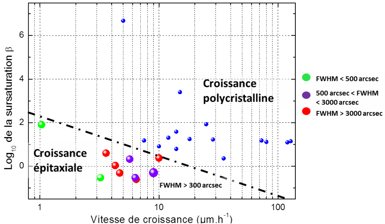
Figure 5.5: Comparaison entre la vitesse de croissance et la sursaturation \beta de la phase gazeuse pour le dépôt de couche épitaxiales (large sphères pleines) et polycristallines (petite sphères pleines).
