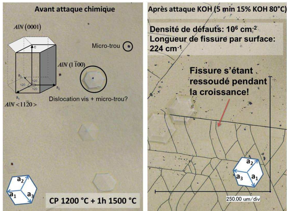
Figure 3.19 : image réalisée au microscope optique de l'échantillon AIN-12 avant et après attaque chimique basique.
