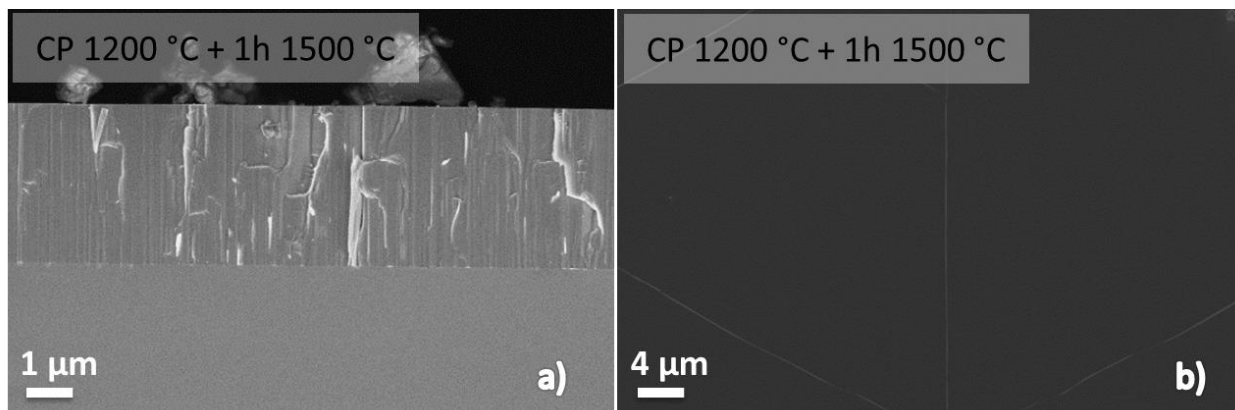
Figure 3.13 : Image MEB FEG de la coupe transversale et de la surface de l'échantillon AlN-12.
