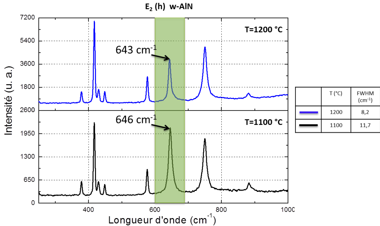
Figure 3.12 : spectre Raman des échantillons AlN-12 et AlN-37.
