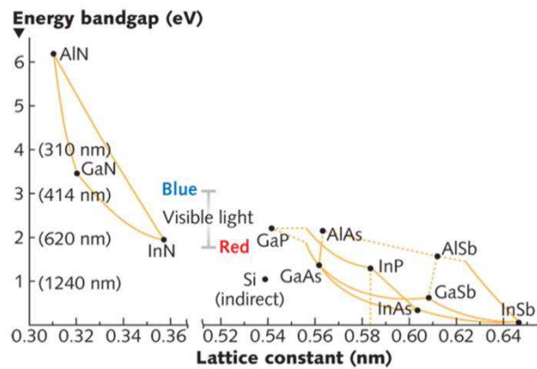
Figure 1.1 : valeur de bande interdite des nitrures III/V en fonction du paramètre de maille a [5].
