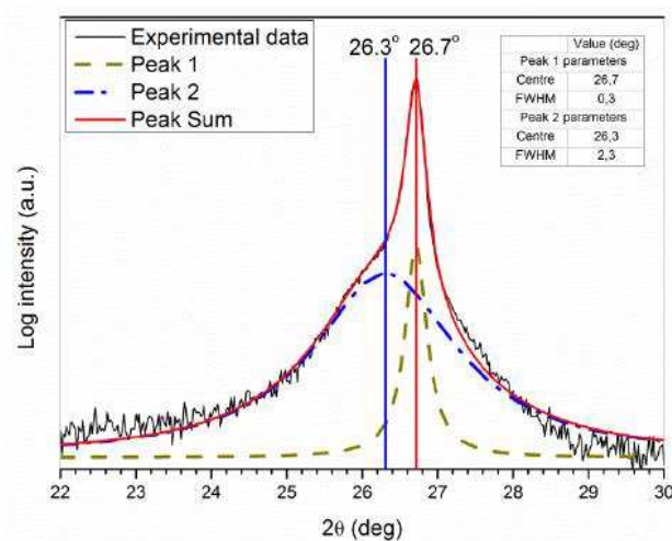
Figure 1.25: spectre XRD en mode Bragg-Brentano autour du pic (0002) de r-BN (courbe noir). En bleu et en vert, les déconvolutions du signal visant à faire apparaître la contribution des phases turbostratique et rhomboédrique de BN [18].
