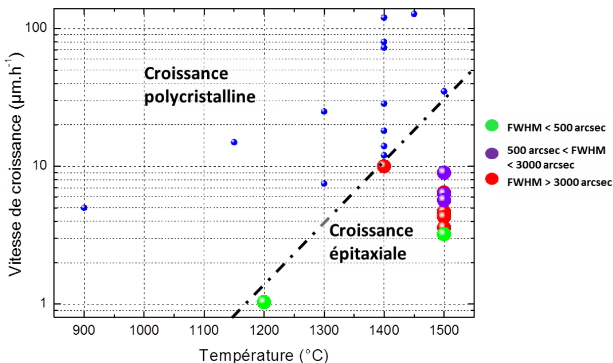
Figure 5.4 : Comparaison entre la température et la vitesse de croissance pour le dépôt de couche épitaxiales (large sphères pleines) et polycristalline (petite sphères pleines).
