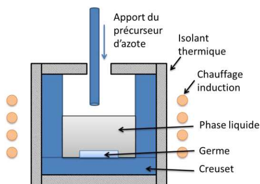
Figure 1.11 : schéma type d'un réacteur d'építaxie phase liquide pour nitrures III/V avec chauffage induction.
