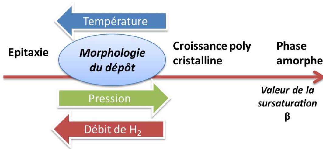
Figure 2.15 : effets de la température, de la pression et du débit de H_2 injectés dans le réacteur sur la sursaturation de phase gazeuse lors de la croissance de l'AlN.
