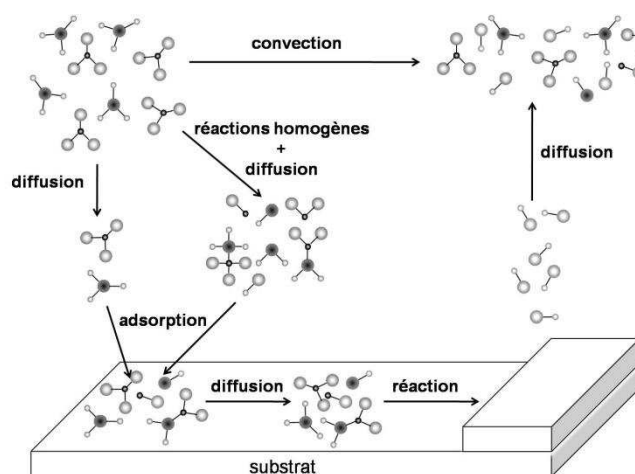
Figure 1.18: Mécanismes physico-chimique d'une croissance par CVD [11].
