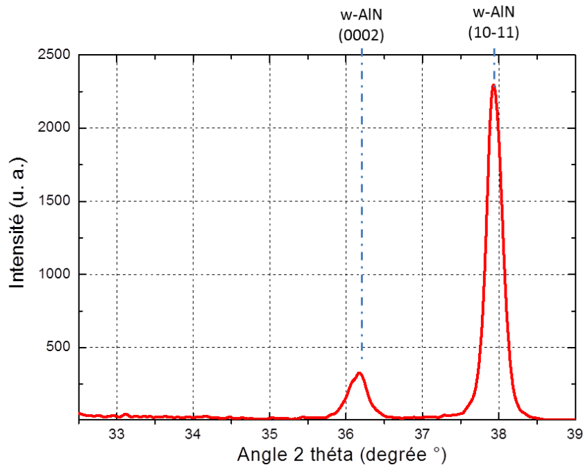
Figure 3.23 : spectre XRD de l'échantillon AlN-Si-03.
