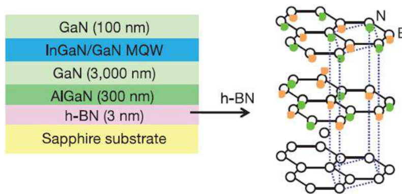
Figure 1.3 : schéma d'un dispositif LED III/V émettant dans la couleur bleu (434 nm) avec l'utilisation de BN hexagonal comme couche tampon [9].
