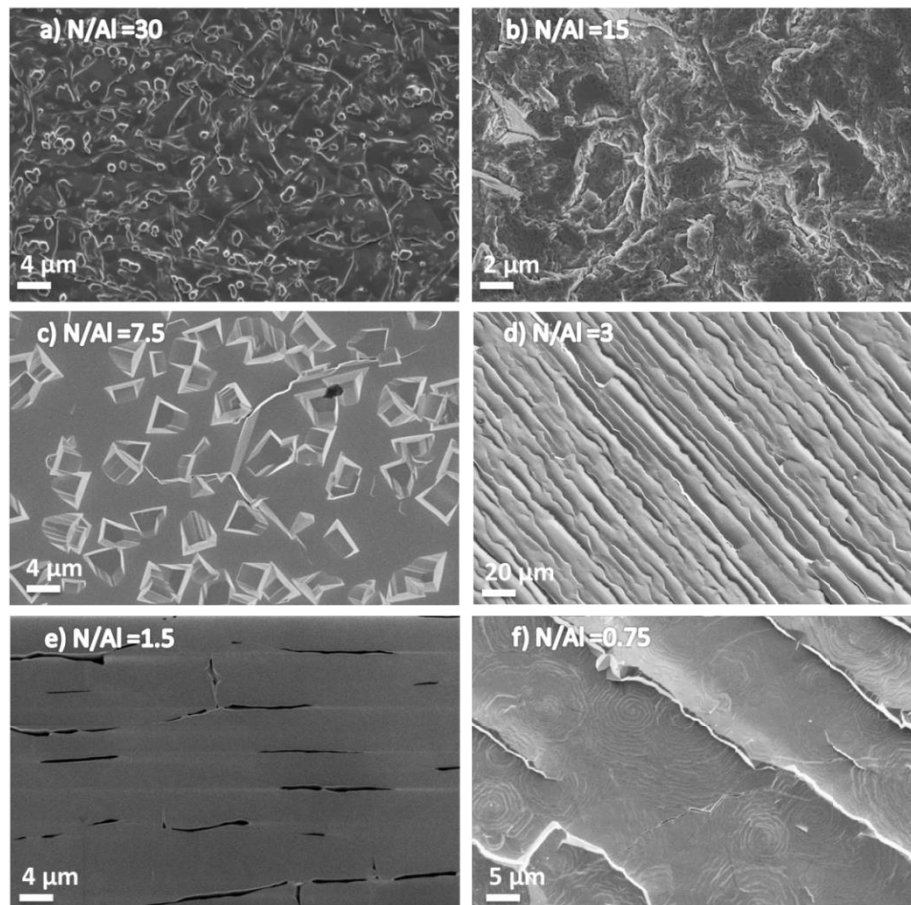
Figure 3.5 : image MEB FEG de la surface des échantillons a) AlN-03, b) AlN-04, c) AlN-05, d) AlN-06, e) AlN-07 et f) AlN-08 élaborés pour une température du substrat de 1500°C.
